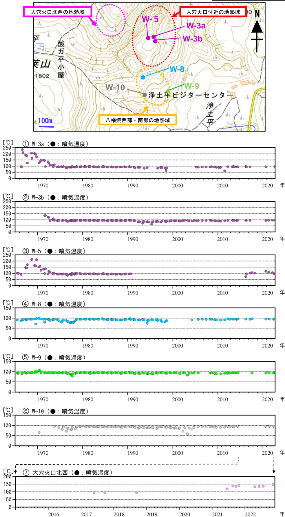
図13 吾妻山 大穴火口周辺の噴気温度の経過（1965年7月～2022年11月）
