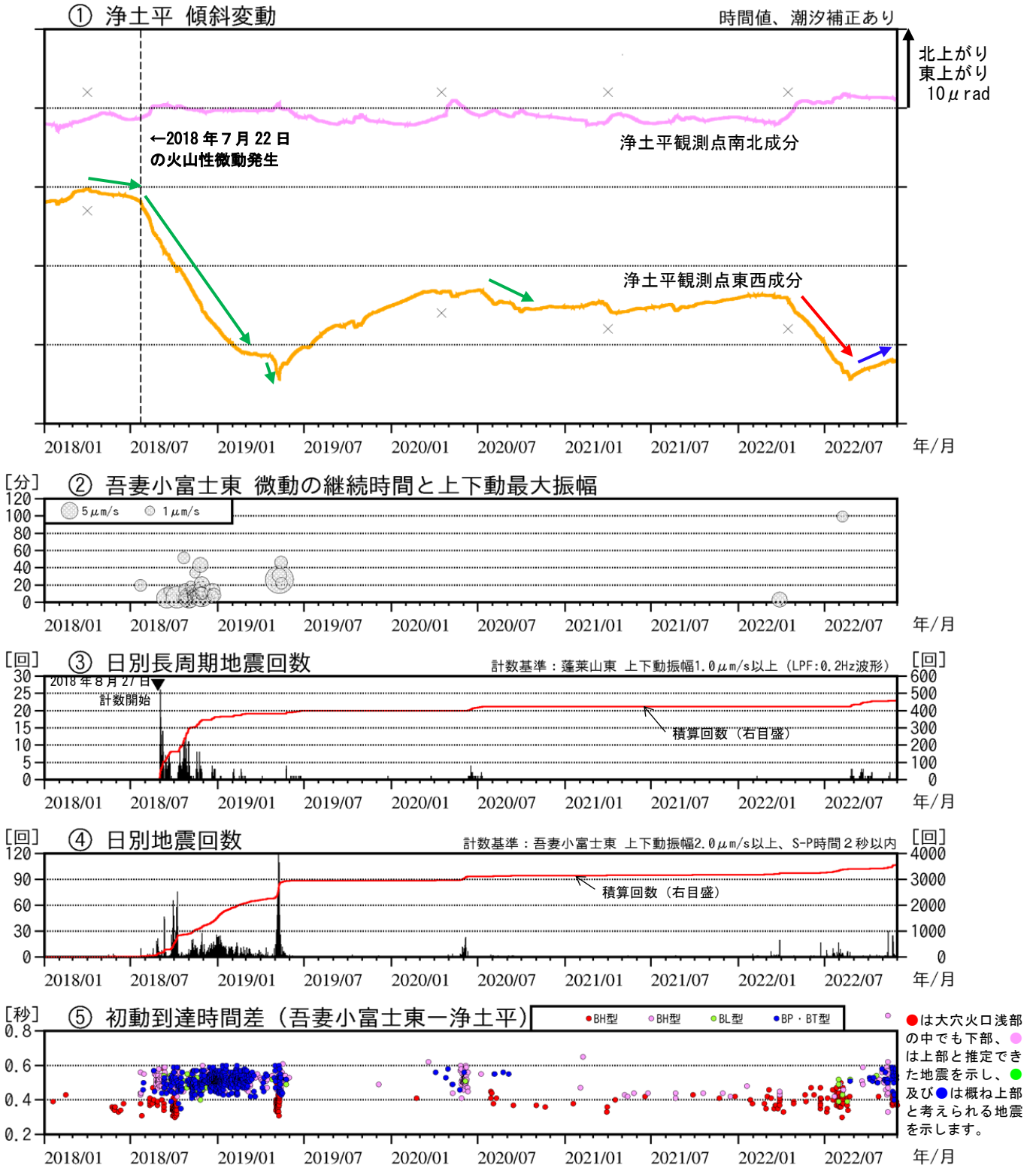
図3 吾妻山 火山活動経過図 (2018年1月～2022年11月)
