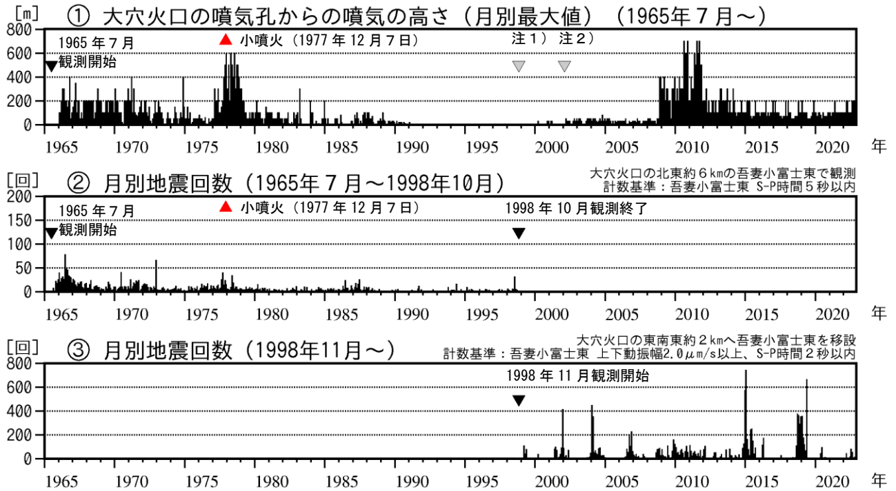
図1 吾妻山 長期的な火山活動の経過（1965年7月～2022年11月）
