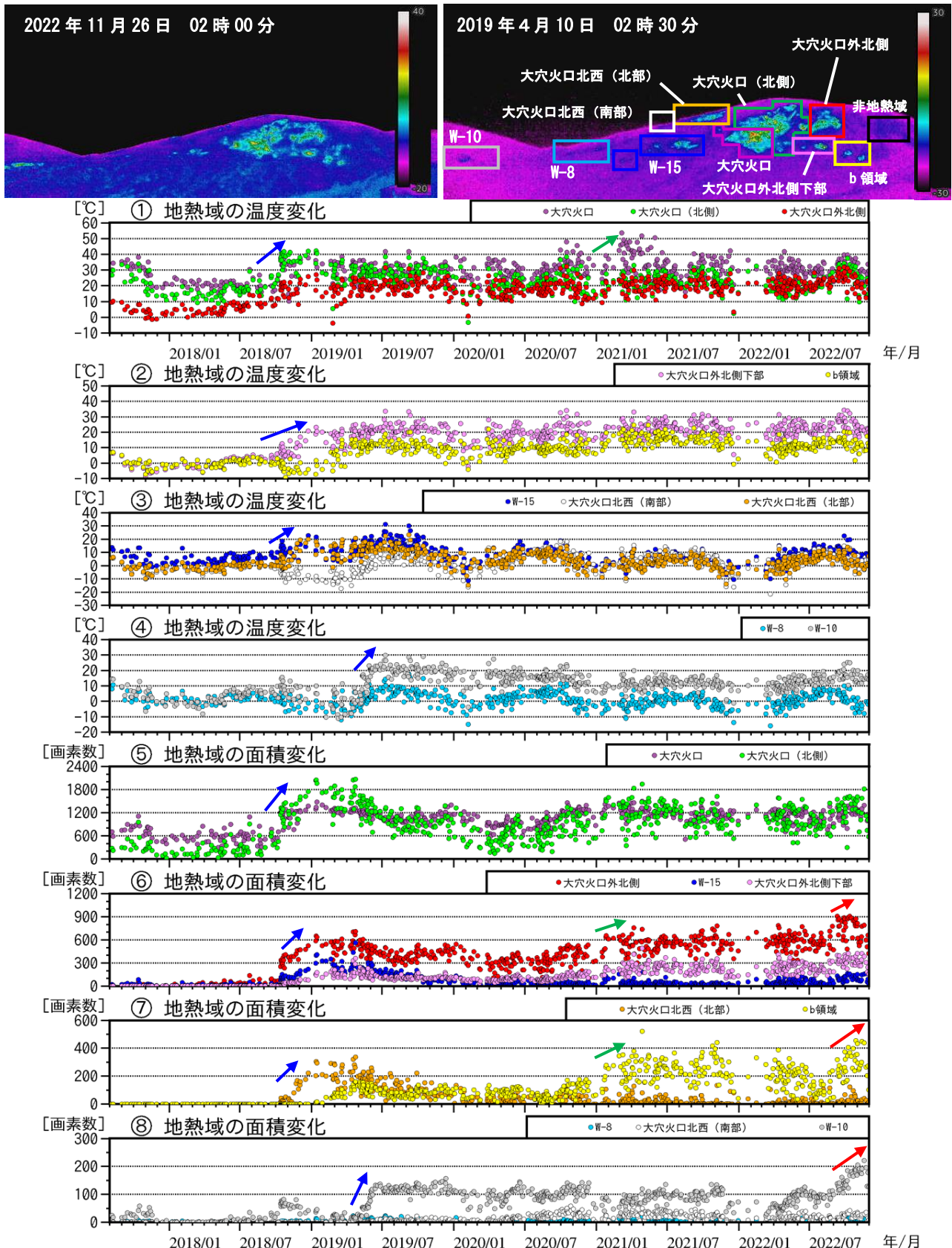
図7 吾妻山 監視カメラによる大穴火口周辺の地熱域の経過（2017年8月～2022年11月）
