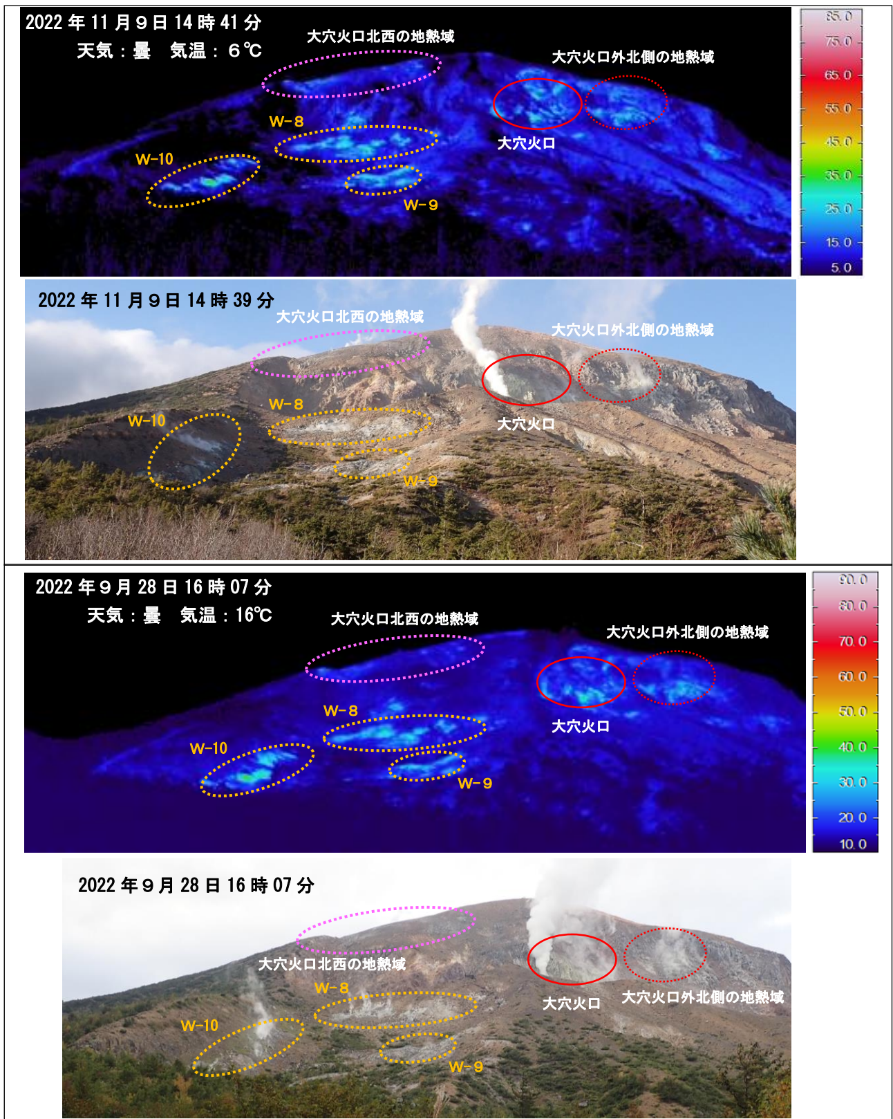
図12 吾妻山 大穴火口周辺及び八幡焼の状況（下）と地表面温度分布（上）
