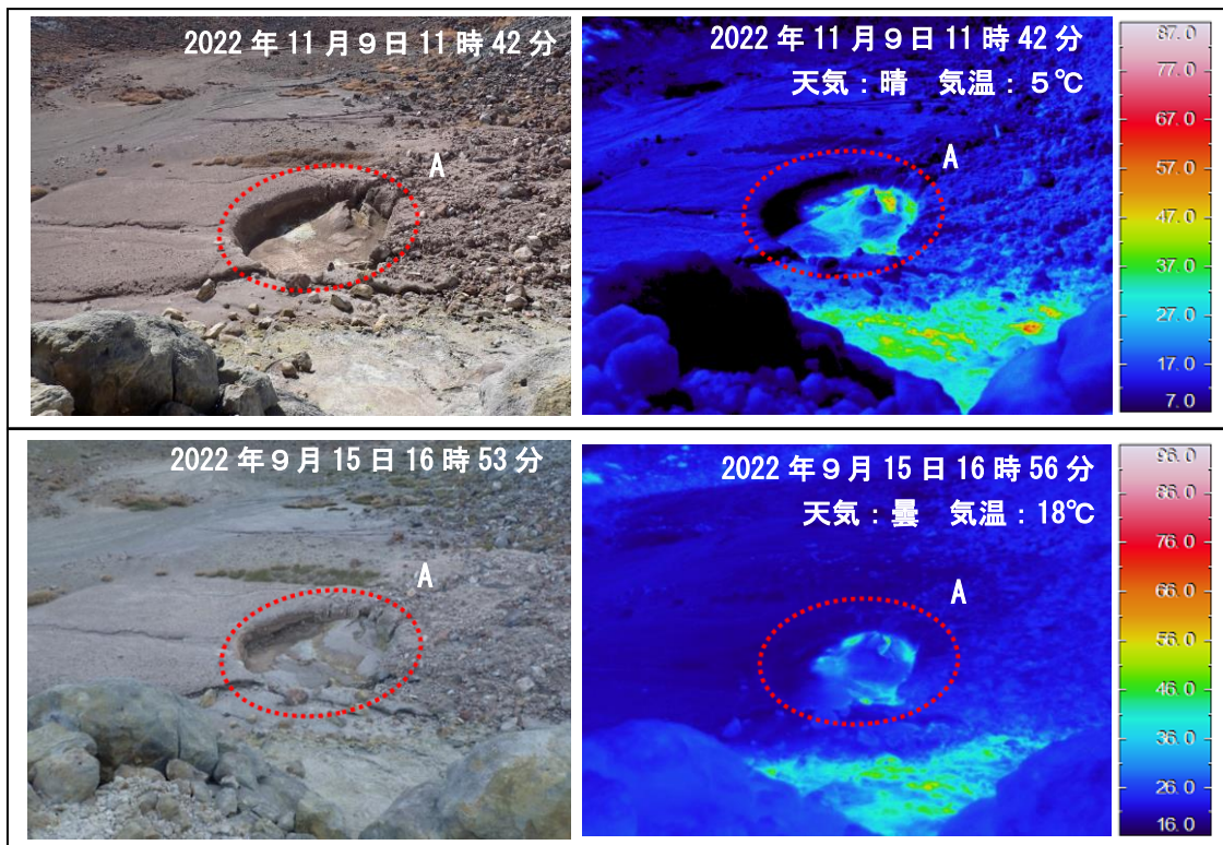
図 11 吾妻山 大穴火口内北側の陥没孔周辺の状況（左）と地表面温度分布（右）
