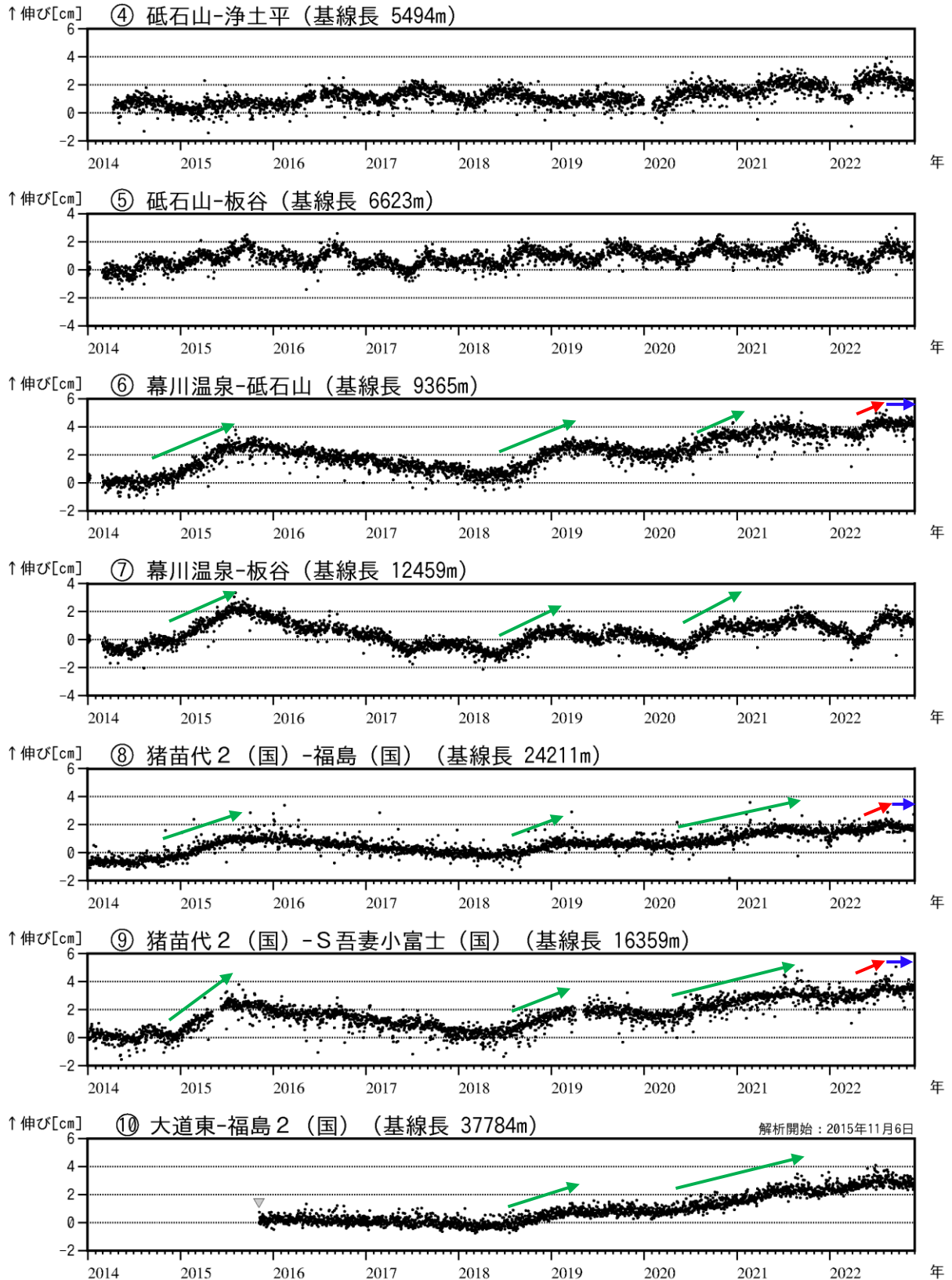
図6 吾妻山 吾妻山深部の地殻変動（2014年1月～2022年11月）
