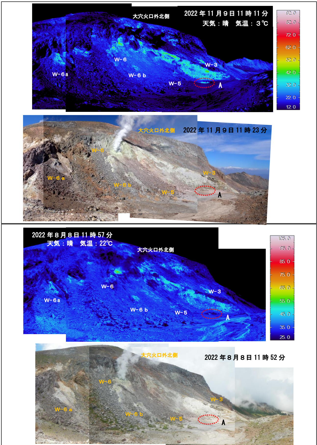
図10 吾妻山 大穴火口付近及びその周辺の状況（下）と地表面温度分布（上） ・噴気や雲のため、一部の地熱域が隠れています。
