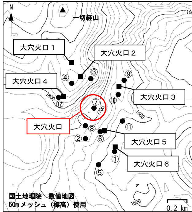
図 15 吾妻山 全磁力観測点配置図
