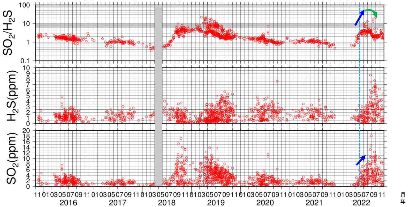
図14 吾妻山 火山ガス観測装置による観測（2015年11月～2022年11月）
