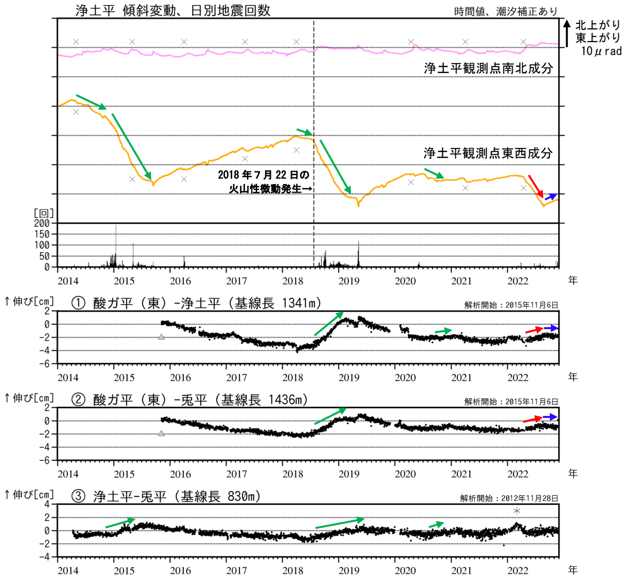
図5 吾妻山 大穴火口浅部の地殻変動（2014年1月～2022年11月）
