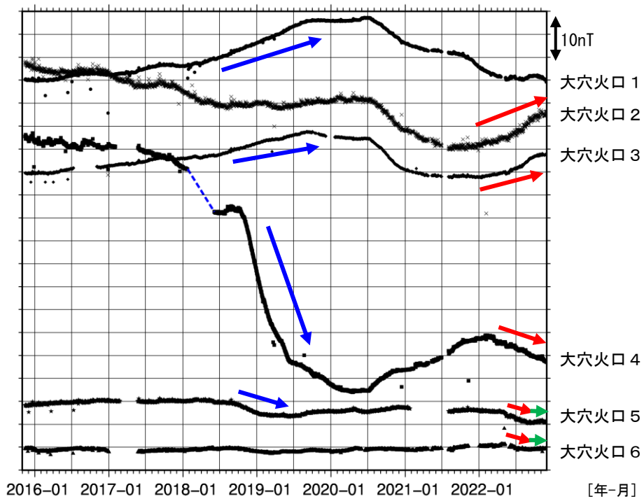
図 16 吾妻山 全磁力連続観測点の全磁力値変化 (2015年11月~2022年11月)
