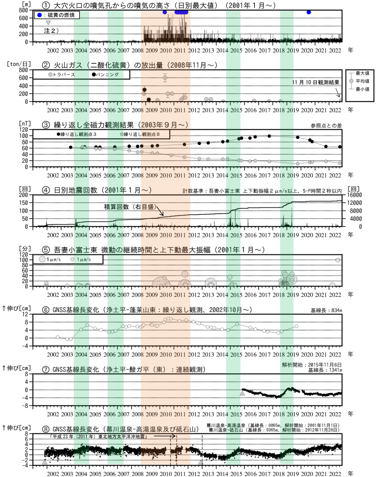
図2 吾妻山 中期的な火山活動の経過（2001年1月～2022年11月）
