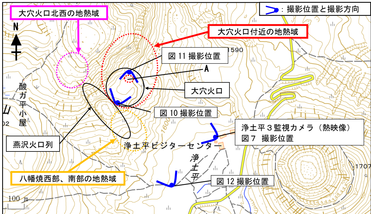
図9 吾妻山 大穴火口周辺の地熱域の分布及び熱映像撮影方向
