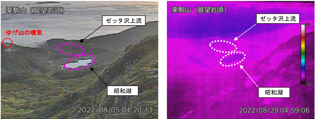
図2 栗駒山 昭和湖及びゼッタ沢上流周辺の状況（可視：8月5日、赤外：8月29日） ・展望岩頭監視カメラ（昭和湖の南南西約900m）の映像です。
