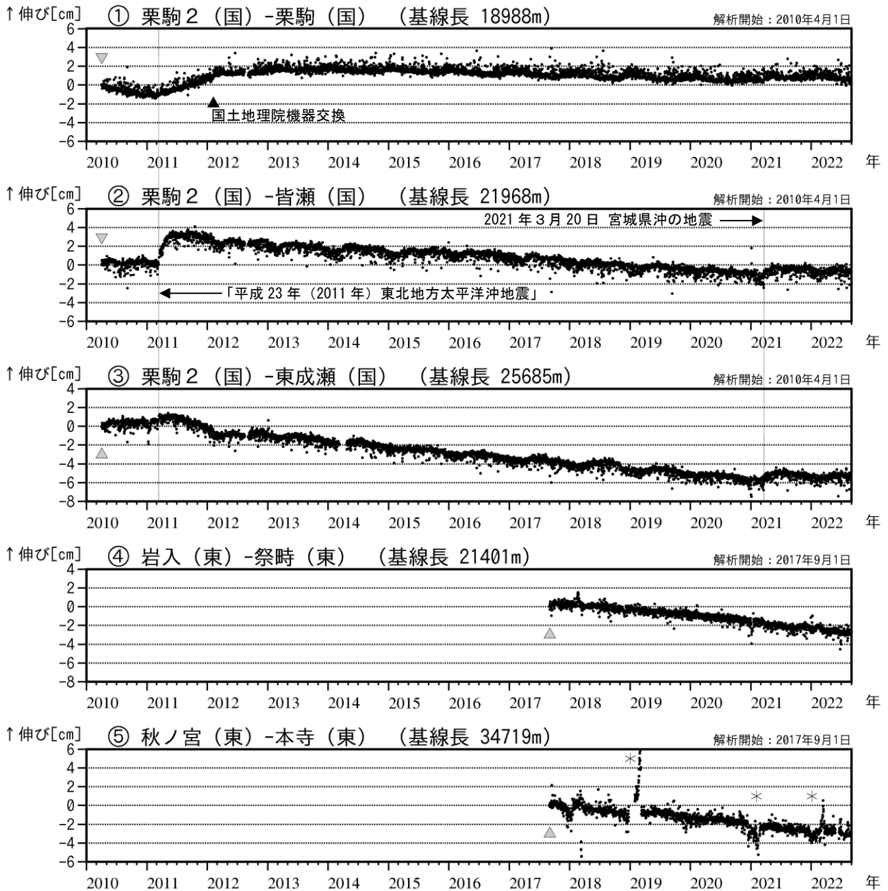
図7 栗駒山 GNSS 基線長変化図（2010年4月～2022年8月）
