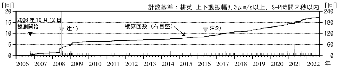
図6 栗駒山 日別地震回数（2006年10月～2022年8月）
