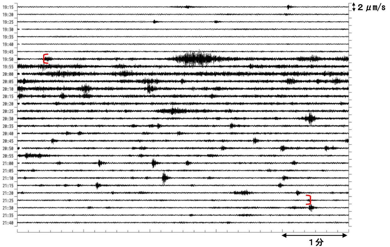
図4 吾妻山 吾妻小富士東観測点（上下成分）での火山性微動及び火山性地震の発生状況 （2022年8月7日19時15分～21時45分）
