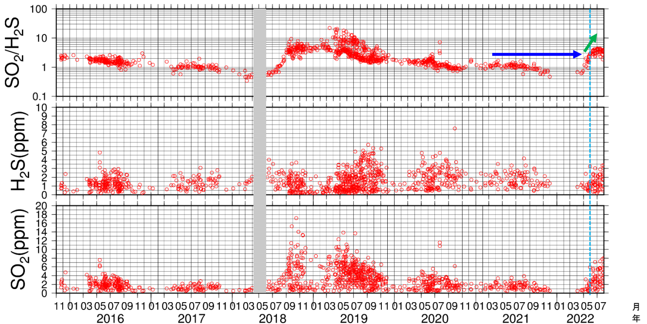
図17 吾妻山 火山ガス観測装置による観測（2015年11月～2022年7月）
