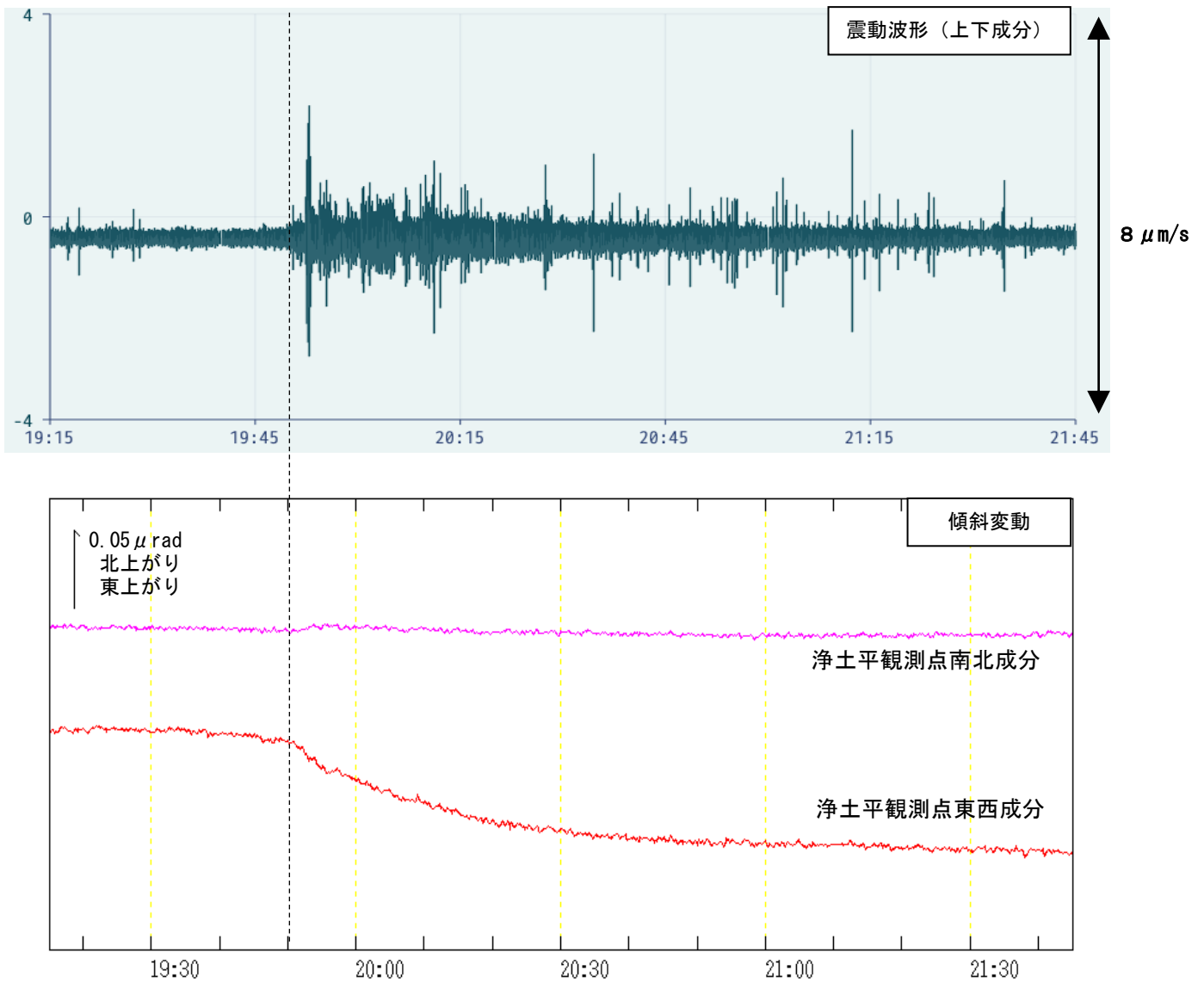
図5 吾妻山 吾妻小富士東観測点での震動波形及び浄土平観測点での傾斜変動 (2022年8月7日19時15分～21時45分)
