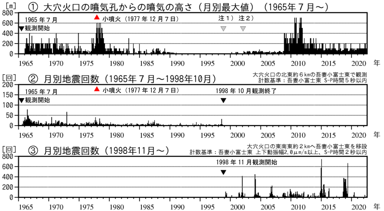
図1 吾妻山 長期的な火山活動の経過（1965年7月～2022年7月）
