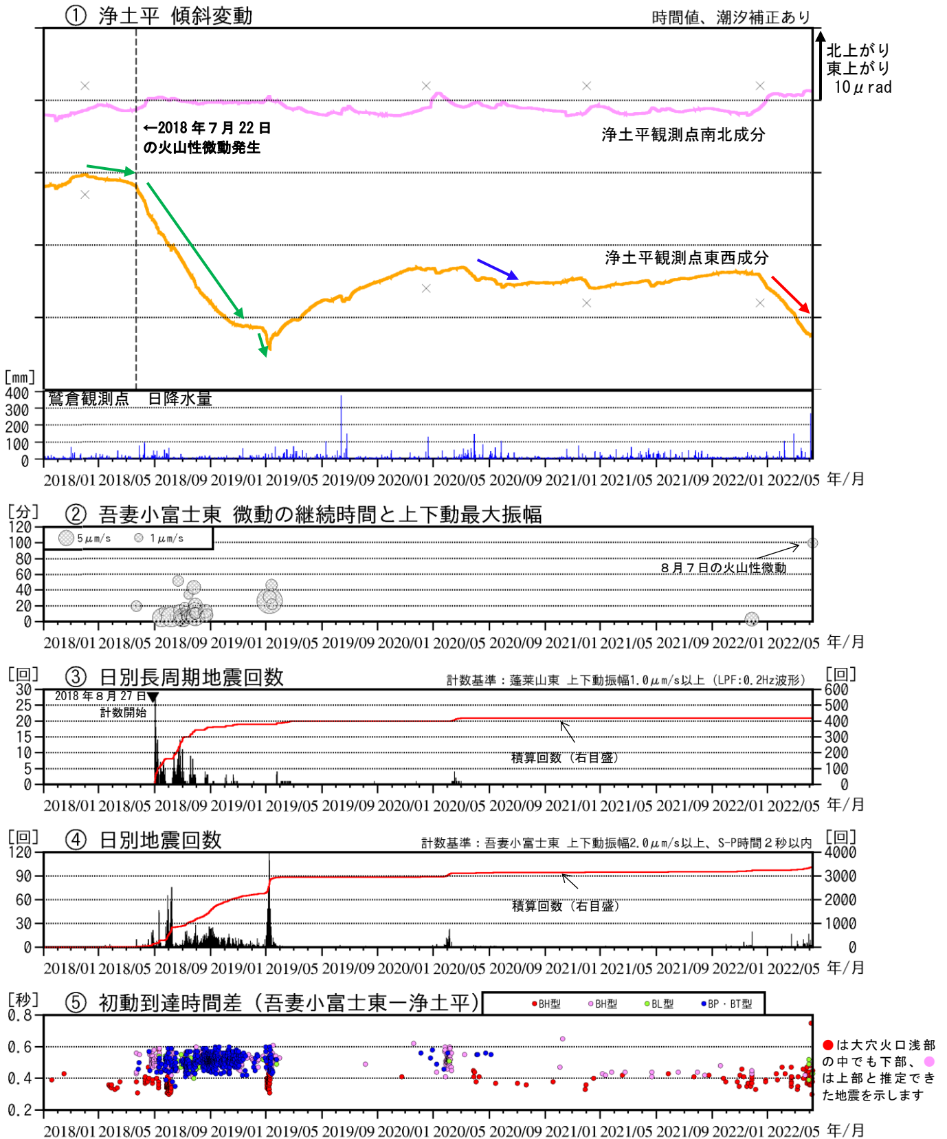
図3 吾妻山 火山活動経過図 (2018年1月~2022年8月7日、速報値含む)
