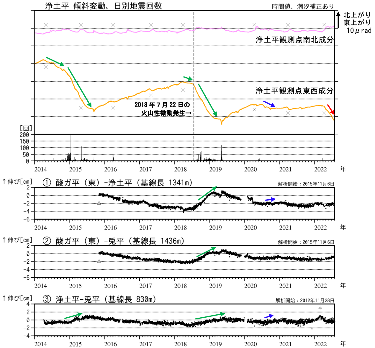
図7 吾妻山 大穴火口浅部の地殻変動（2014年1月～2022年7月）
