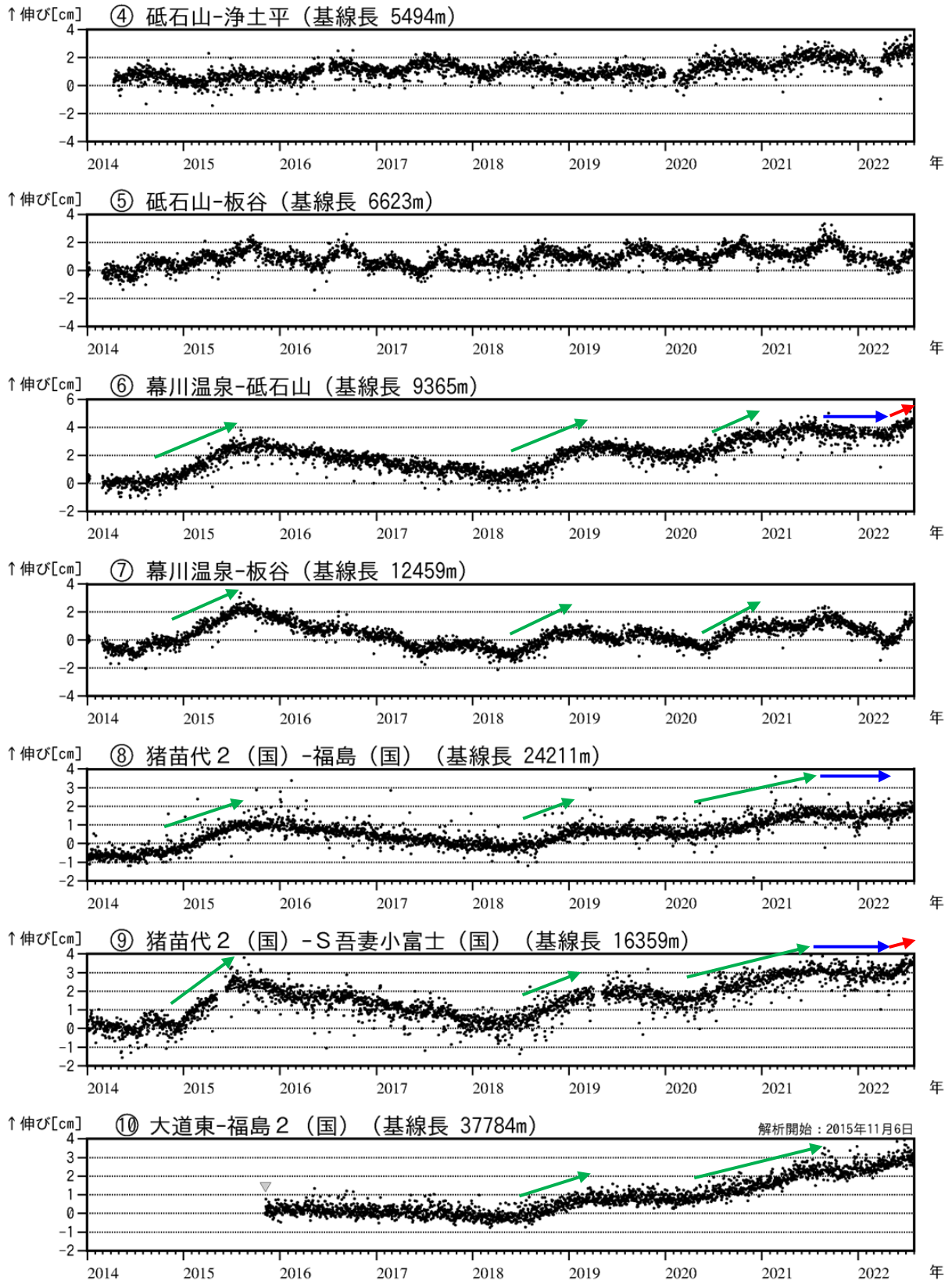
図8 吾妻山 吾妻山深部の地殻変動（2014年1月～2022年7月）
