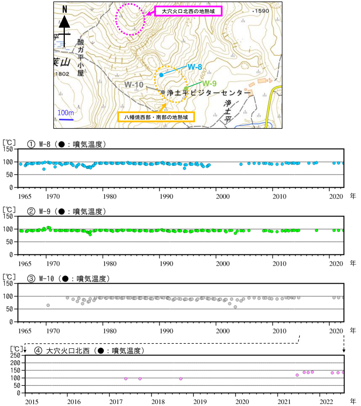
図16 吾妻山 大穴火口周辺の噴気温度の経過（1965年7月～2022年7月）
