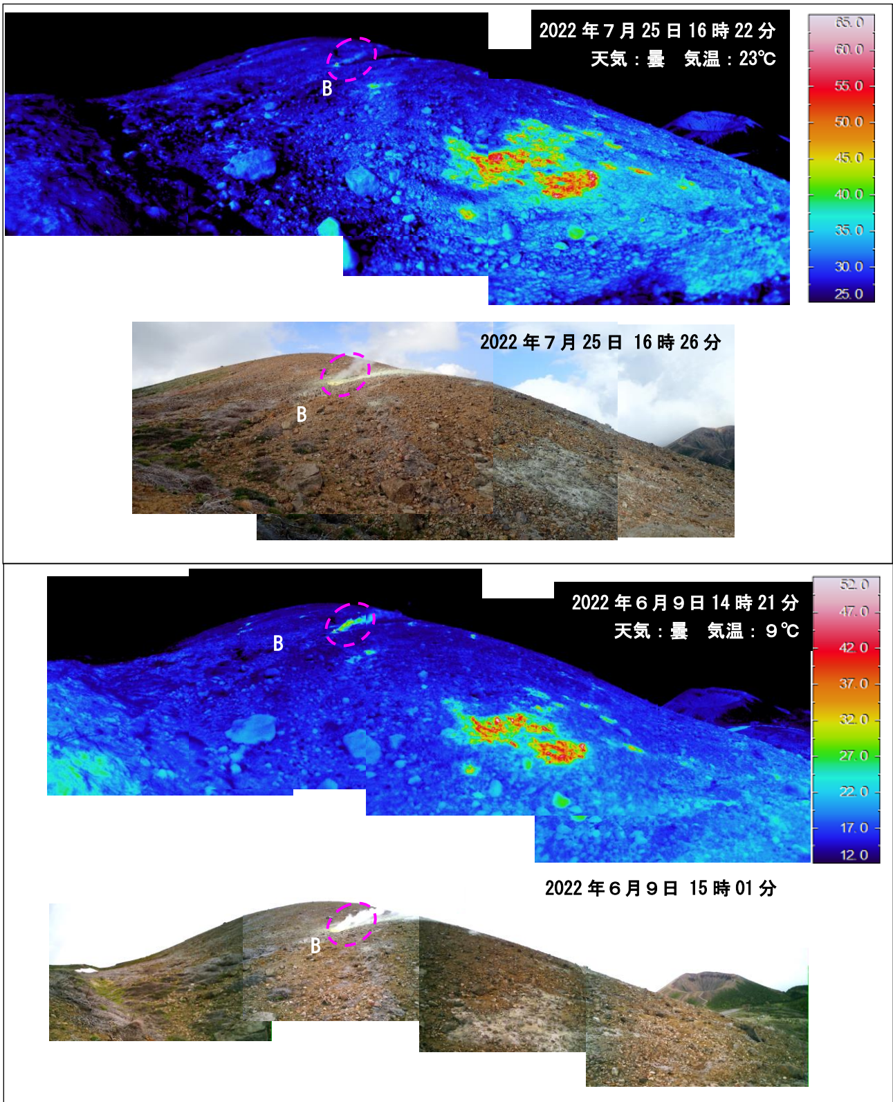
図14 吾妻山 大穴火口北西の状況（下）と地表面温度分布（上）
