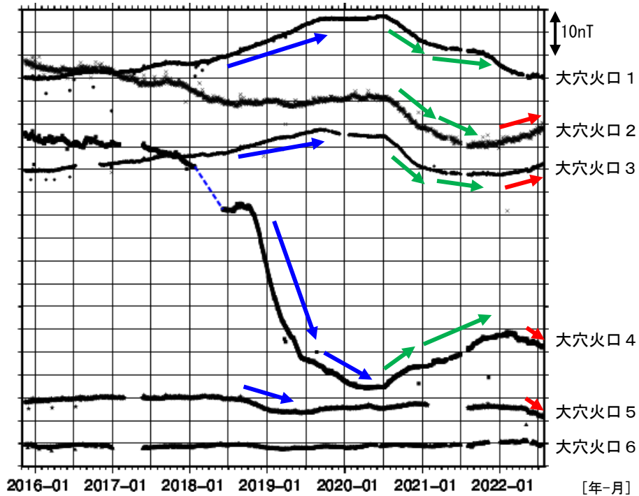
図19 吾妻山 全磁力連続観測点の全磁力値変化（2015年11月～2022年7月）
