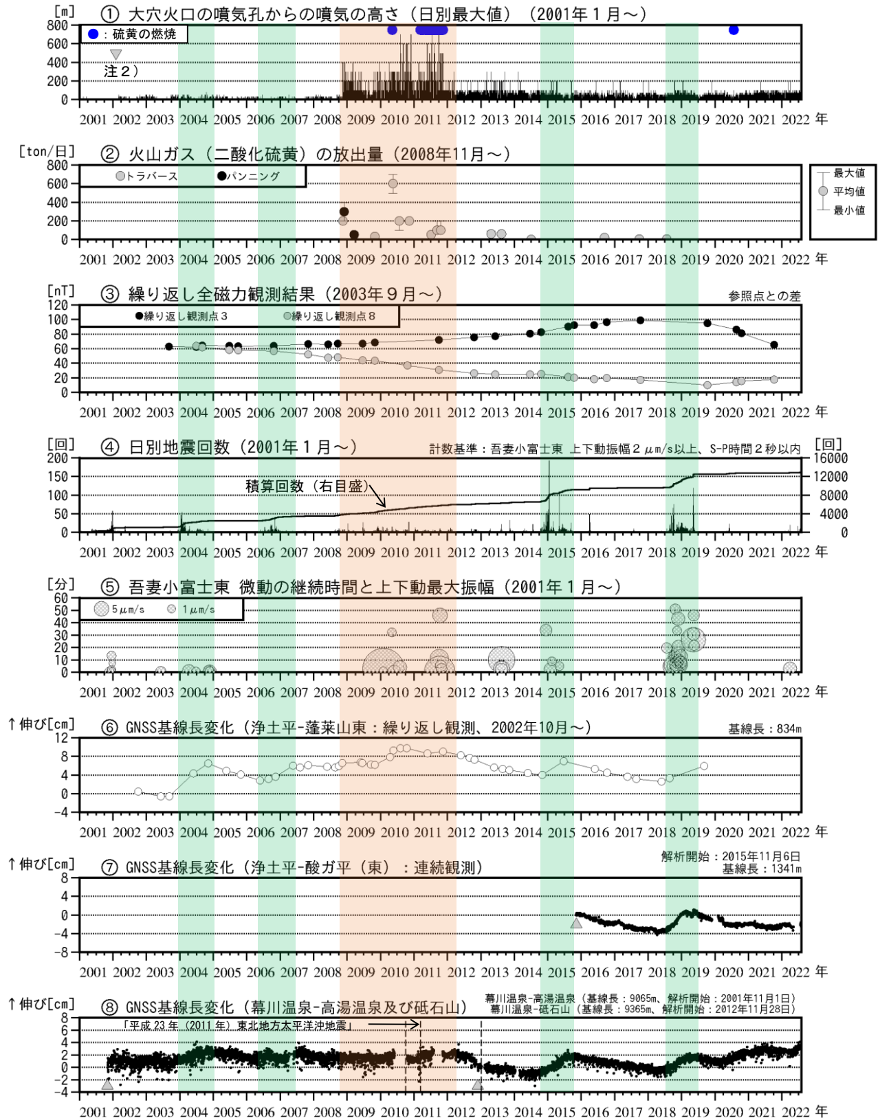
図2 吾妻山 中期的な火山活動の経過（2001年1月～2022年7月）
