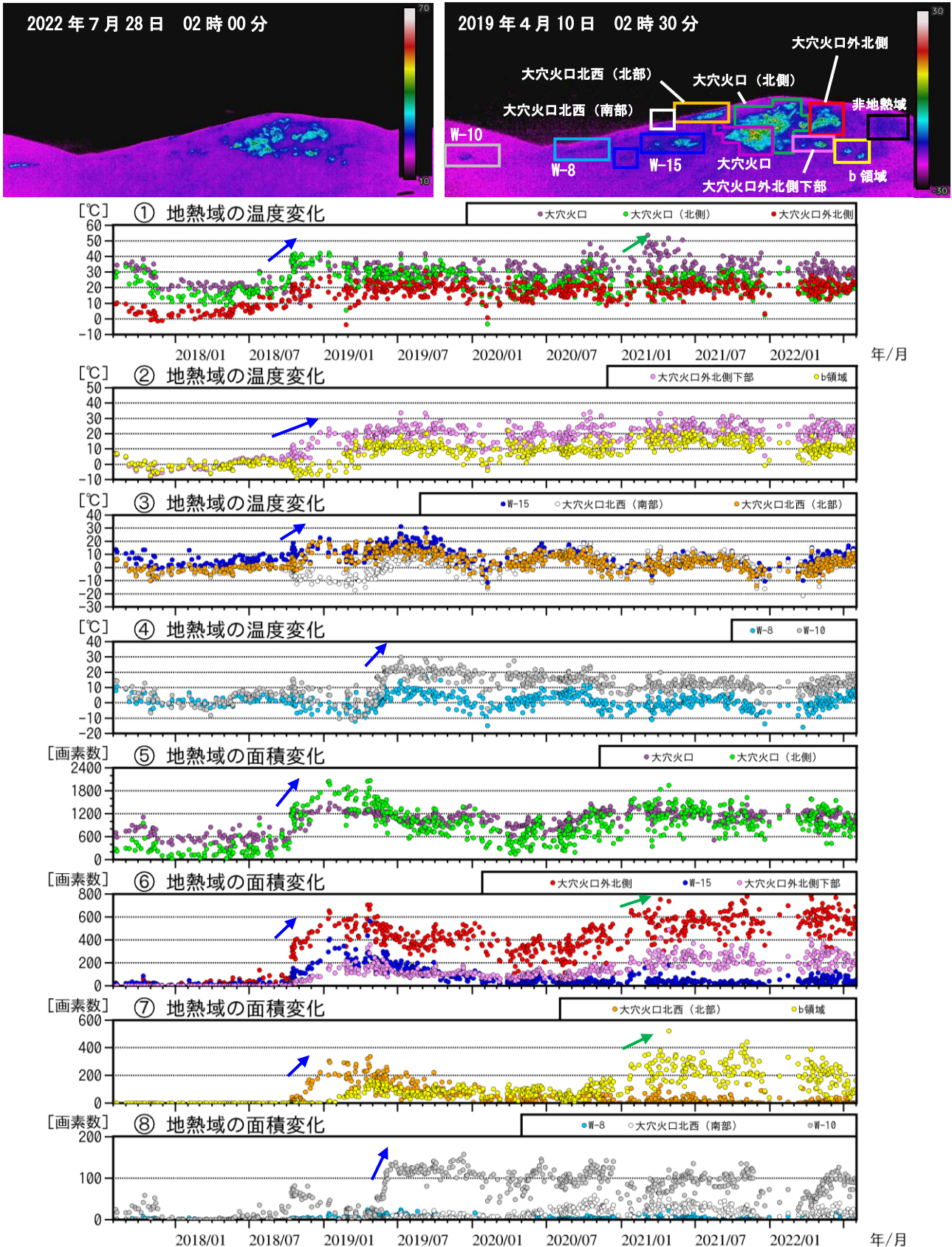
図9 吾妻山 監視カメラによる大穴火口周辺の地熱域の経過（2017年8月～2022年7月）
