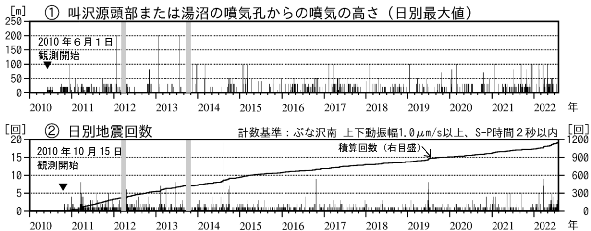
図3 秋田焼山 火山活動経過図（2010年6月～2022年7月）
