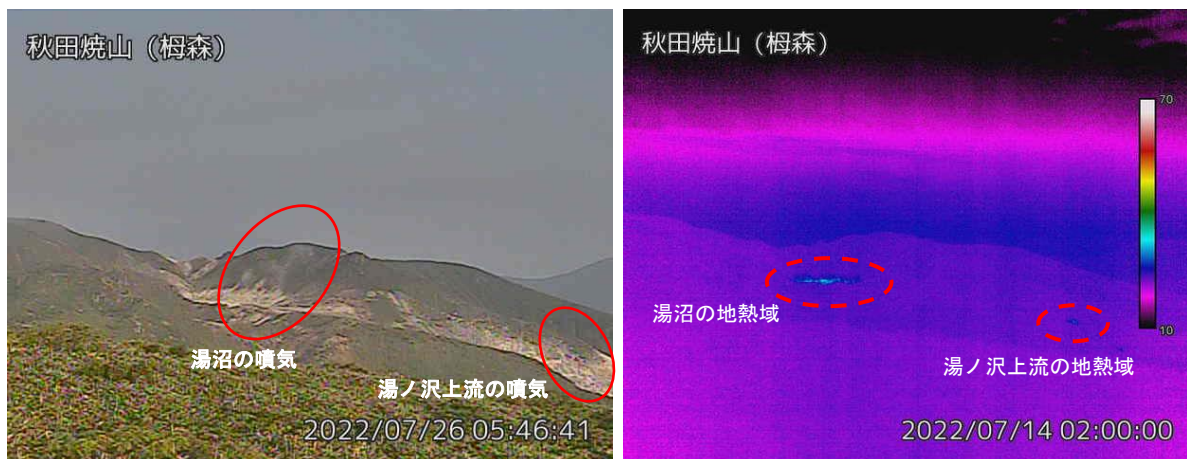
図2 秋田焼山 湯沼と湯ノ沢上流の状況（7月26日）と地表面温度分布（7月14日） ・柵森監視カメラ（湯沼の東約1 km）の映像です。
