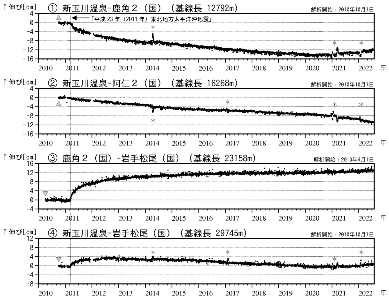
図4 秋田焼山 GNSS 基線長変化図（2010年4月～2022年7月）
