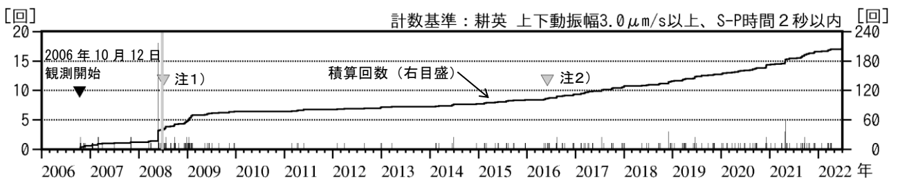
図3 栗駒山 日別地震回数（2006年10月～2022年6月）
