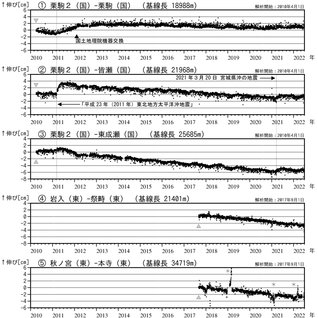
図4 栗駒山 GNSS 基線長変化図（2010年4月～2022年6月）
