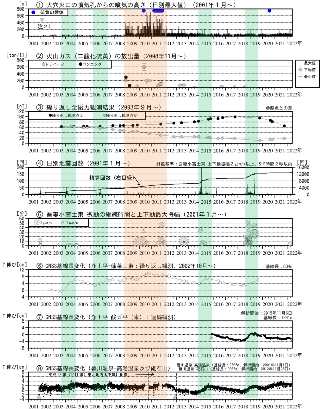
図2 吾妻山 中期的な火山活動の経過（2001年1月～2022年5月）
