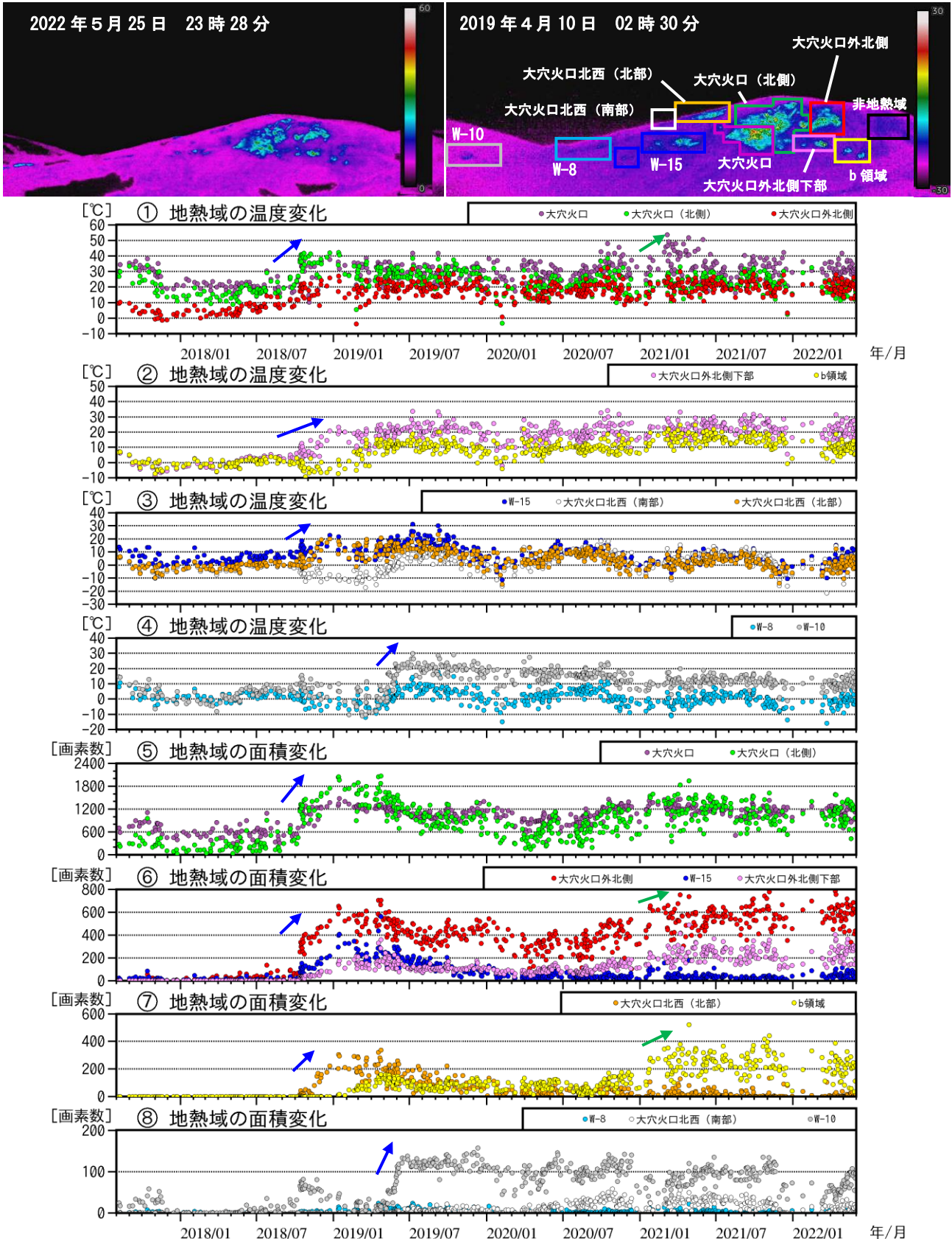
図7 吾妻山 監視カメラによる大穴火口周辺の地熱域の経過（2017年8月～2022年5月）
