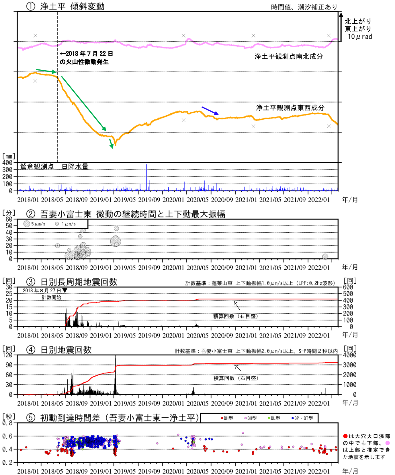
図3 吾妻山 火山活動経過図（2018年1月～2022年5月）
