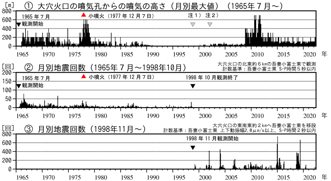
図1 吾妻山 長期的な火山活動の経過（1965年7月～2022年5月）
