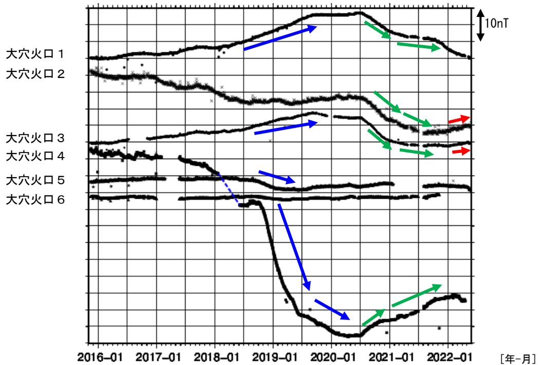
図11 吾妻山 全磁力連続観測点の全磁力値変化 (2015年11月~2022年5月)
