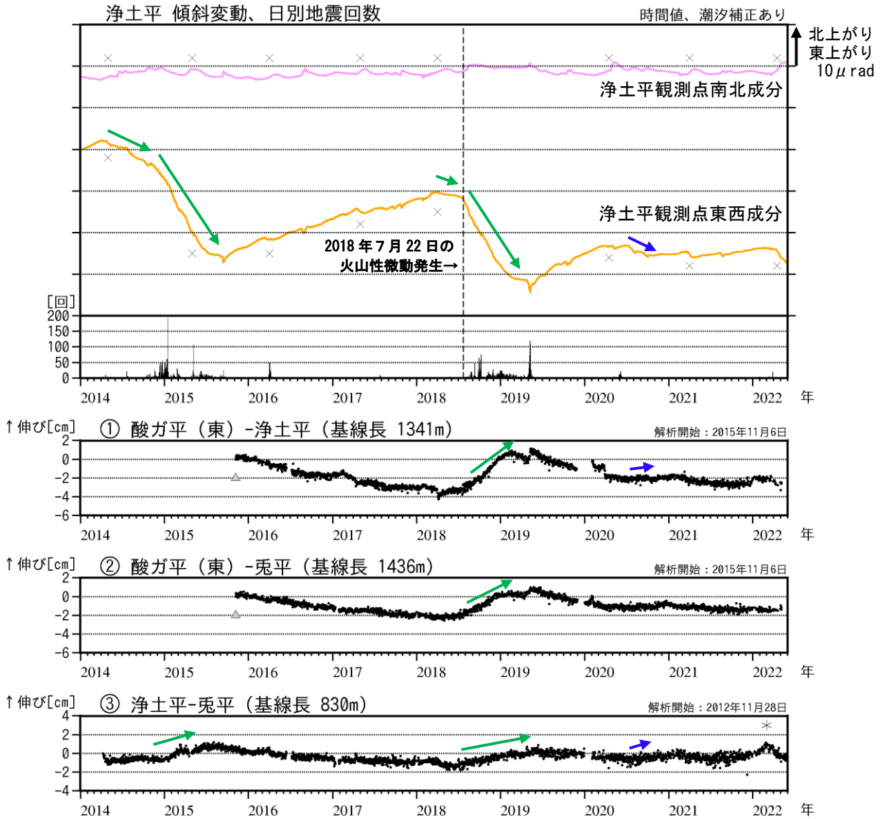
図5 吾妻山 大穴火口浅部の地殻変動（2014年1月～2022年5月）
