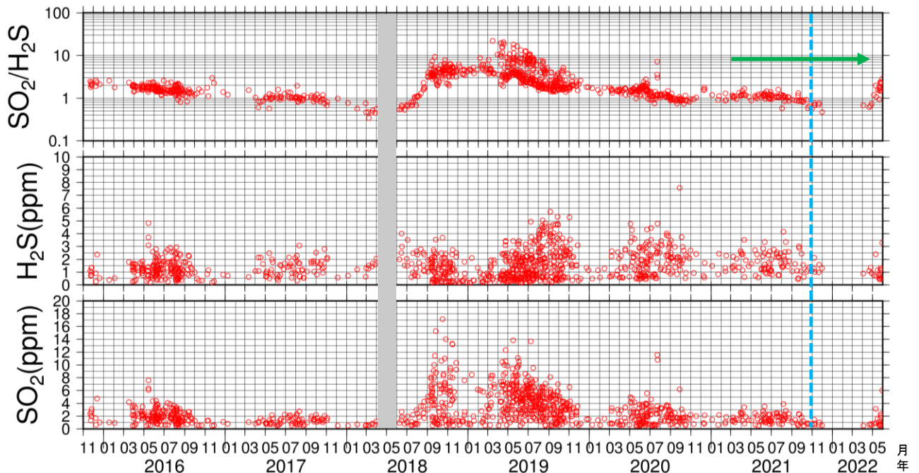
図9 吾妻山 火山ガス観測装置による観測（2015年11月～2022年5月）
