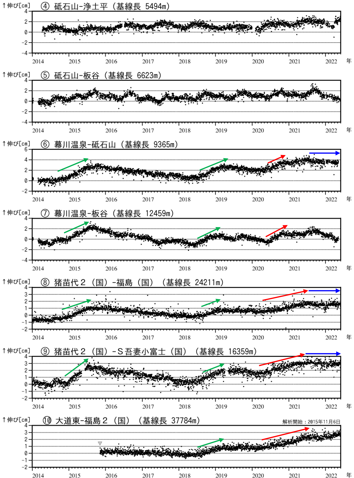
図6 吾妻山 吾妻山深部の地殻変動（2014年1月～2022年5月）
