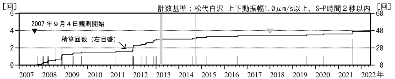
図2 岩木山 日別地震回数（2007年9月～2022年5月）
