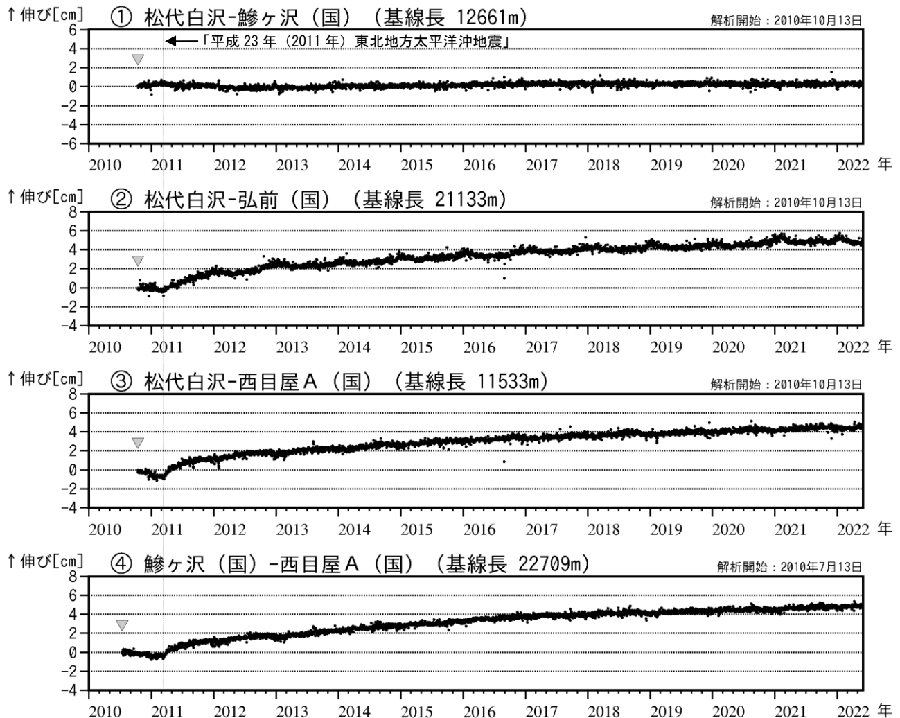
図3 岩木山 GNSS 基線長変化図（2010年7月～2022年5月）
