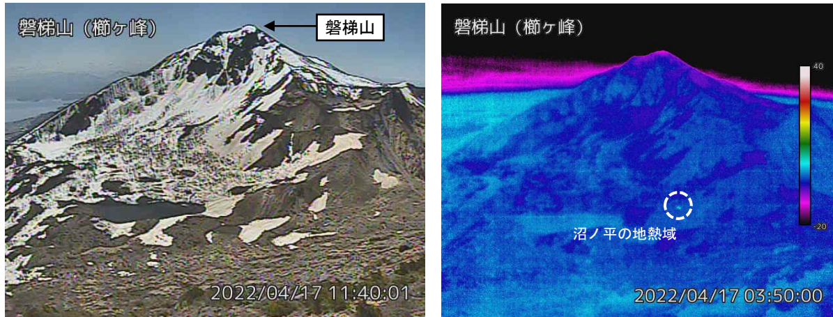
図2 磐梯山 沼ノ平周辺の状況と地表面温度分布（4月17日）
