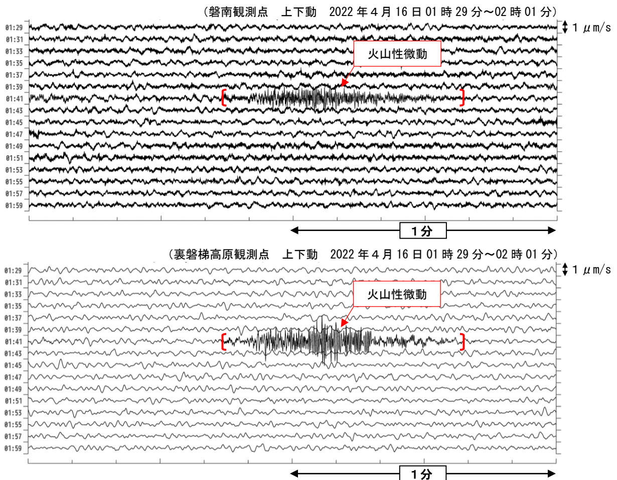
図3 磐梯山 火山性微動の発生状況
