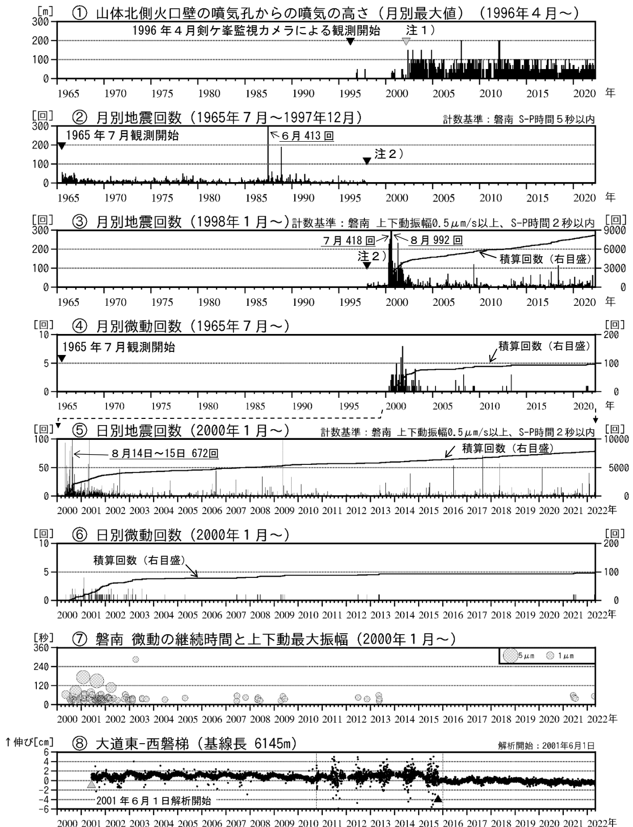
図4 磐梯山 火山活動経過図（1965年7月～2022年4月）
