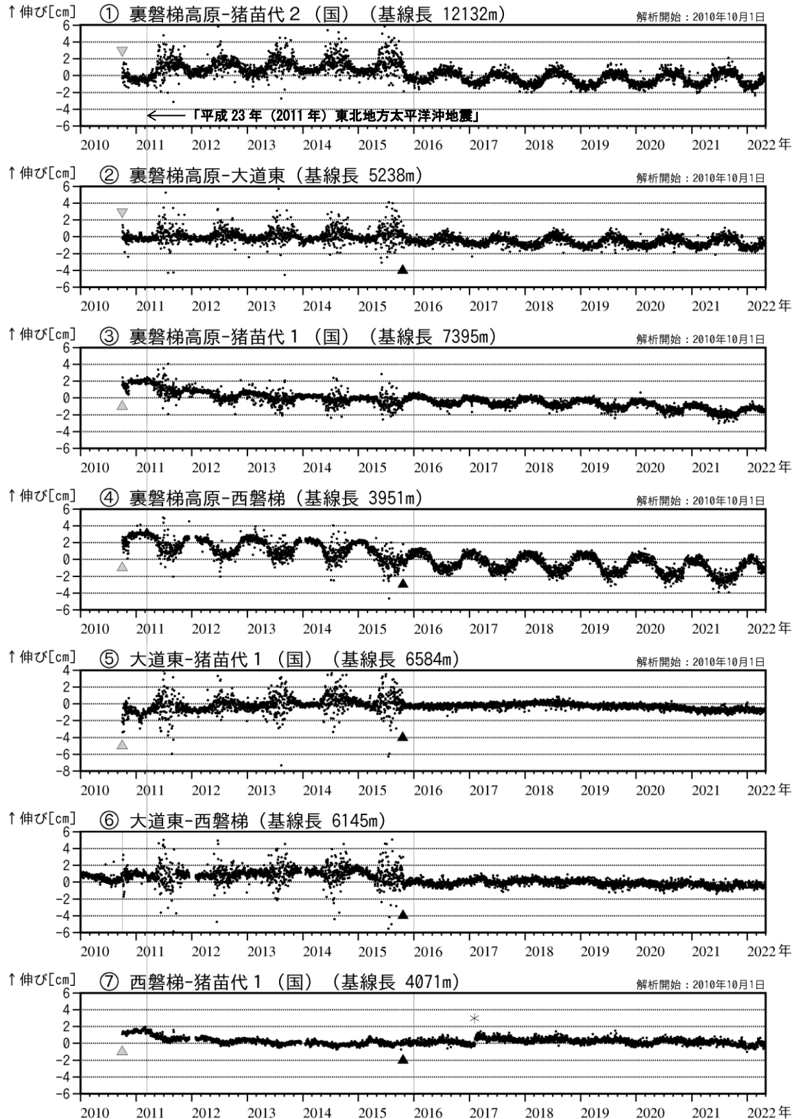
図5 磐梯山 GNSS 基線長変化図 (2010年1月～2022年4月)
