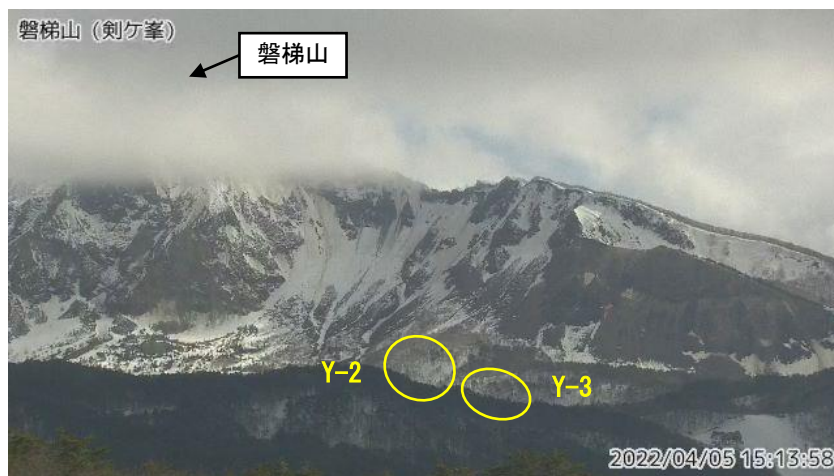
図1 磐梯山 山体北側火口壁の噴気の状況（4月5日）
