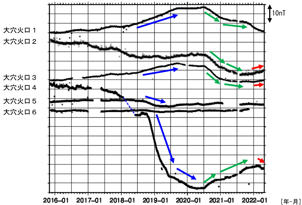
図 18 吾妻山 全磁力連続観測点の全磁力値変化 (2015年11月~2022年4月)
