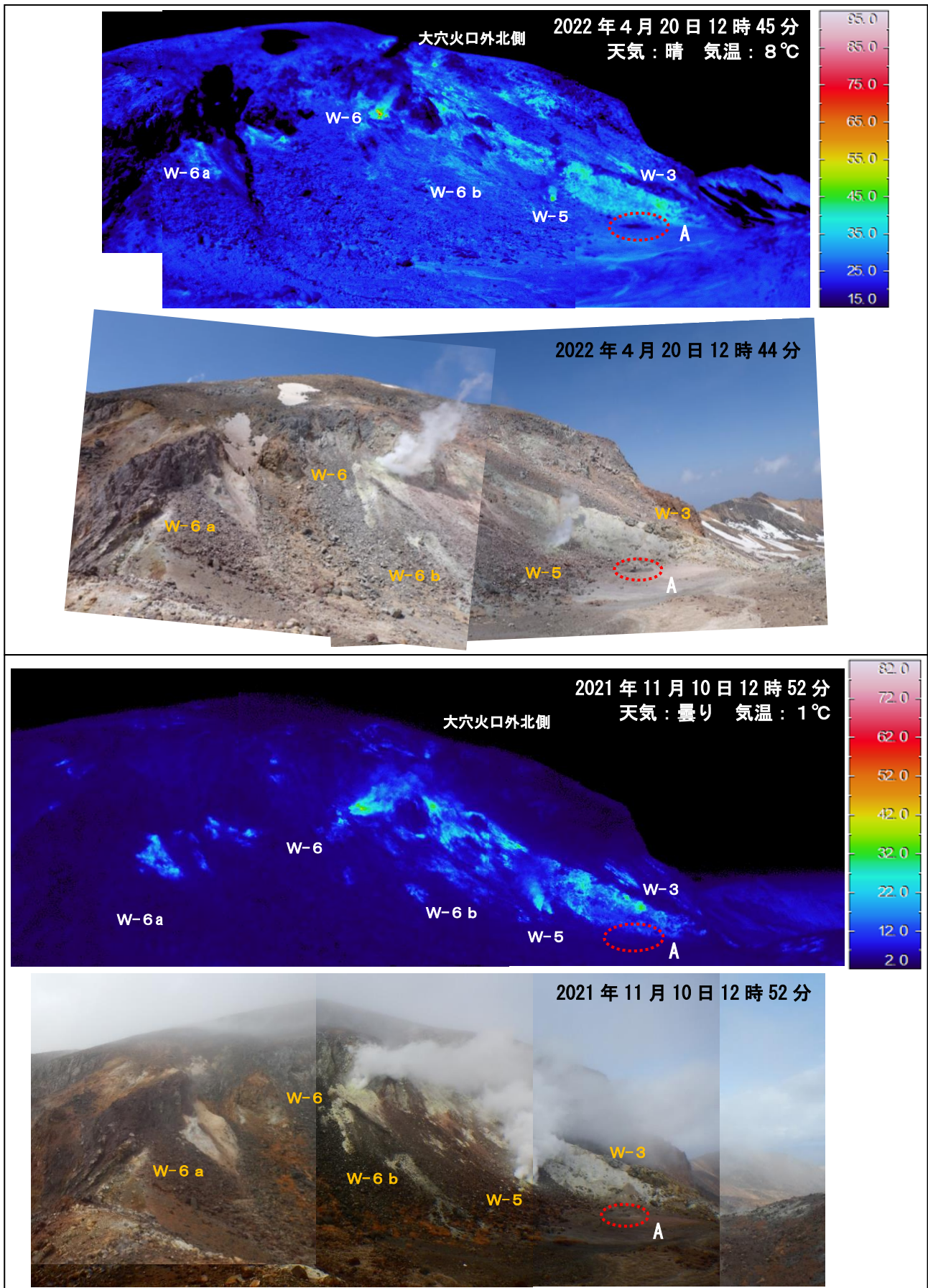
図10 吾妻山 大穴火口付近及びその周辺の状況（下）と地表面温度分布（上）
