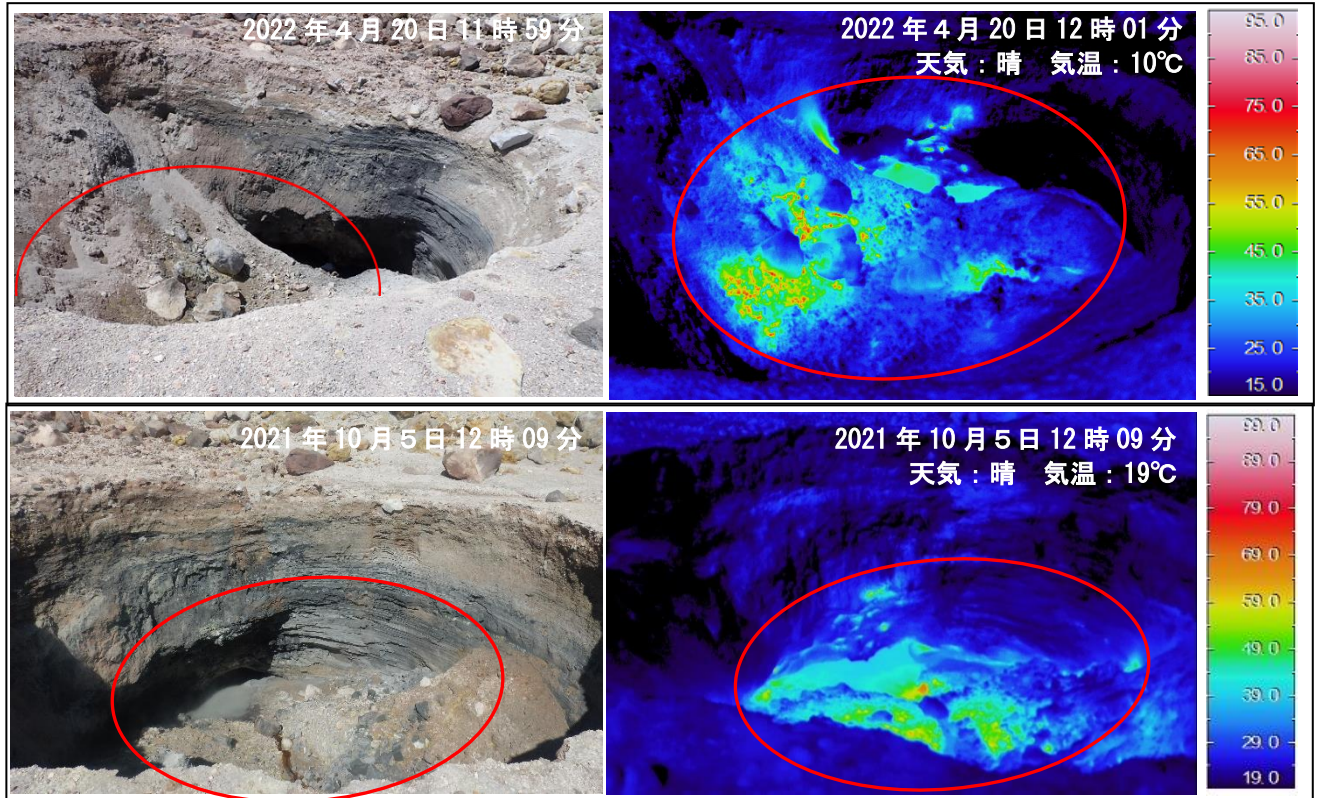
図 12 吾妻山 陥没孔内の状況（左）と表面温度分布（右）
