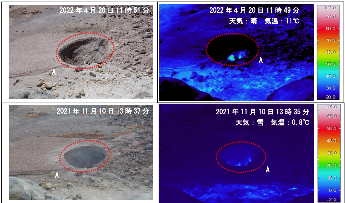
図 11 吾妻山 大穴火口内北側の陥没孔周辺の状況（左）と地表面温度分布（右）
