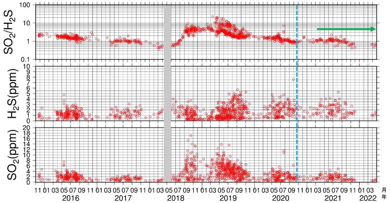
図 16 吾妻山 火山ガス観測装置による観測（2015年11月～2022年4月）
