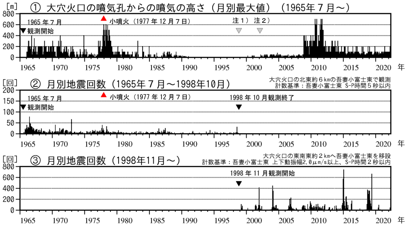
図1 吾妻山 長期的な火山活動の経過（1965年7月～2022年4月）
