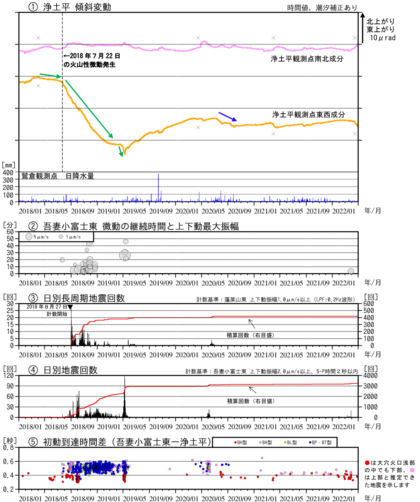
図3 吾妻山 火山活動経過図 (2018年1月～2022年4月)
