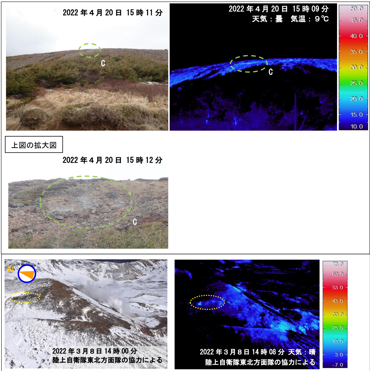
図 14 吾妻山 大穴火口北西の北西端の状況（左）と地表面温度分布（右）
