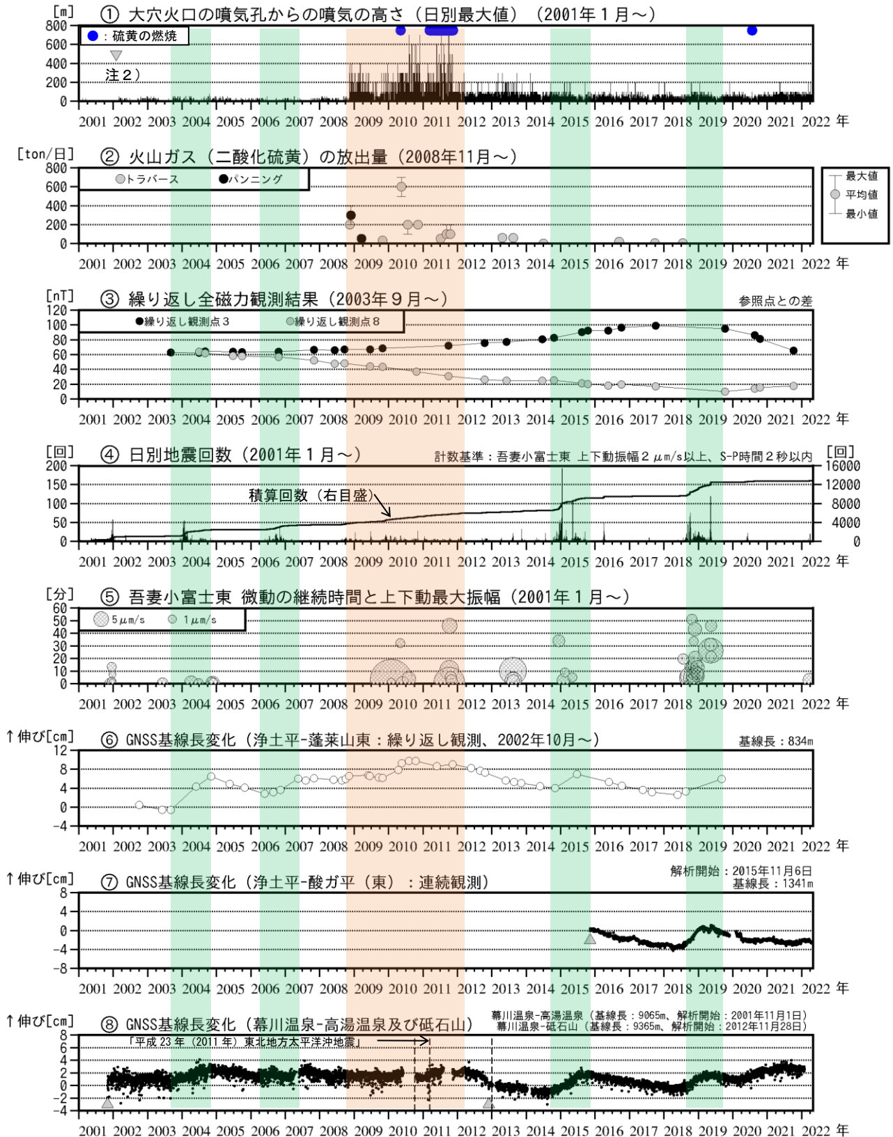
図2 吾妻山 中期的な火山活動の経過（2001年1月～2022年4月）
