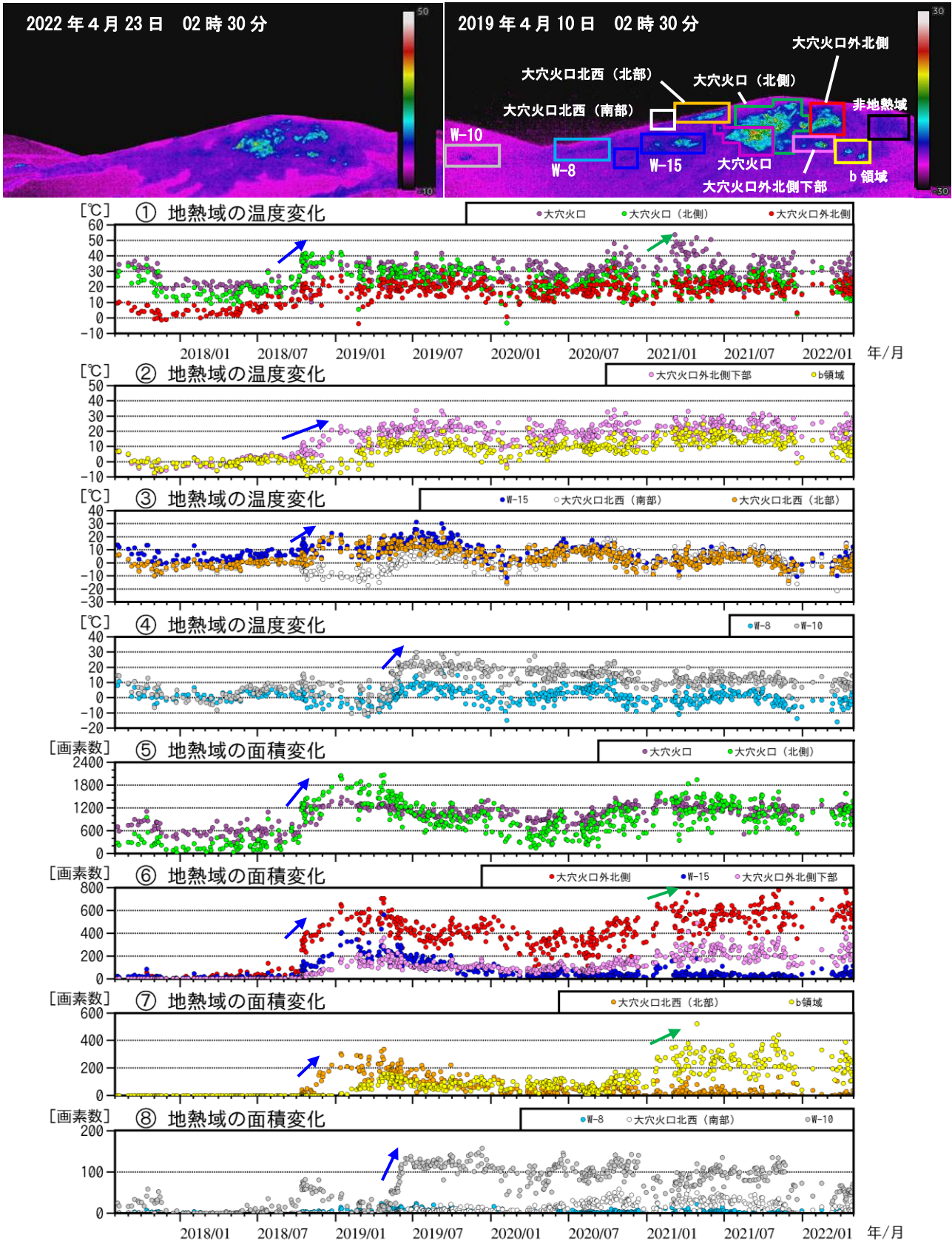
図7 吾妻山 監視カメラによる大穴火口周辺の地熱域の経過（2017年8月～2022年4月）
