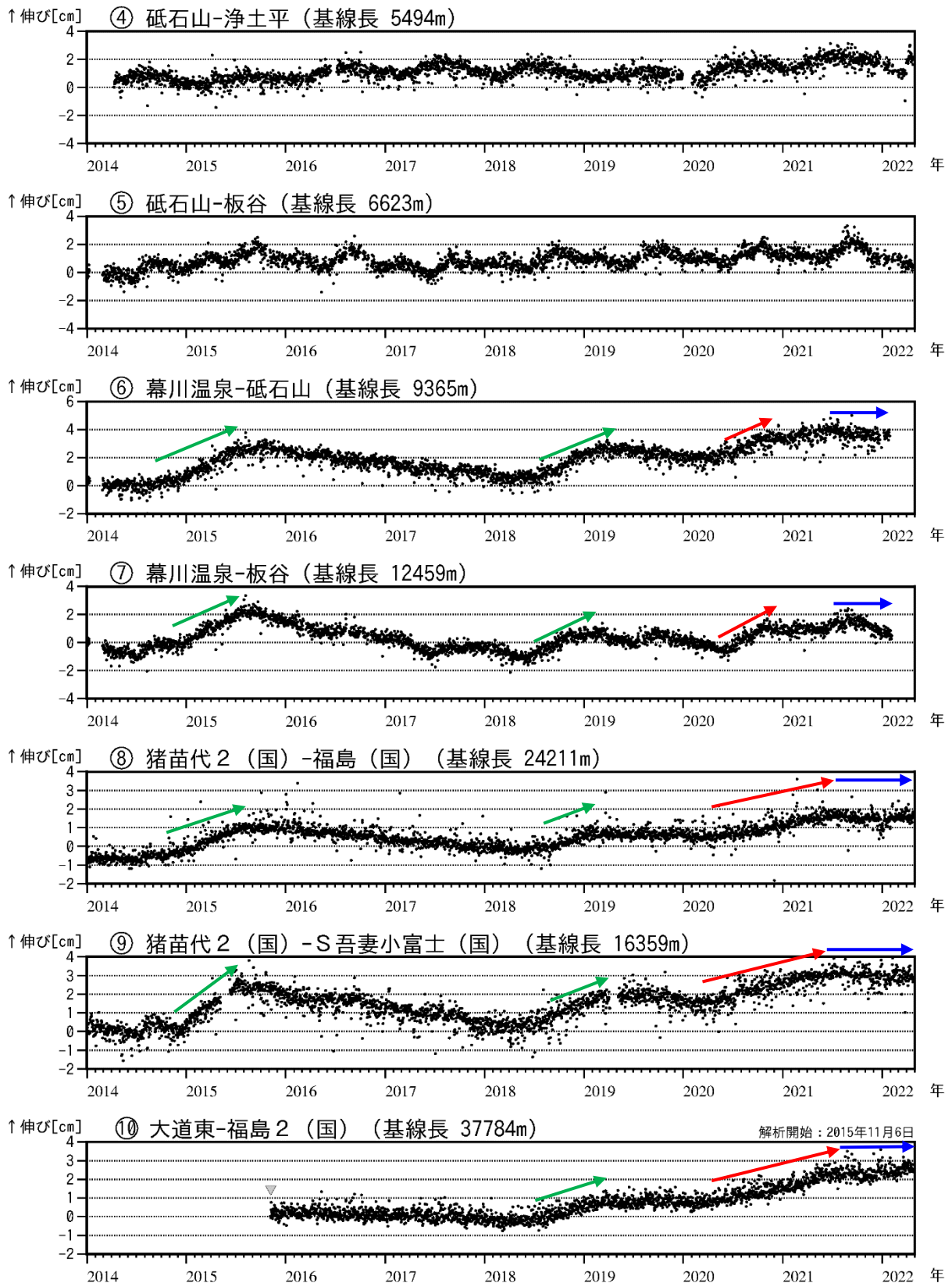
図6 吾妻山 吾妻山深部の地殻変動（2014年1月～2022年4月）
