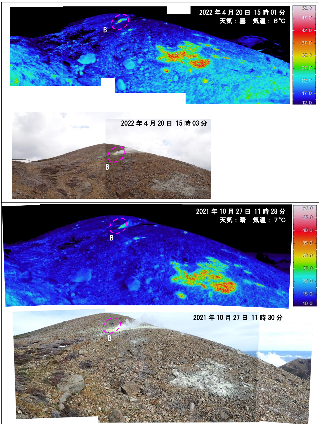
図13 吾妻山 大穴火口北西の状況（下）と地表面温度分布（上）
