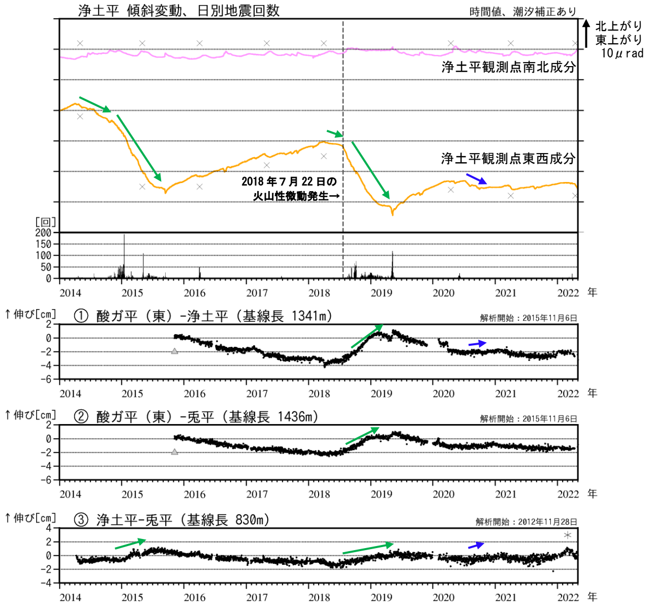
図5 吾妻山 大穴火口浅部の地殻変動 (2014年1月～2022年4月)
