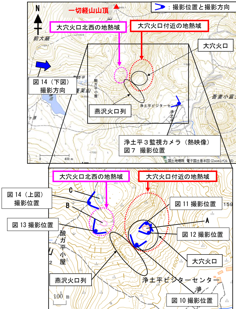
図9 吾妻山 大穴火口周辺の地熱域の分布及び熱映像撮影方向
