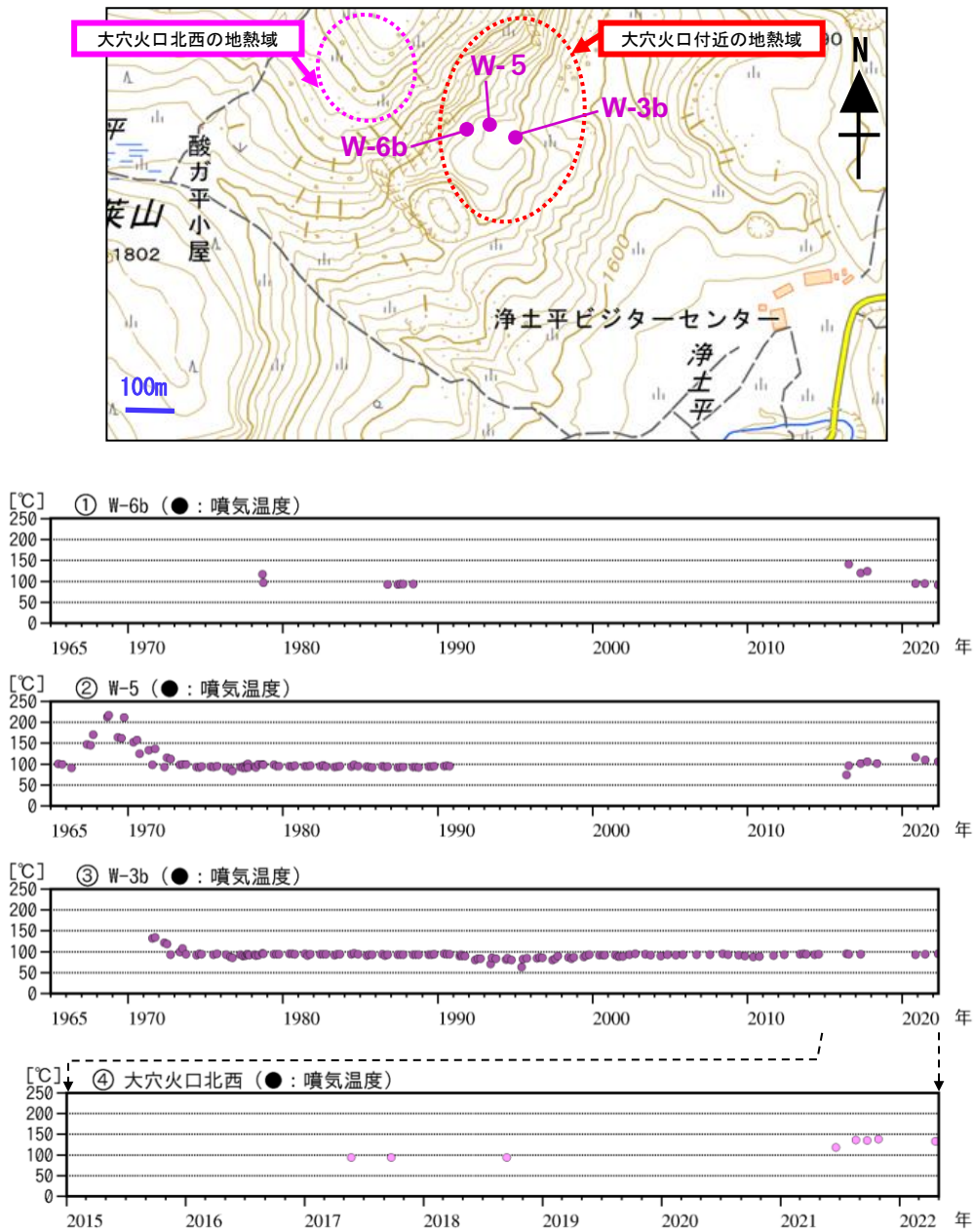
図15 吾妻山 大穴火口周辺の噴気温度の経過（1965年7月～2022年4月）
