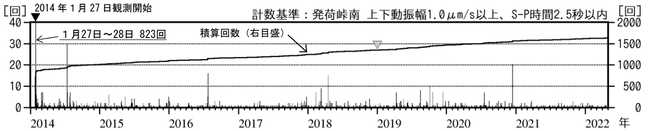
図2 十和田 日別地震回数（2014年1月～2022年4月）
