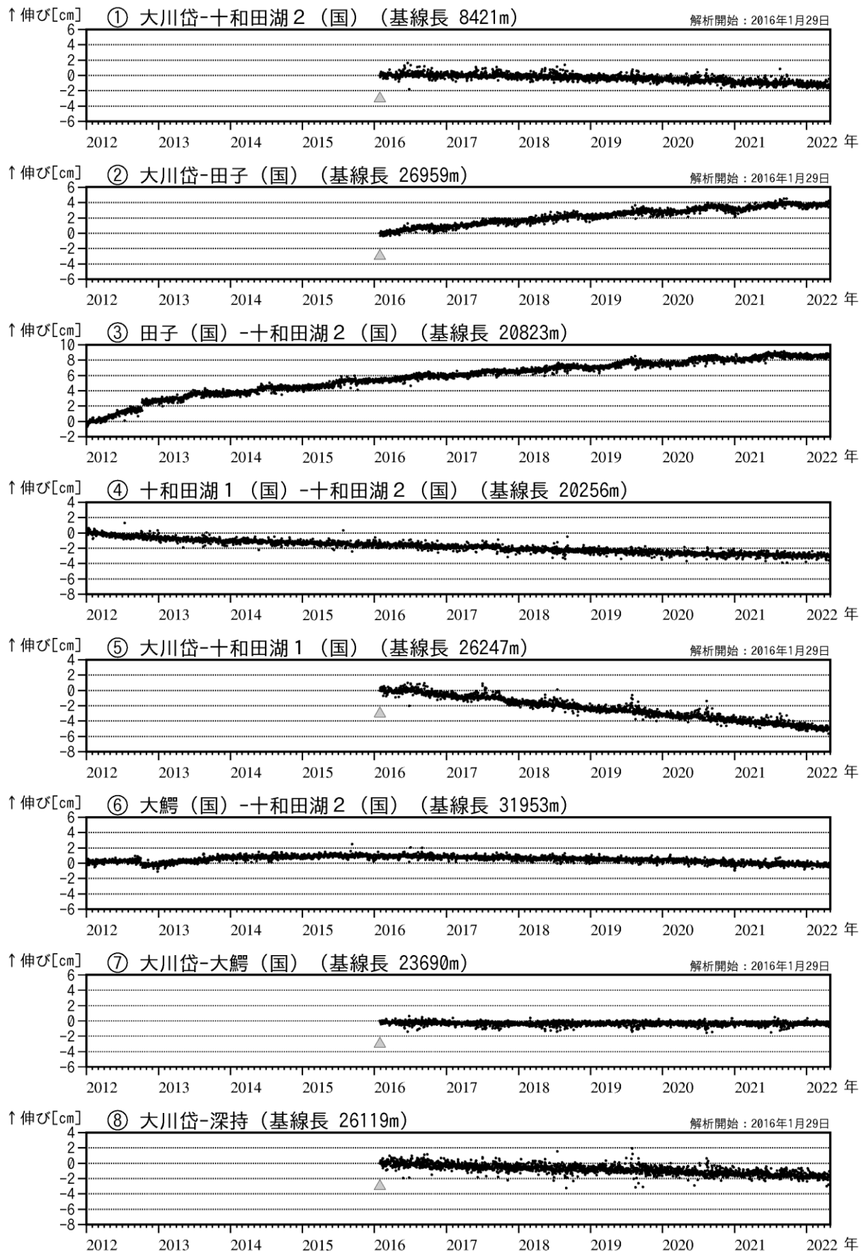
図4 十和田 GNSS 基線長変化図 (2012年1月~2022年4月)
