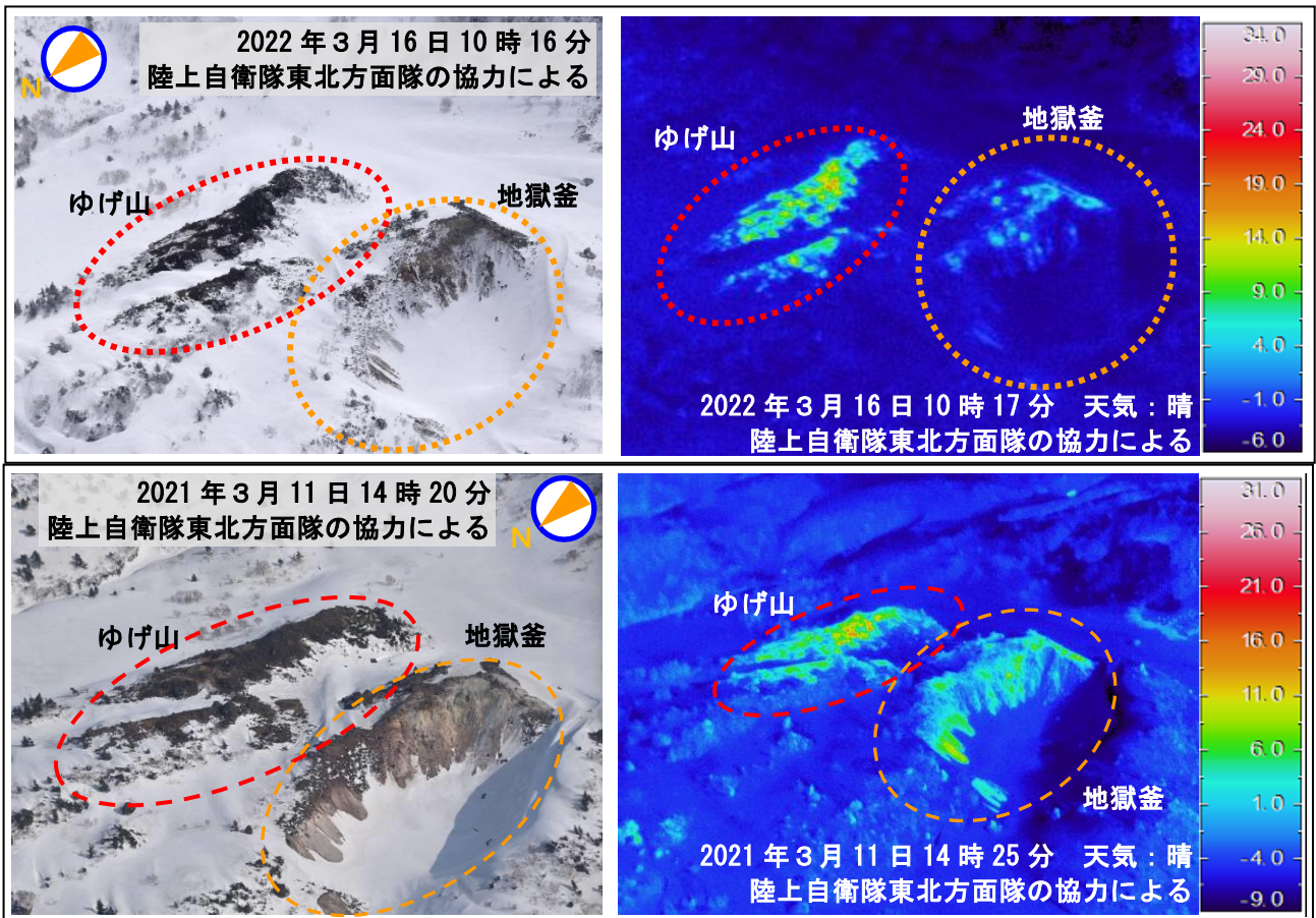
図5 栗駒山 上空からのゆげ山及び地獄釜の状況と地表面温度分布
