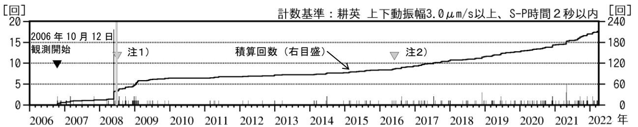
図6 栗駒山 日別地震回数（2006年10月～2022年3月）
