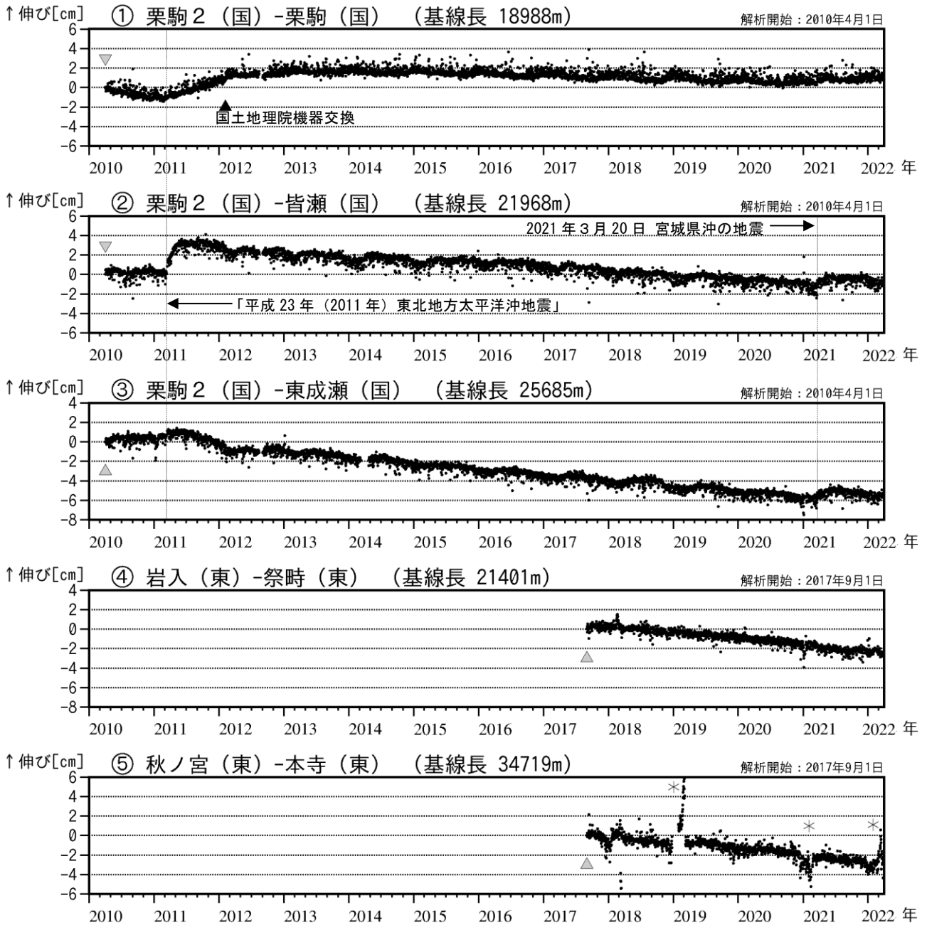
図7 栗駒山 GNSS 基線長変化図 (2010年4月~2022年3月)
