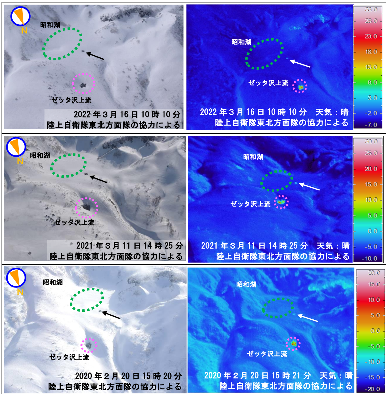
図4 栗駒山 上空からのゼッタ沢上流及び昭和湖の状況と地表面温度分布
