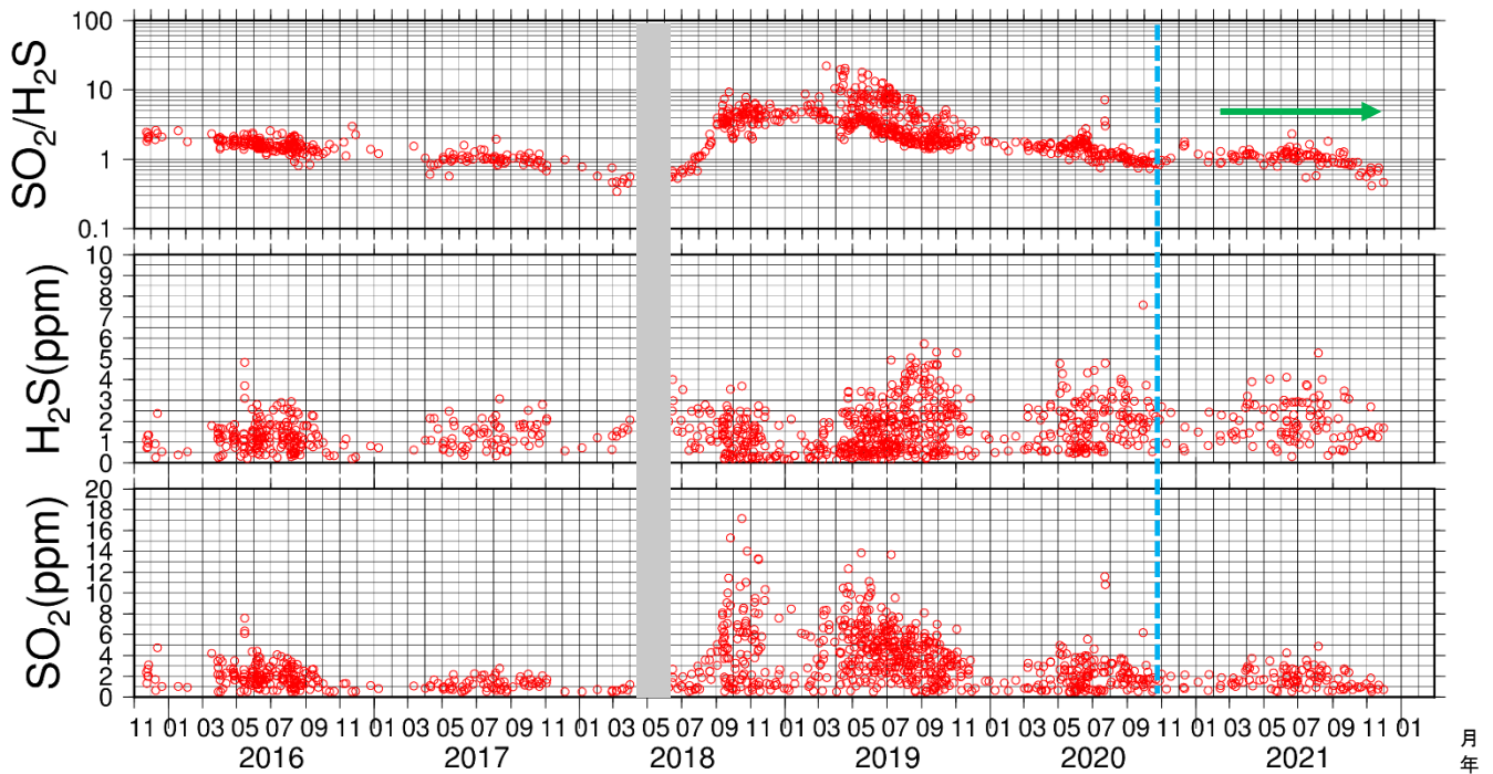
図10 吾妻山 火山ガス観測装置による観測（2015年11月～2022年2月）
