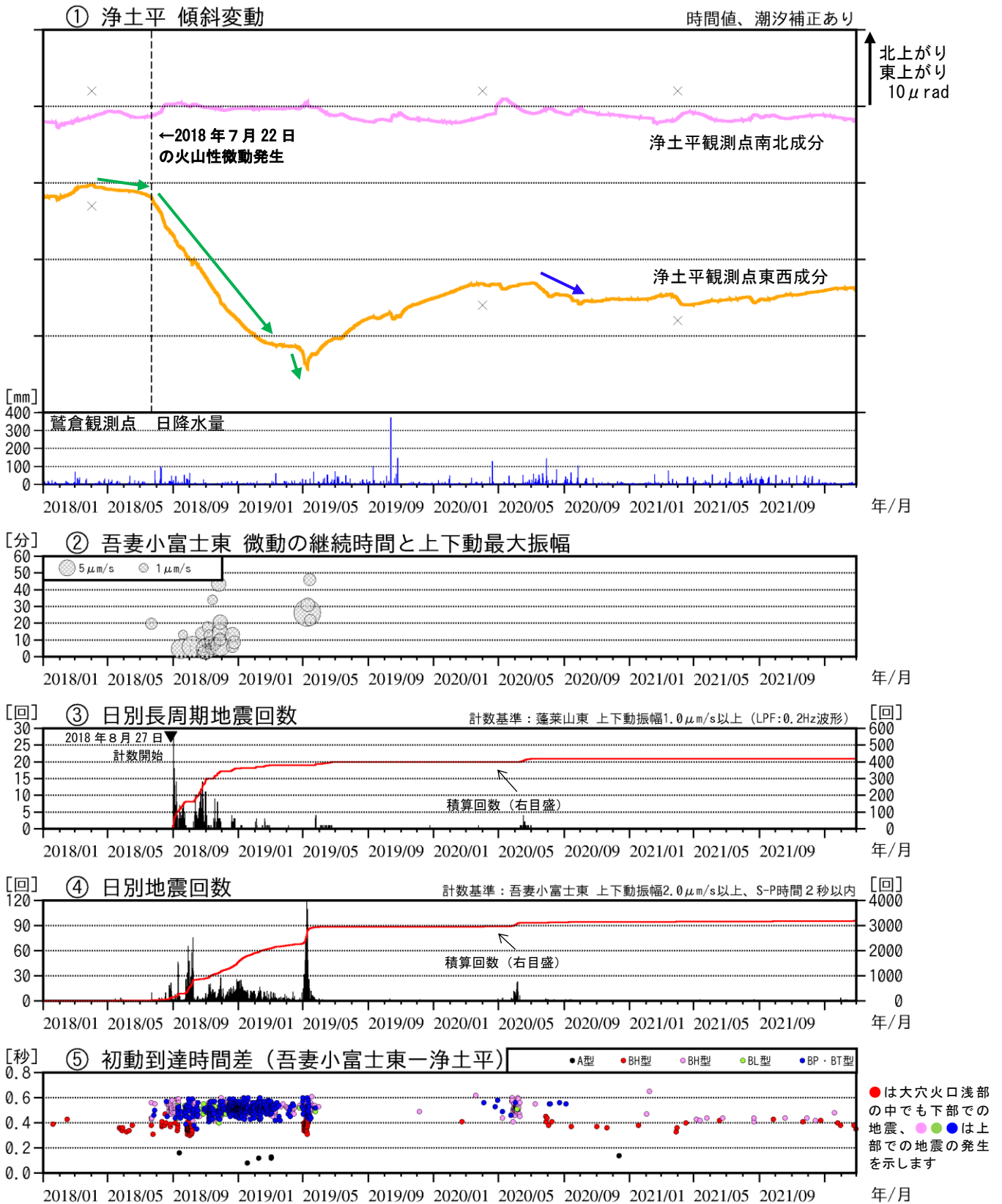
図3 吾妻山 火山活動経過図 (2018年1月~2022年2月)
