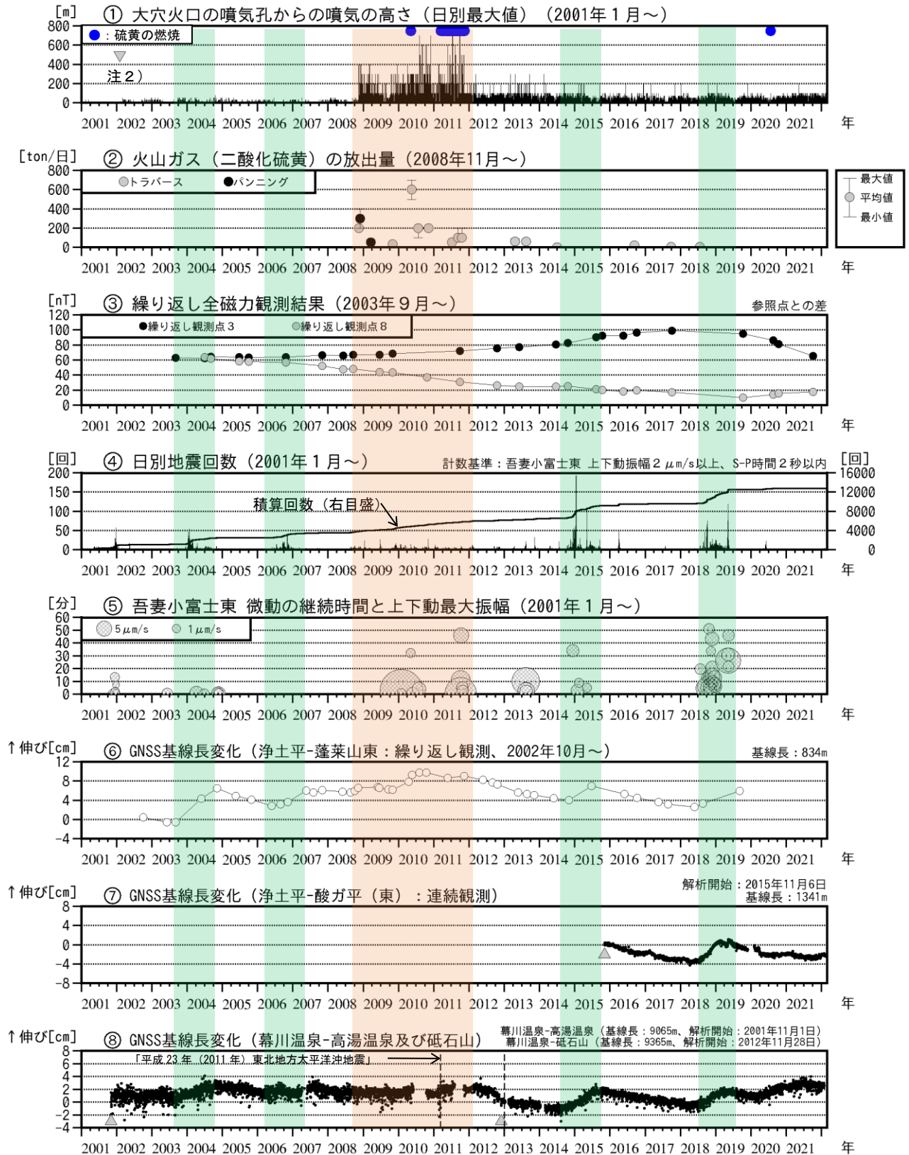
図2 吾妻山 中期的な火山活動の経過（2001年1月～2022年2月）
