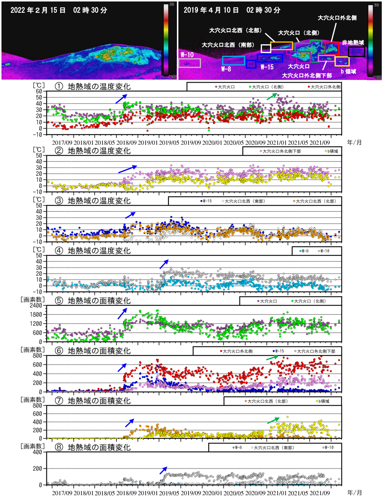
図8 吾妻山 監視カメラによる大穴火口周辺の地熱域の経過（2017年8月～2022年2月）
