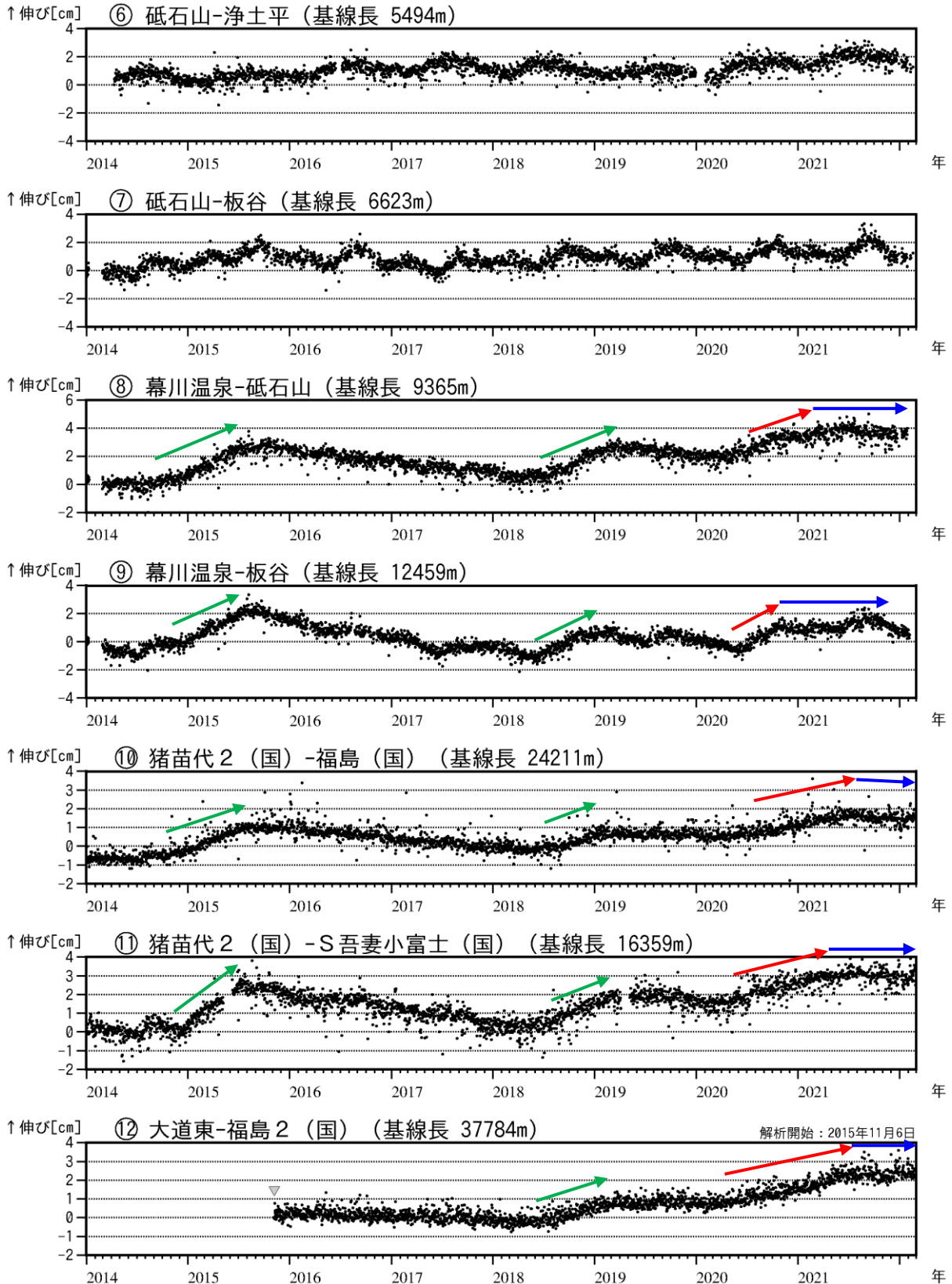
図7 吾妻山 吾妻山深部の地殻変動（2014年1月～2022年2月）
