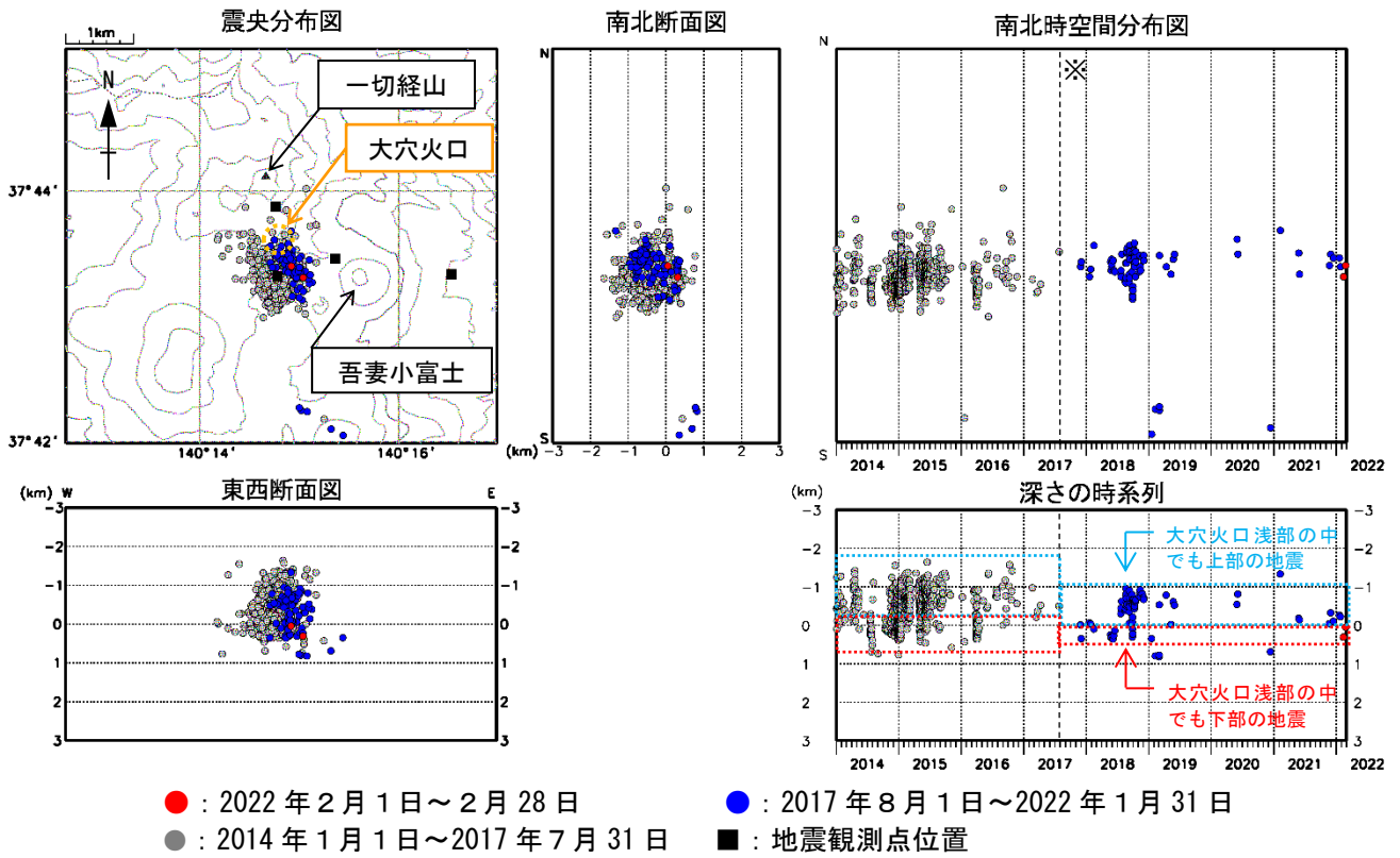
図4 吾妻山 地震活動（2014年1月～2022年2月）
