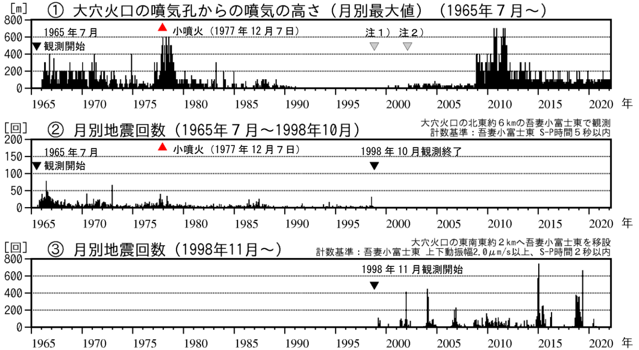
図1 吾妻山 長期的な火山活動の経過（1965年7月～2022年2月）
