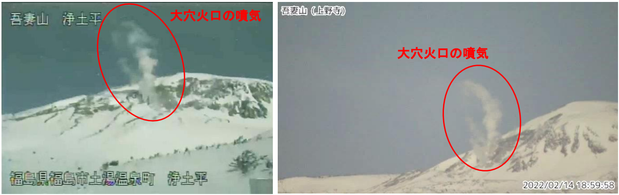
図9 吾妻山 大穴火口周辺の噴気の状態（2月14日）
