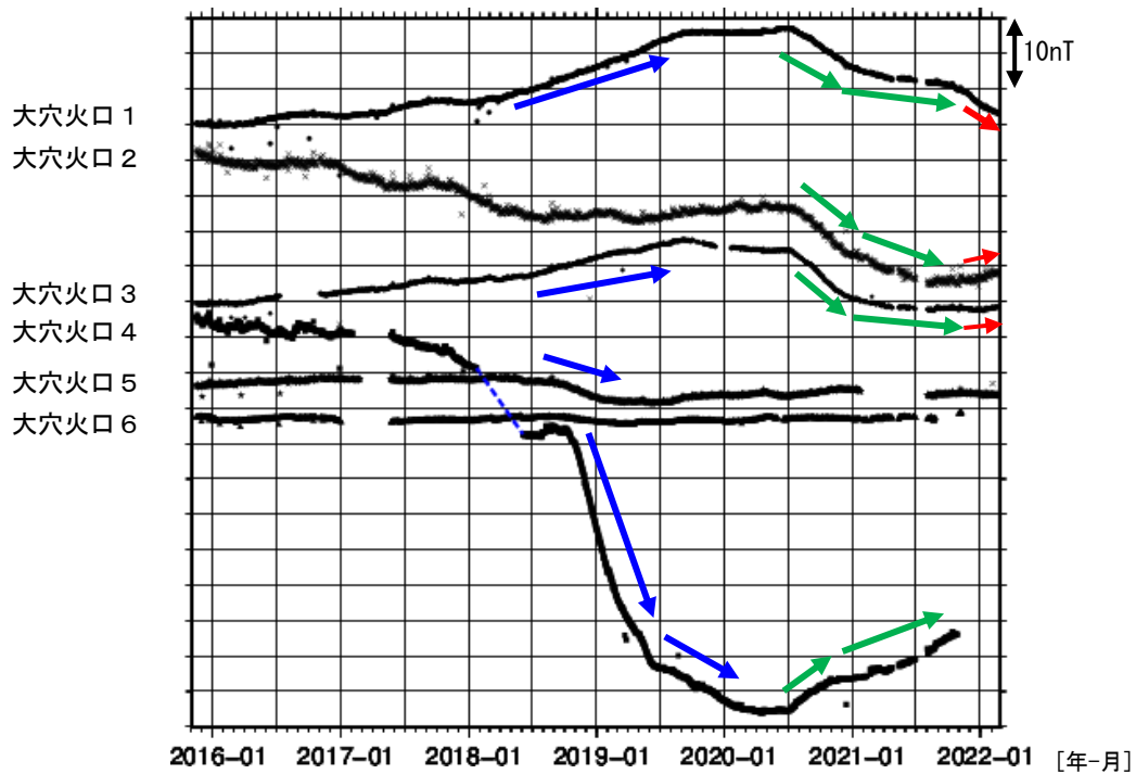
図 12 吾妻山 全磁力連続観測点の全磁力値変化 (2015年11月~2022年2月)
