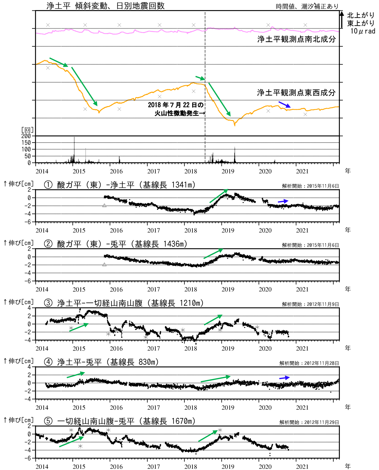
図6 吾妻山 大穴火口浅部の地殻変動（2014年1月～2022年2月）
