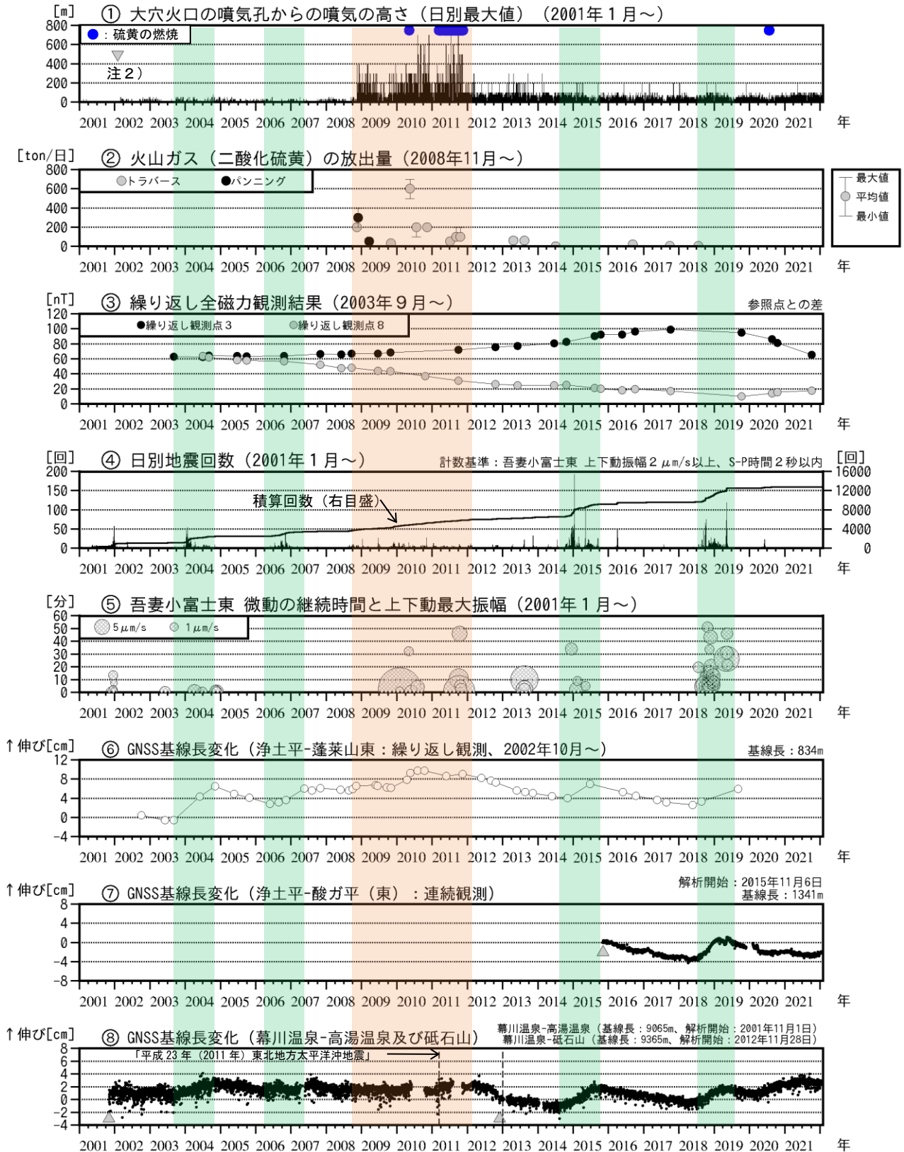
図2 吾妻山 中期的な火山活動の経過（2001年1月～2022年1月）
