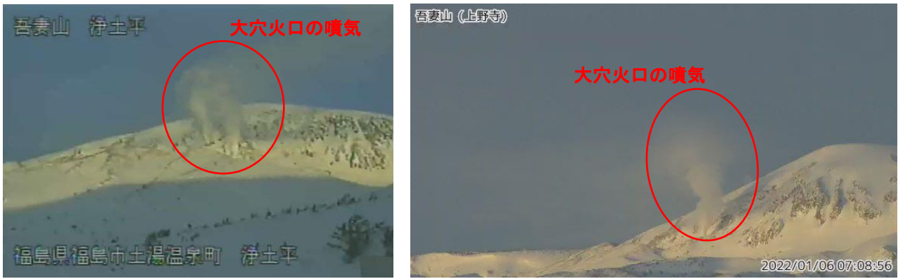
図8 吾妻山 大穴火口周辺の噴気の状態（1月6日）
