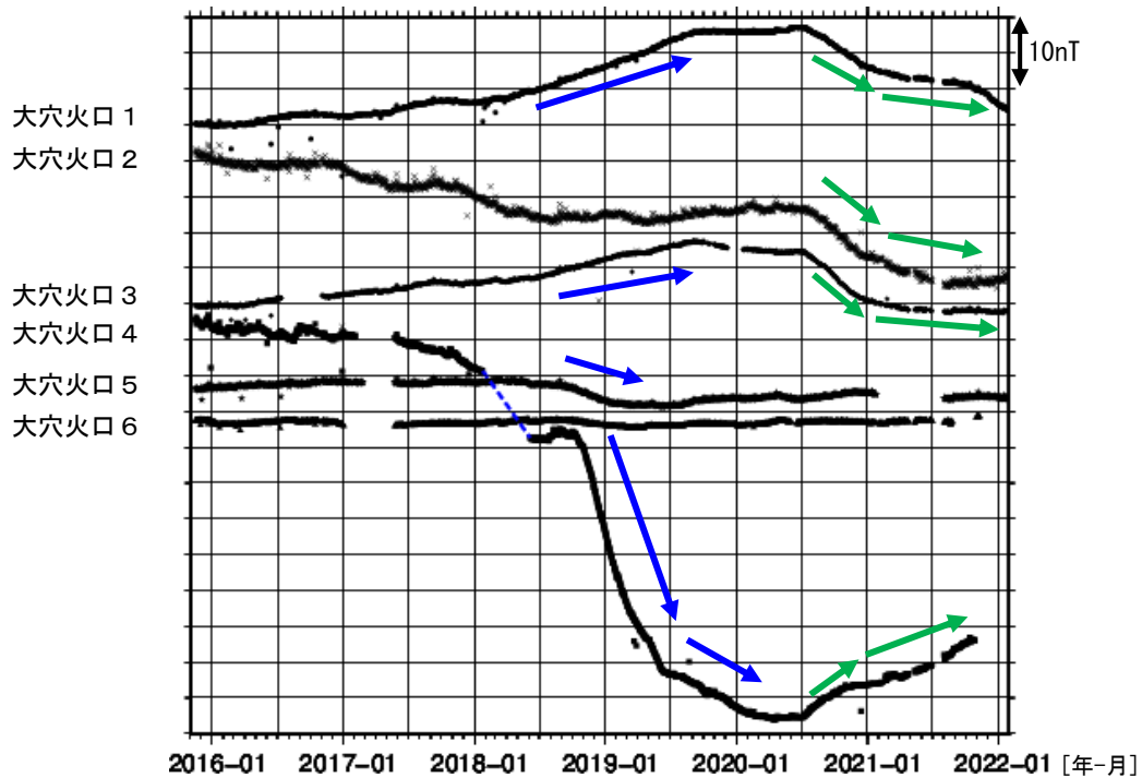
図11 吾妻山 全磁力連続観測点の全磁力値変化 (2015年11月~2022年1月)
