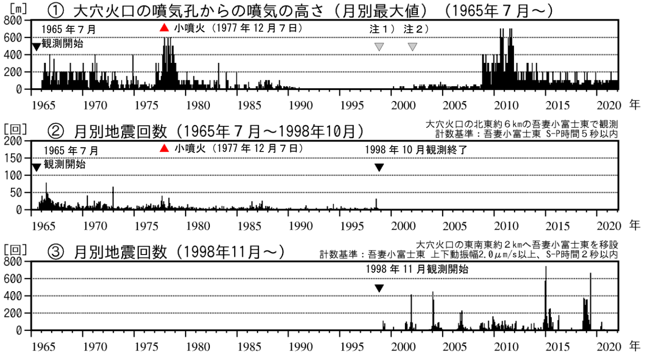
図1 吾妻山 長期的な火山活動の経過（1965年7月～2022年1月）
