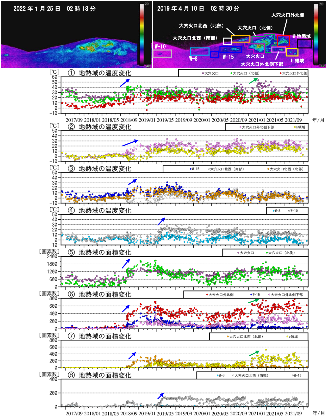
図7 吾妻山 監視カメラによる大穴火口周辺の地熱域の経過（2017年8月～2022年1月）
