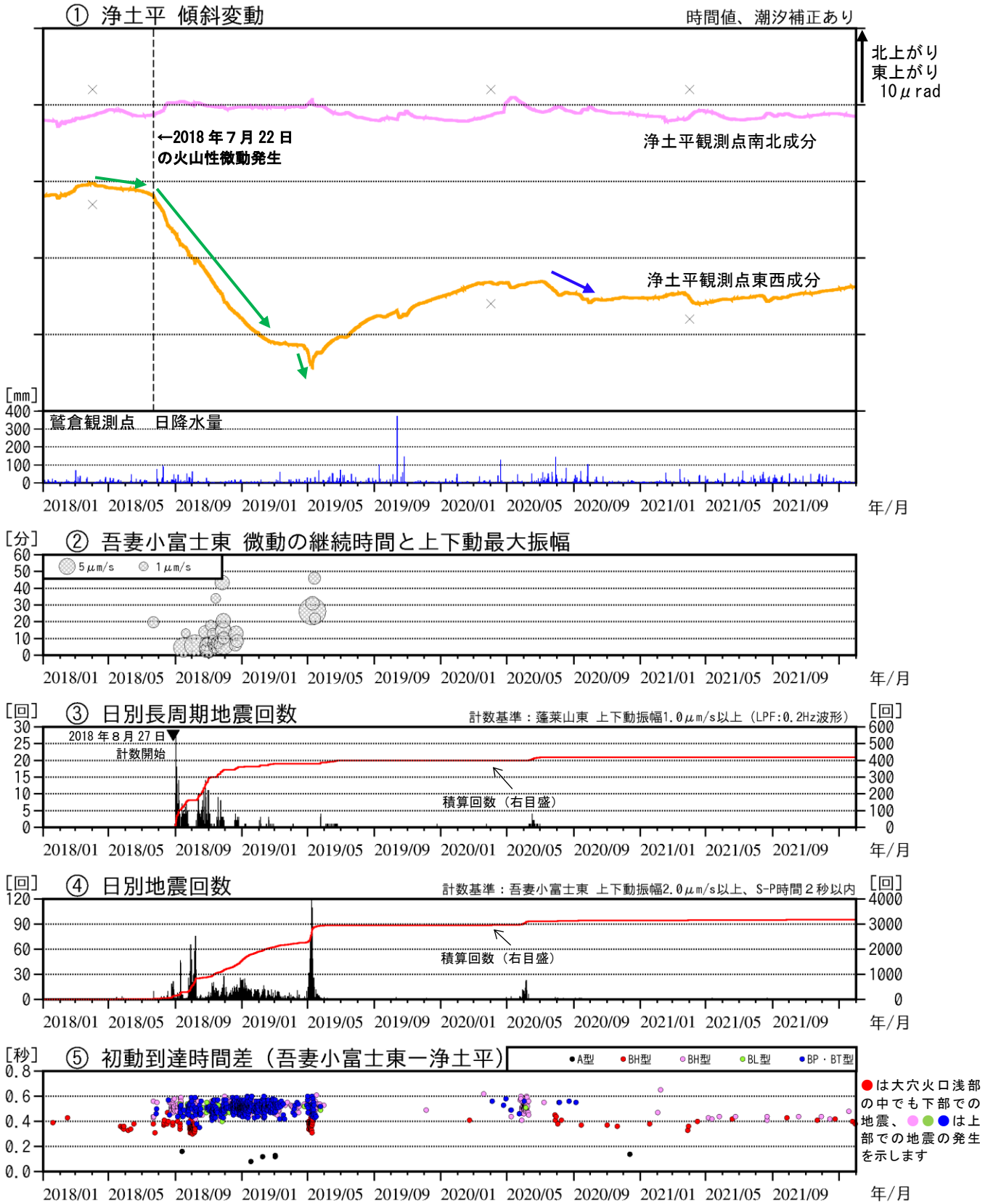
図3 吾妻山 火山活動経過図 (2018年1月～2022年1月)
