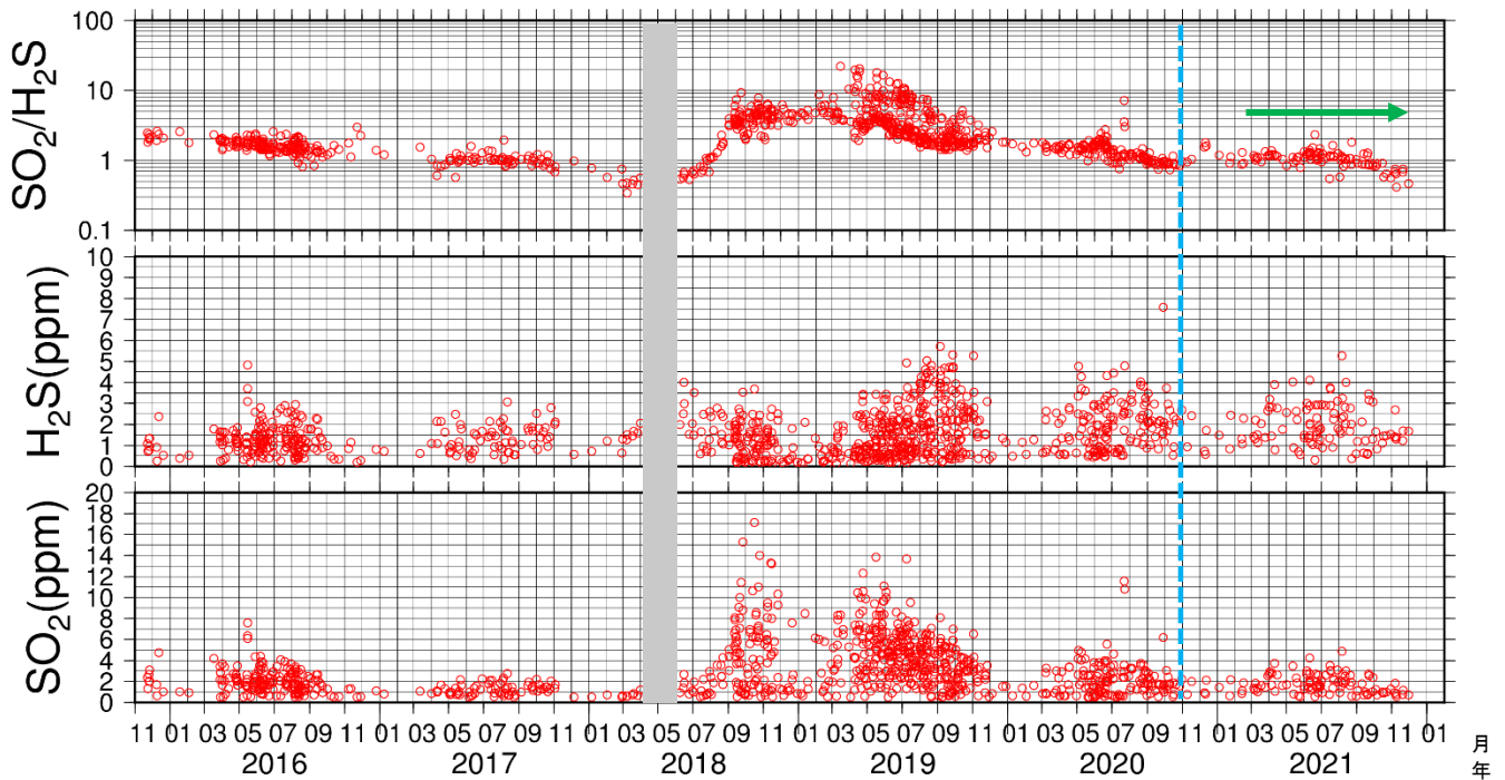
図9 吾妻山 火山ガス観測装置による観測（2015年11月～2022年1月）
