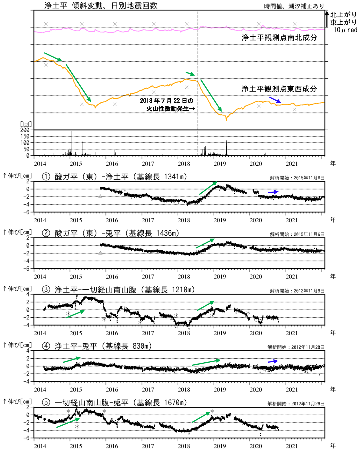
図5 吾妻山 大穴火口浅部の地殻変動（2014年1月～2022年1月）
