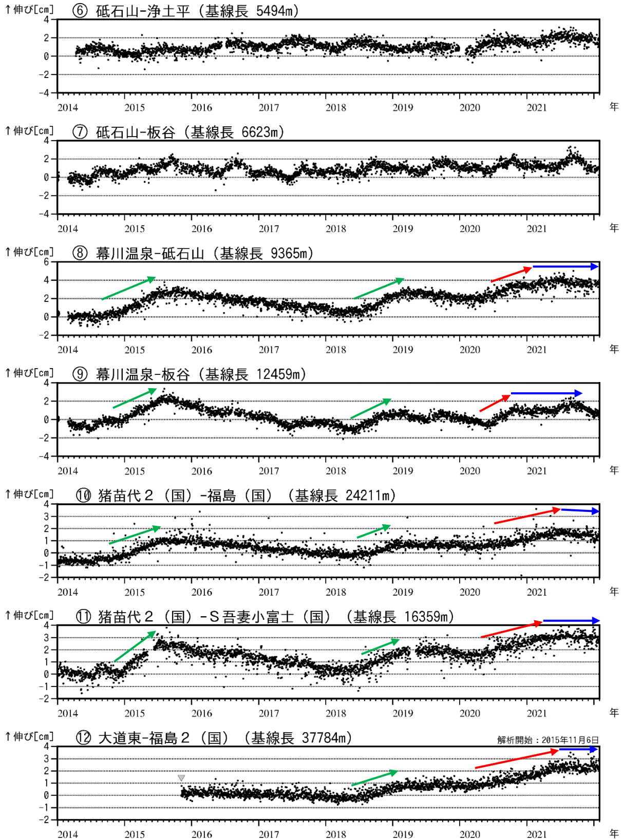
図6 吾妻山 吾妻山深部の地殻変動（2014年1月～2022年1月）
