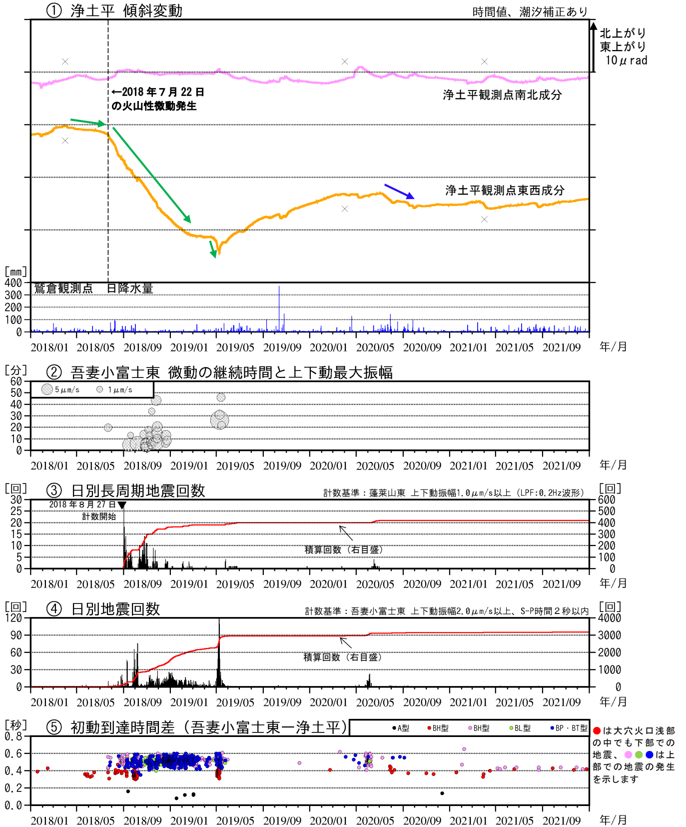
図3 吾妻山 火山活動経過図（2018年1月～2021年12月）
