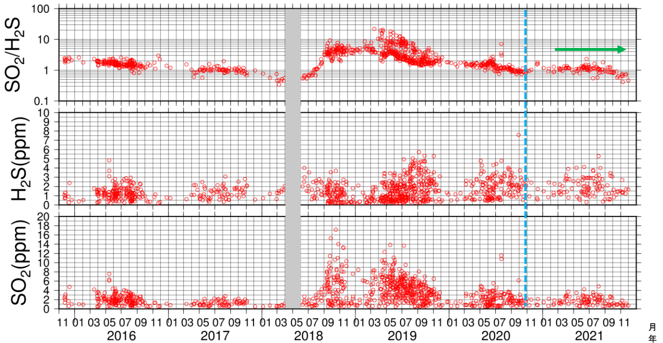
図9 吾妻山 火山ガス観測装置による観測（2015年11月～2021年12月）
