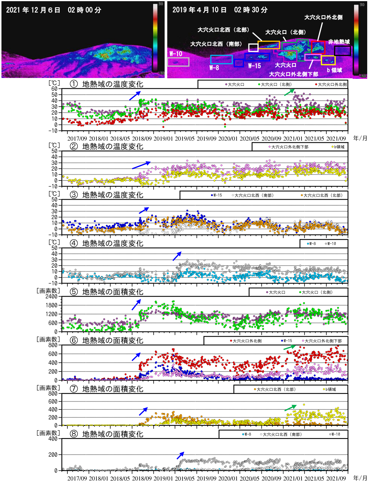
図7 吾妻山 監視カメラによる大穴火口周辺の地熱域の経過（2017年8月～2021年12月）
