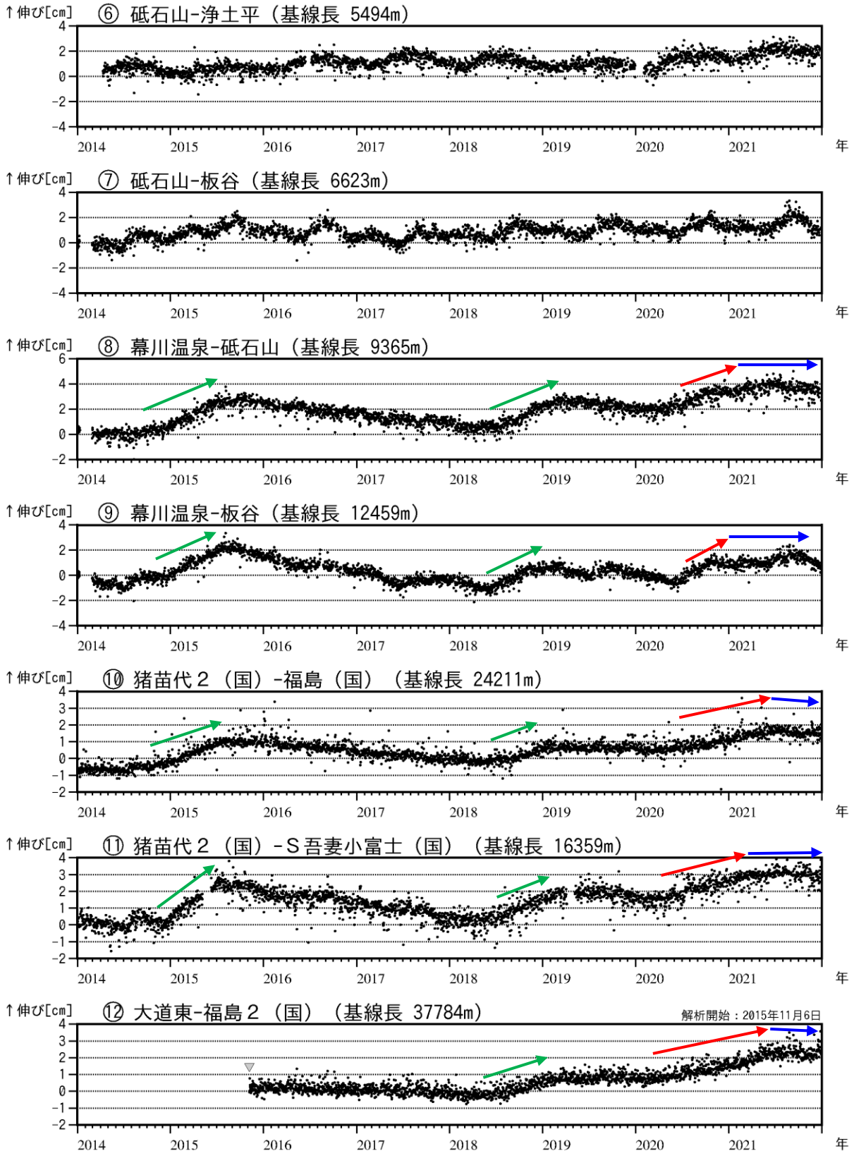
図6 吾妻山 吾妻山深部の地殻変動（2014年1月～2021年12月）
