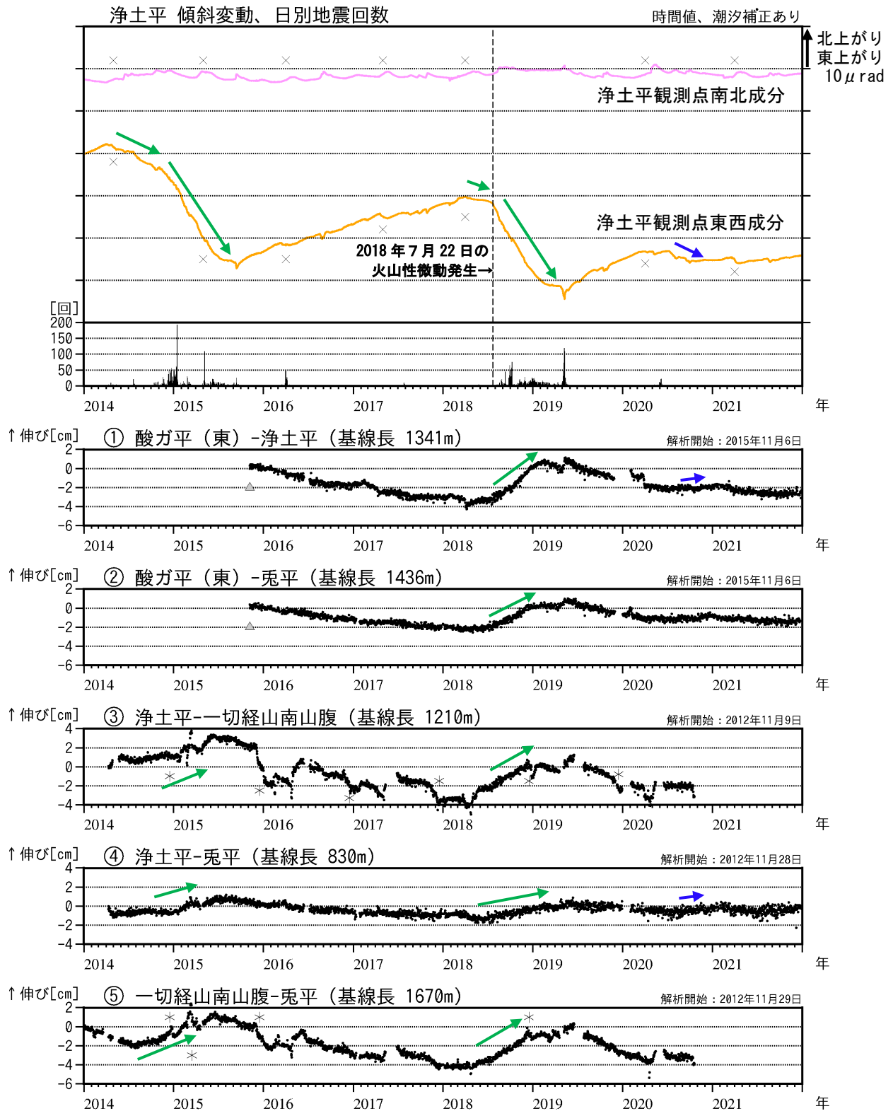
図5 吾妻山 大穴火口浅部の地殻変動（2014年1月～2021年12月）
