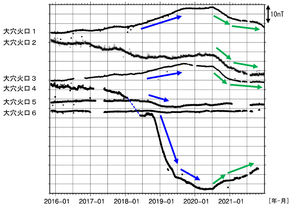
図11 吾妻山 全磁力連続観測点の全磁力値変化（2015年11月～2021年12月）
