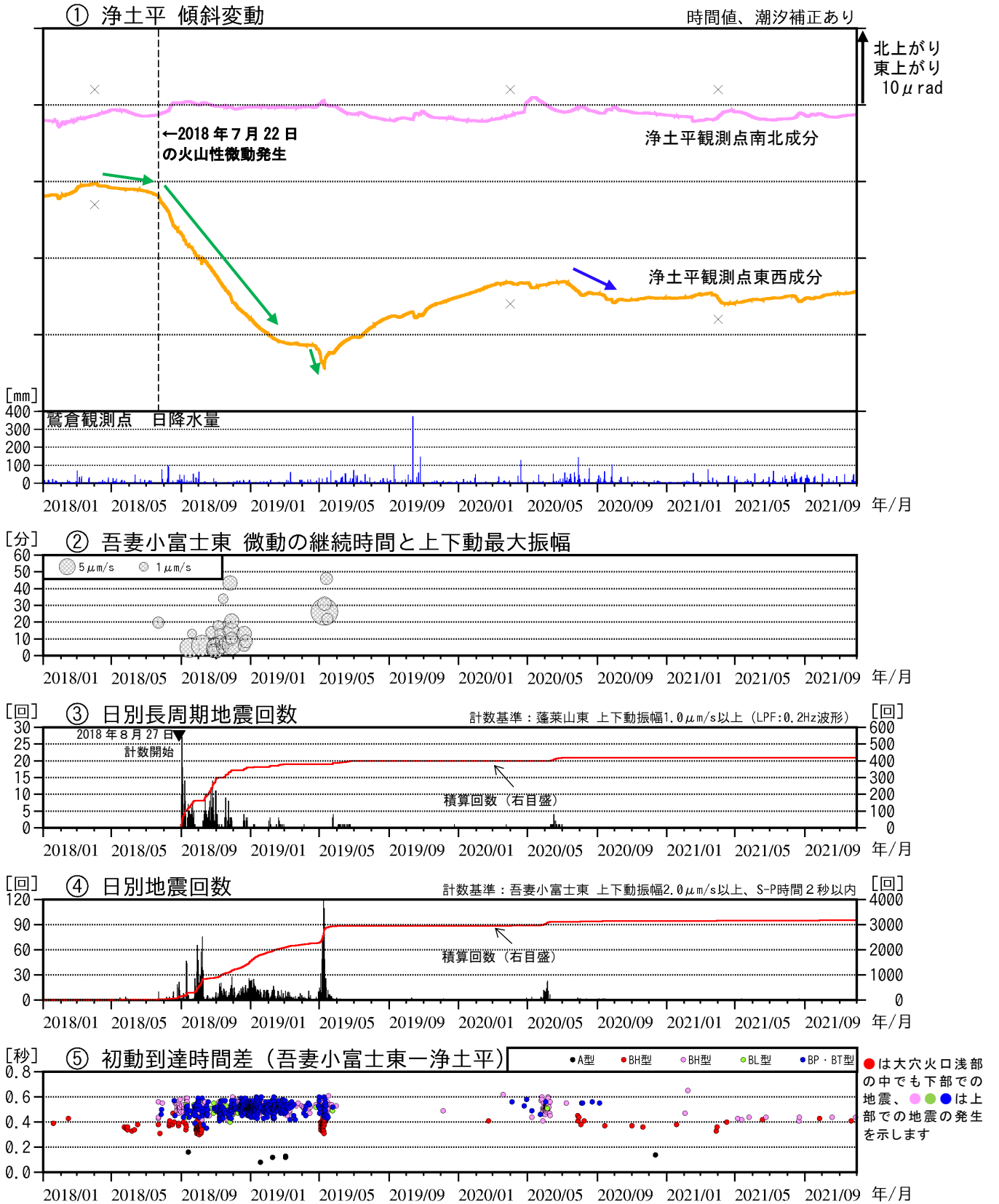
図3 吾妻山 火山活動経過図 (2018年1月~2021年11月)
