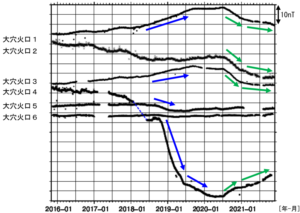
図14 吾妻山 全磁力連続観測点の全磁力値変化 (2015年11月~2021年11月)
