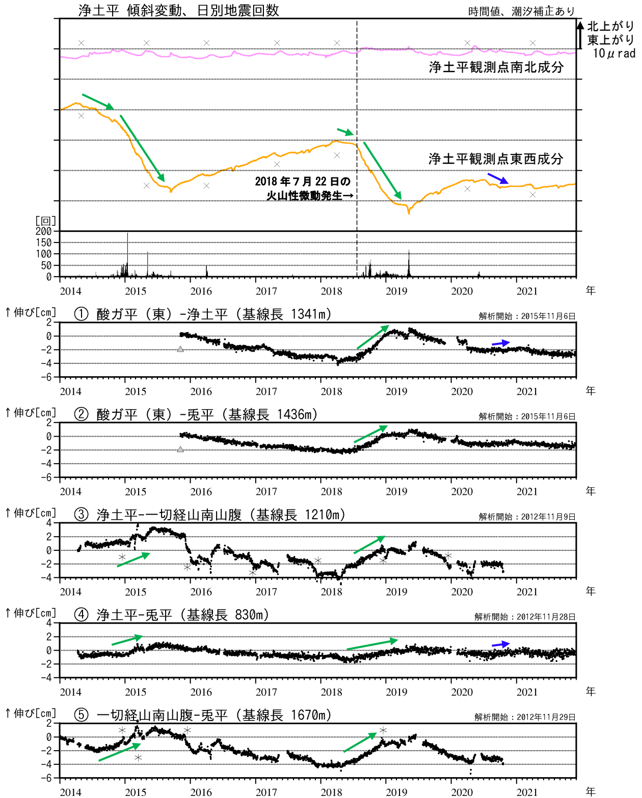
図5 吾妻山 大穴火口浅部の地殻変動（2014年1月～2021年11月）
