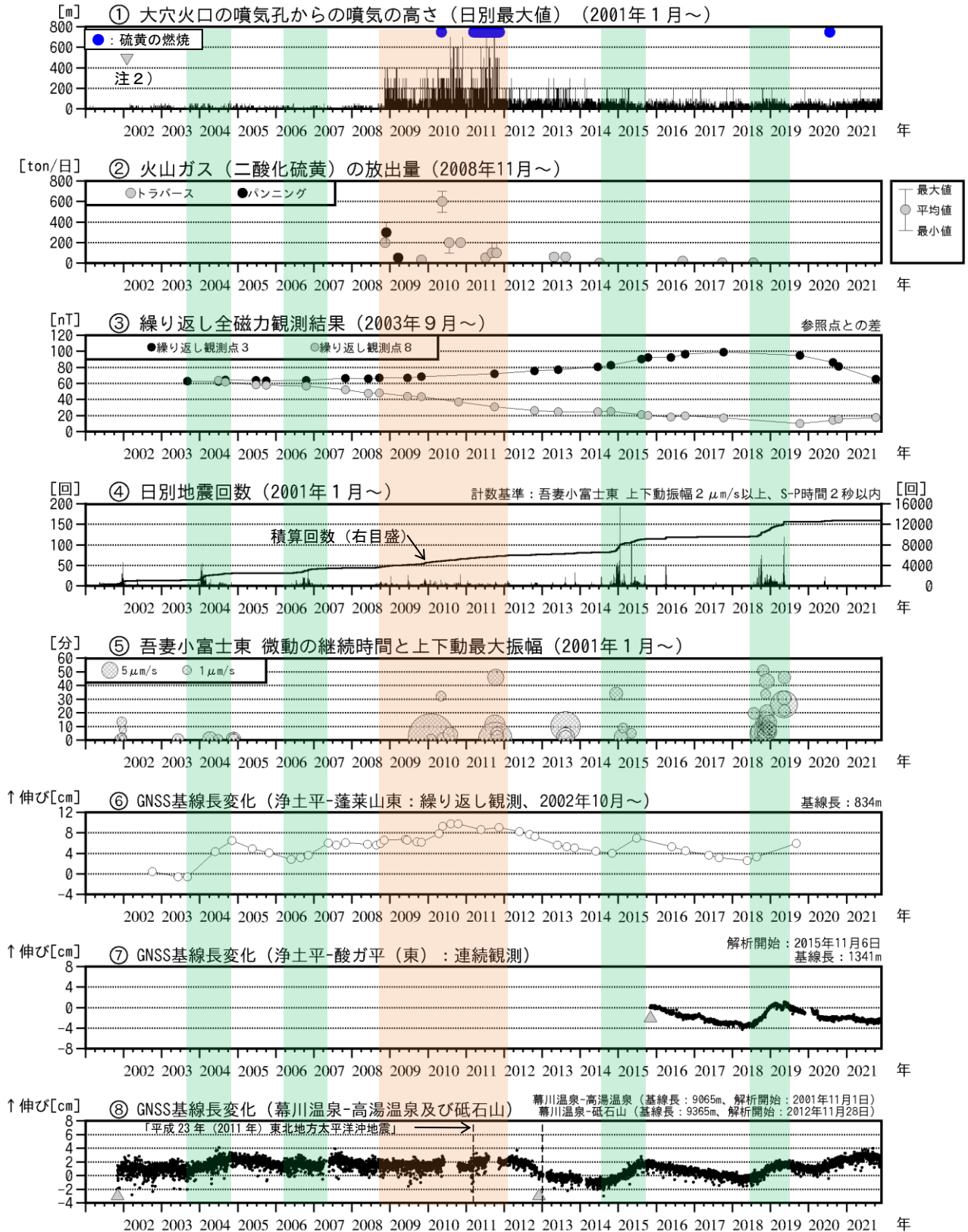
図2 吾妻山 中期的な火山活動の経過（2001年1月～2021年11月）
