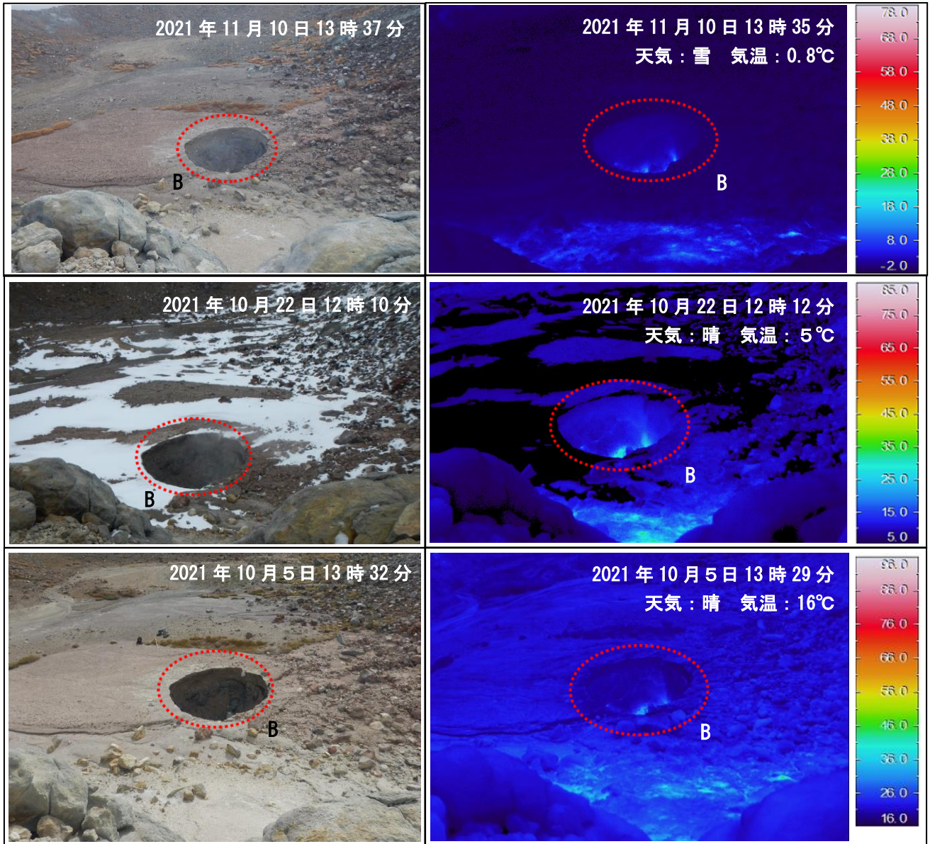
図11 吾妻山 大穴火口内の陥没孔周辺の状況（左）と地表面温度分布（右）
