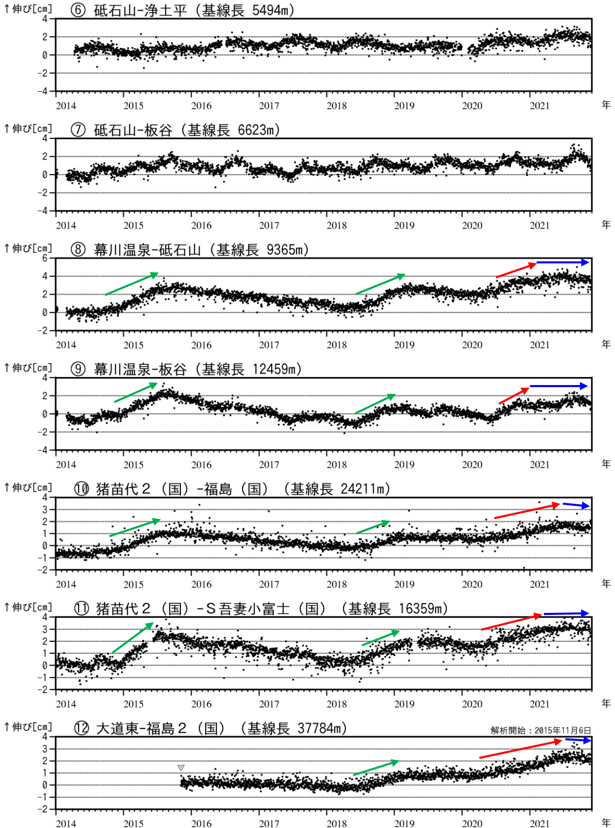
図6 吾妻山 吾妻山深部の地殻変動（2014年1月～2021年11月）
