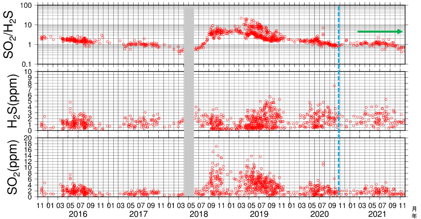
図12 吾妻山 火山ガス観測装置による観測（2015年11月～2021年11月）
