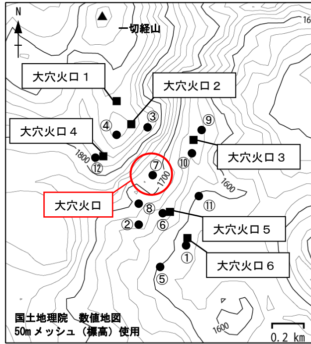
図13 吾妻山 全磁力観測点配置図
