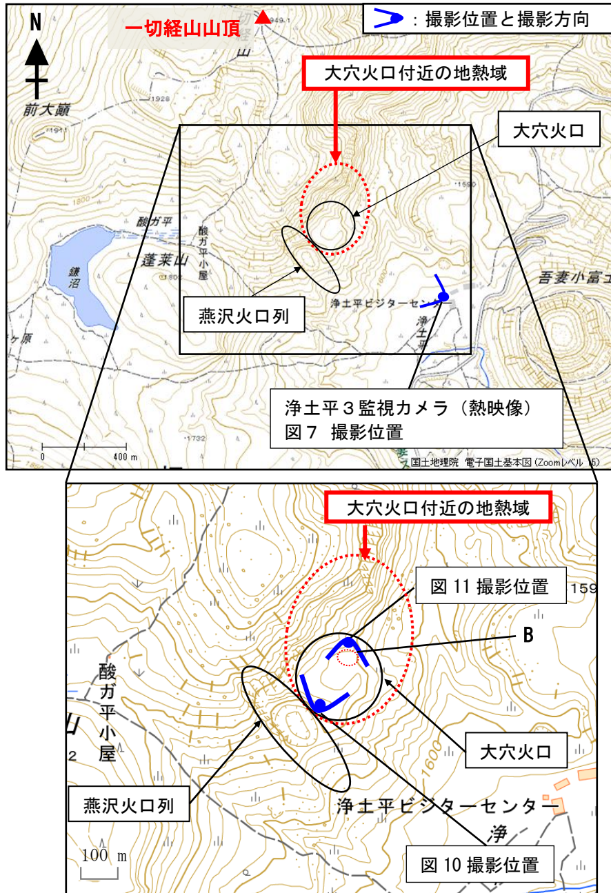
図8 吾妻山 大穴火口周辺の地熱域の分布及び熱映像撮影方向
