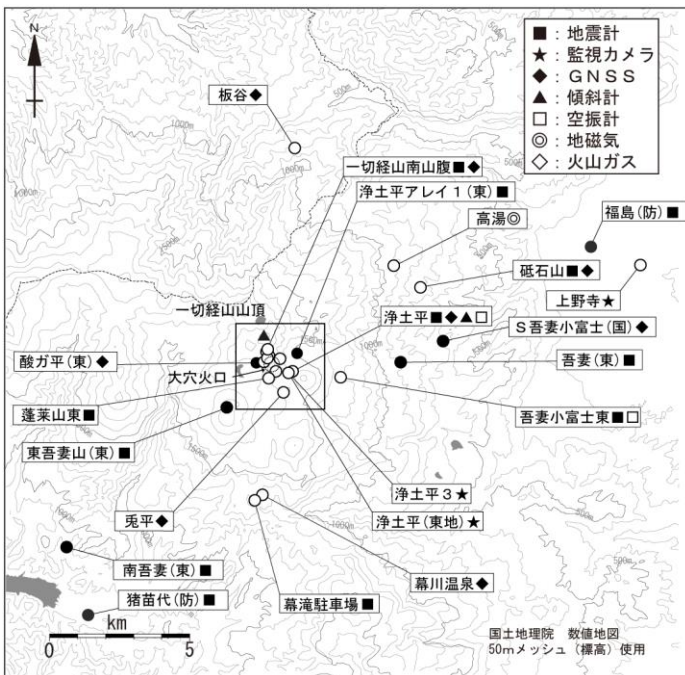
図 16 吾妻山 観測点配置図
