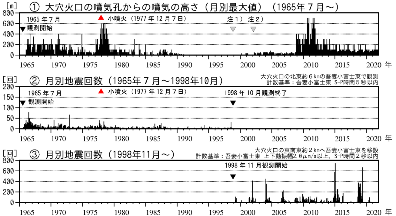
図1 吾妻山 長期的な火山活動の経過（1965年7月～2021年11月）
