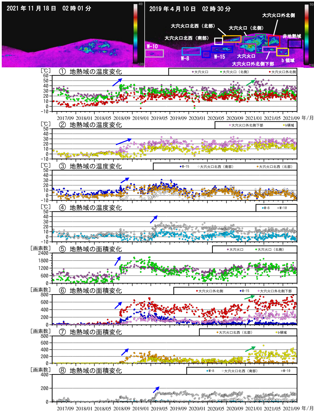
図7 吾妻山 監視カメラによる大穴火口周辺の地熱域の経過（2017年8月～2021年11月）
