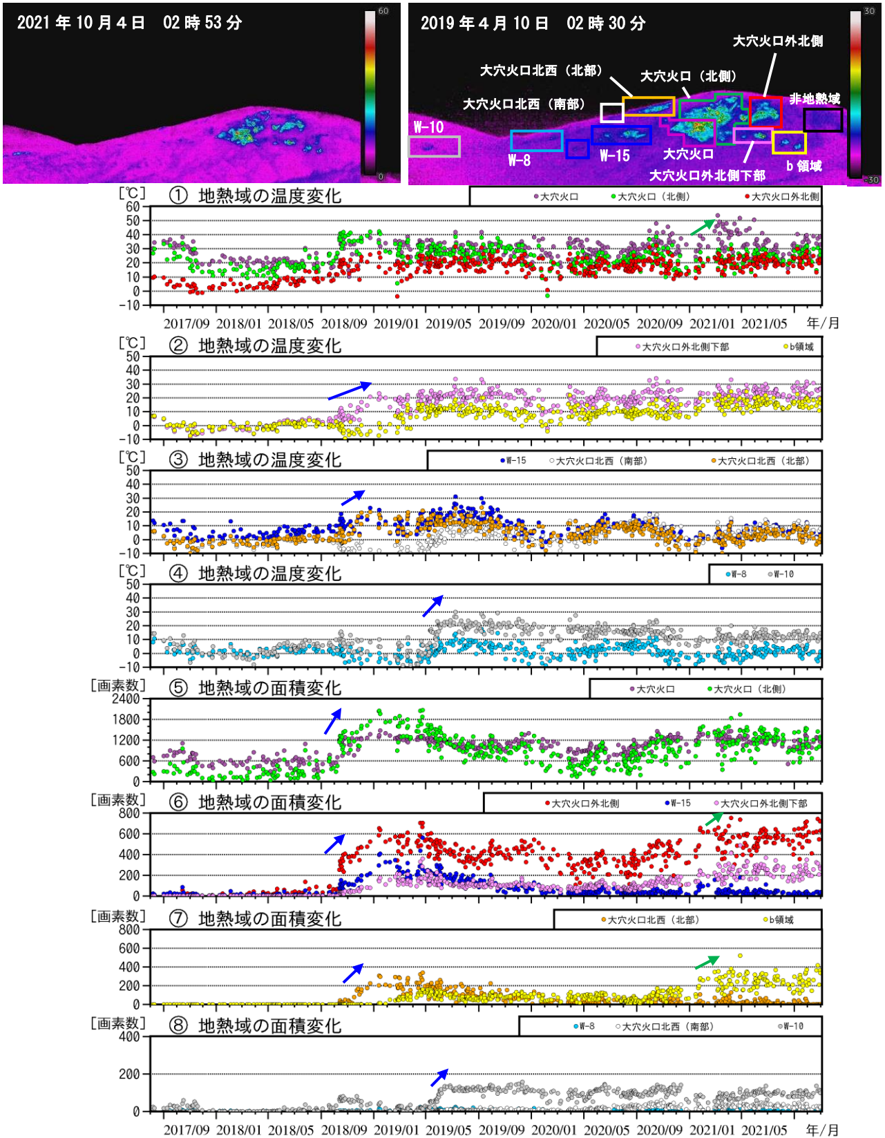
図7 吾妻山 監視カメラによる大穴火口周辺の地熱域の経過（2017年8月～2021年10月）
