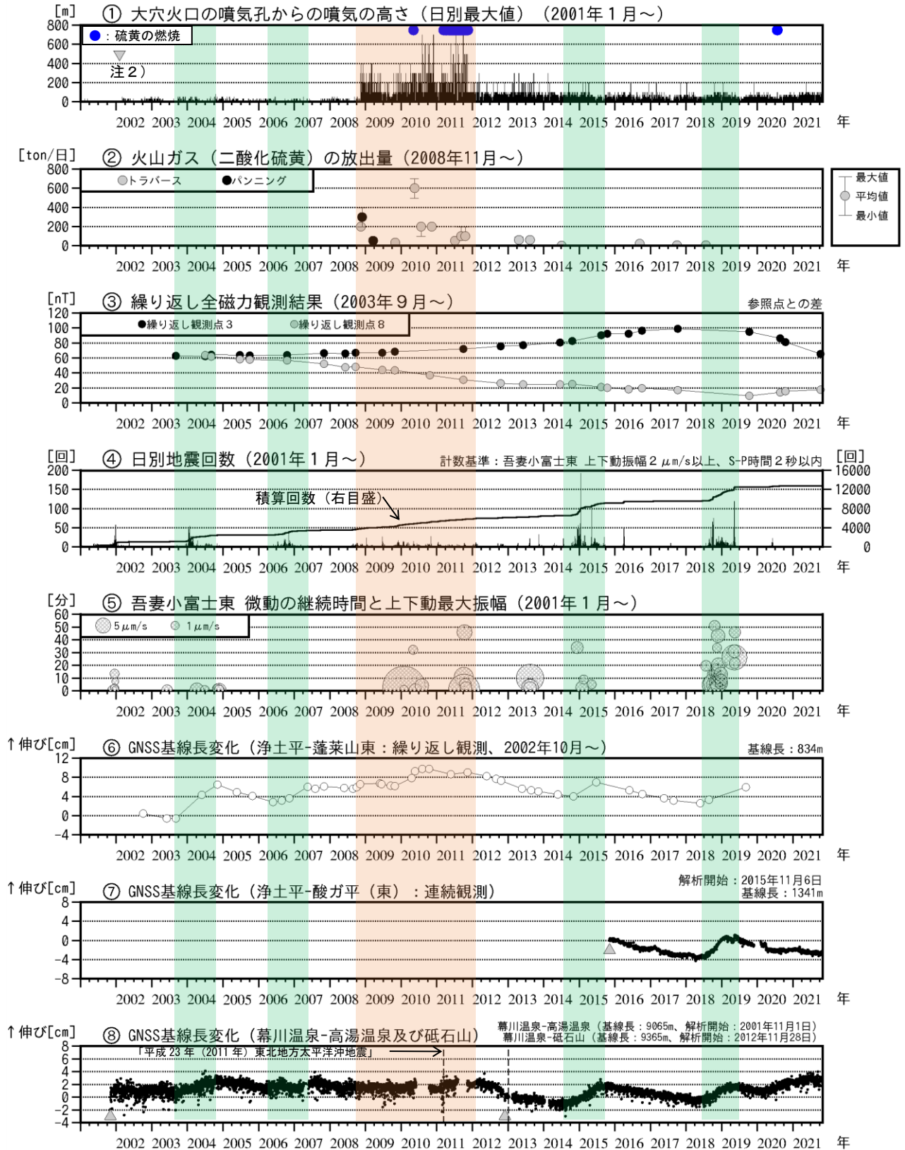
図2 吾妻山 中期的な火山活動の経過（2001年1月～2021年10月）
