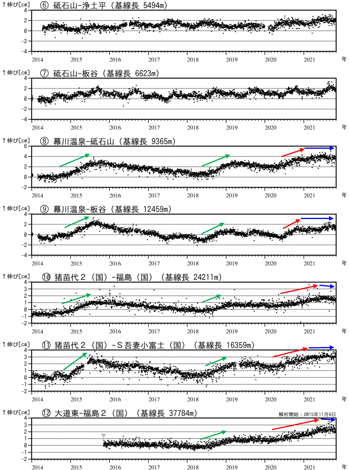
図6 吾妻山 吾妻山深部の地殻変動（2014年1月～2021年10月）
