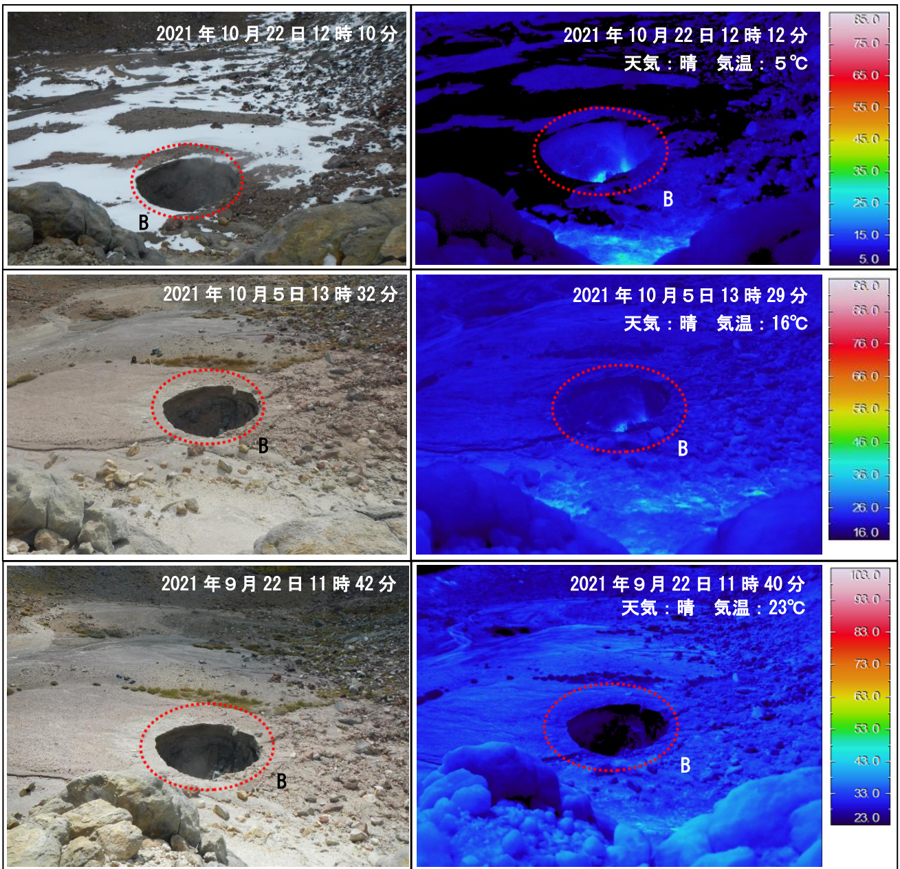
図 11 吾妻山 大穴火口内の陥没孔周辺の状況（左）と地表面温度分布（右）
