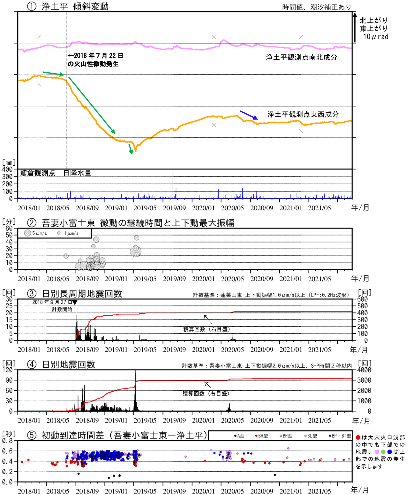
図3 吾妻山 火山活動経過図（2018年1月～2021年10月）
