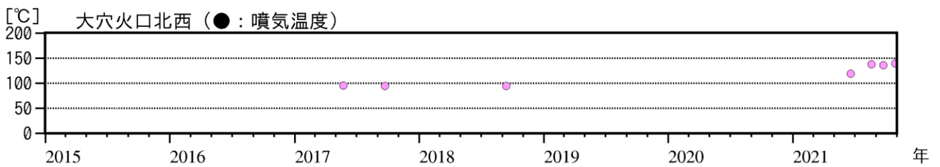
図16 吾妻山 大穴火口北西の噴気温度の経過（2015年1月～2021年10月）
