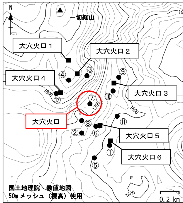
図 19 吾妻山 全磁力観測点配置図
