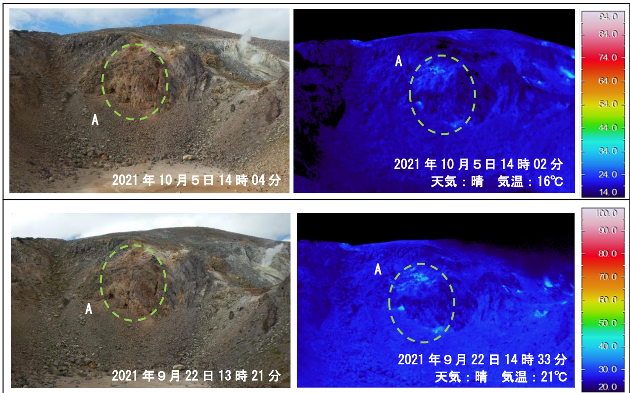
図13 吾妻山 燕沢火口列北側火口壁の状況（左）と地表面温度分布（右）
