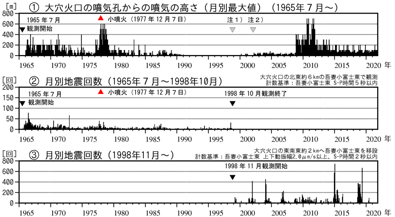
図1 吾妻山 長期的な火山活動の経過（1965年7月～2021年10月）
