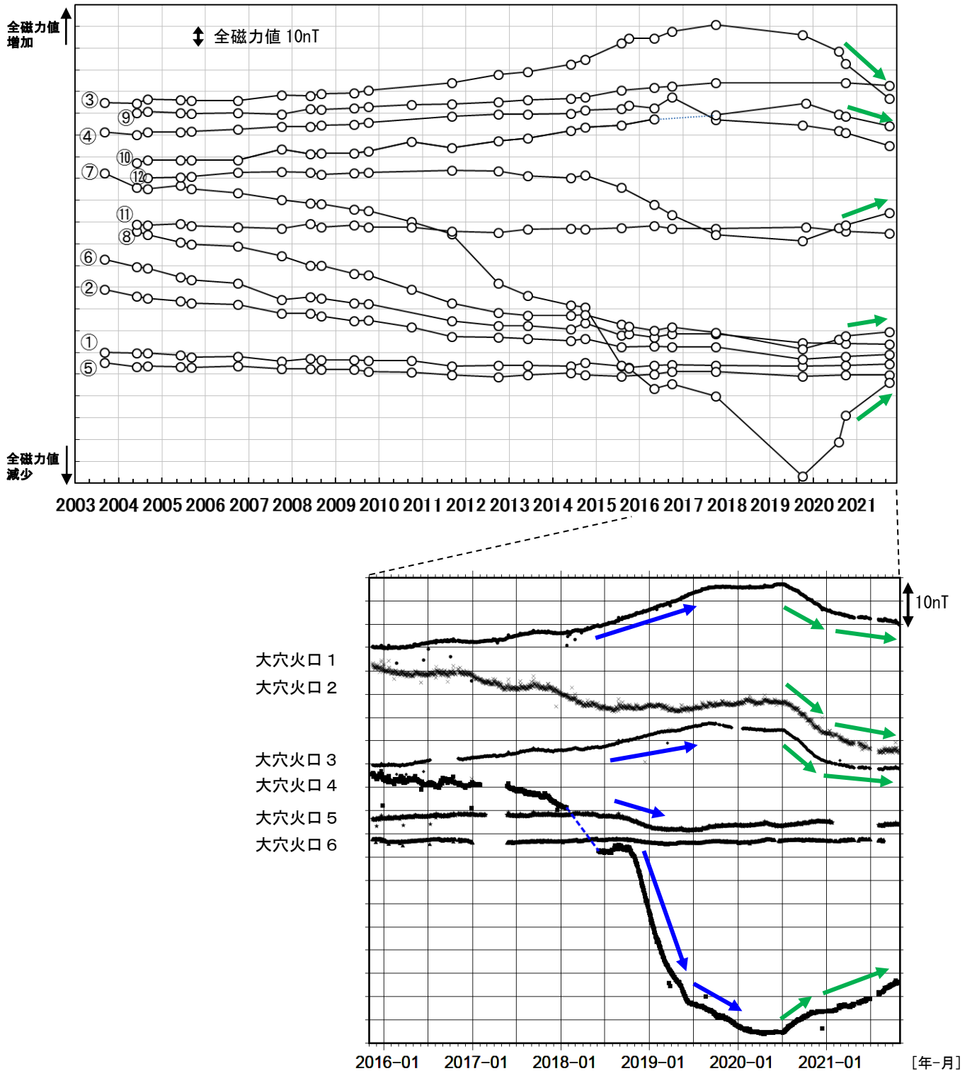
図 18 吾妻山 全磁力繰り返し観測（上）及び連続観測（下）の全磁力値変化 (2003年9月～2021年10月)
