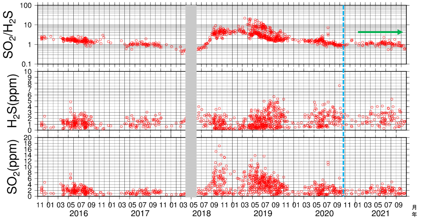
図17 吾妻山 火山ガス観測装置による観測（2015年11月～2021年10月）
