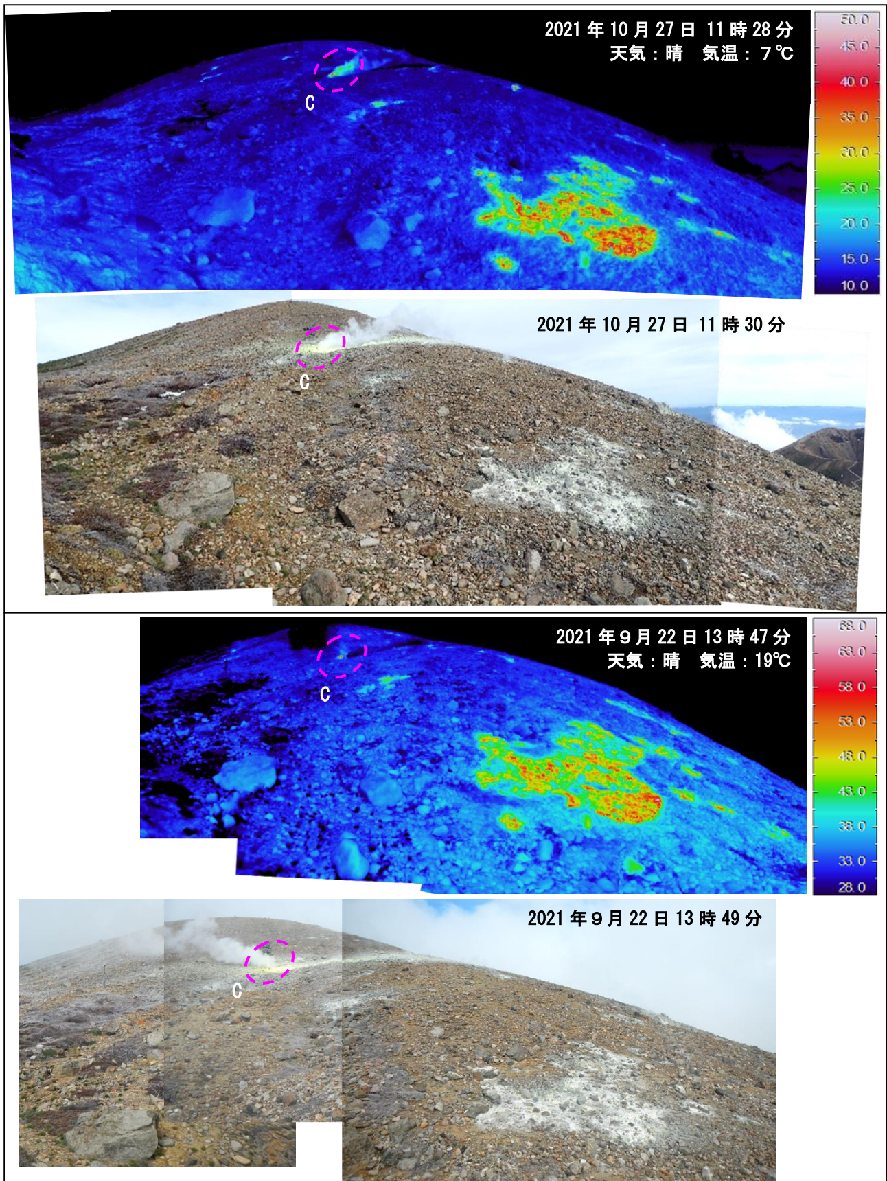
図14 吾妻山 大穴火口北西の状況（下）と地表面温度分布（上）
