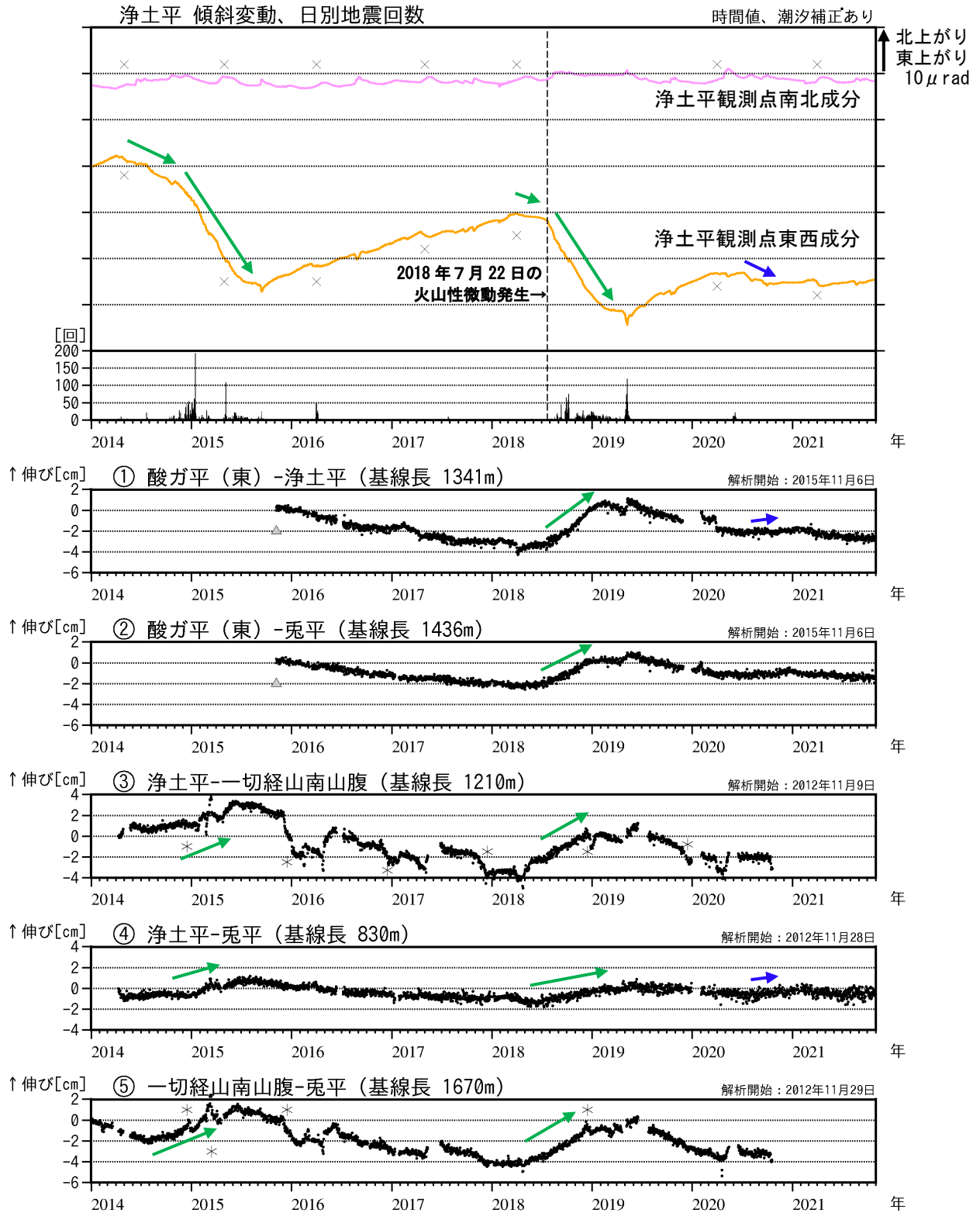
図5 吾妻山 大穴火口浅部の地殻変動（2014年1月～2021年10月）
