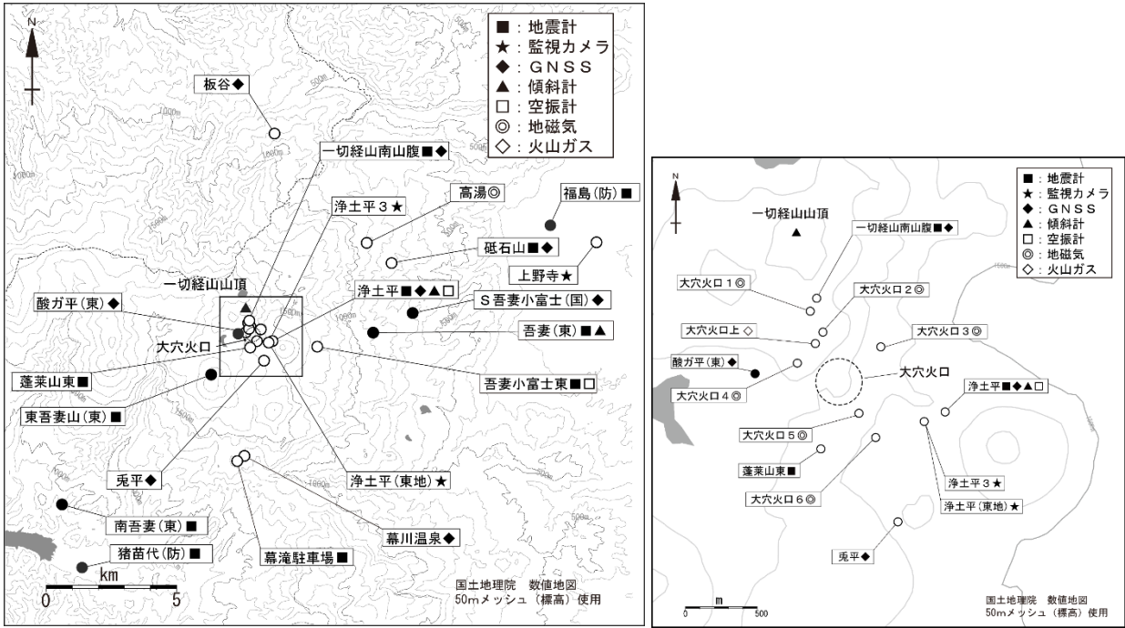
図 21 吾妻山 観測点配置図
