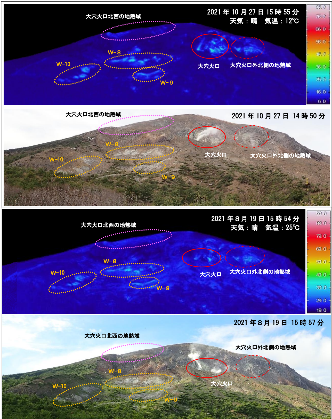
図15 吾妻山 大穴火口付近及び八幡焼の状況（下）と地表面温度分布（上）
