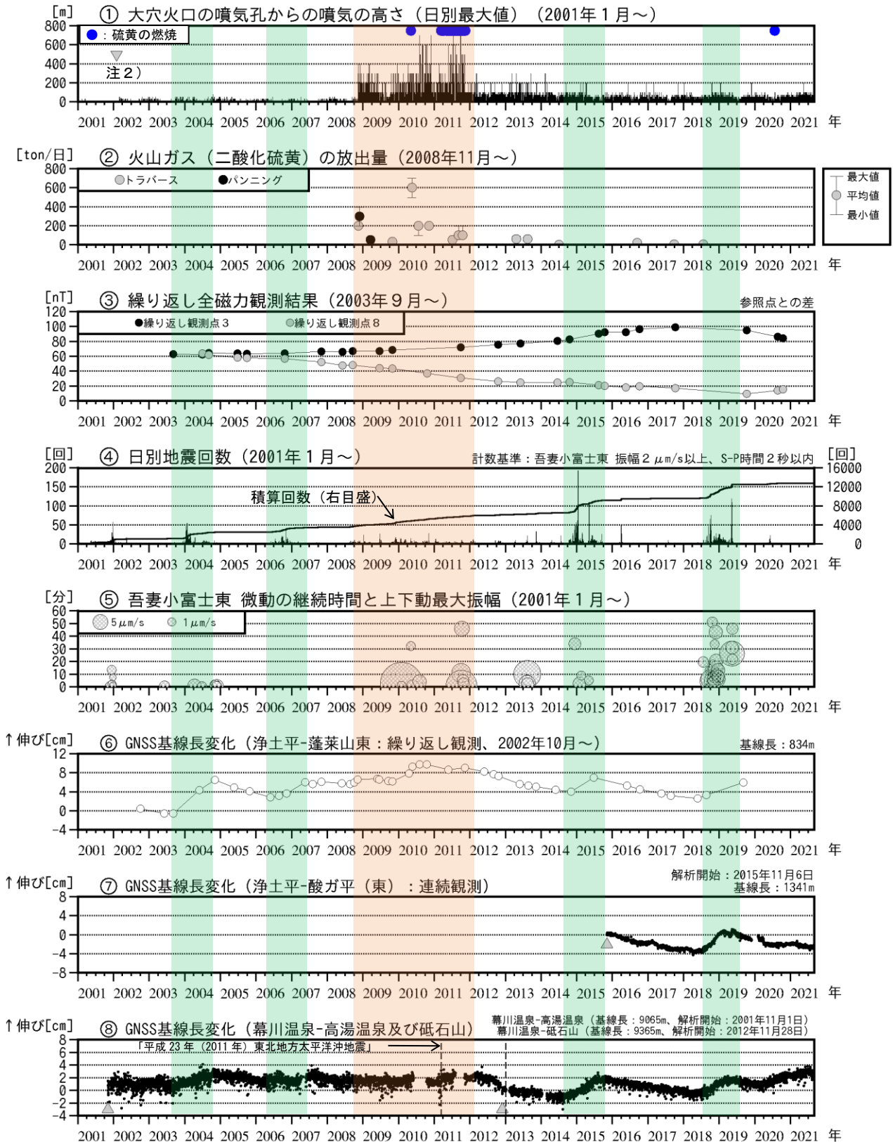
図2 吾妻山 中期的な火山活動の経過（2001年1月～2021年8月）
