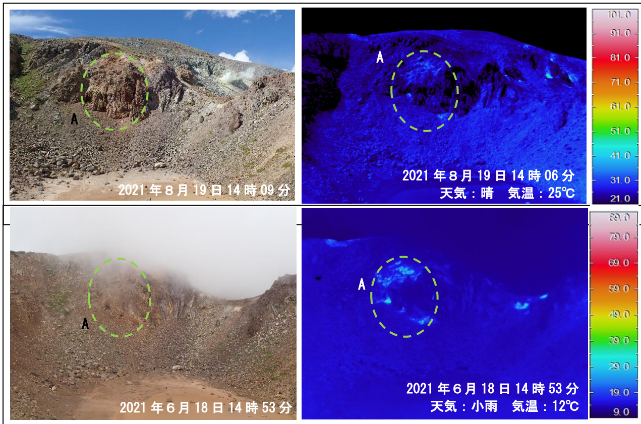
図11 吾妻山 燕沢火口列北側火口壁の状況（左）と地表面温度分布（右）
