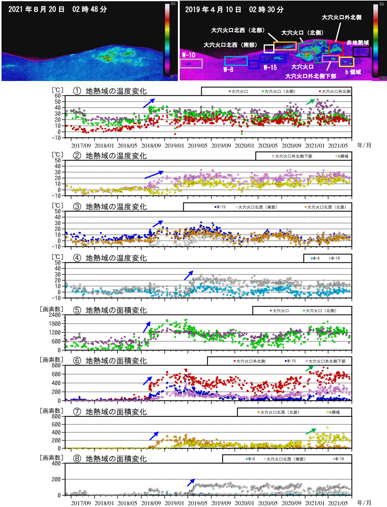
図7 吾妻山 監視カメラによる大穴火口周辺の地熱域の経過（2017年8月～2021年8月）
