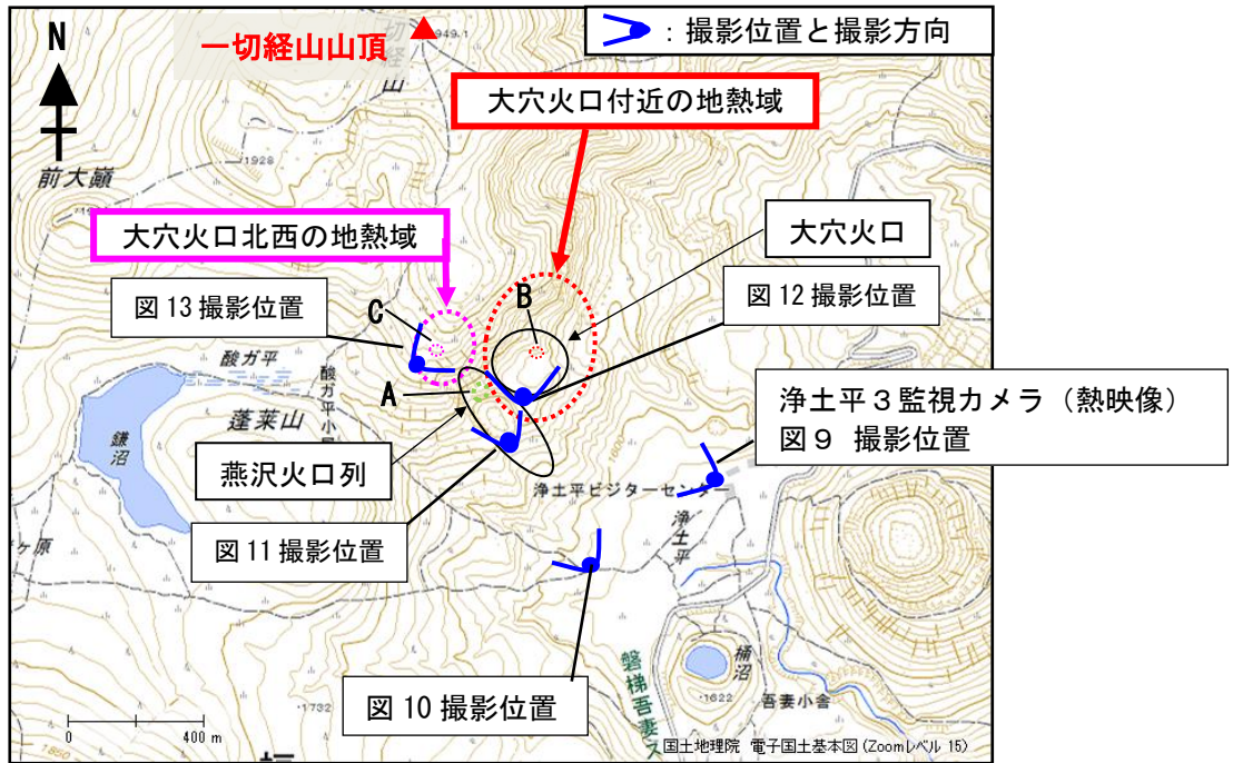
図8 吾妻山 大穴火口周辺の地熱域の分布及び熱映像撮影方向
