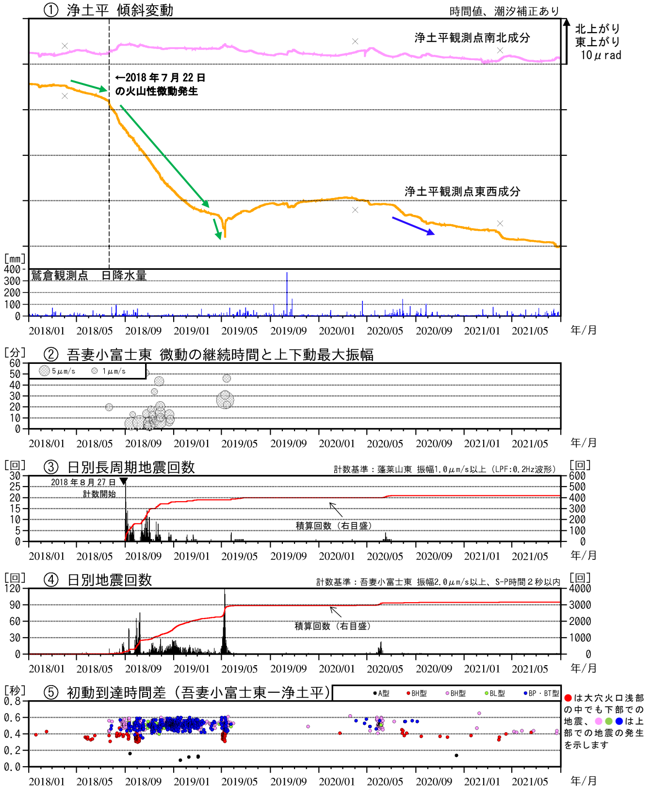
図3 吾妻山 火山活動経過図（2018年1月～2021年8月）
