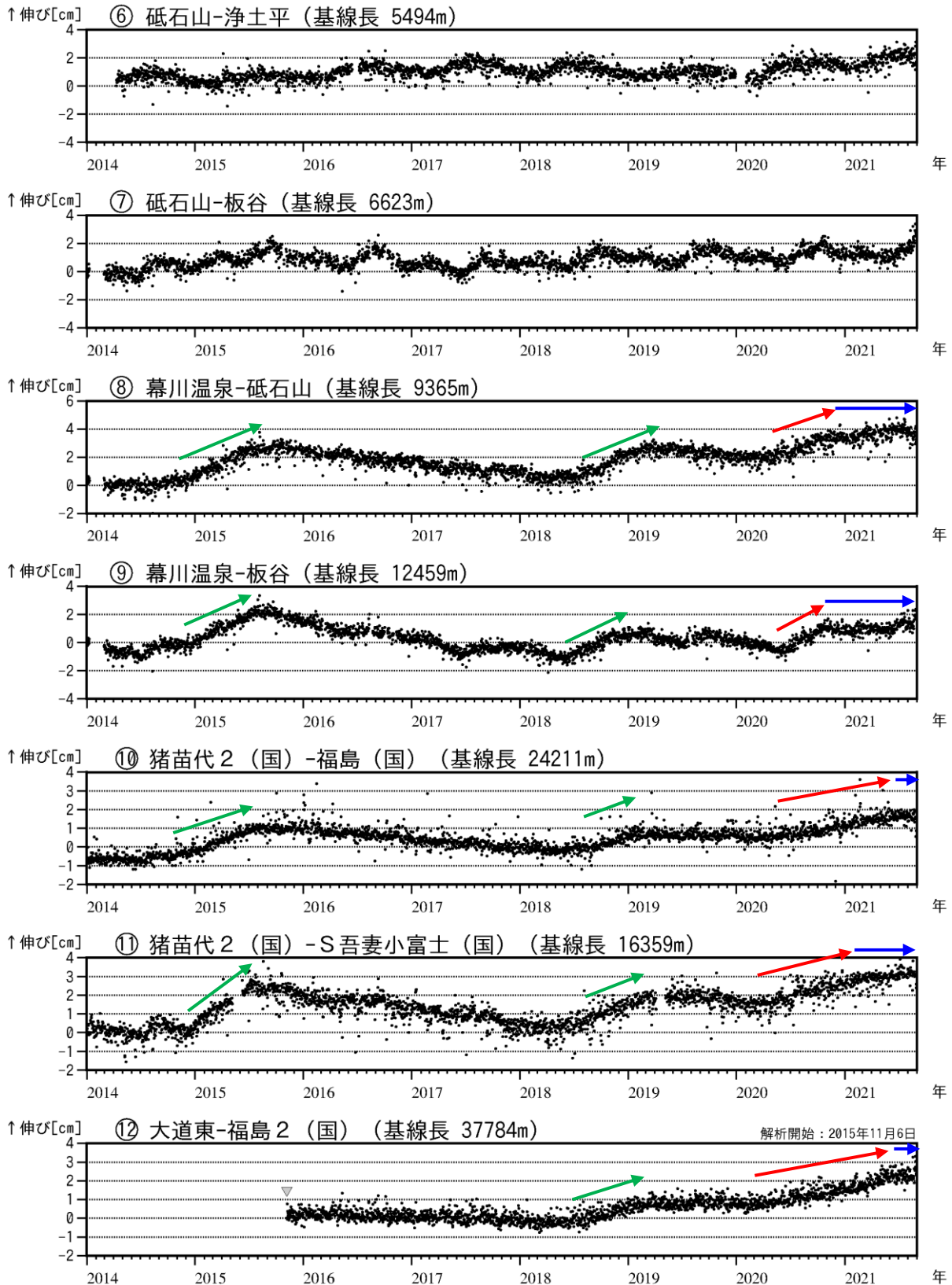
図6 吾妻山 吾妻山深部の地殻変動（2014年1月～2021年8月）
