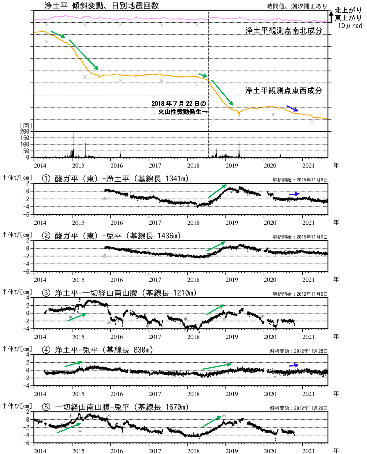
図5 吾妻山 大穴火口浅部の地殻変動（2014年1月～2021年8月）
