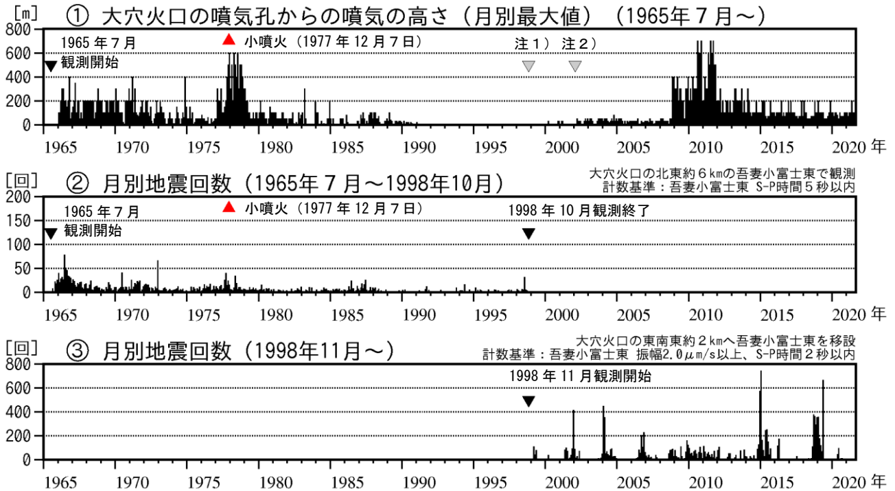
図1 吾妻山 長期的な火山活動の経過（1965年7月～2021年8月）
