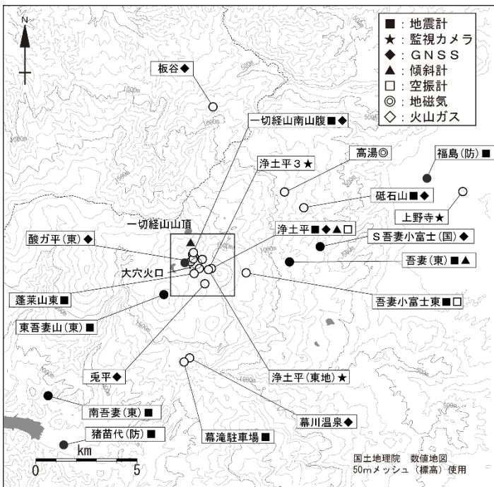
図 19 吾妻山 観測点配置図
