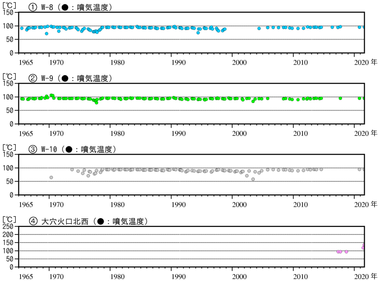
図14 吾妻山 大穴火口周辺の噴気温度の経過（1965年7月～2021年8月）
