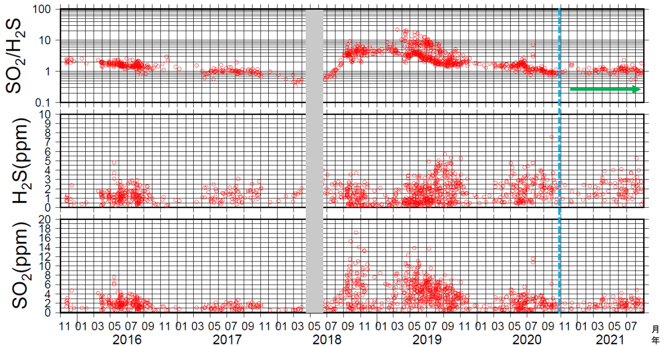
図15 吾妻山 火山ガス観測装置による観測（2015年11月～2021年8月）
