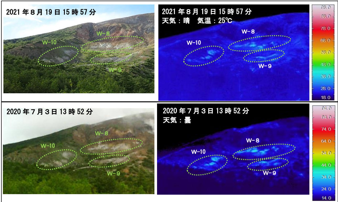
図10 吾妻山 八幡焼の状況（左）と地表面温度分布（右）
