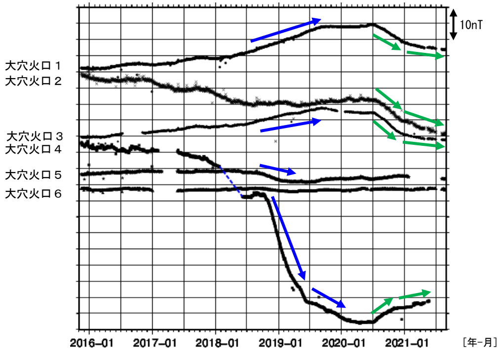
図 17 吾妻山 全磁力連続観測点の全磁力値変化（2015年11月～2021年8月）
