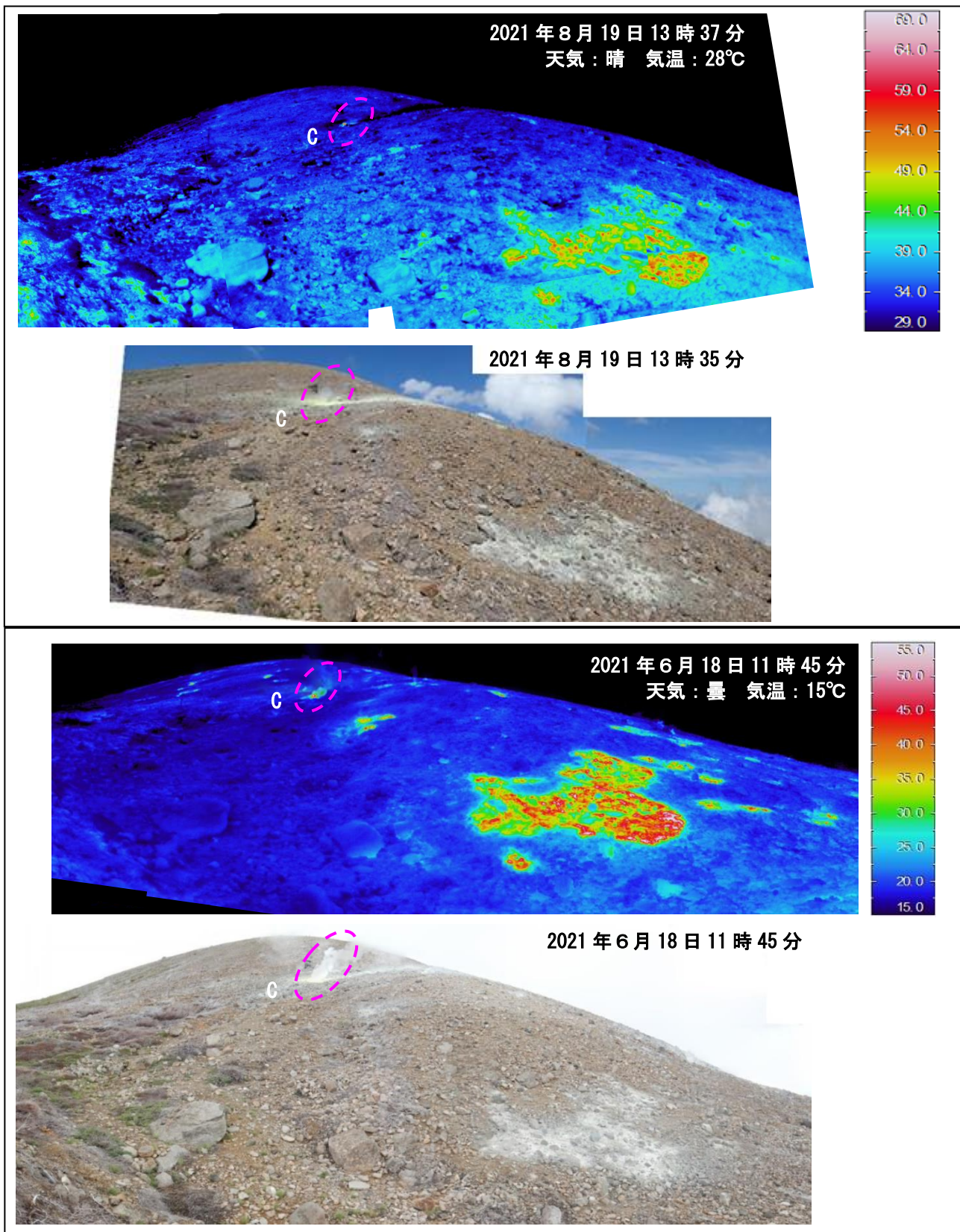
図13 吾妻山 大穴火口北西の状況（下）と地表面温度分布（上）
