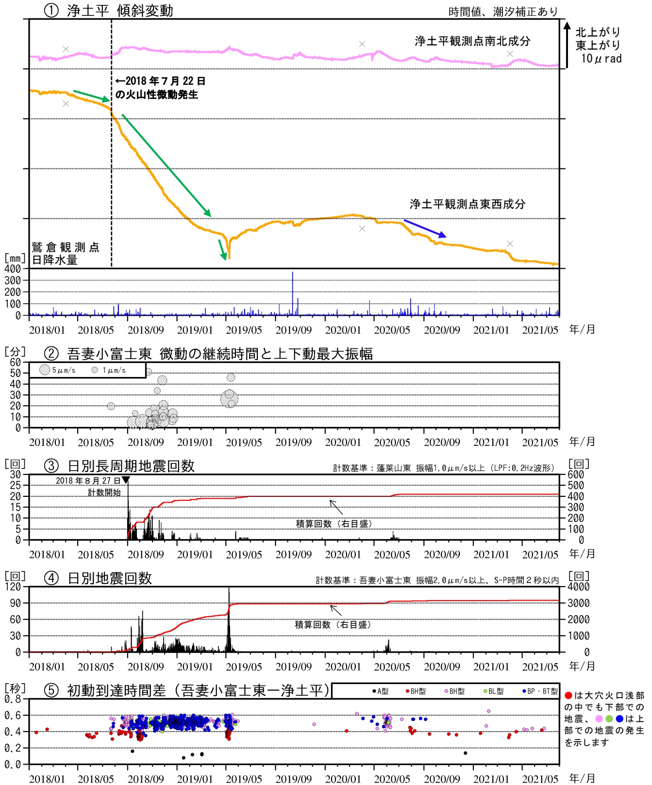
図3 吾妻山 火山活動経過図（2018年1月～2021年7月）
