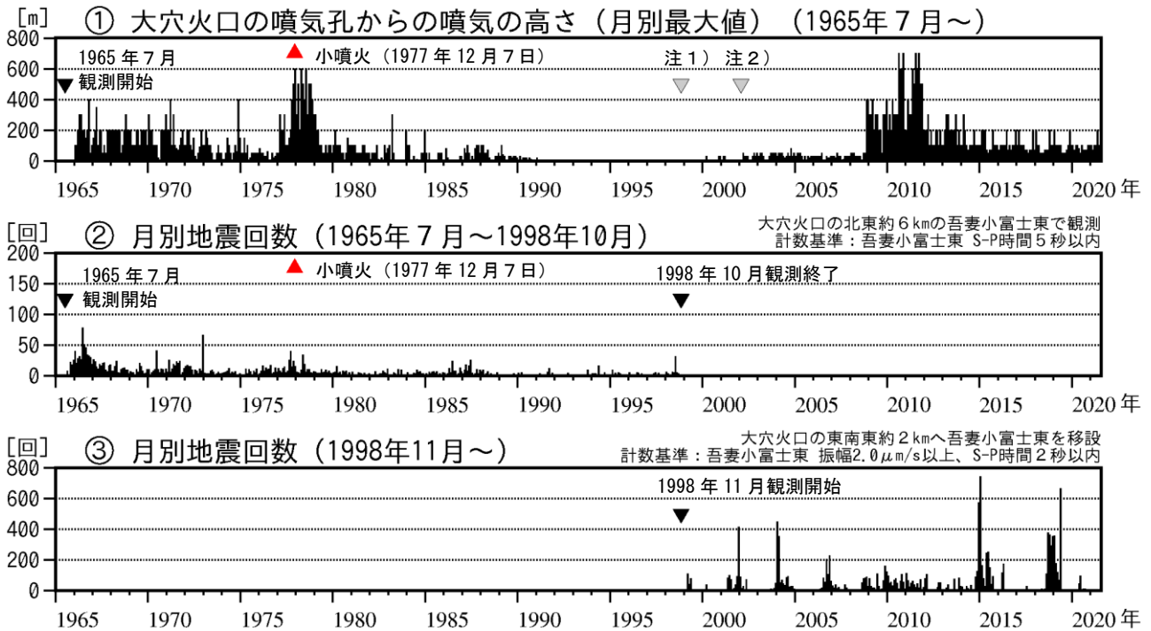
図1 吾妻山 長期的な火山活動の経過（1965年7月～2021年7月）
