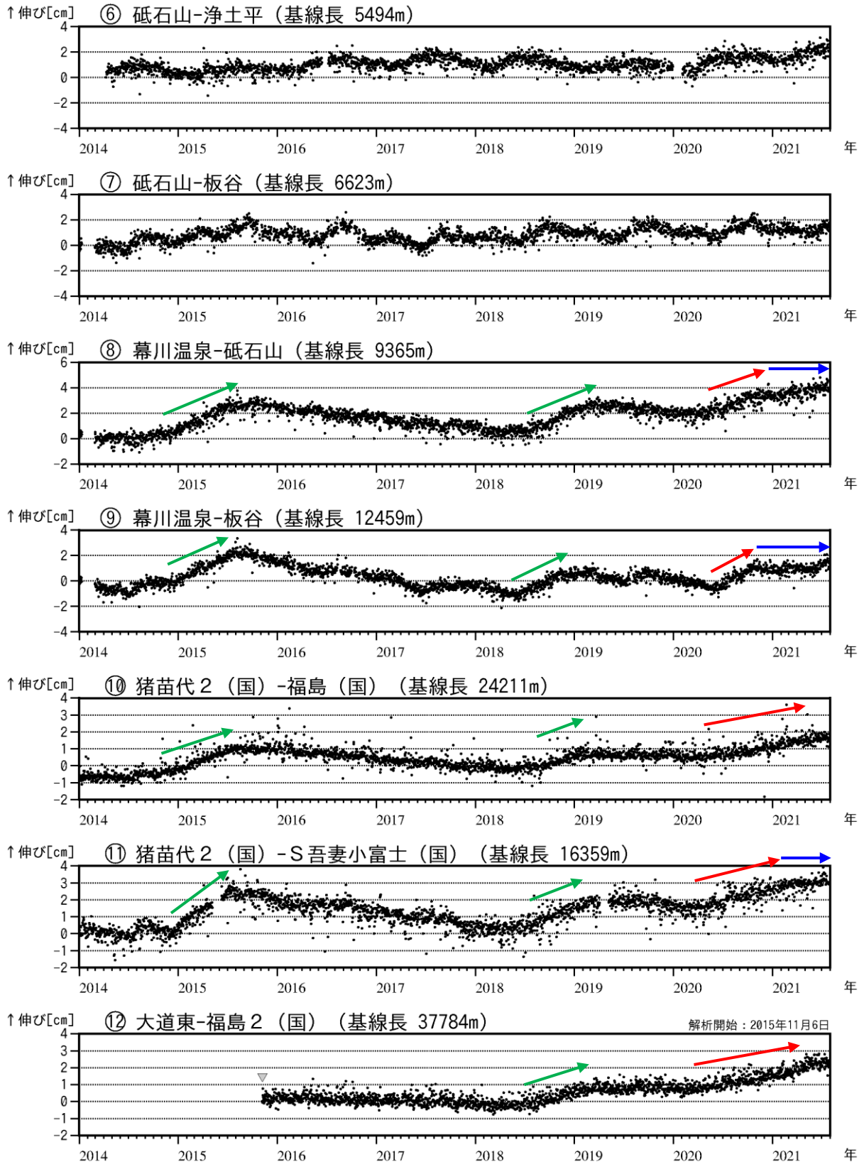
図6 吾妻山 吾妻山深部の地殻変動（2014年1月～2021年7月）
