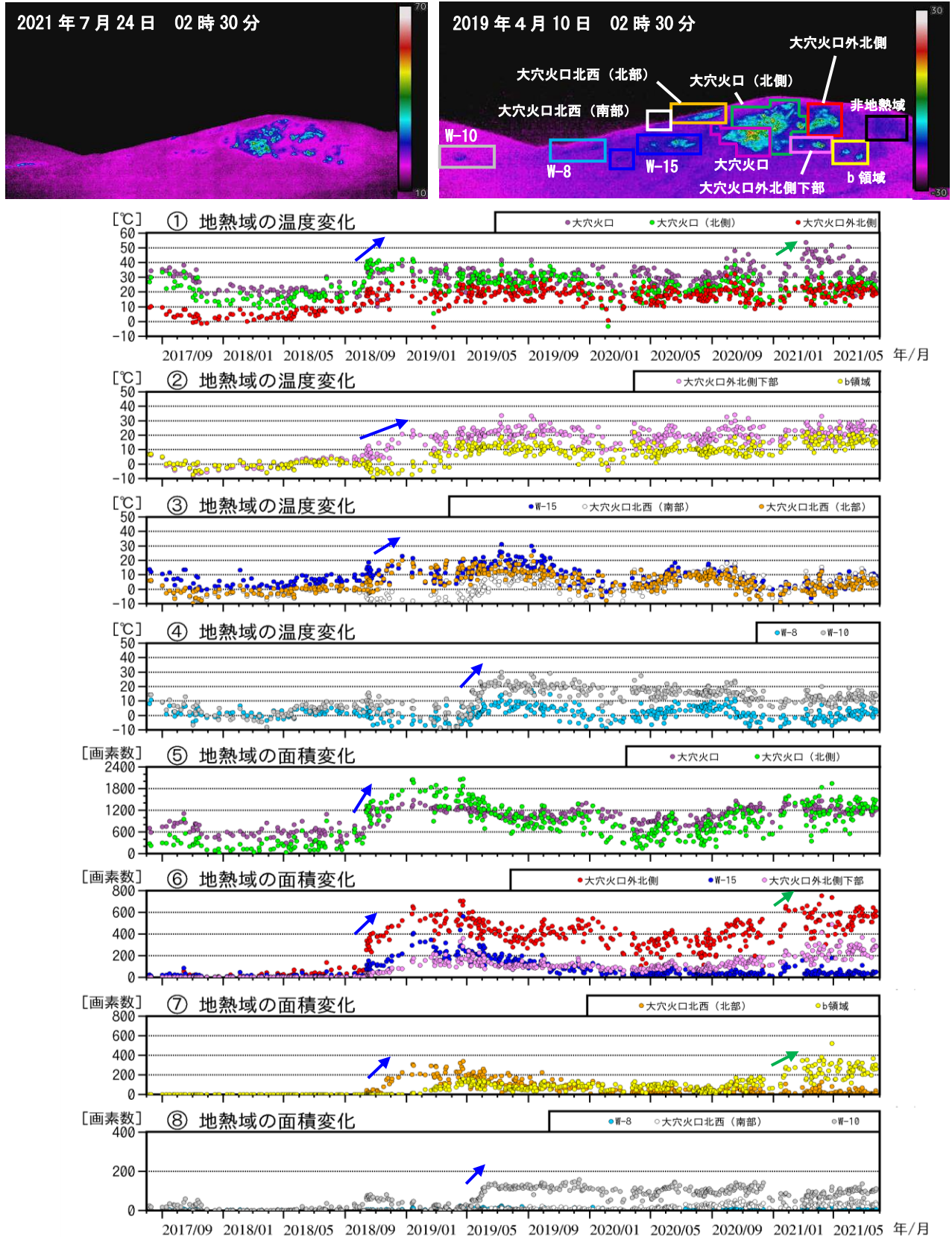
図7 吾妻山 監視カメラによる大穴火口周辺の地熱域の経過（2017年8月～2021年7月）
