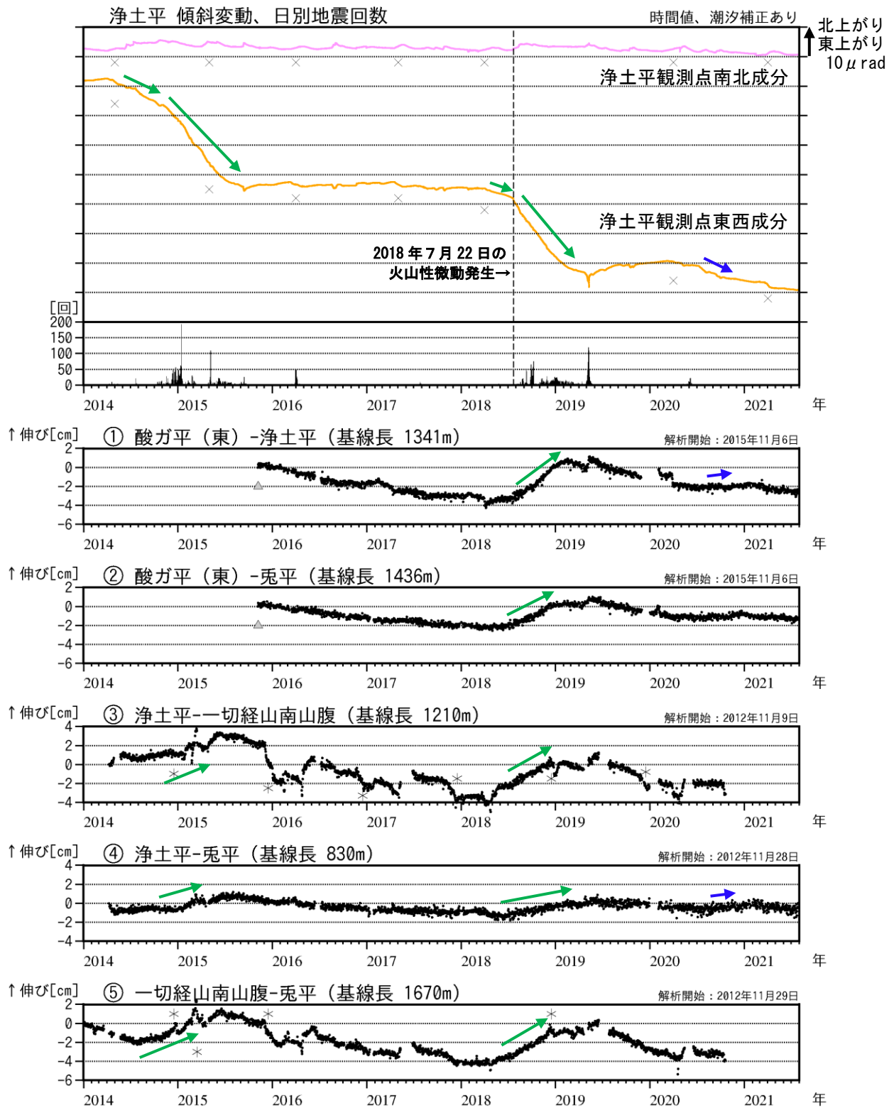
図5 吾妻山 大穴火口浅部の地殻変動（2014年1月～2021年7月）
