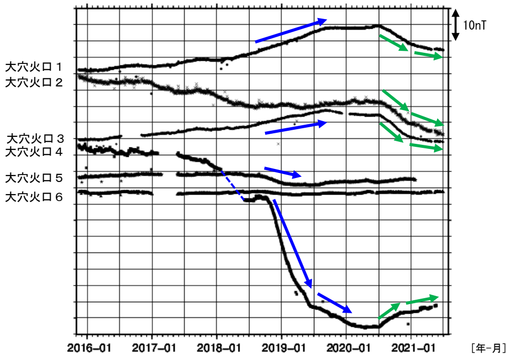
図11 吾妻山 全磁力連続観測点の全磁力値変化（2015年11月～2021年7月）
