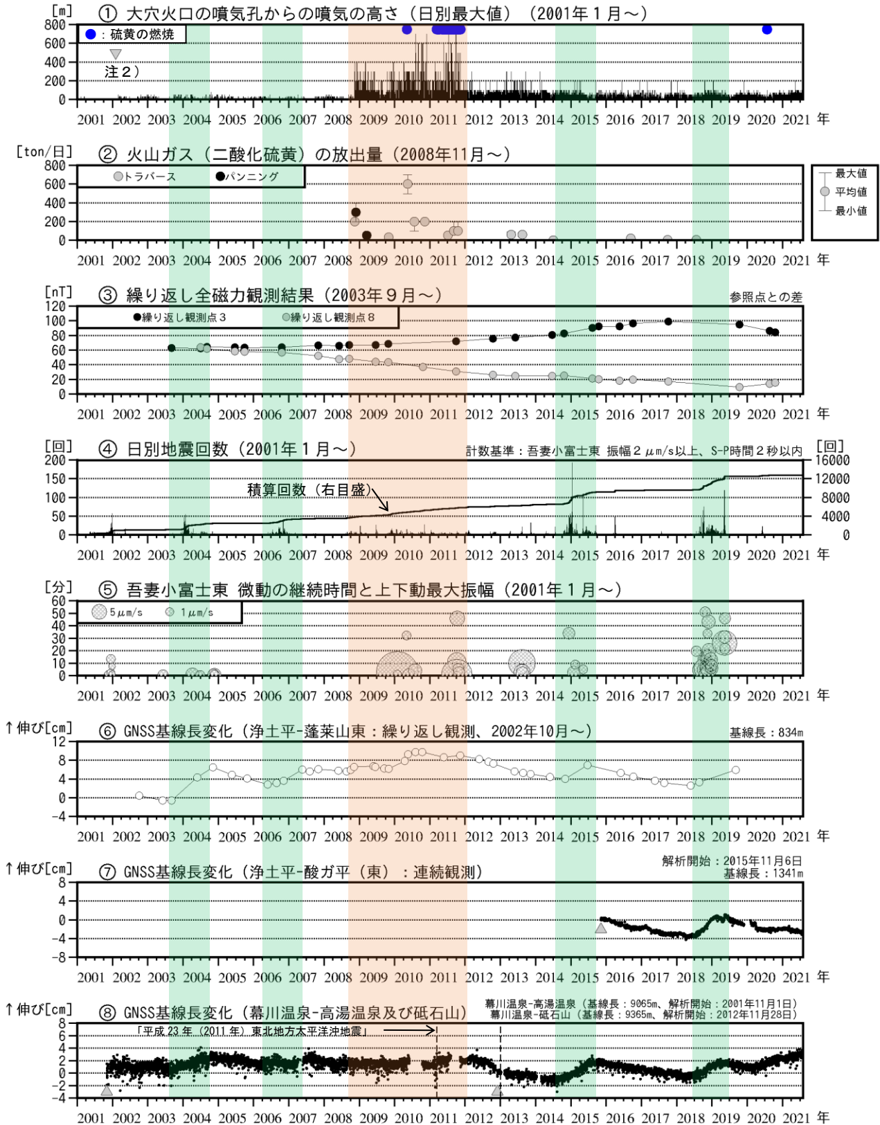
図2 吾妻山 中期的な火山活動の経過（2001年1月～2021年7月）
