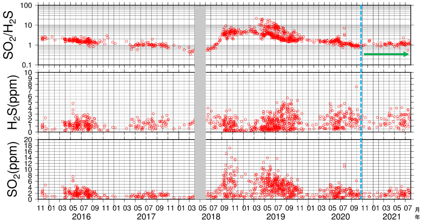
図9 吾妻山 火山ガス観測装置による観測（2015年11月～2021年7月）
