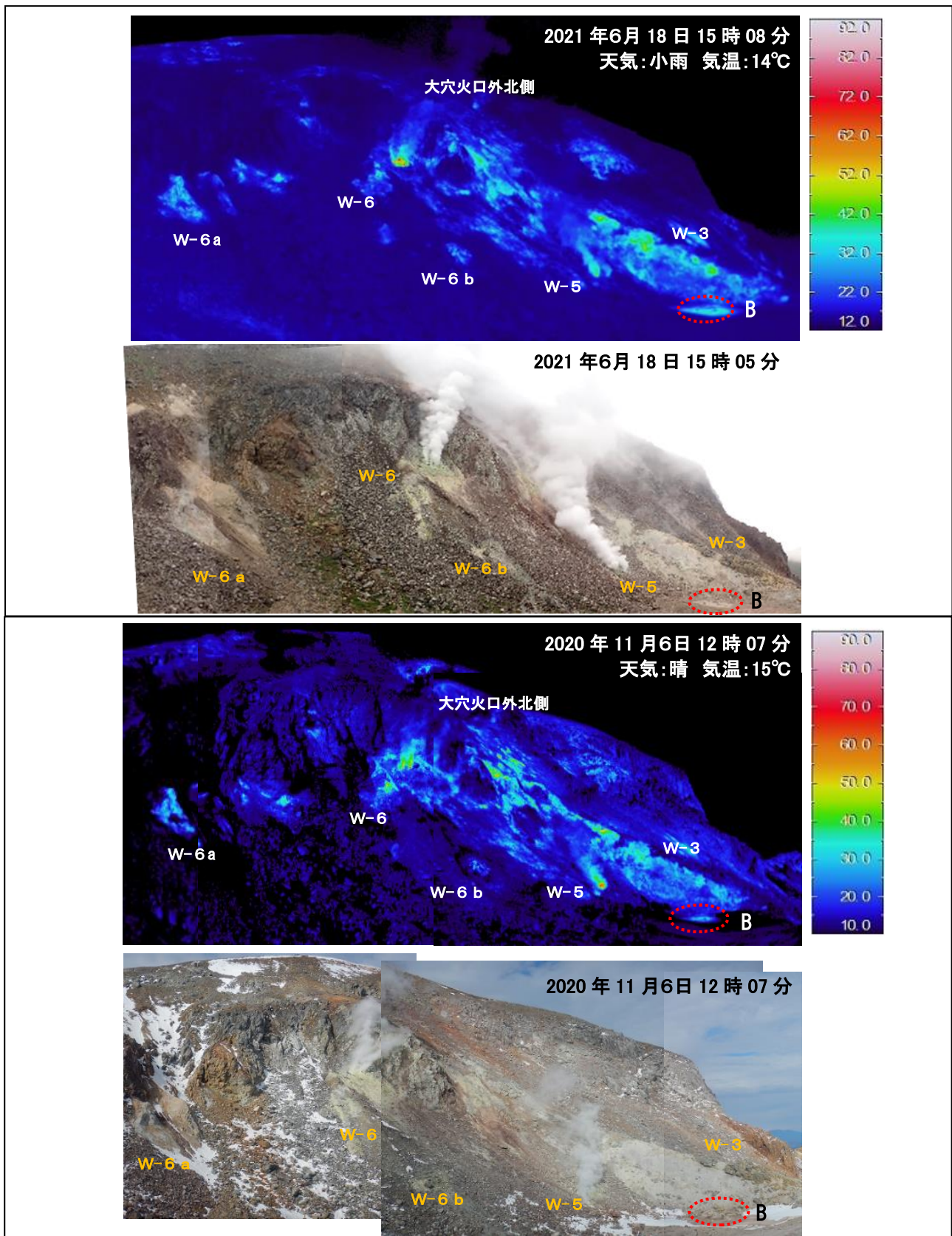
図 11 吾妻山 大穴火口付近及びその周辺の状況（下）と地表面温度分布（上）
