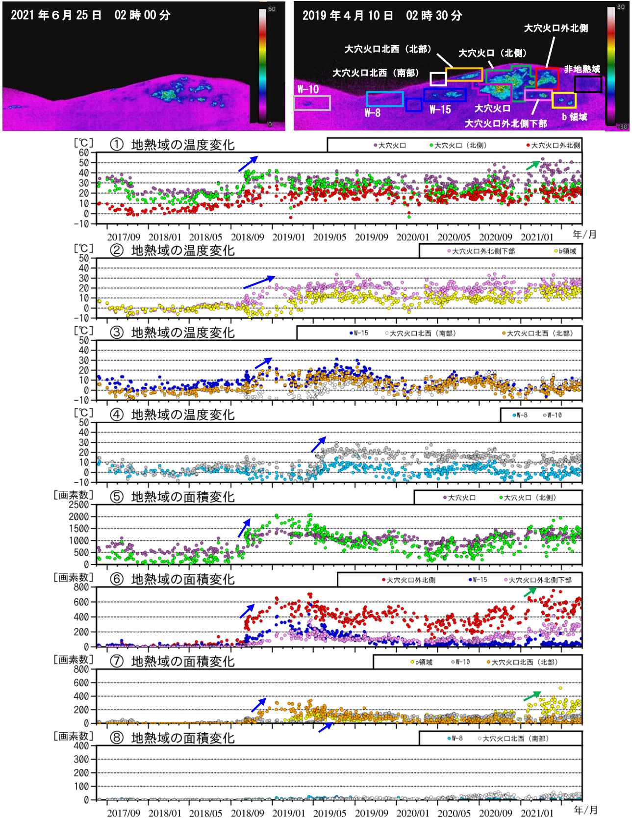
図7 吾妻山 監視カメラによる大穴火口周辺の地熱域の経過（2017年8月～2021年6月）
