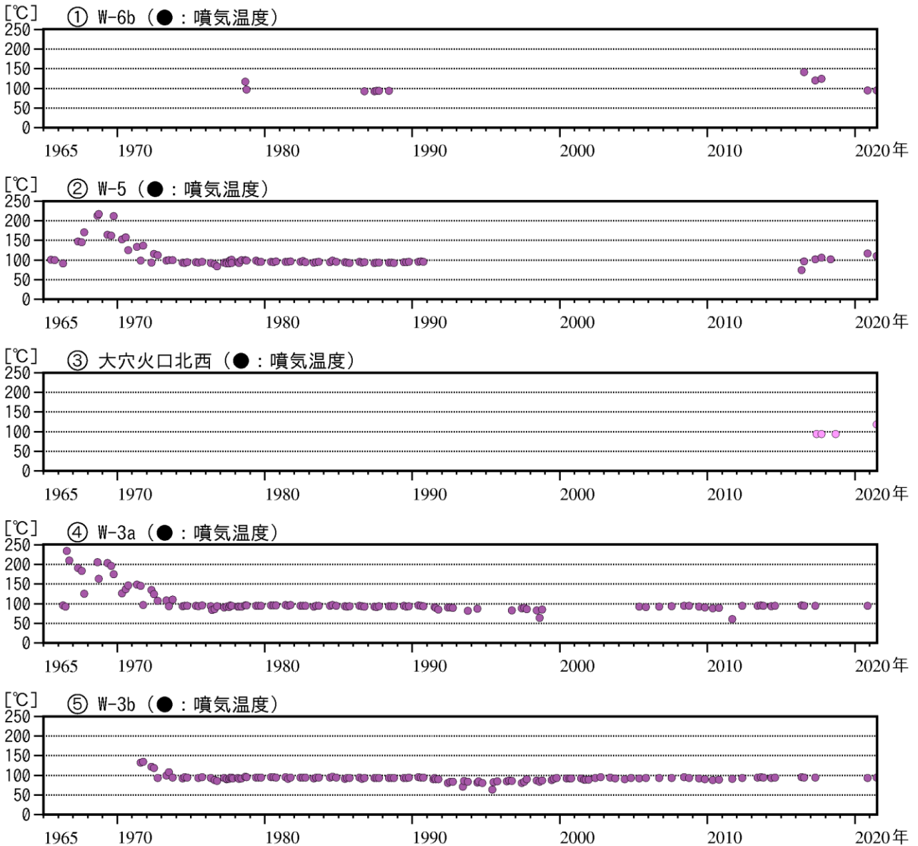
図14 吾妻山 大穴火口周辺の噴気温度の経過(1965年7月～2021年6月)
