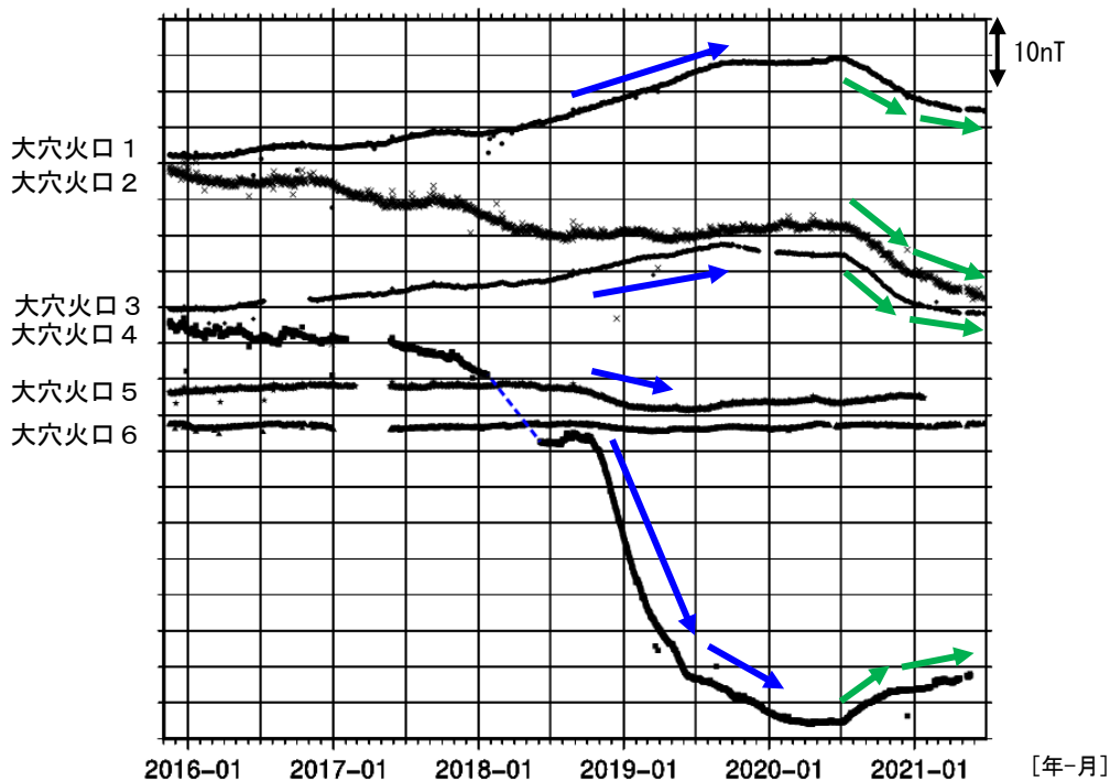
図 17 吾妻山 全磁力連続観測点の全磁力値変化 (2015年11月~2021年6月)
