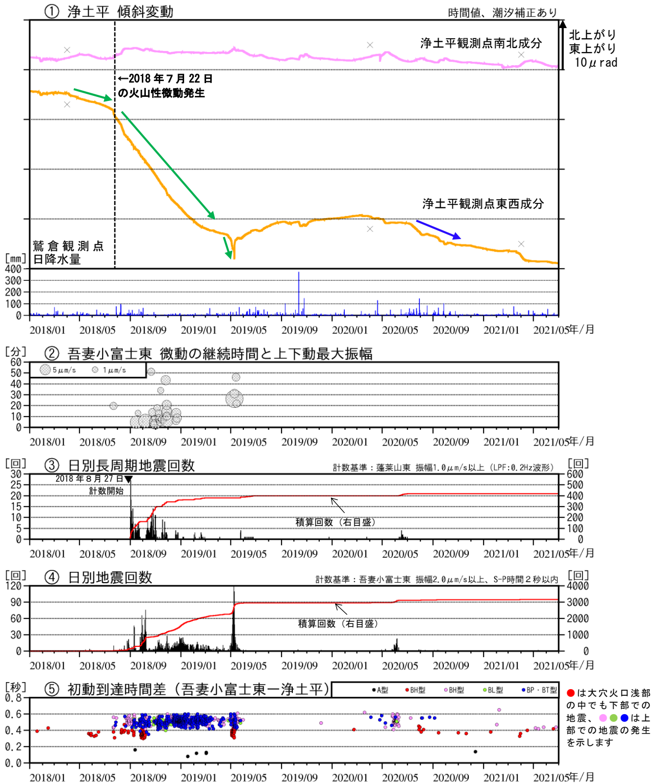
図3 吾妻山 火山活動経過図 (2018年1月～2021年6月)
