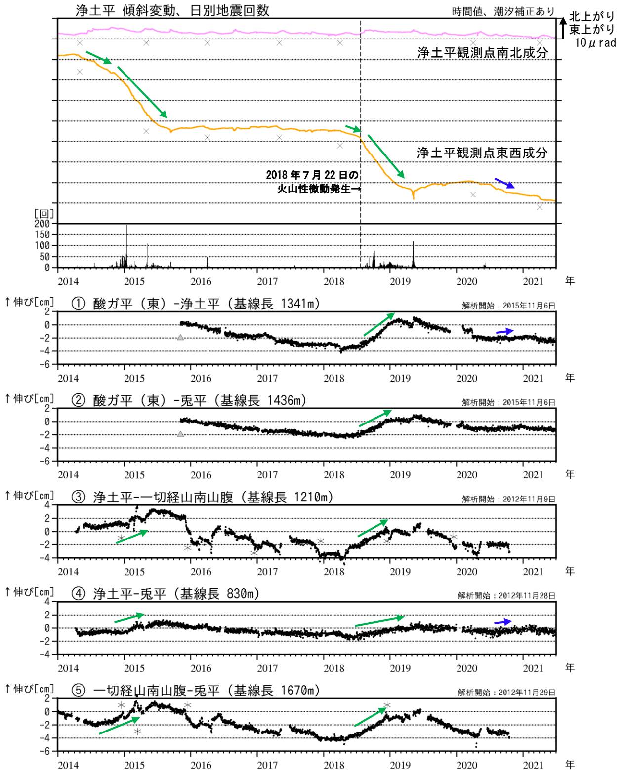
図5 吾妻山 大穴火口浅部の地殻変動（2014年1月～2021年6月）
