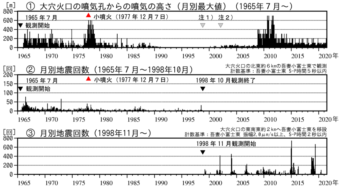
図1 吾妻山 長期的な火山活動の経過（1965年7月～2021年6月）
