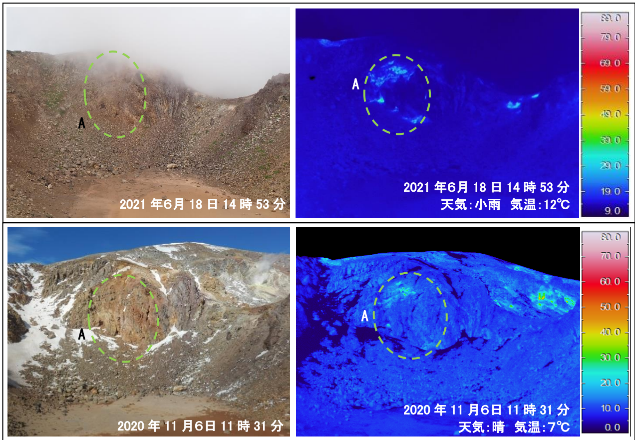
図 10 吾妻山 燕沢火口列北側火口壁の状況（左）と地表面温度分布（右）
