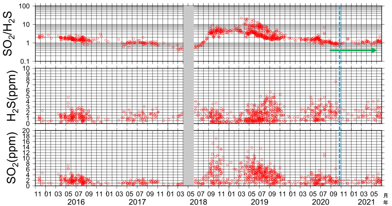
図15 吾妻山 火山ガス観測装置による観測（2015年11月～2021年6月）
