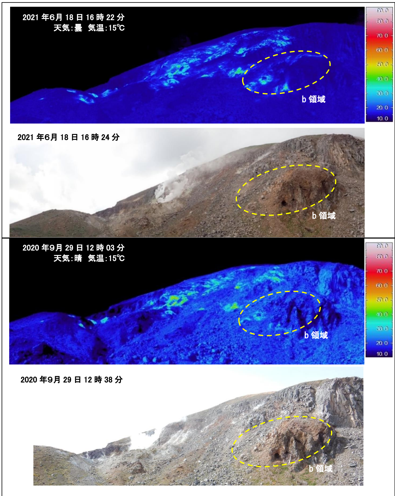
図 12 吾妻山 大穴火口北側の状況(下)と地表面温度分布(上)
