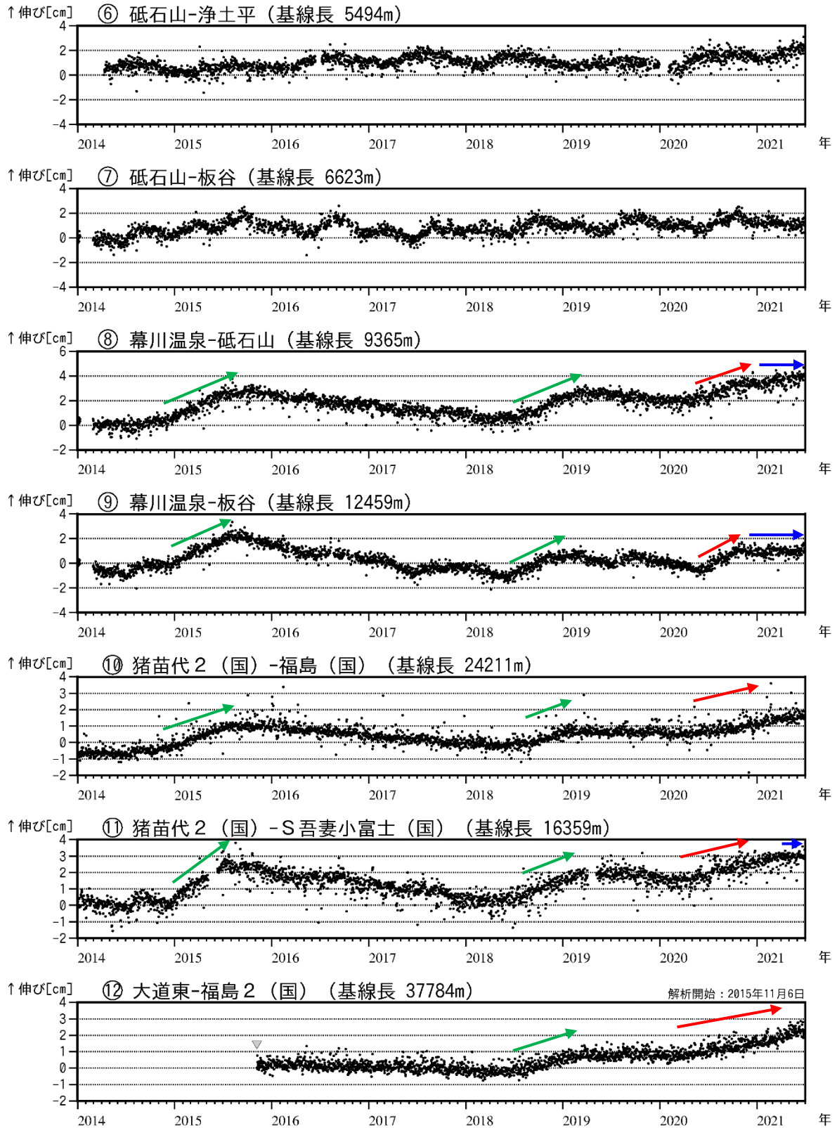
図6 吾妻山 吾妻山深部の地殻変動（2014年1月～2021年6月）
