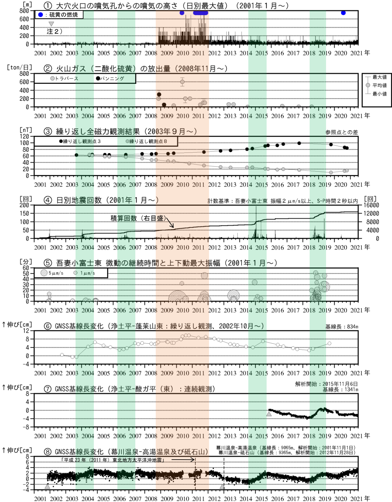
図2 吾妻山 中期的な火山活動の経過（2001年1月～2021年6月）
