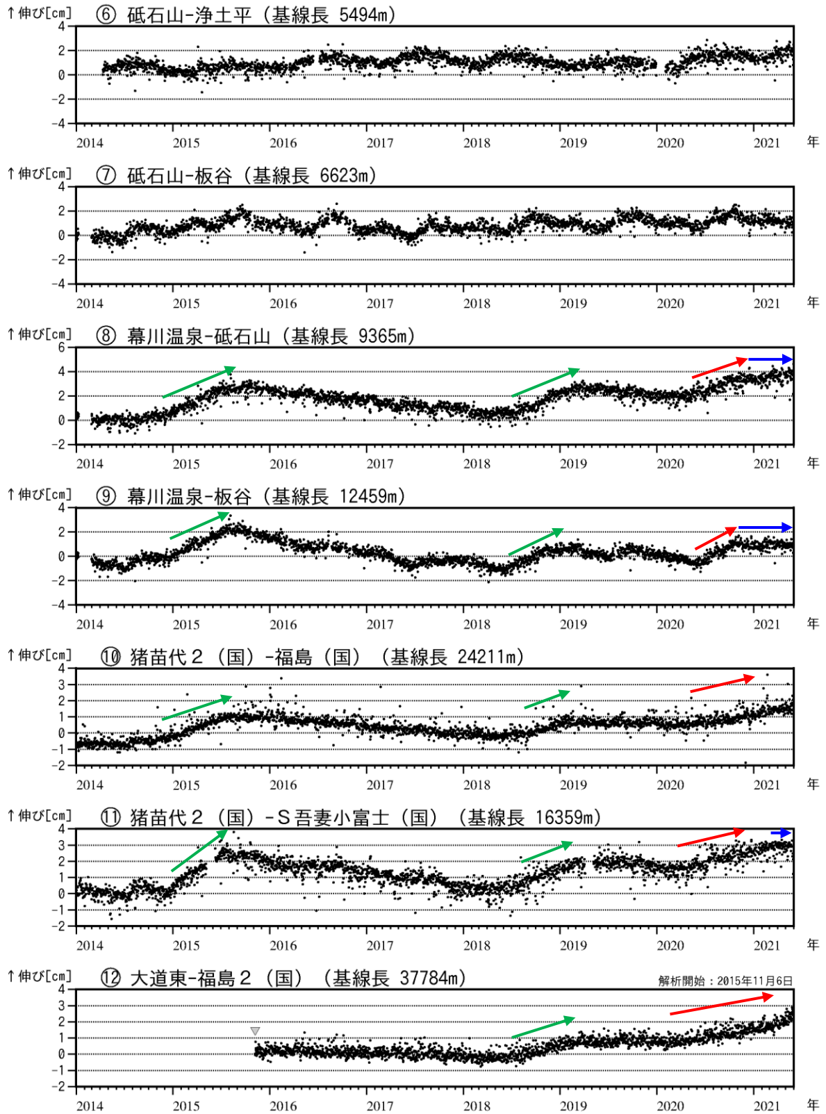
図6 吾妻山 吾妻山深部の地殻変動（2014年1月～2021年5月）
