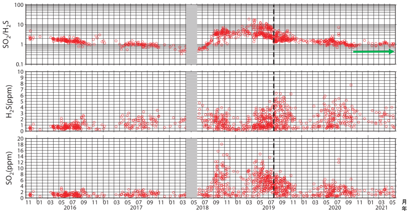
図9 吾妻山 火山ガス観測装置による観測（2015年11月～2021年5月）
