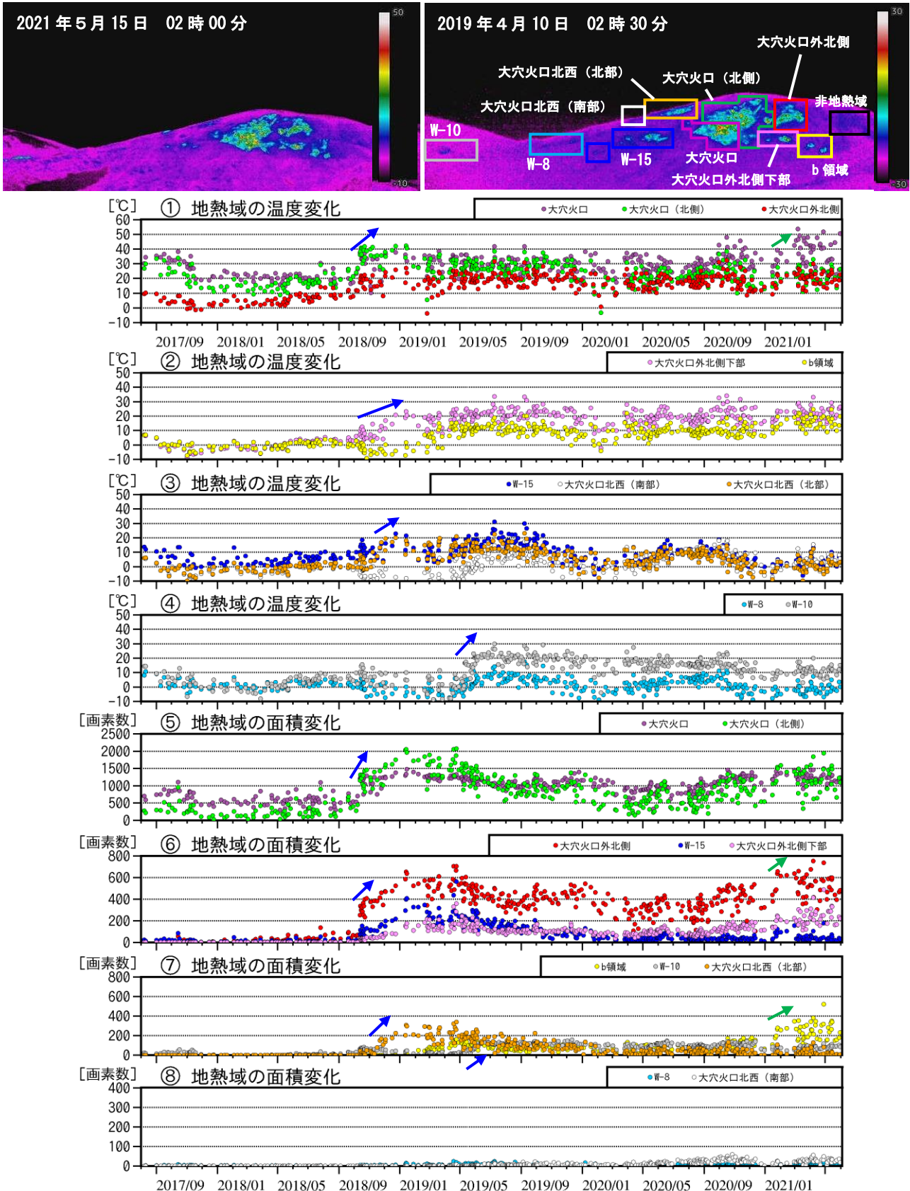
図7 吾妻山 監視カメラによる大穴火口周辺の地熱域の経過（2017年8月～2021年5月）
