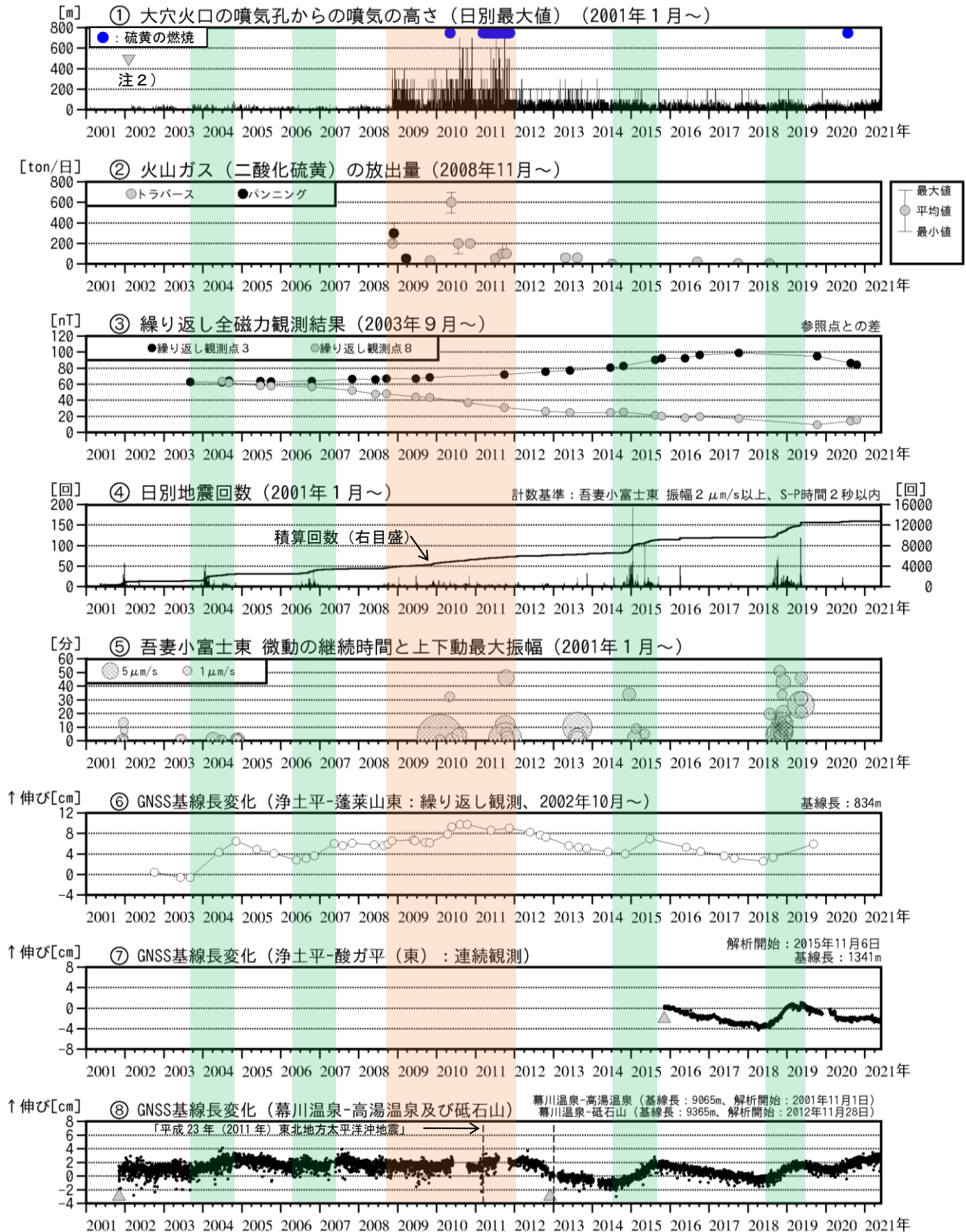
図2 吾妻山 中期的な火山活動の経過（2001年1月～2021年5月）
