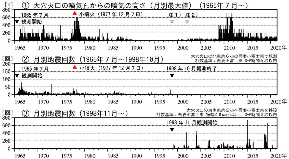
図1 吾妻山 長期的な火山活動の経過（1965年7月～2021年5月）
