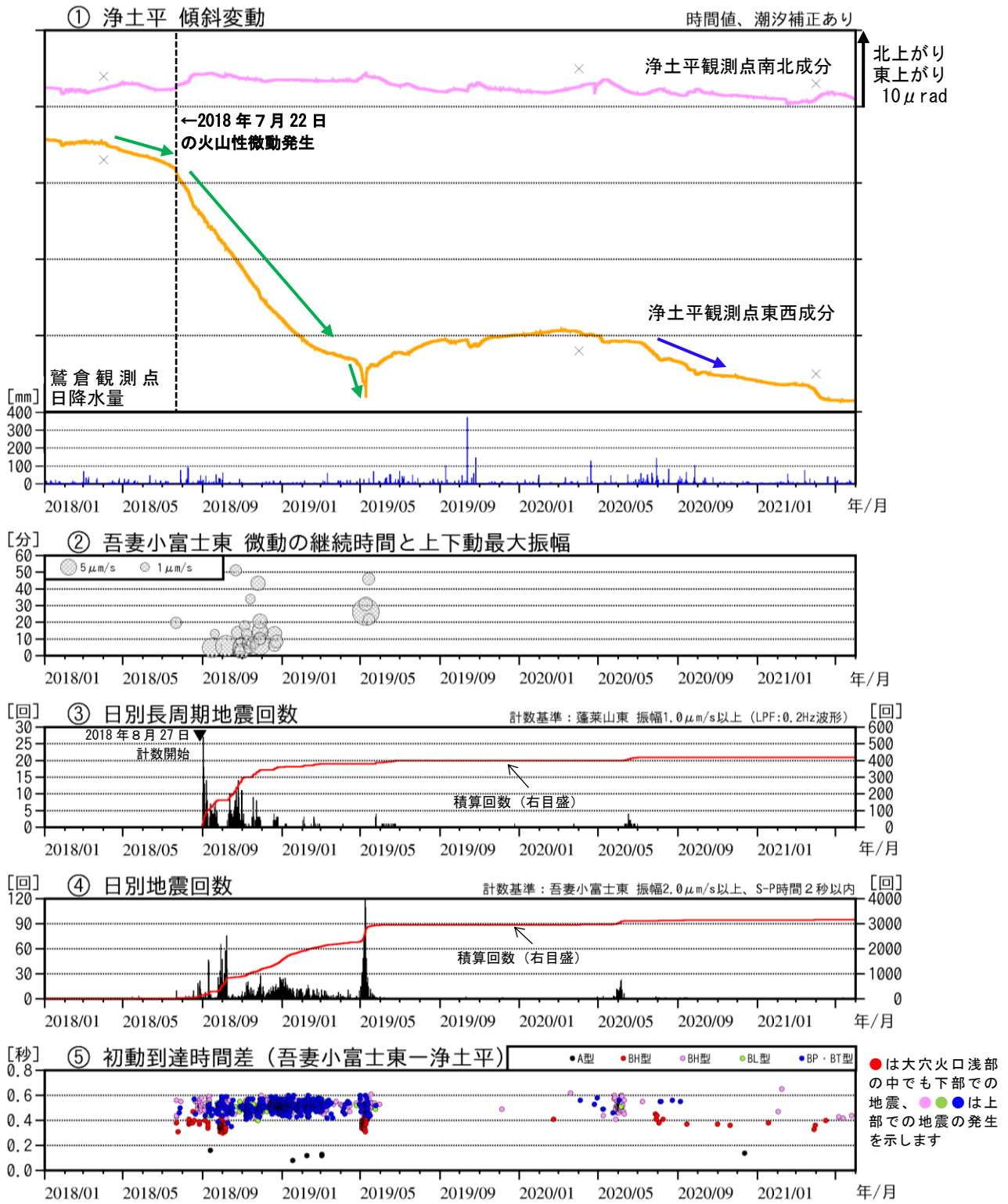
図3 吾妻山 火山活動経過図 (2018年1月~2021年5月)
