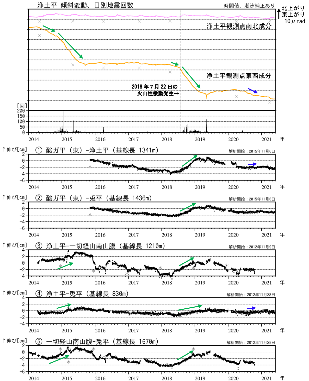
図5 吾妻山 大穴火口浅部の地殻変動（2014年1月～2021年5月）
