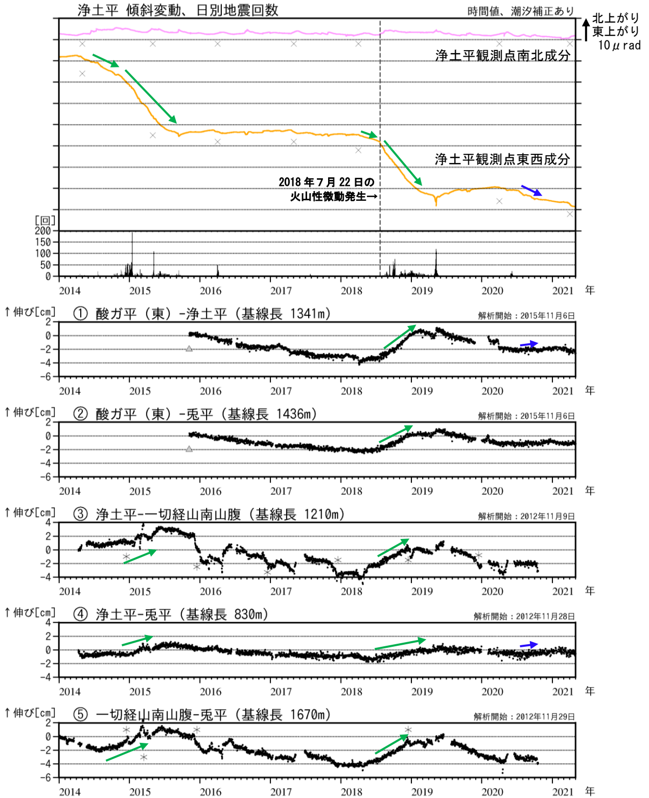
図5 吾妻山 大穴火口浅部の地殻変動（2014年1月～2021年4月）
