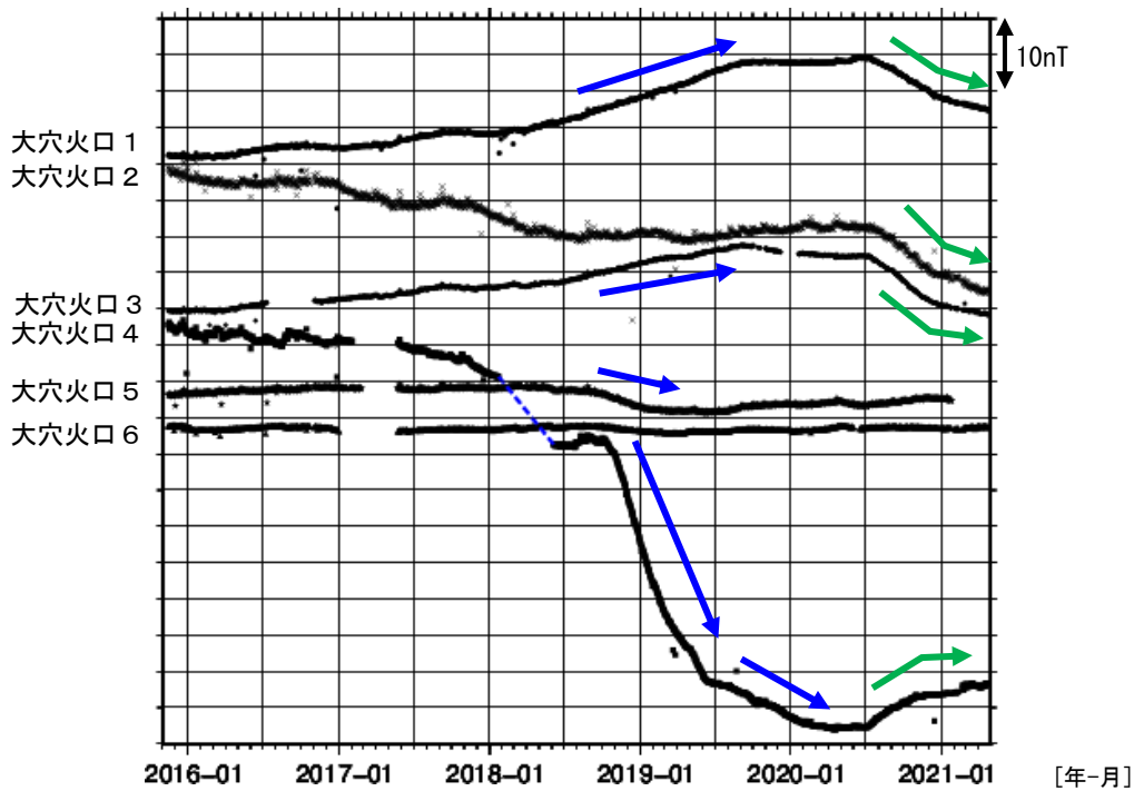
図 11 吾妻山 全磁力連続観測点の全磁力値変化 (2015年11月~2021年4月)
