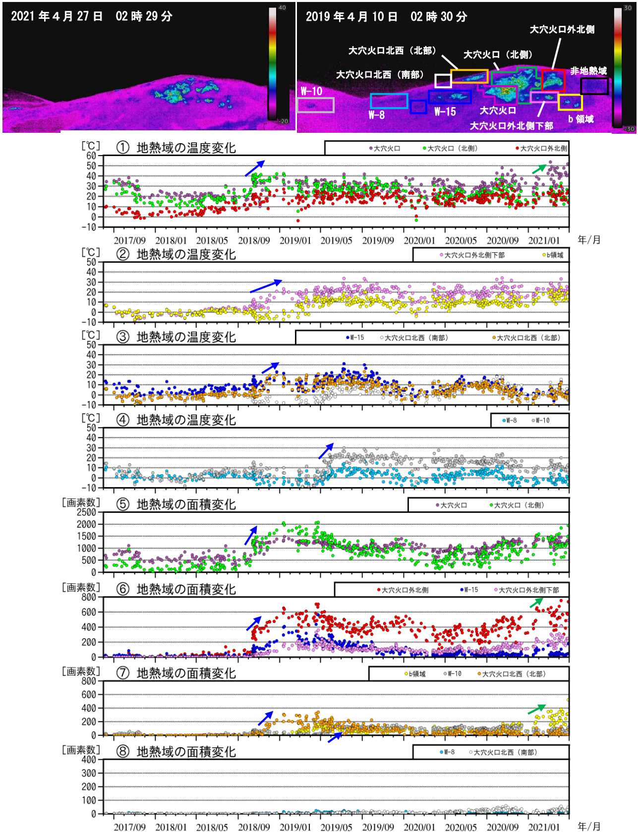
図7 吾妻山 監視カメラによる大穴火口周辺の地熱域の経過（2017年8月～2021年4月）
