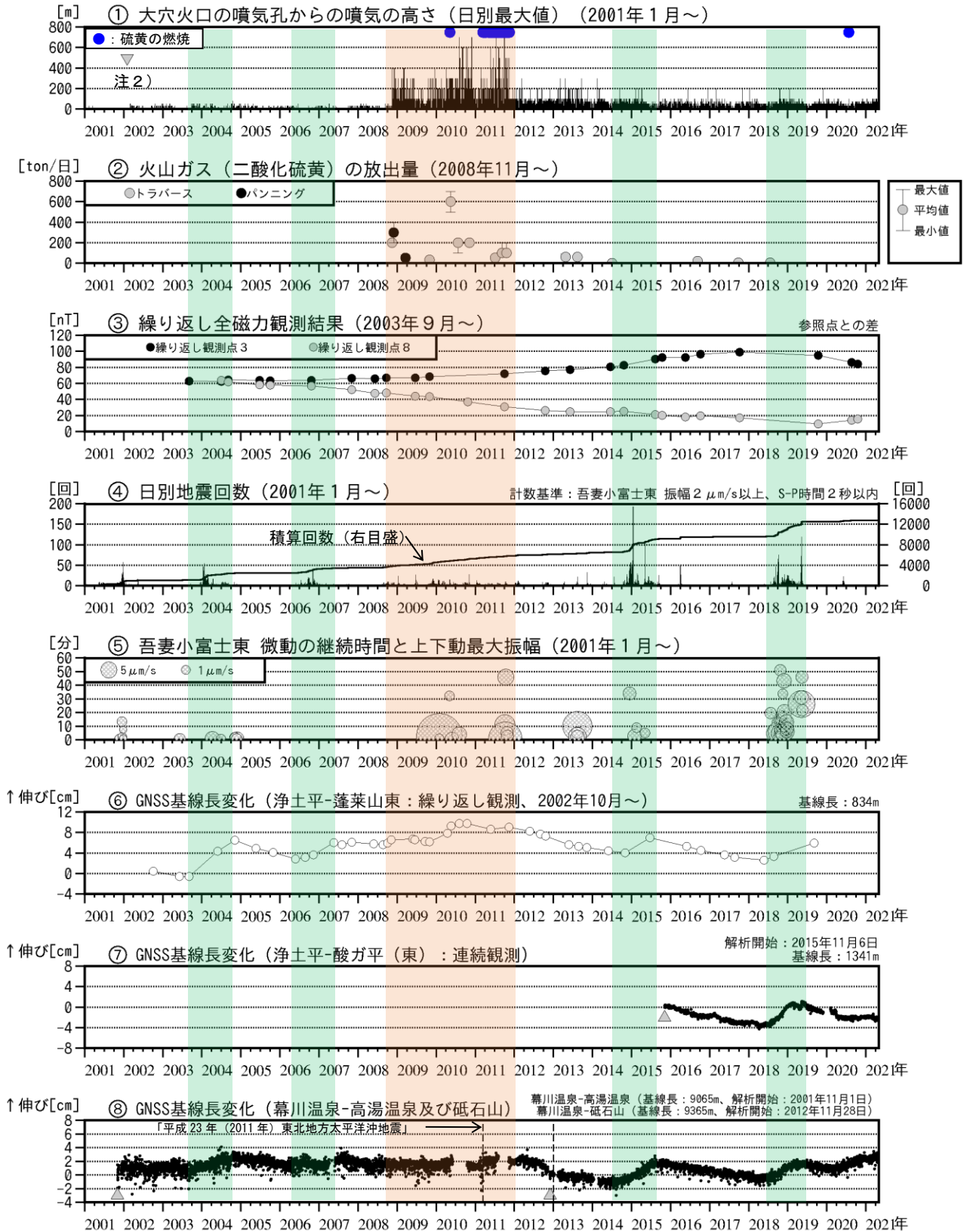
図2 吾妻山 中期的な火山活動の経過（2001年1月～2021年4月）
