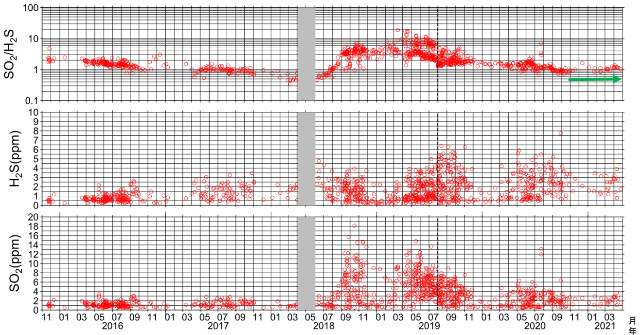
図9 吾妻山 火山ガス観測装置による観測（2015年11月～2021年4月）
