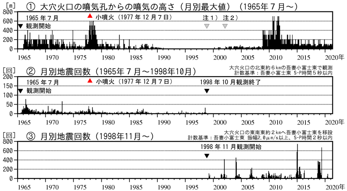
図1 吾妻山 長期的な火山活動の経過（1965年7月～2021年4月）
