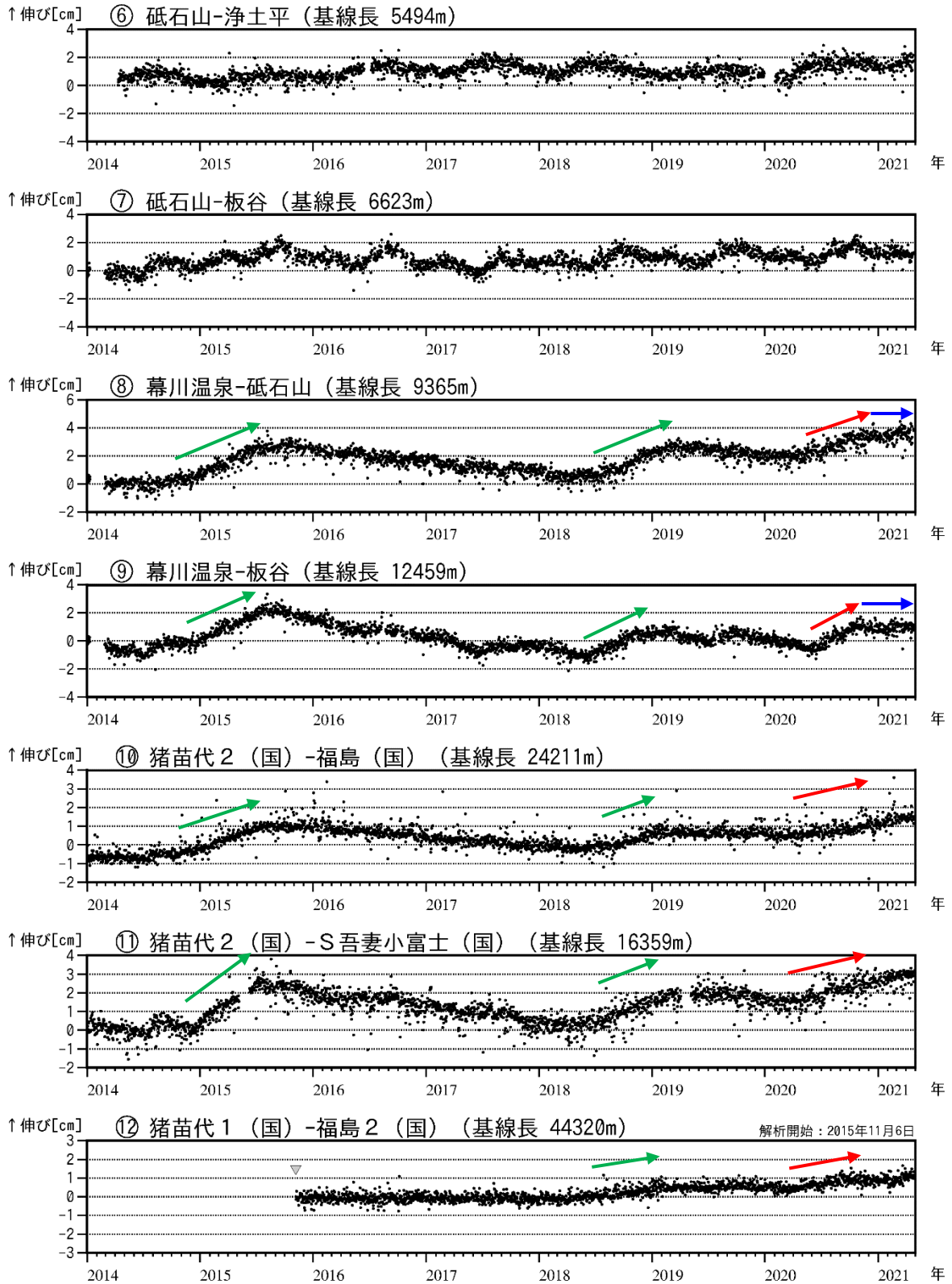
図6 吾妻山 吾妻山深部の地殻変動（2014年1月～2021年4月）
