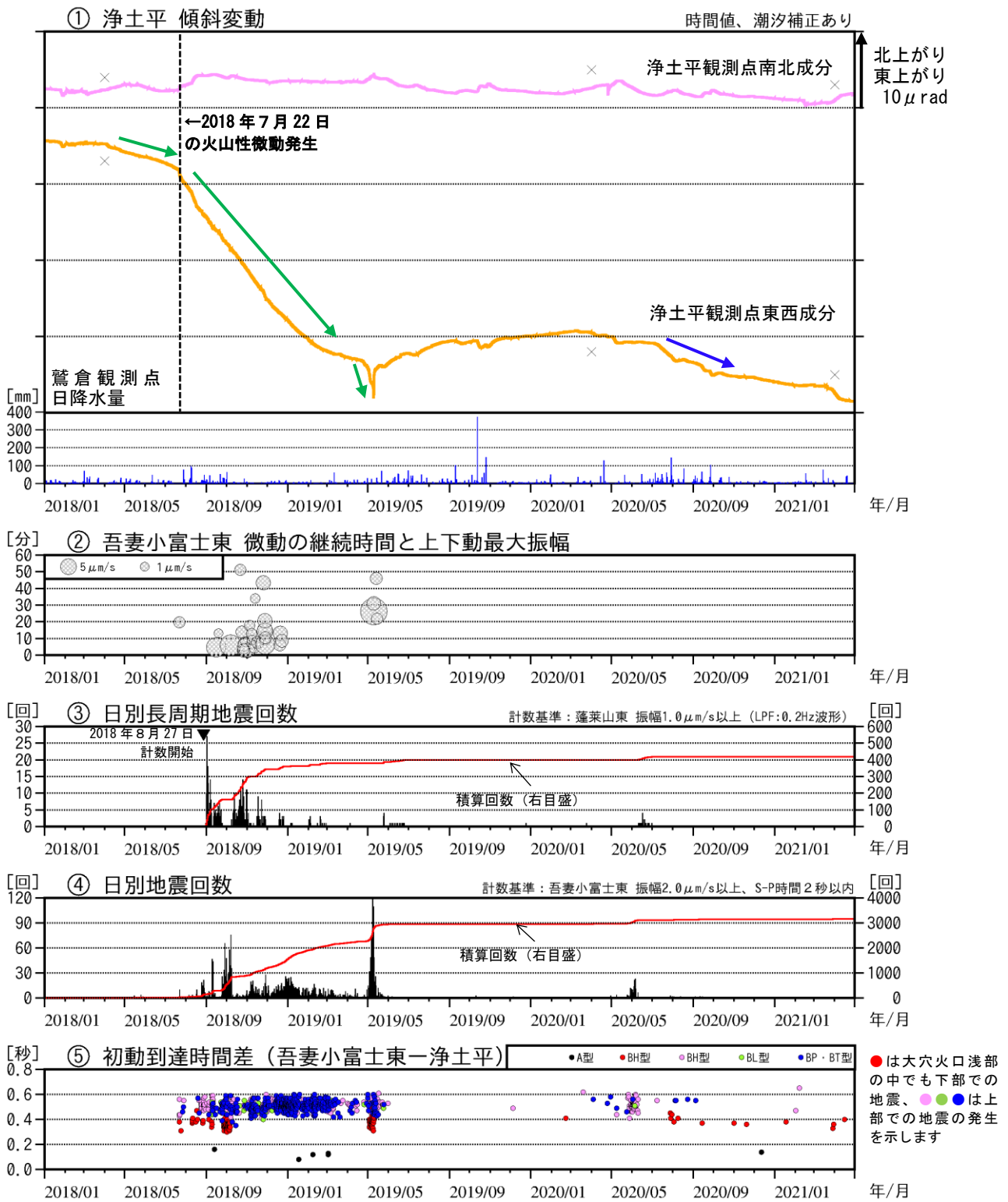
図3 吾妻山 火山活動経過図（2018年1月～2021年4月）
