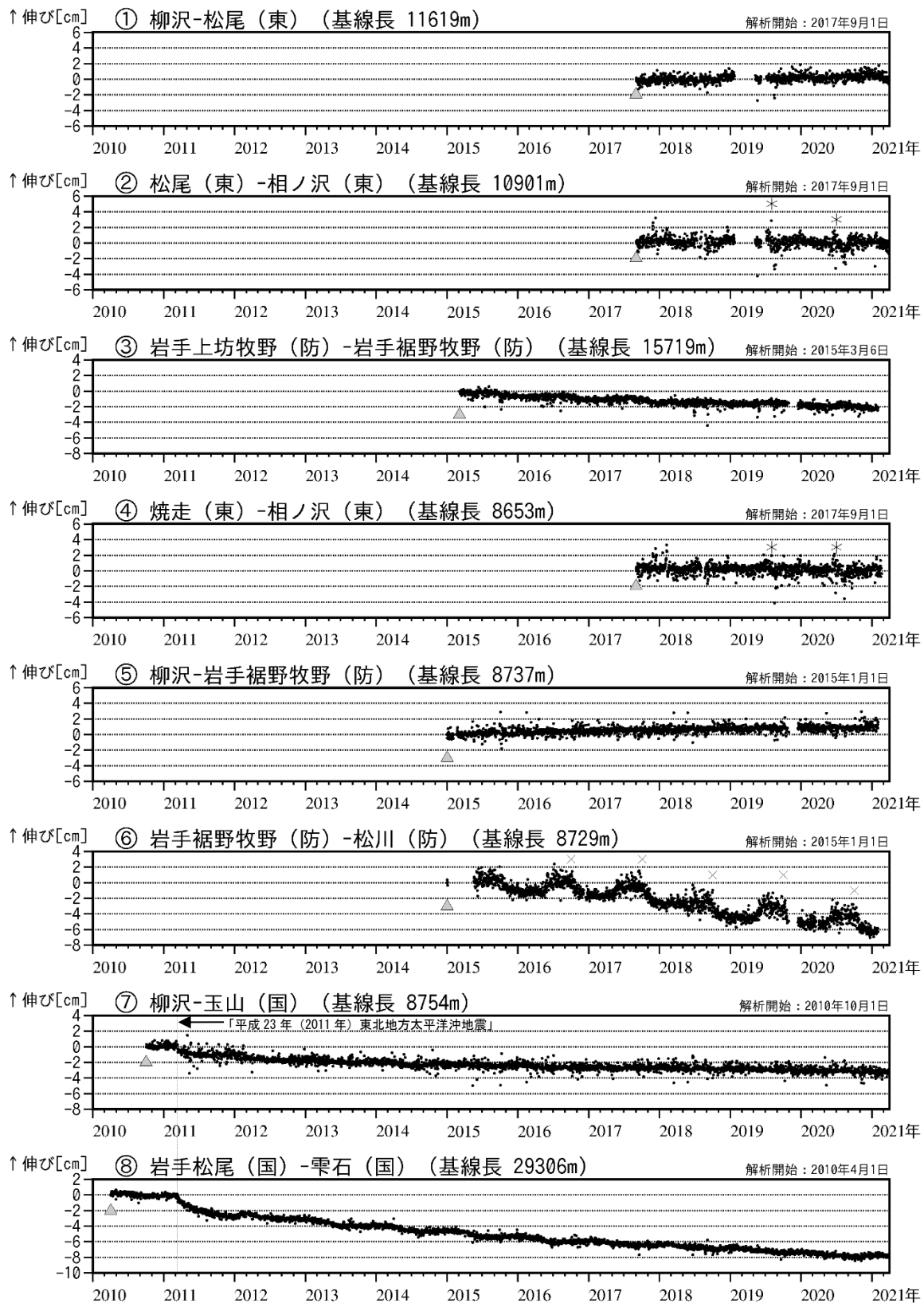
図8 岩手山 GNSS 基線長変化図 (2010年4月~2021年3月)
