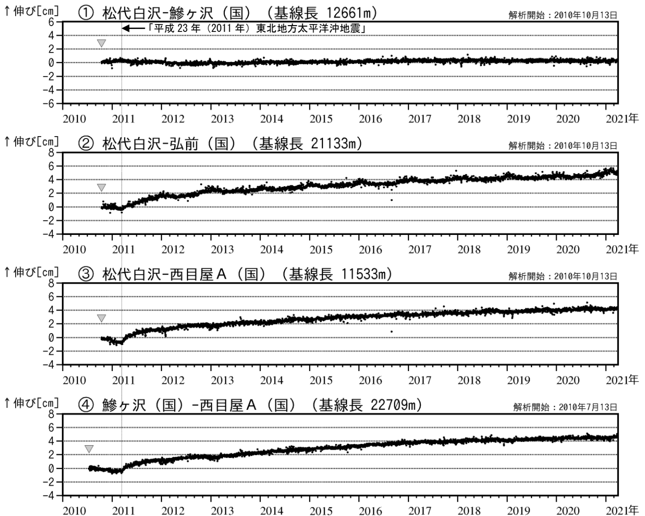
図3 岩木山 GNSS 基線長変化図（2010年7月～2021年3月）
