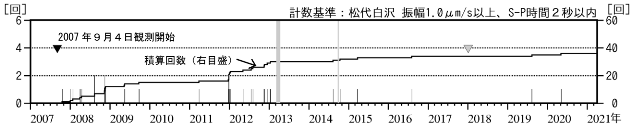
図2 岩木山 日別地震回数（2007年9月～2021年3月）
