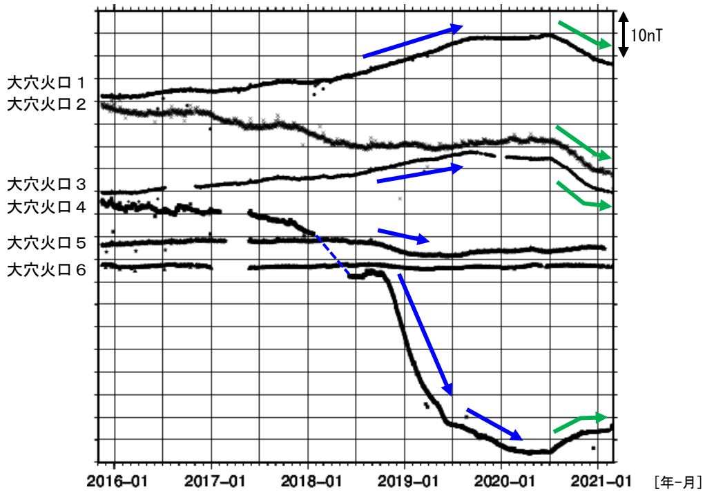
図11 吾妻山 全磁力連続観測点の全磁力値変化（2015年11月～2021年2月）
