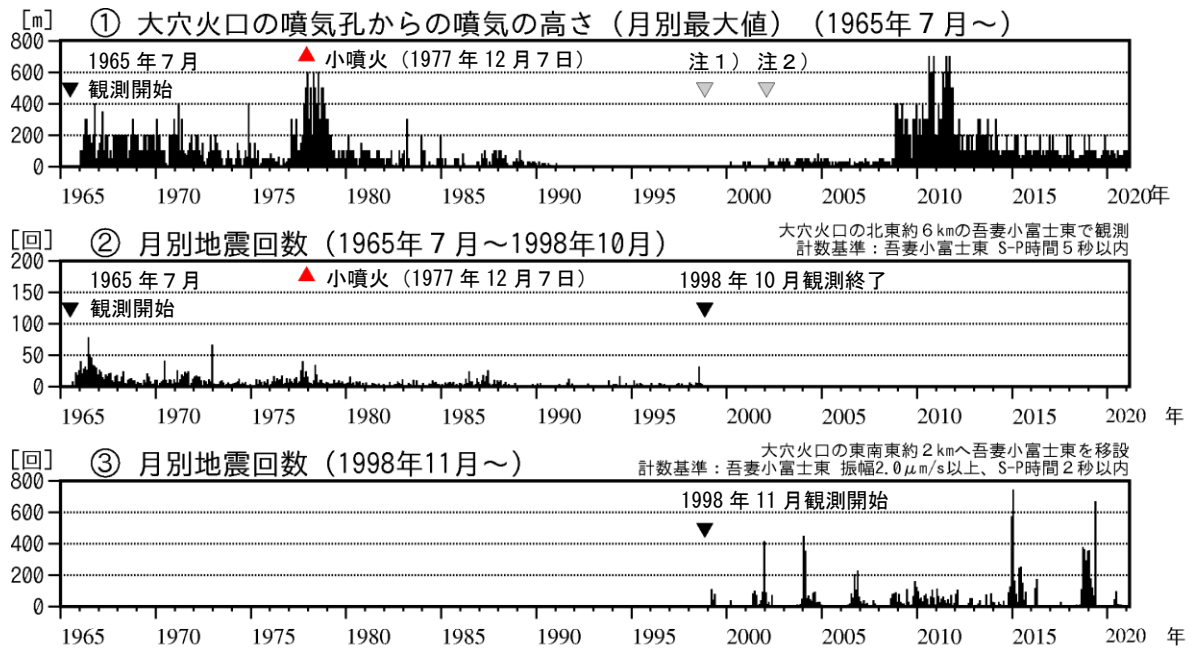
図1 吾妻山 長期的な火山活動の経過（1965年7月～2021年2月）
