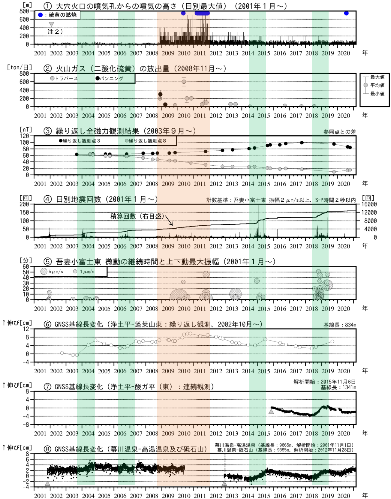
図2 吾妻山 中期的な火山活動の経過（2001年1月～2021年2月）
