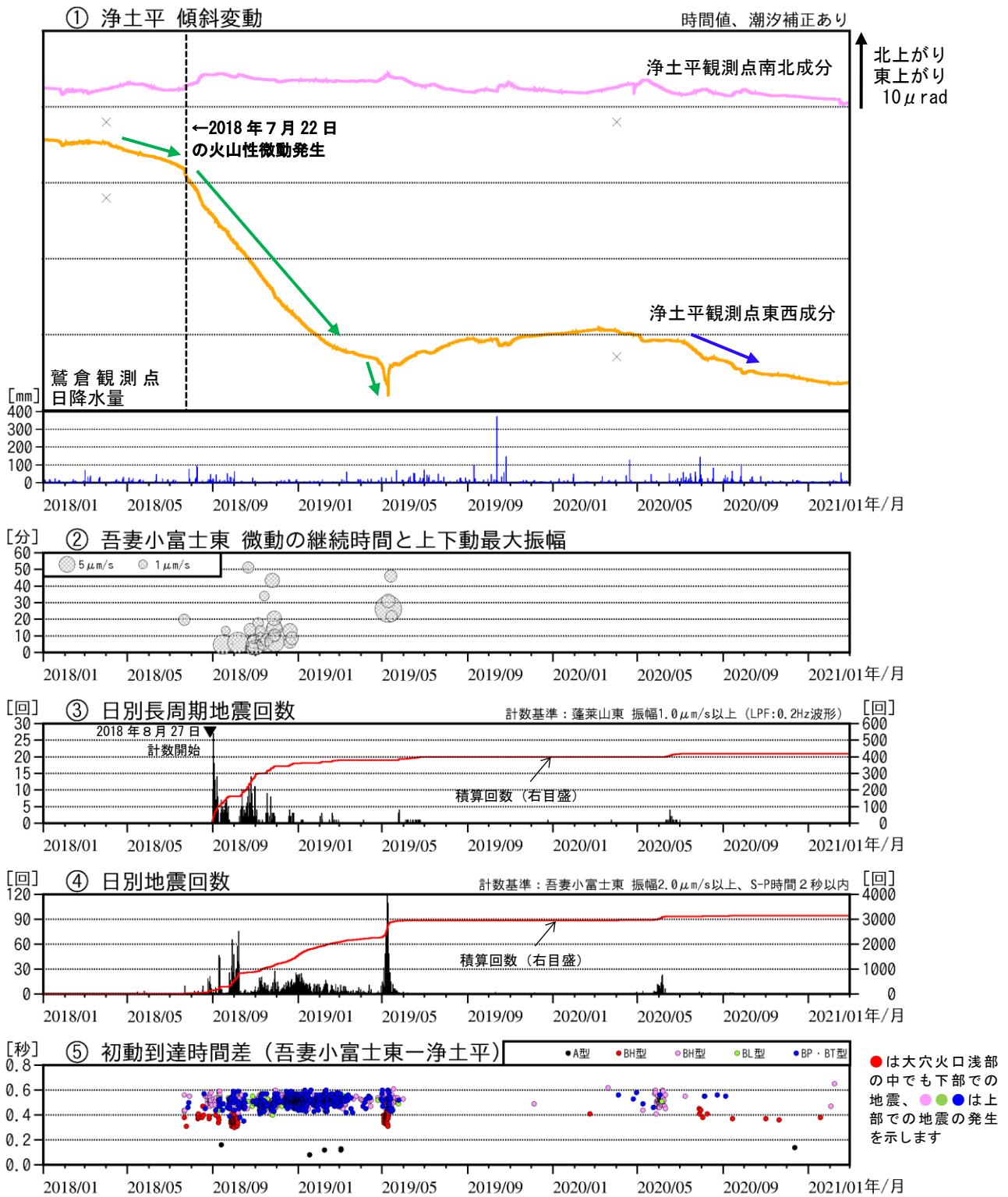
図3 吾妻山 火山活動経過図 (2018年1月～2021年2月)
