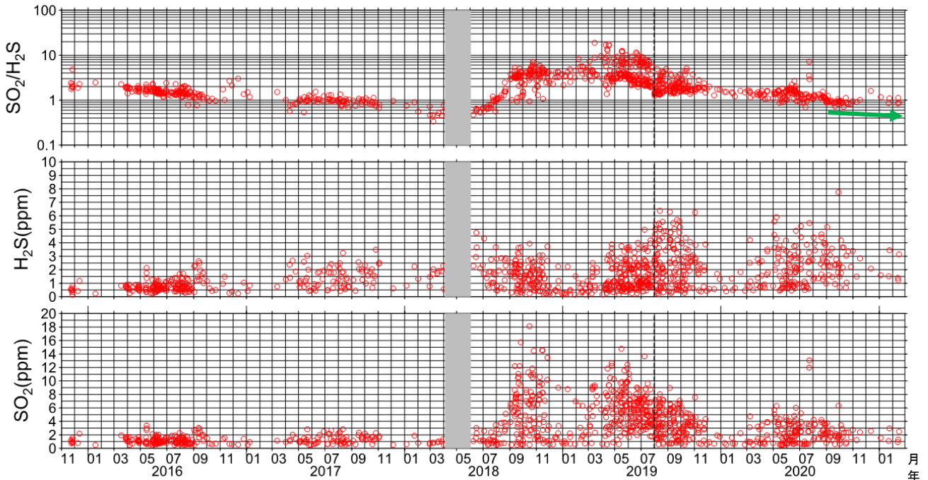
図9 吾妻山 火山ガス観測装置による観測（2015年11月～2021年2月）
