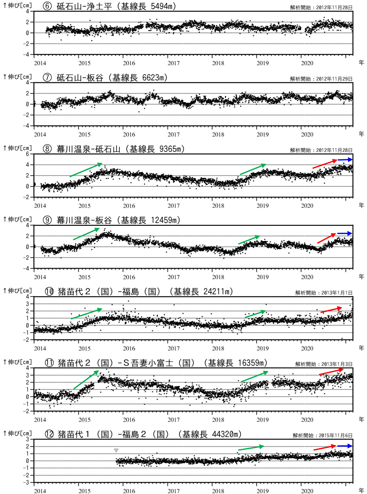
図6 吾妻山 吾妻山深部の地殻変動（2014年1月～2021年2月）
