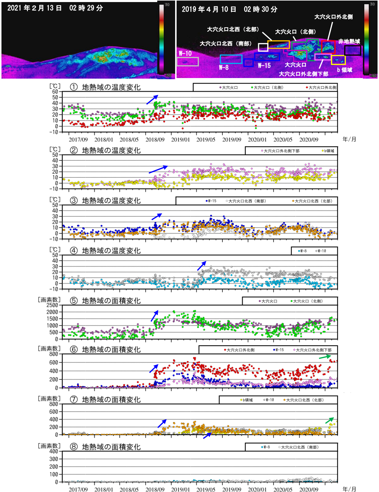
図7 吾妻山 監視カメラによる大穴火口周辺の地熱域の経過（2017年8月～2021年2月）
