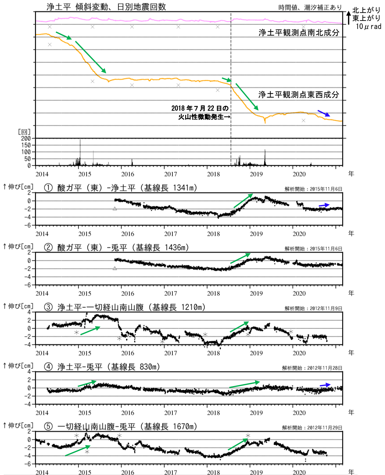
図5 吾妻山 大穴火口浅部の地殻変動（2014年1月～2021年2月）
