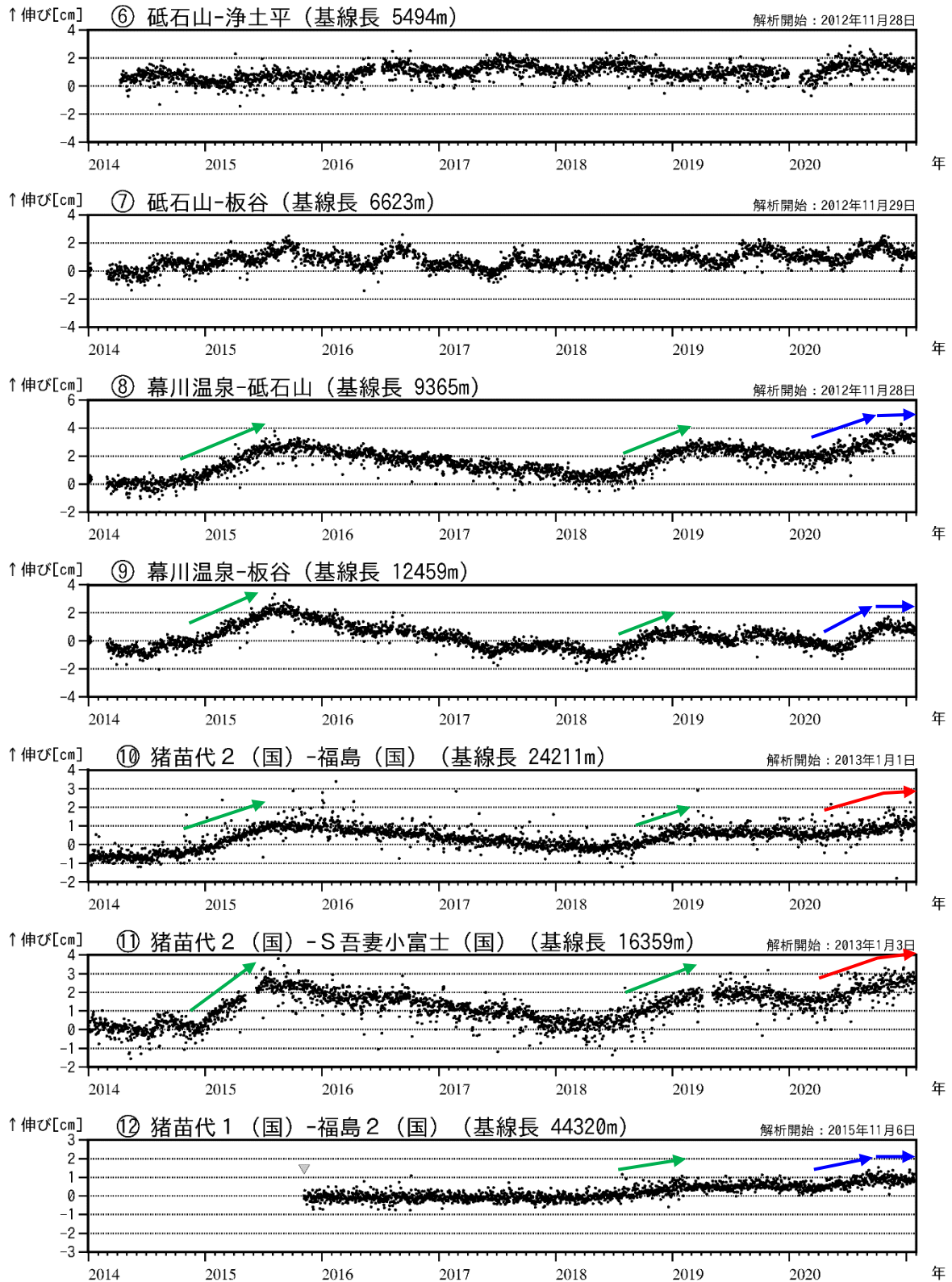
図6 吾妻山 吾妻山深部の地殻変動（2014年1月～2021年1月）
