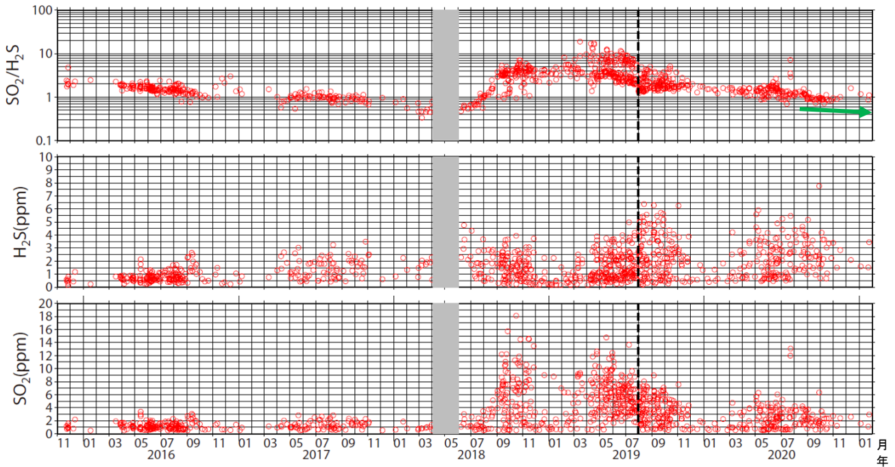
図9 吾妻山 火山ガス観測装置による観測（2015年11月～2021年1月）
