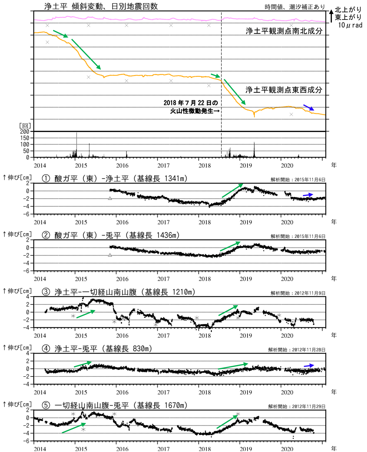
図5 吾妻山 大穴火口浅部の地殻変動（2014年1月～2021年1月）
