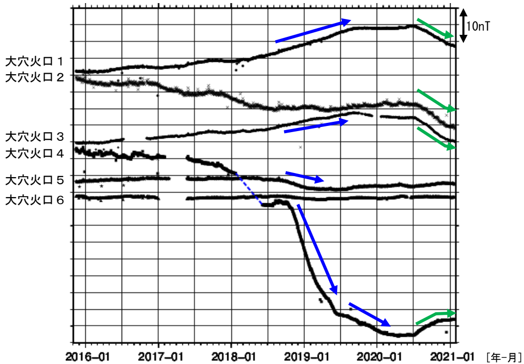
図 11 吾妻山 全磁力連続観測点の全磁力値変化 (2015年11月~2021年1月)
