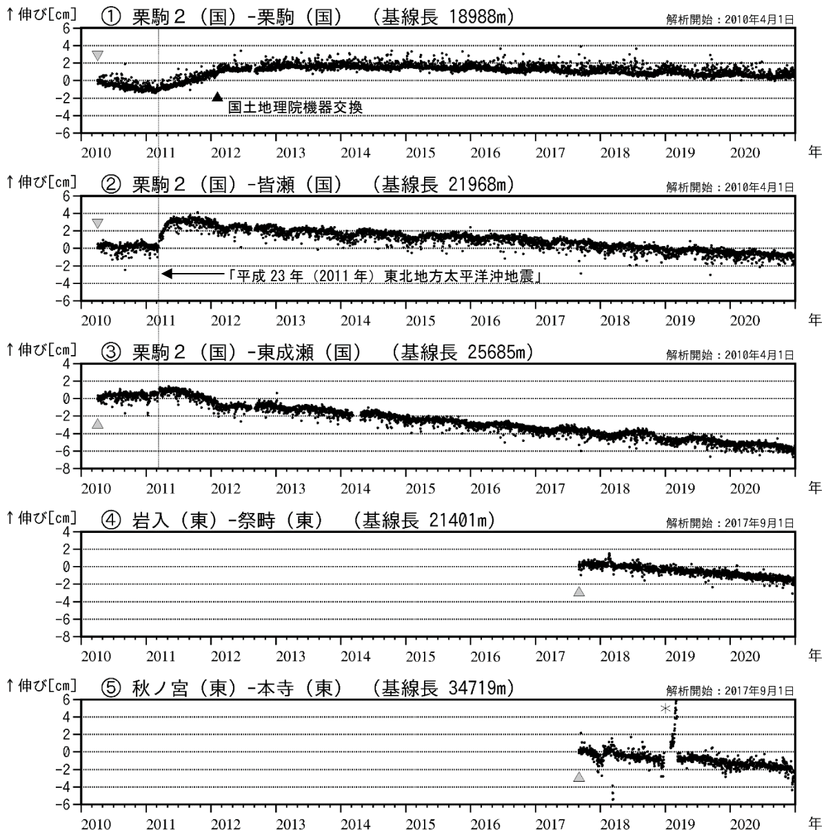
図3 栗駒山 GNSS 基線長変化図 (2010年4月～2020年12月)
