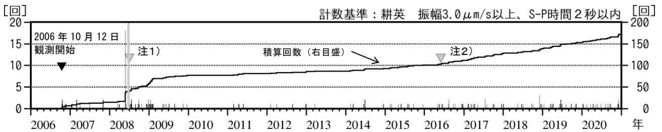
図2 栗駒山 日別地震回数（2006年10月～2020年12月）
