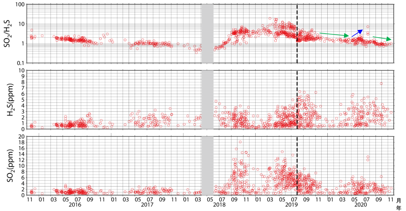
図14 吾妻山 火山ガス観測装置による観測（2015年11月～2020年11月）
