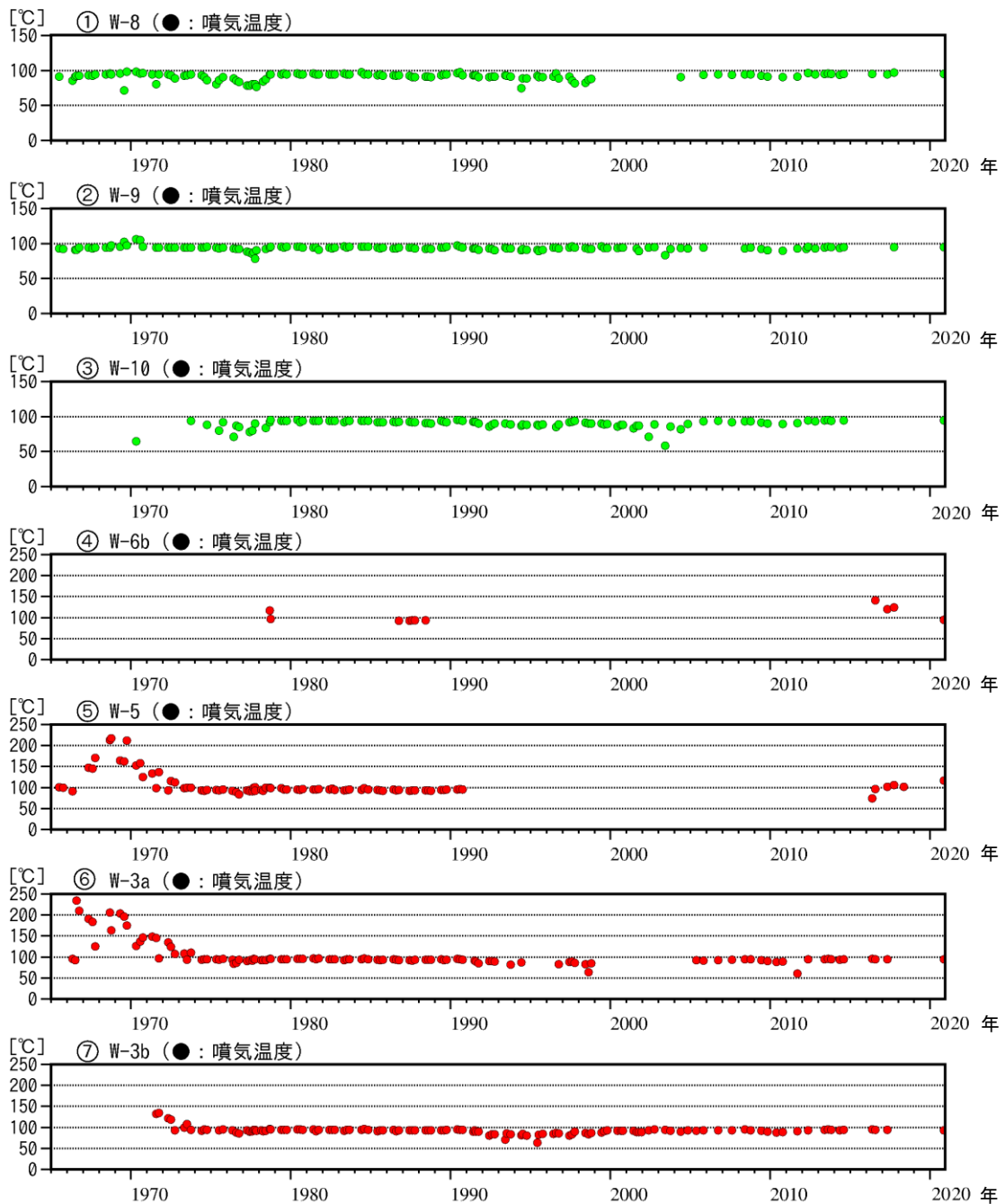
図13 吾妻山 大穴火口付近及び八幡焼付近の噴気温度の経過（1965年7月～2020年11月）
