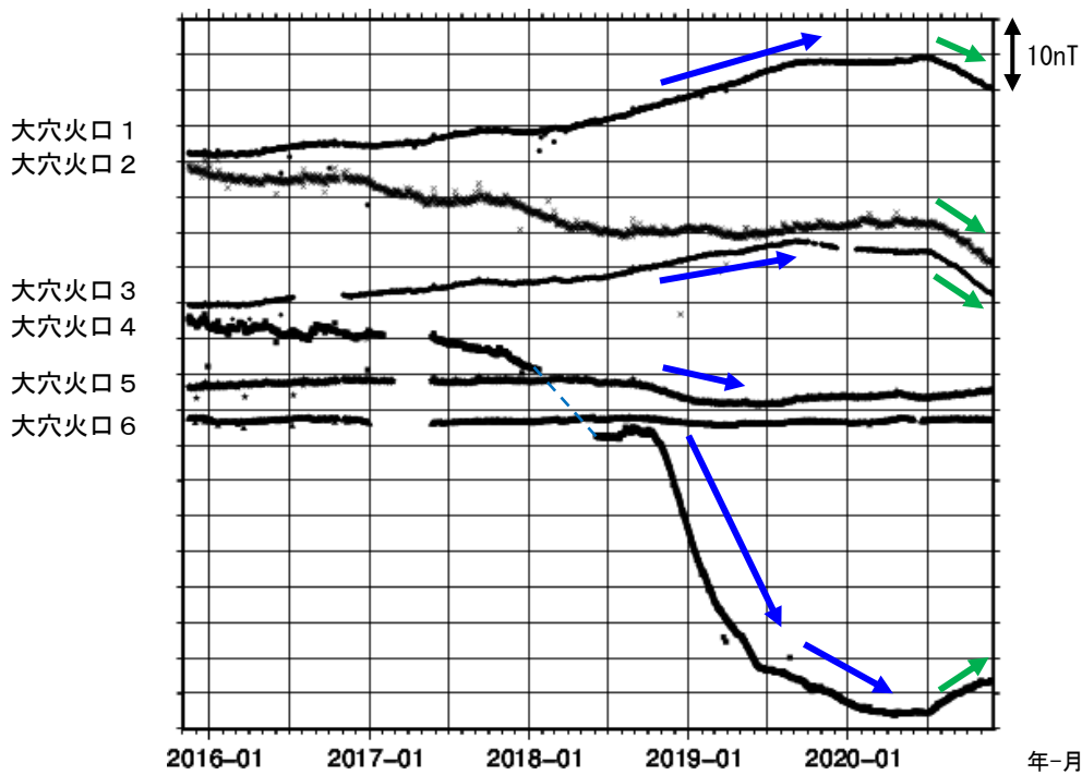
図 16 吾妻山 全磁力連続観測点の全磁力値変化 (2015年11月~2020年11月)
