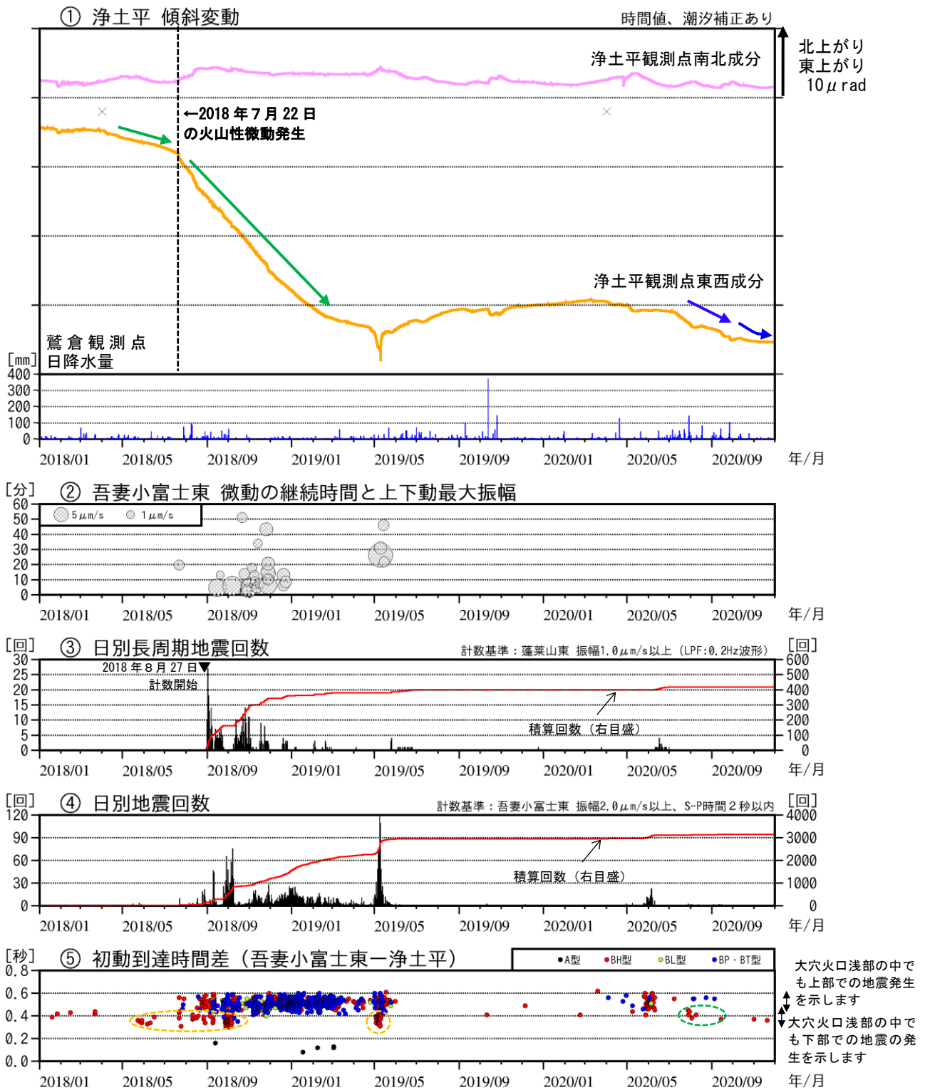
図3 吾妻山 火山活動経過図（2018年1月～2020年11月）
