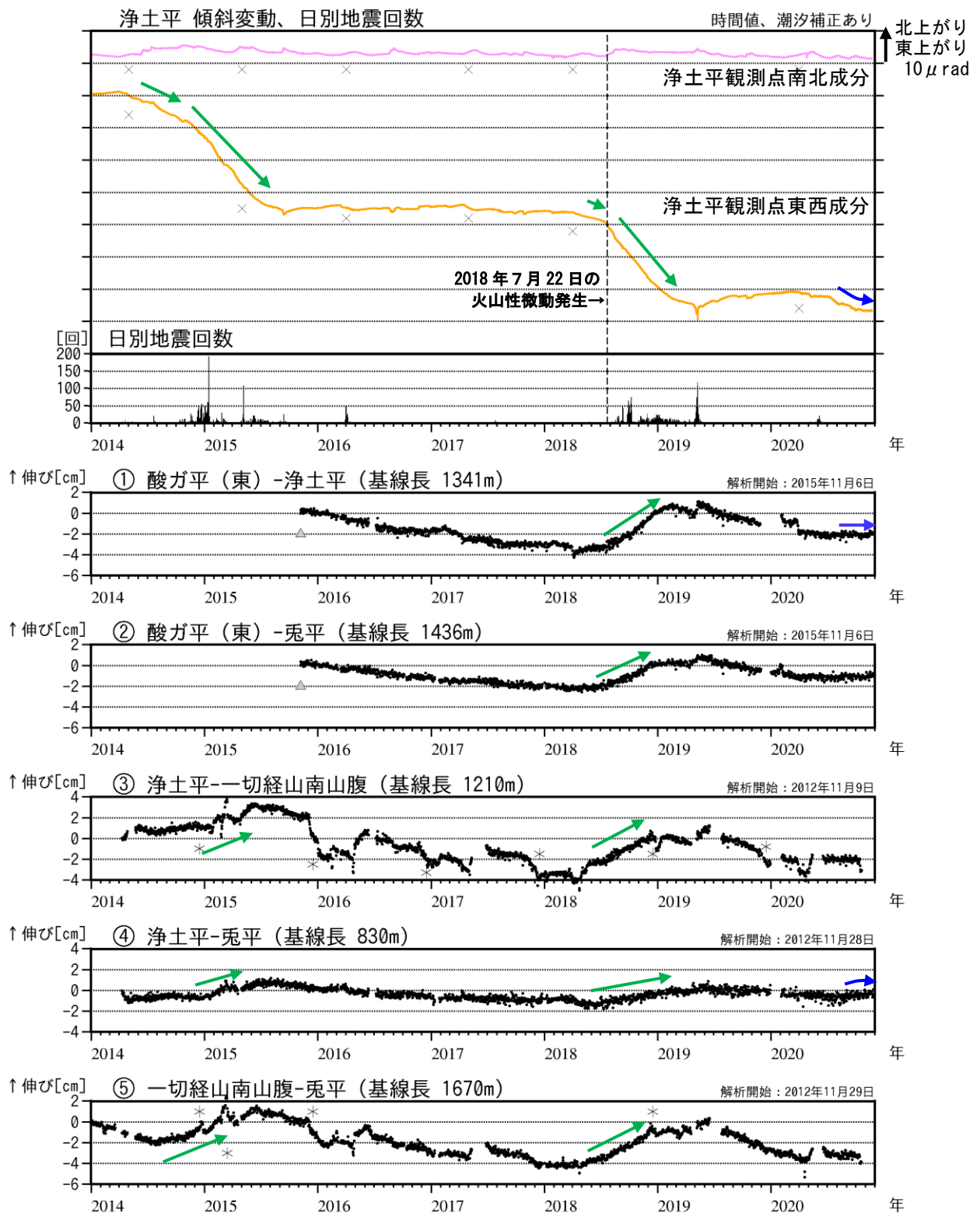
図5 吾妻山 大穴火口浅部の地殻変動（2014年1月～2020年11月）
