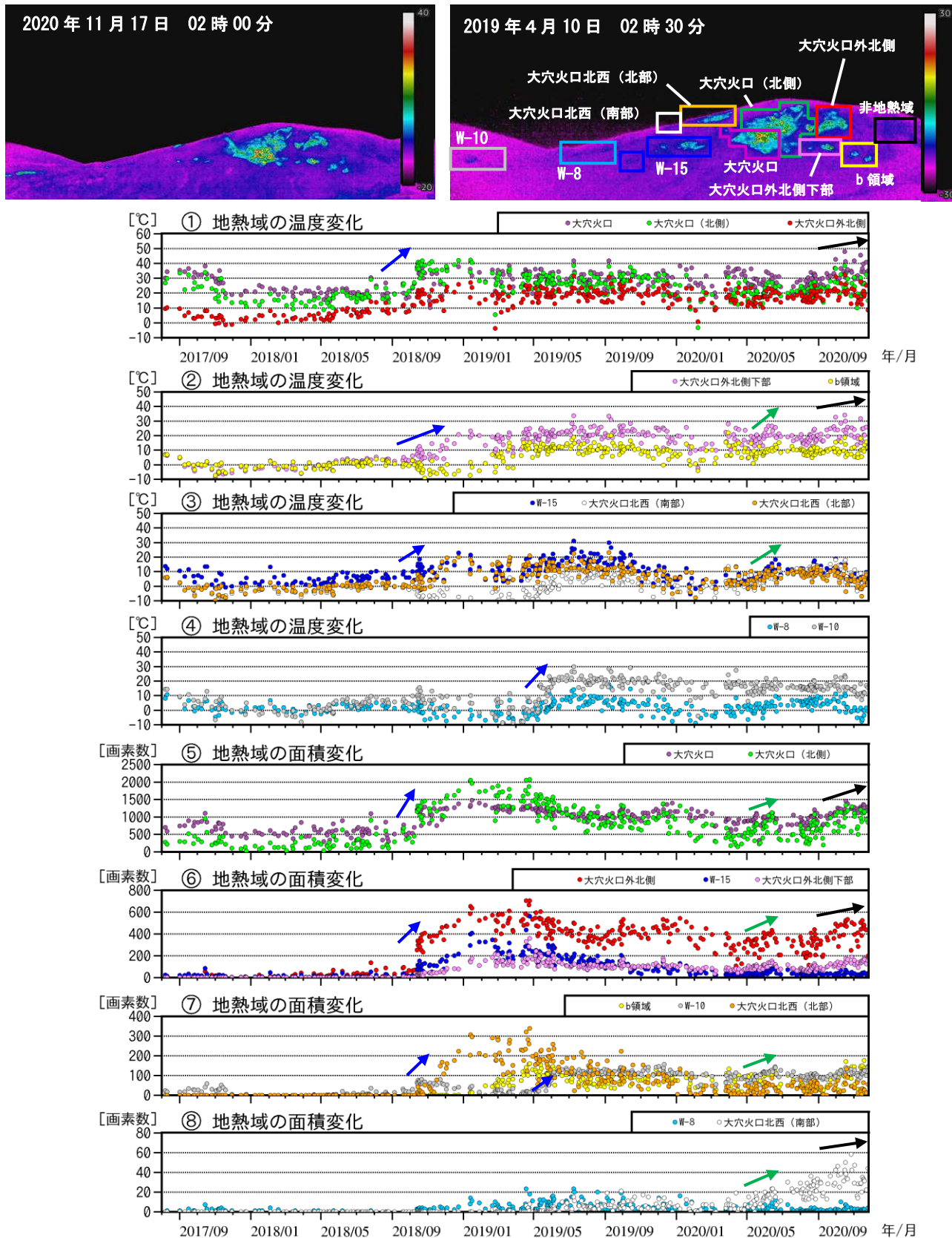
図7 吾妻山 監視カメラによる大穴火口周辺の地熱域の経過 (2017年8月~2020年11月)
