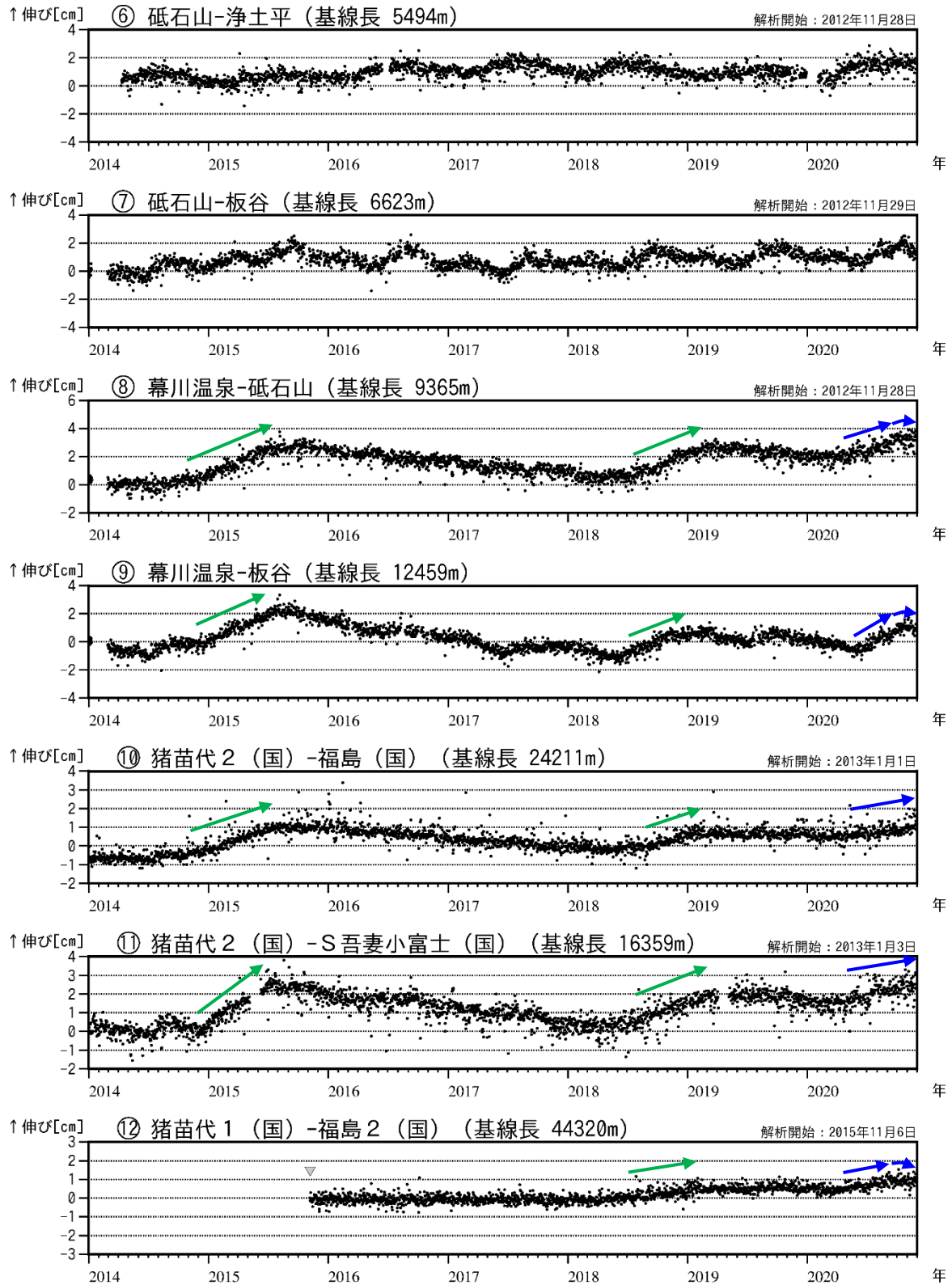
図6 吾妻山 吾妻山深部の地殻変動（2014年1月～2020年11月）
