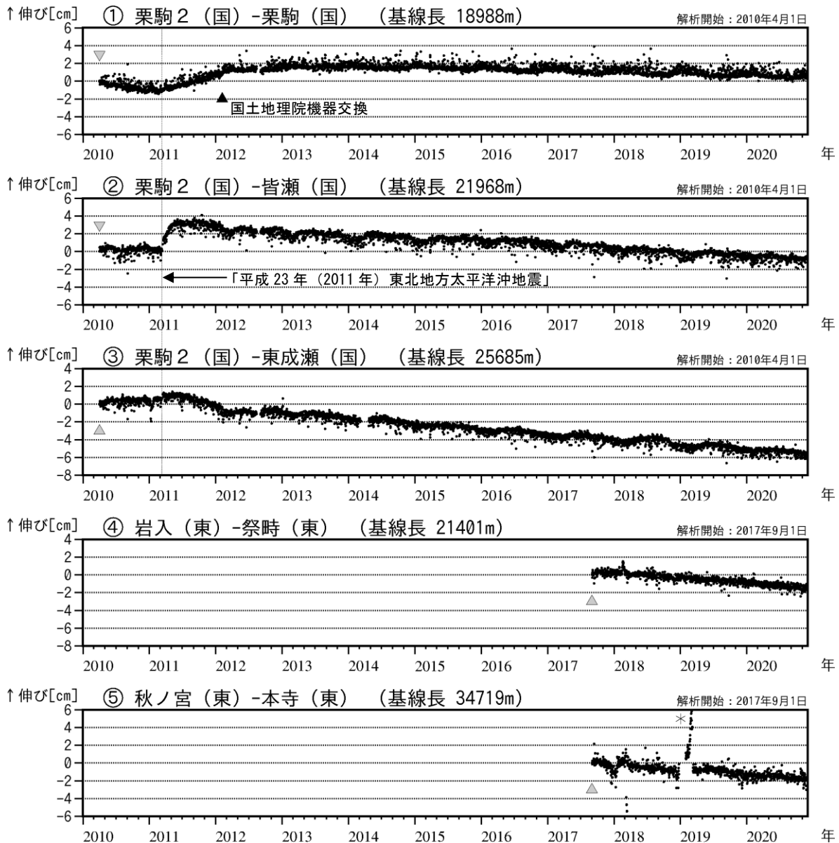
図4 栗駒山 GNSS 基線長変化図（2010年4月～2020年11月）
