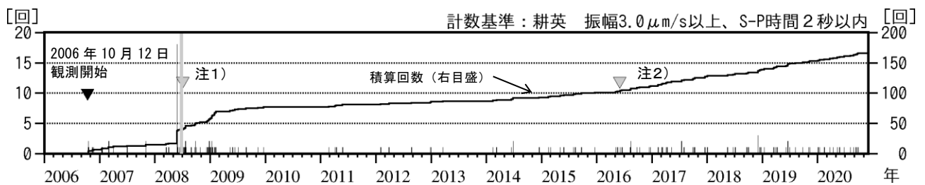
図3 栗駒山 日別地震回数（2006年10月～2020年11月）
