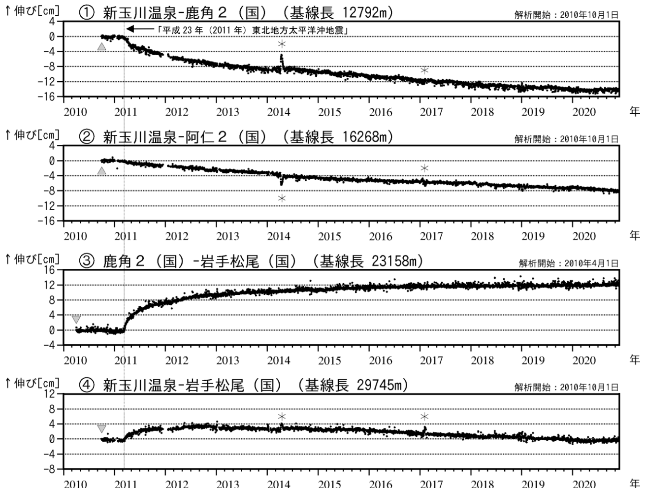
図4 秋田焼山 GNSS 基線長変化図（2010年4月～2020年11月）
