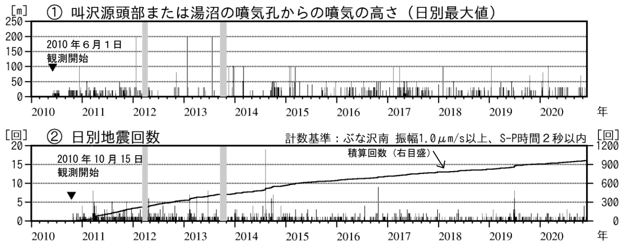
図3 秋田焼山 火山活動経過図（2010年6月～2020年11月）
