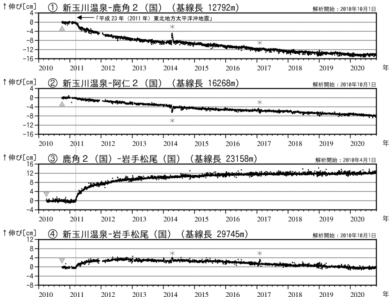
図4 秋田焼山 GNSS 基線長変化図（2010年4月～2020年10月）
