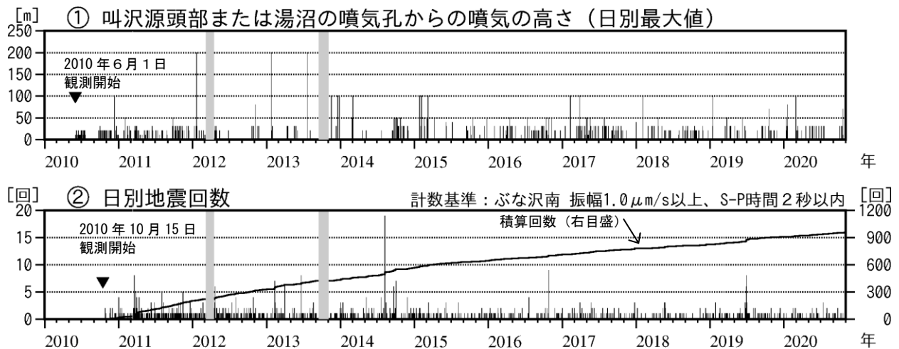
図3 秋田焼山 火山活動経過図（2010年6月～2020年10月）
