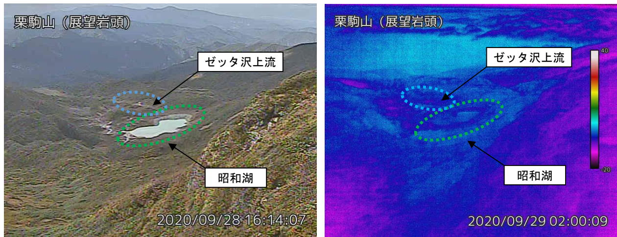
図2 栗駒山 昭和湖及びゼッタ沢上流周辺の状況（9月28日）と地表面温度分布（9月29日） ・展望岩頭監視カメラ（昭和湖の南南西約900m）の映像です。
