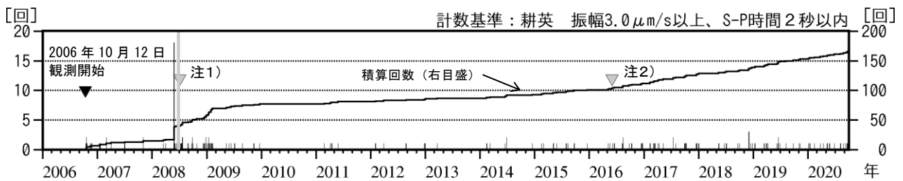
図3 栗駒山 日別地震回数（2006年10月～2020年9月）
