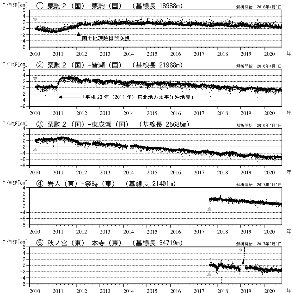
図4 栗駒山 GNSS 基線長変化図 (2010年4月～2020年9月)
