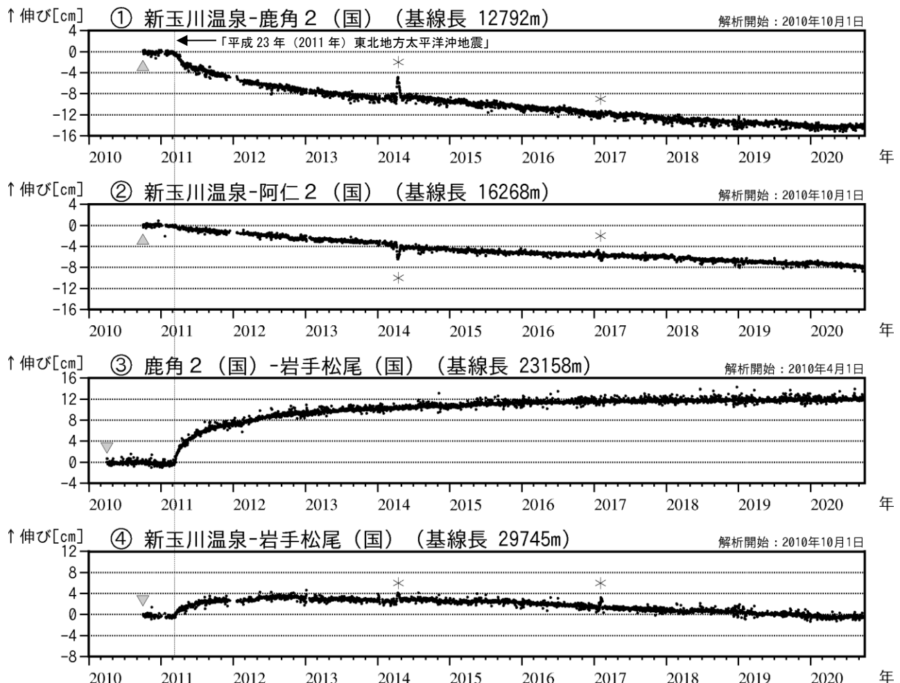
図4 秋田焼山 GNSS 基線長変化図（2010年4月～2020年9月）
