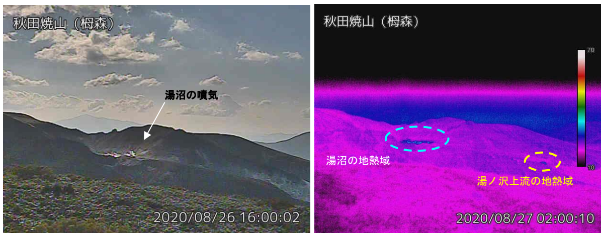
図2 秋田焼山 湯沼と湯ノ沢上流の状況（8月26日）と地表面温度分布（8月27日）
