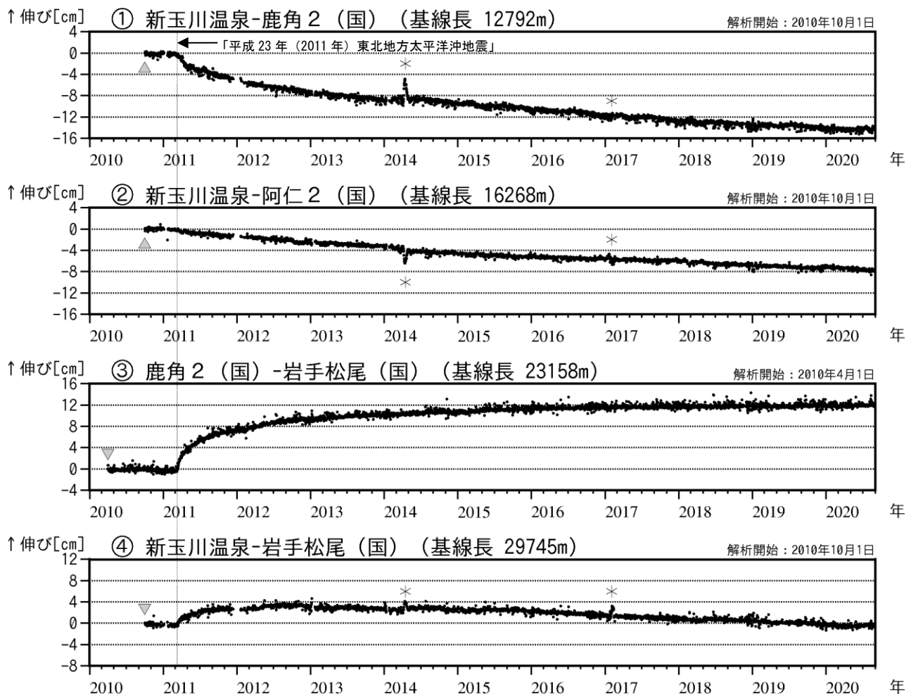
図4 秋田焼山 GNSS 基線長変化図（2010年4月～2020年8月）
