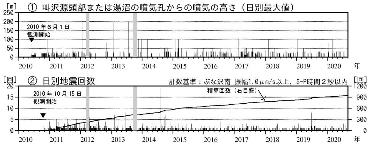
図3 秋田焼山 火山活動経過図（2010年6月～2020年8月）
