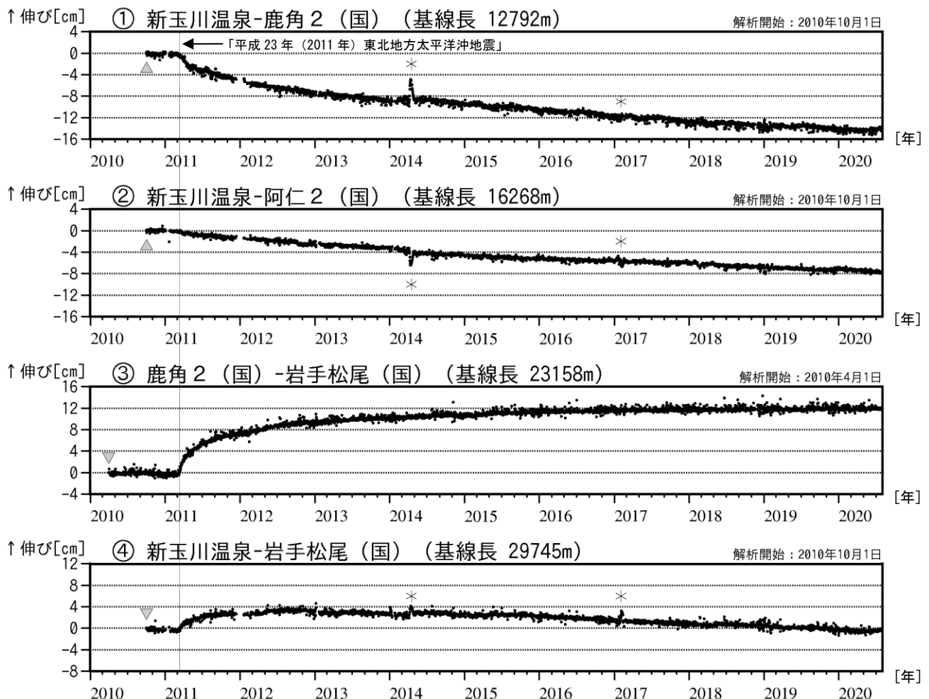
図4 秋田焼山 GNSS 基線長変化図（2010年4月～2020年7月）
