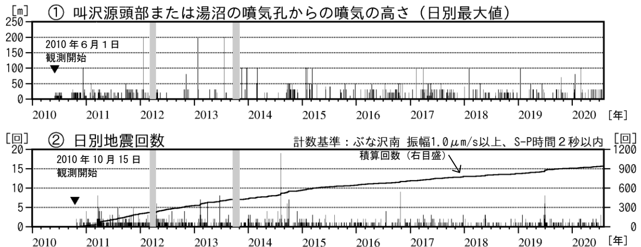
図3 秋田焼山 火山活動経過図（2010年6月～2020年7月）
