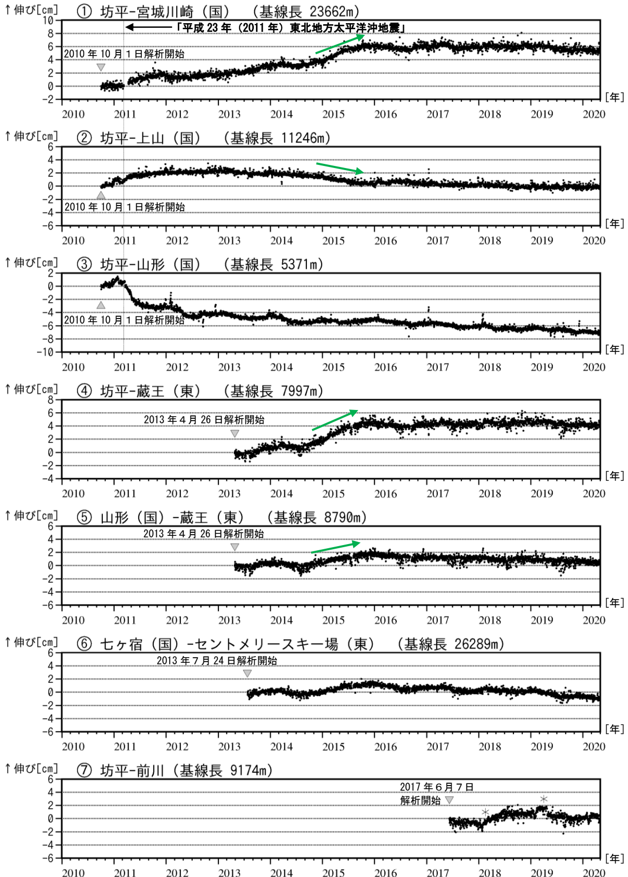
図4 蔵王山 GNSS 基線長変化図（2010 年 10 月～2020 年 4 月）
