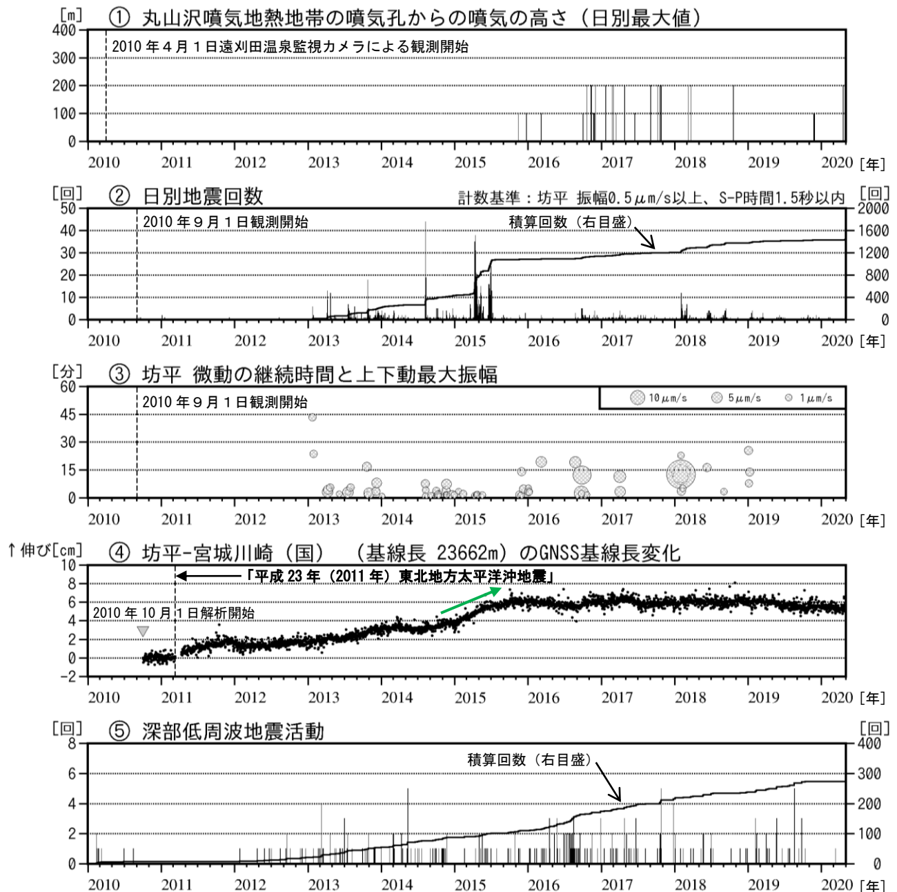
図2 蔵王山 火山活動経過図（2010年4月～2020年4月）
