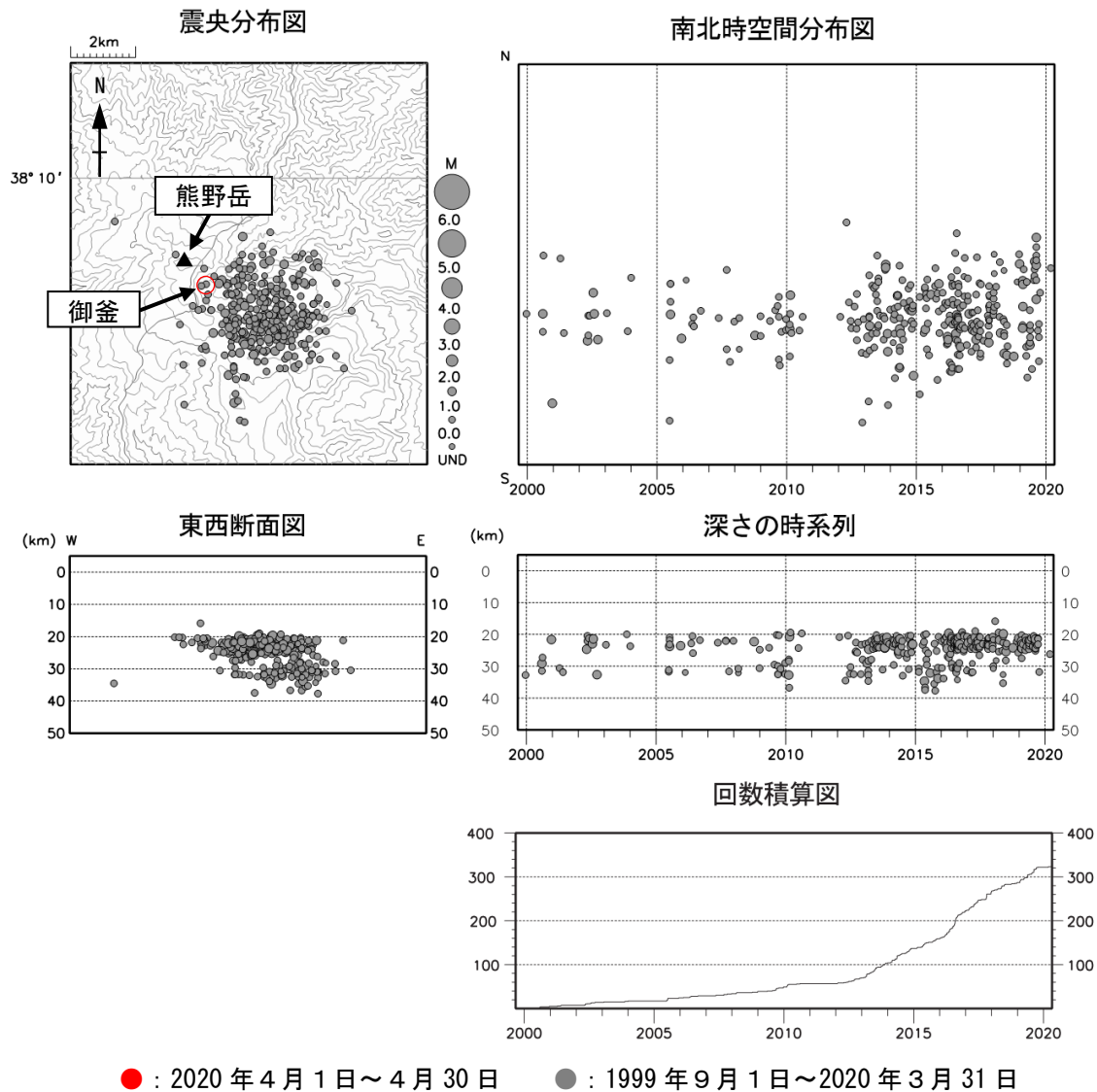
図3 蔵王山 広域地震観測網による深部低周波地震活動（1999年9月～2020年4月）
