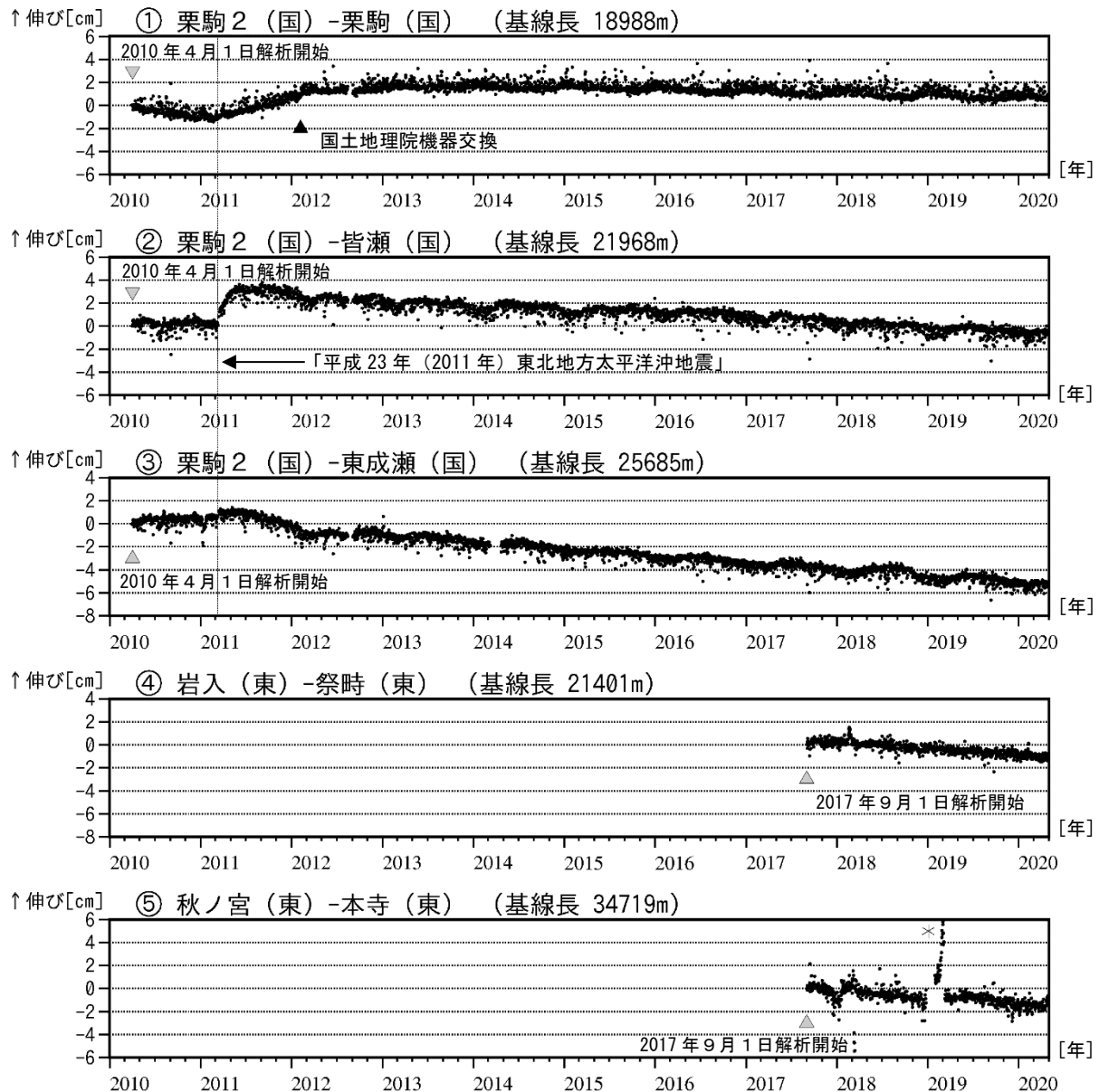
図3 栗駒山 GNSS 基線長変化図（2010年4月～2020年4月）
