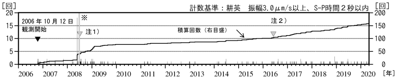
図2 栗駒山 日別地震回数（2006年10月～2020年4月）
