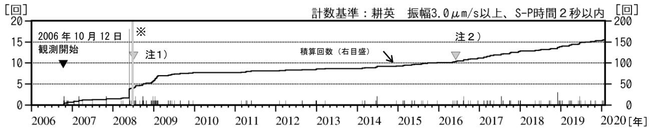
図2 栗駒山 日別地震回数（2006年10月～2020年1月）
