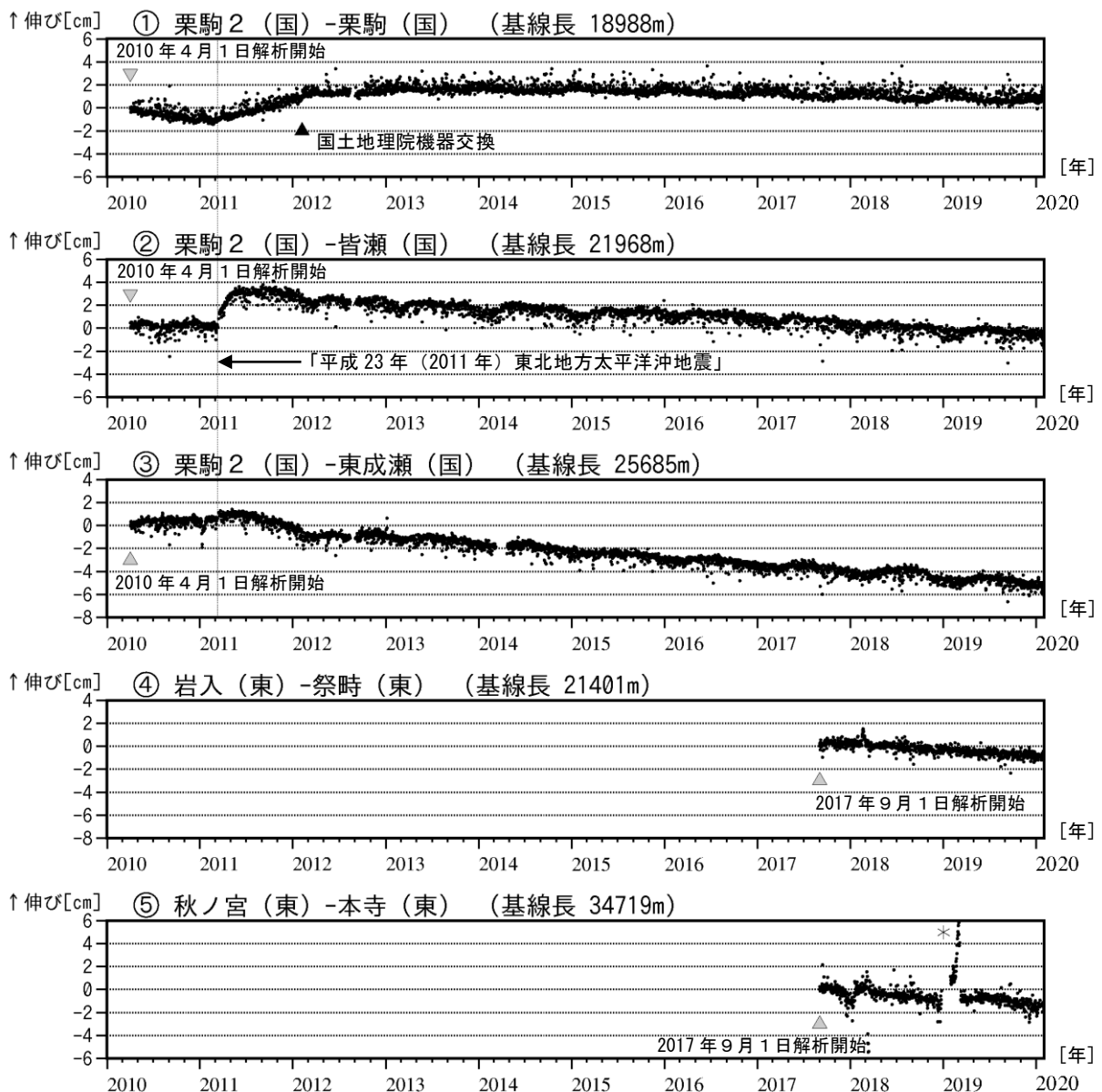
図3 栗駒山 GNSS 基線長変化図（2010年4月～2020年1月）
