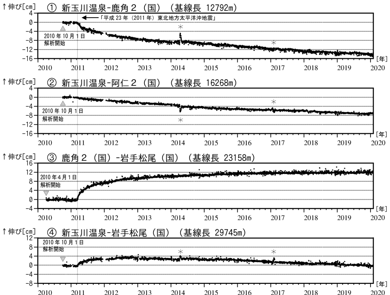
図4 秋田焼山 GNSS 基線長変化図（2010年4月～2020年1月）
