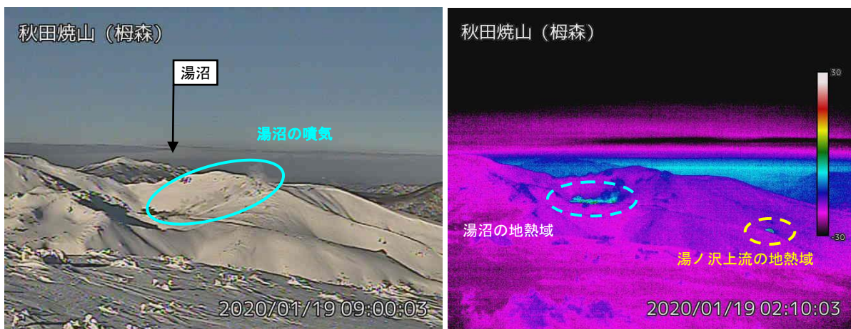
図2 秋田焼山 湯沼と湯ノ沢上流の状況と地表面温度分布（1月19日）
