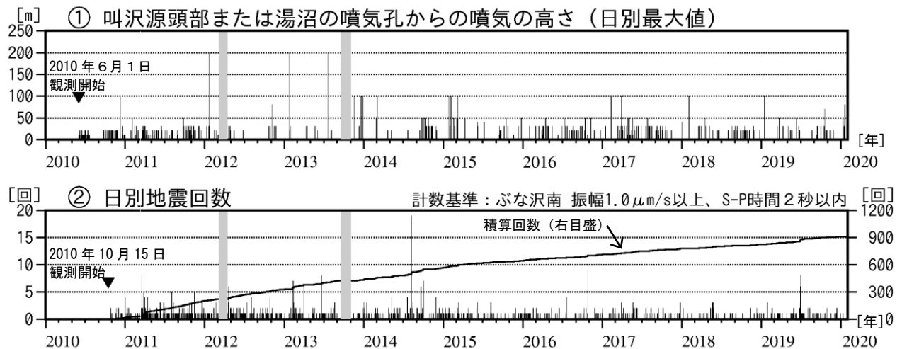
図3 秋田焼山 火山活動経過図（2010年6月～2020年1月）
