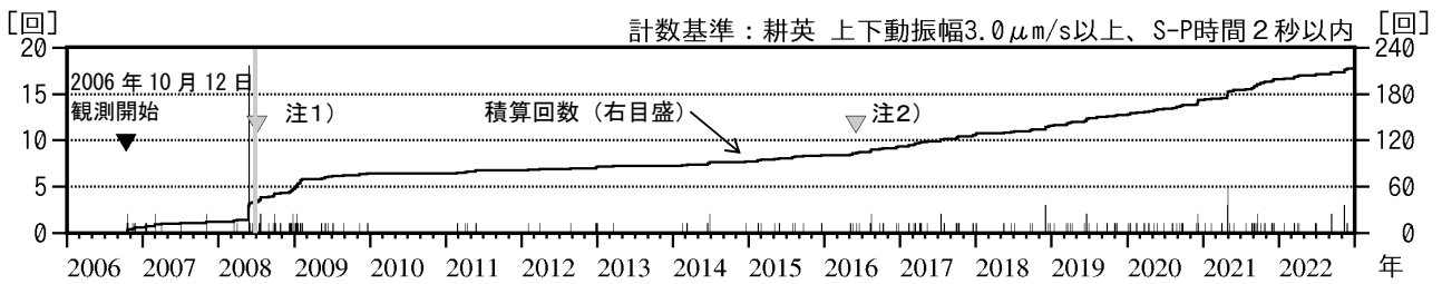
図10 栗駒山 日別地震回数 (2006年10月～2022年12月)
