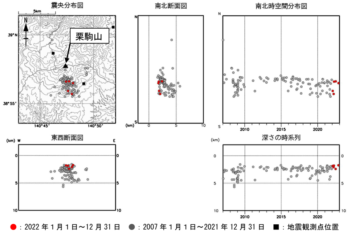
図11 栗駒山 地震活動 (2007年1月～2022年12月)
