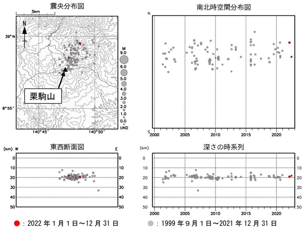
図12 栗駒山 広域地震観測網による深部低周波地震活動 (1999年9月～2022年12月)
