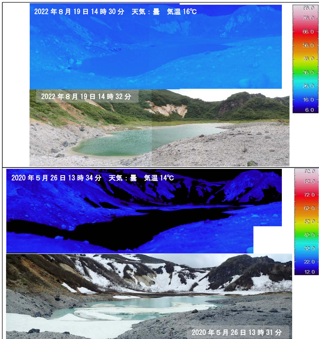
図6 栗駒山 北東から撮影した昭和湖の状況と地表面温度分布
