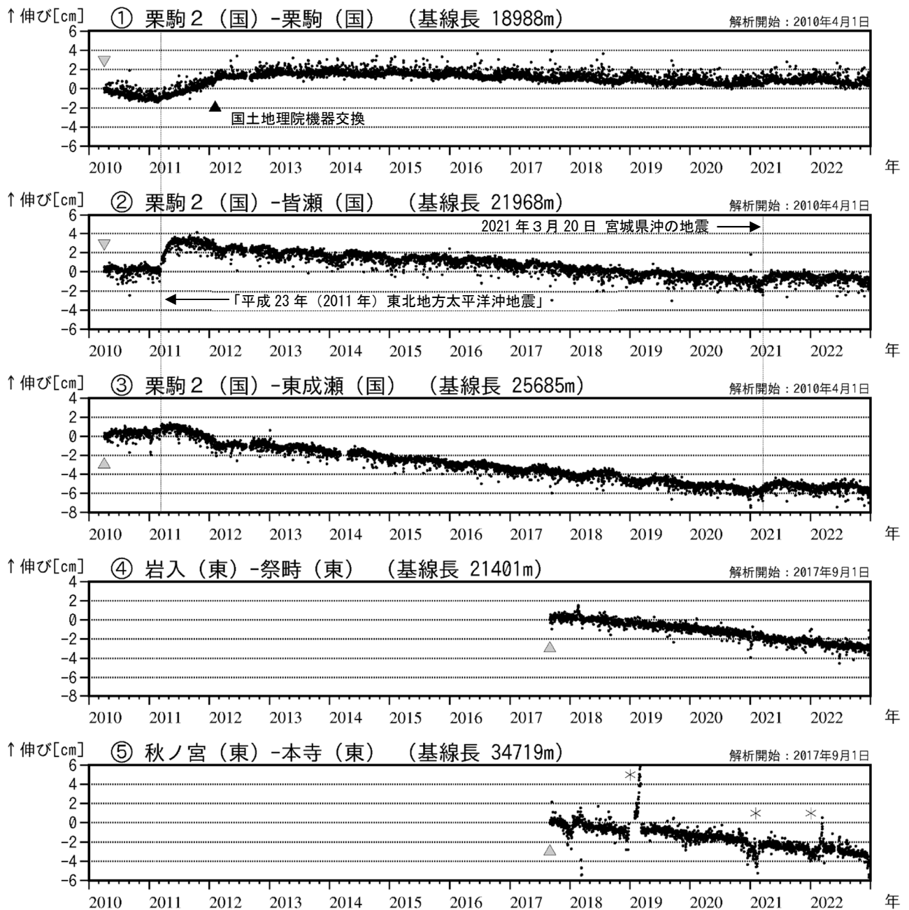
図 13 栗駒山 GNSS 基線長変化図 (2010年4月～2022年12月)
