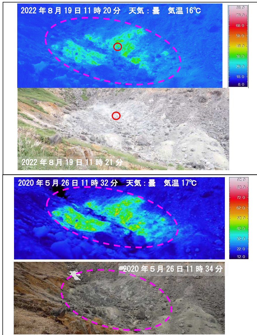
図7 栗駒山 北東から撮影したゼッタ沢上流の状況と地表面温度分布
