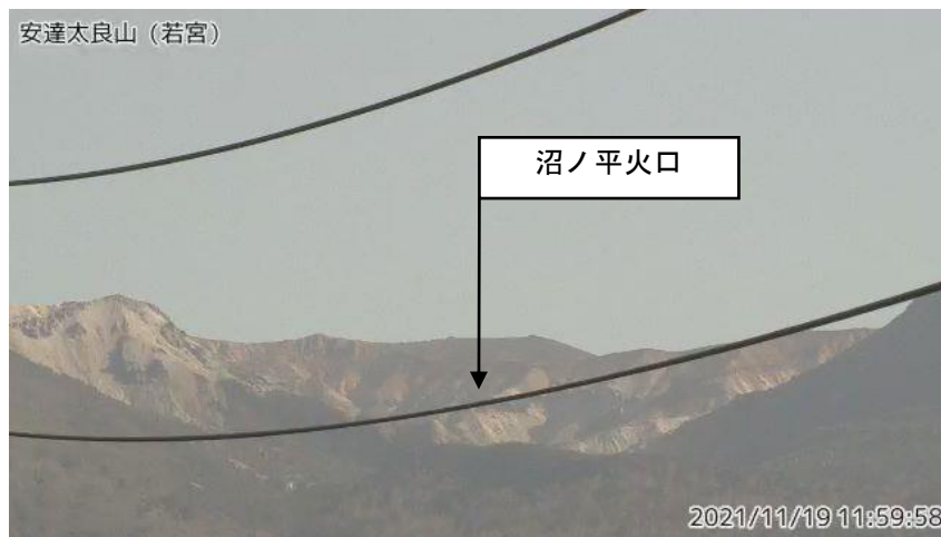
図1 安達太良山 沼ノ平火口周辺の状況（11月19日） ・若宮監視カメラ（沼ノ平火口の西北西約8km）の映像です。
