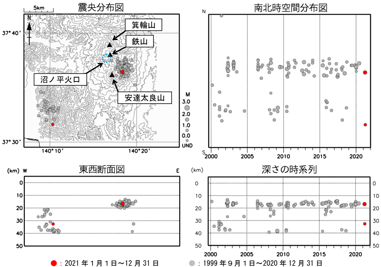
● : 2021年1月1日~12月31日 ● : 1999年9月1日~2020年12月31日 図8 安達太良山 広域地震観測網による深部低周波地震活動 (1999年9月~2021年12月)
