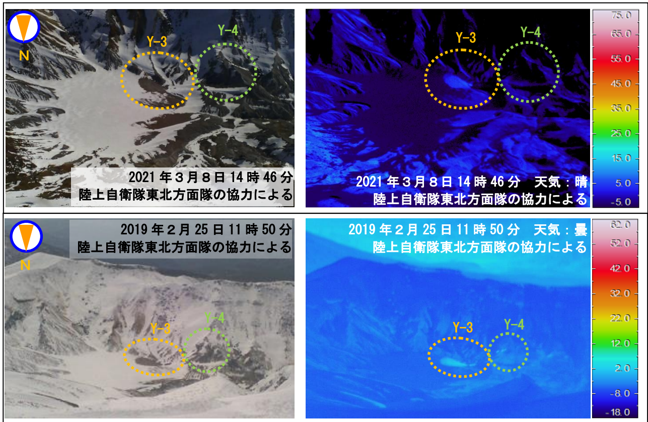
図4 安達太良山 上空から撮影した沼ノ平火口付近の状況と地表面温度分布
