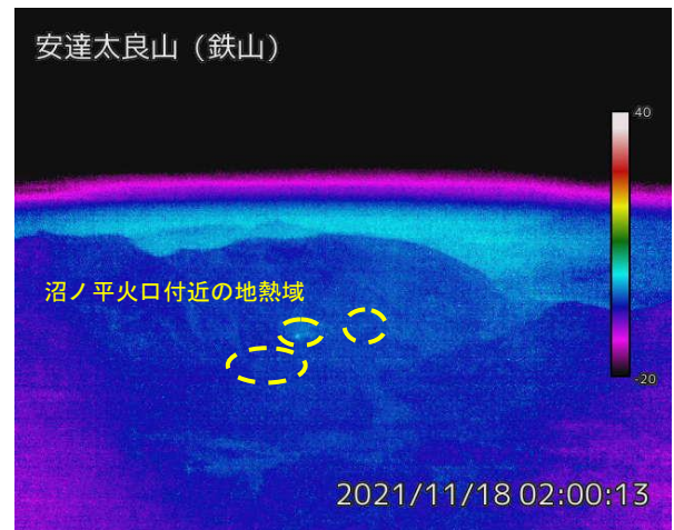
図2 安達太良山 沼ノ平火口周辺の状況と地表面温度分布（左：11月19日、右：11月18日） ・鉄山監視カメラ（沼ノ平火口の北東約700m）の映像です。
