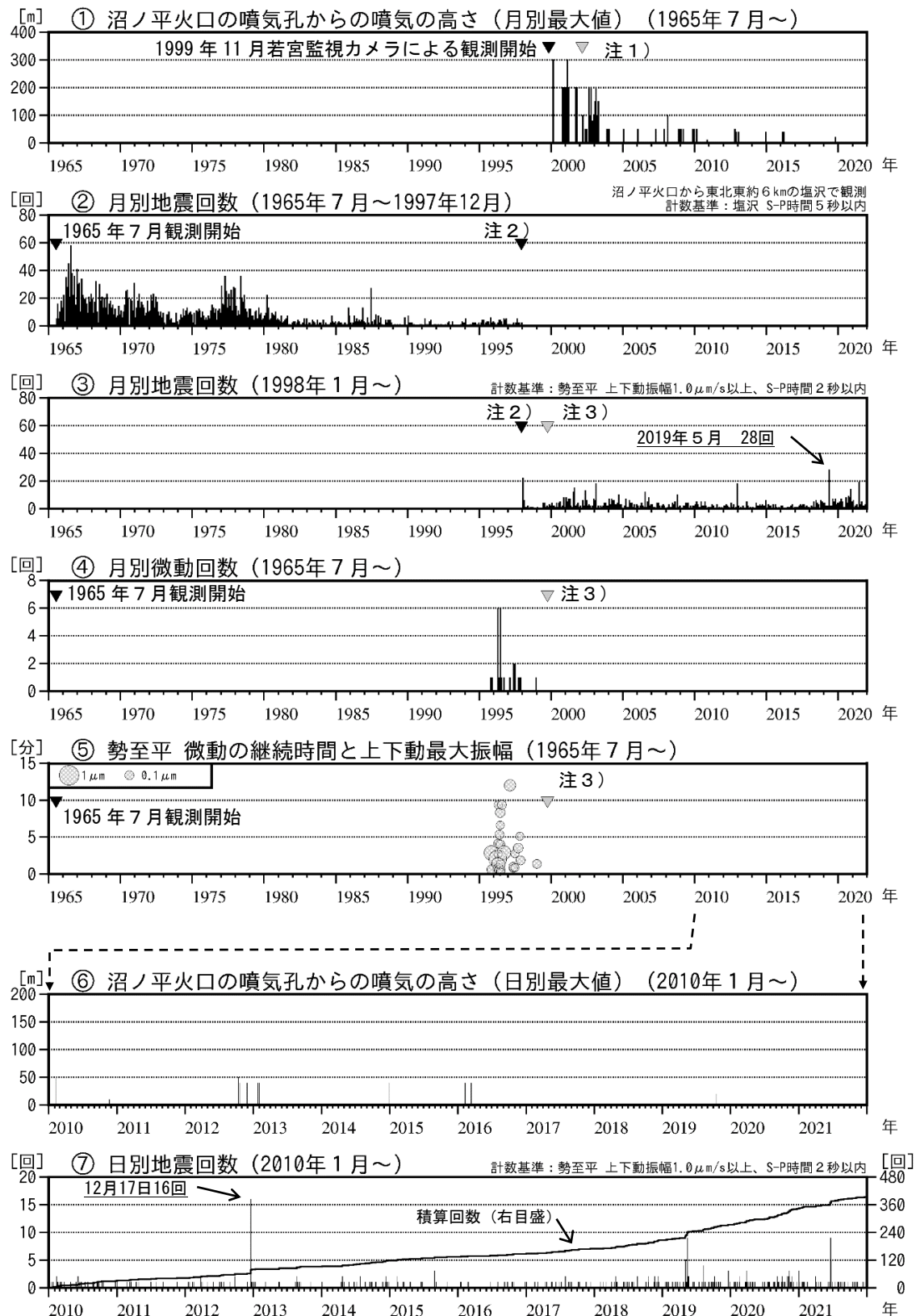
図6 安達太良山 火山活動経過図（1965年7月～2021年12月）
