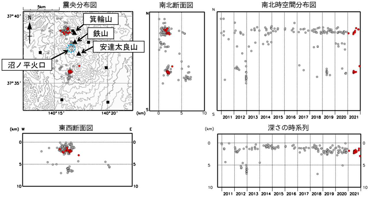
● : 2021年1月1日~12月31日 ● : 2010年9月1日~2020年12月31日 ■ : 地震観測点位置 図7 安達太良山 地震活動 (2010年9月~2021年12月) 火山性地震は少ない状態で経過し、火山性微動は観測されませんでした。
