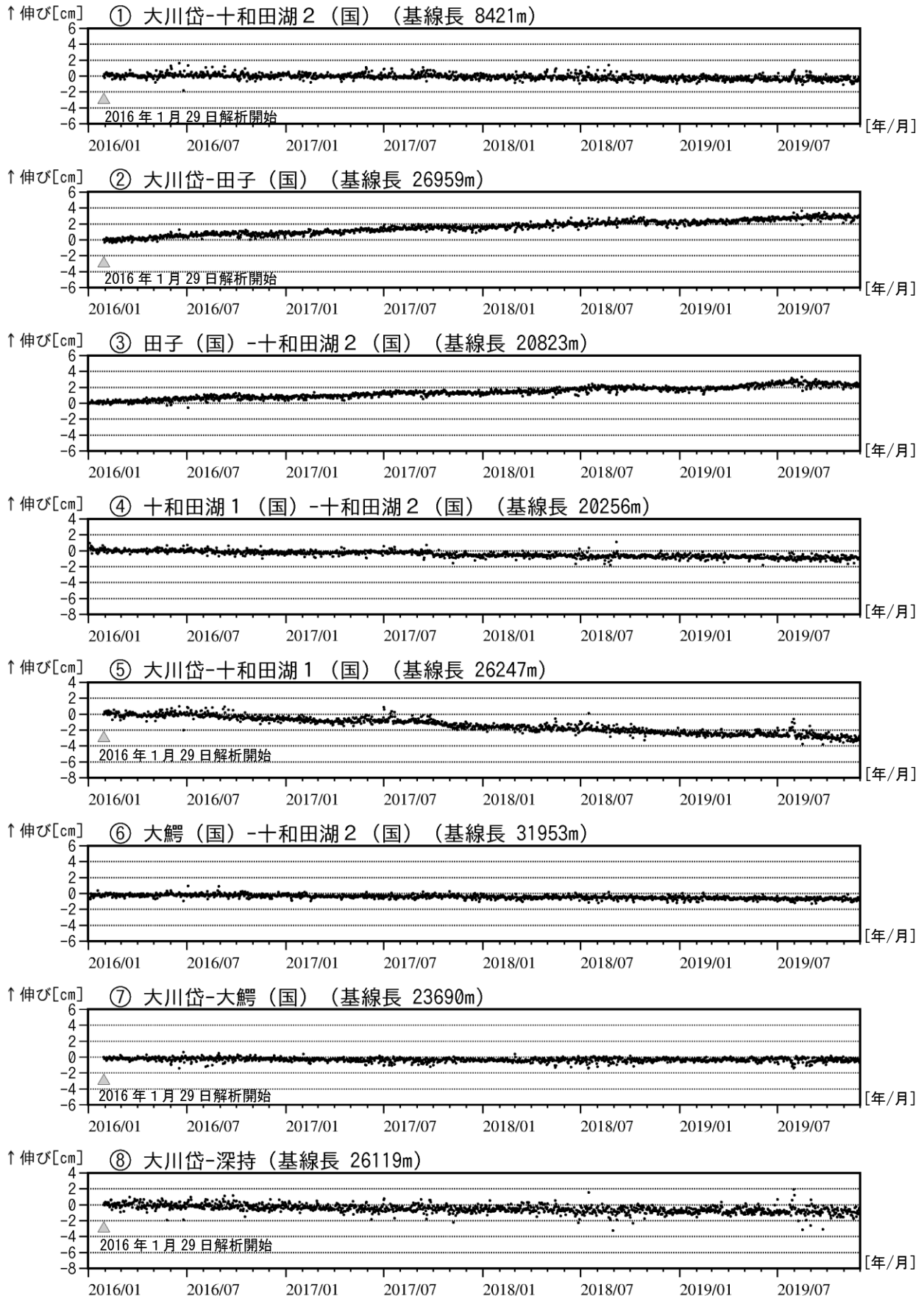
図3 十和田 GNSS 基線長変化図（2016年1月～2019年11月）
