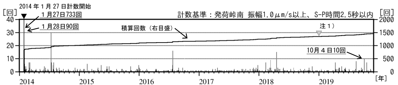
図2 十和田 日別地震回数（2014年1月～2019年11月） ・ 地震の計数基準観測点の変更は次のとおりです。 計数開始 2014年1月27日～ 防災科学技術研究所小坂観測点 注1) 2019年1月1日～ 発荷峠南観測点
