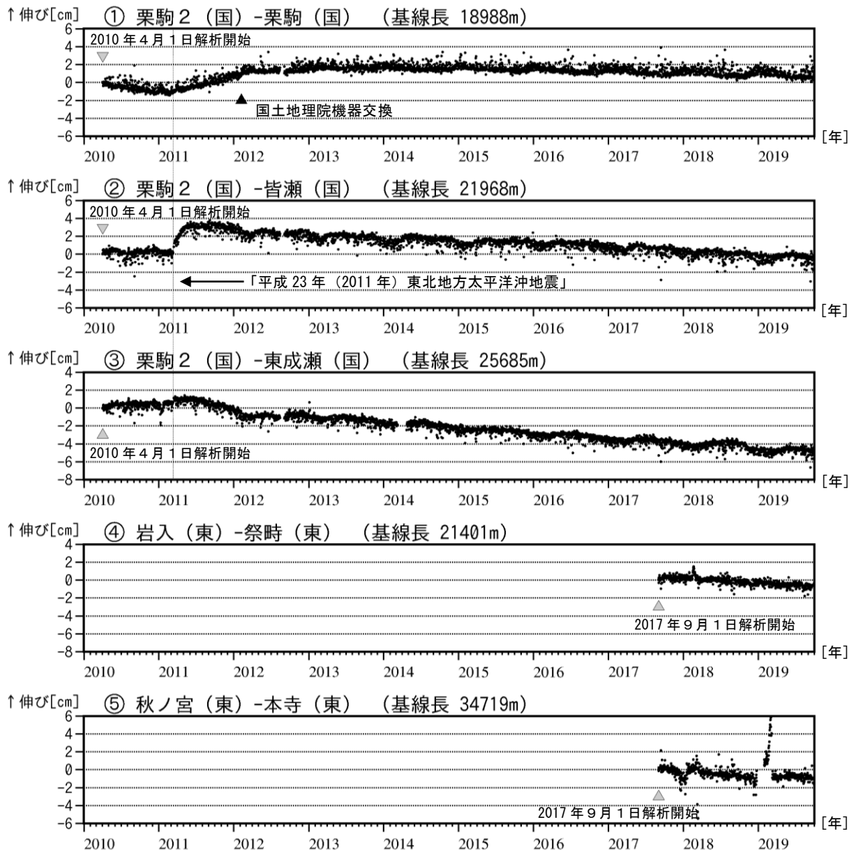
図3 栗駒山 GNSS 基線長変化図（2010年4月～2019年9月）
