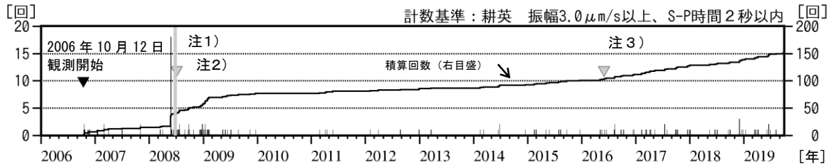
図2 栗駒山 日別地震回数（2006年10月～2019年9月）
