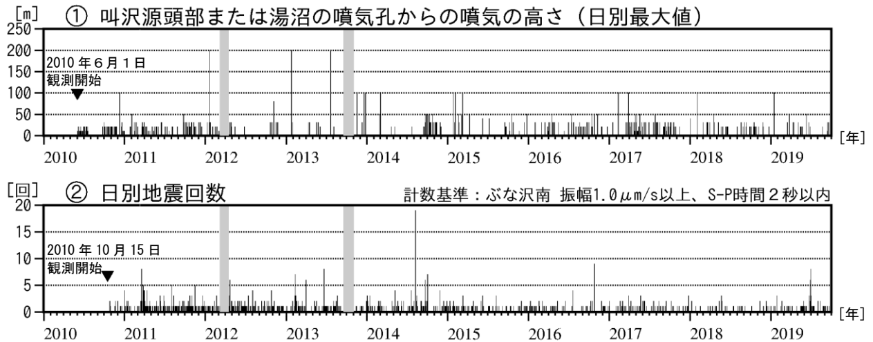
図3 秋田焼山 火山活動経過図（2010年6月～2019年9月）
