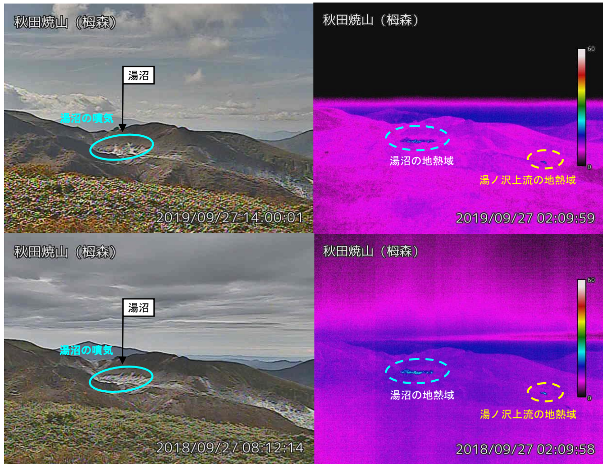
図2 秋田焼山 湯沼と湯ノ沢上流の状況と地表面温度分布（柵森監視カメラによる）
