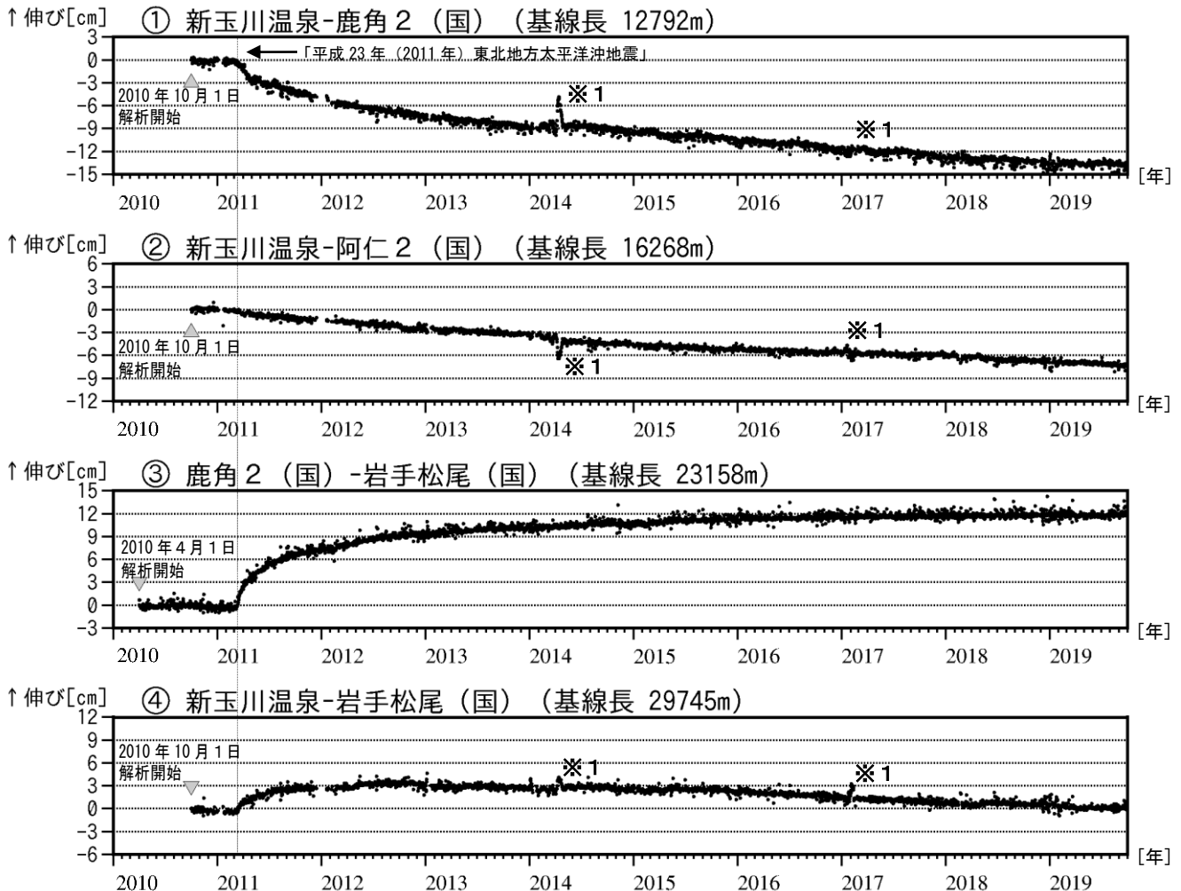
図4 秋田焼山 GNSS 基線長変化図（2010年4月～2019年9月）
