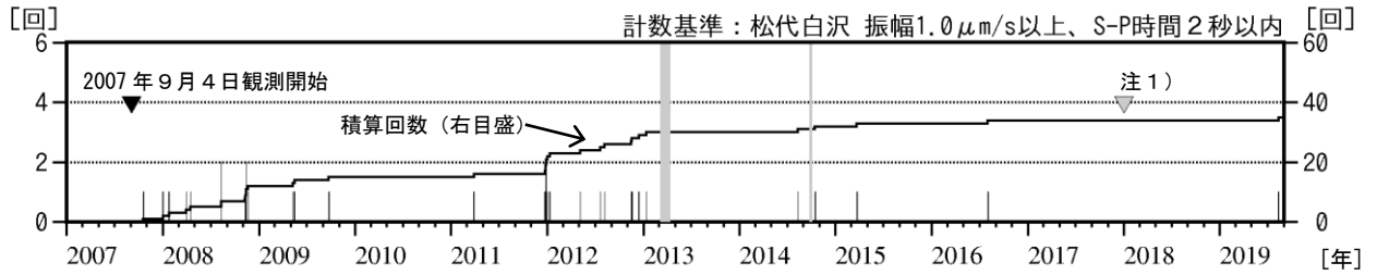
図2 岩木山 日別地震回数（2007年9月～2019年8月）
