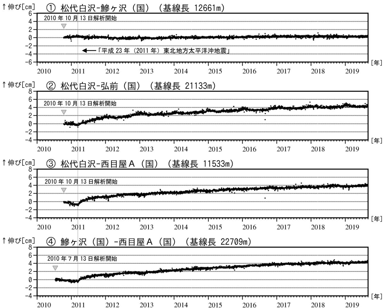
図3 岩木山 GNSS 基線長変化図（2010年7月～2019年8月）
