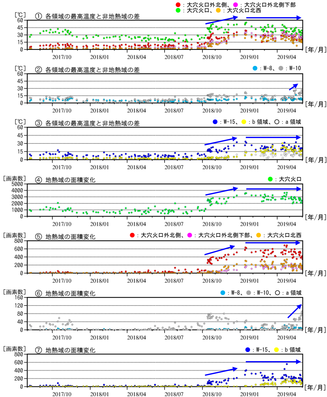
図13 吾妻山 監視カメラによる大穴火口周辺の地熱域の経過（2017年8月～2019年5月）
