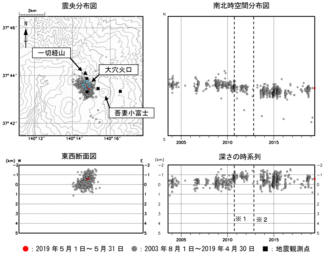
図8 吾妻山 地震活動（2003年8月～2019年5月）
