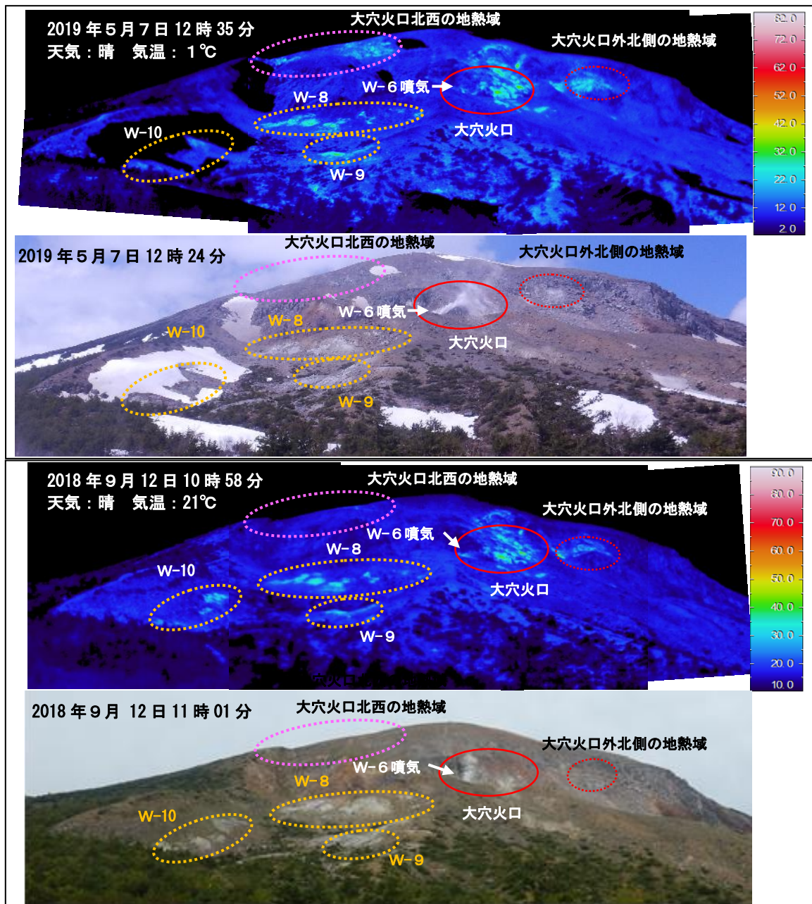
図 17 吾妻山 大穴火口付近及び八幡焼の状況と地表面温度分布
