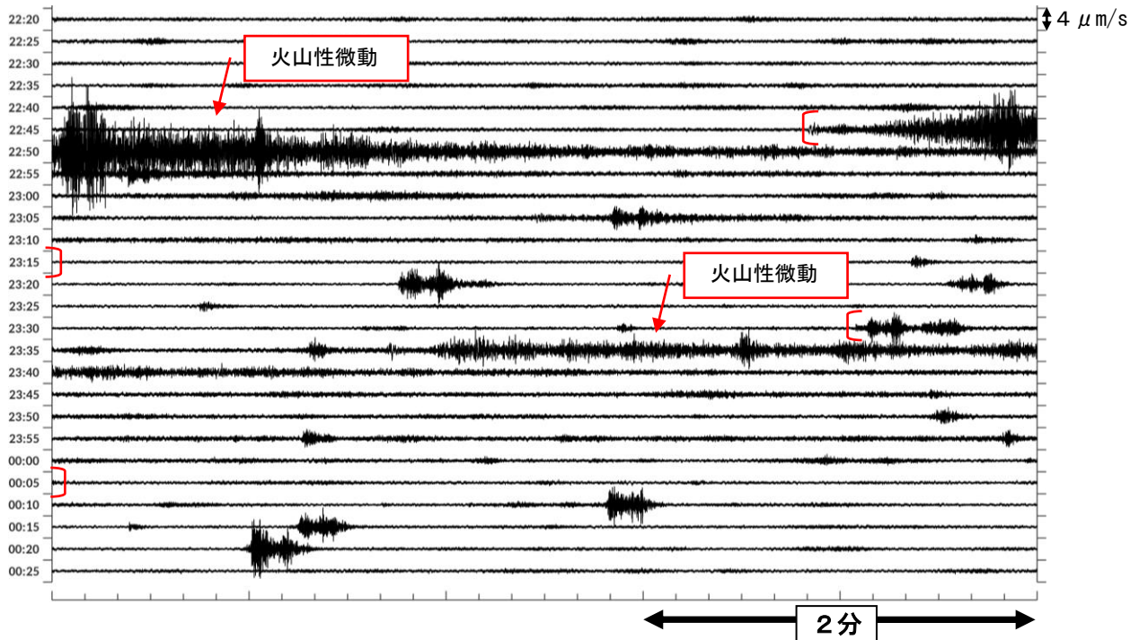
図5 吾妻山 吾妻小富士東観測点（上下成分）での火山性微動と火山性地震の発生状況 （2019年5月9日22時20分～10日00時30分）
