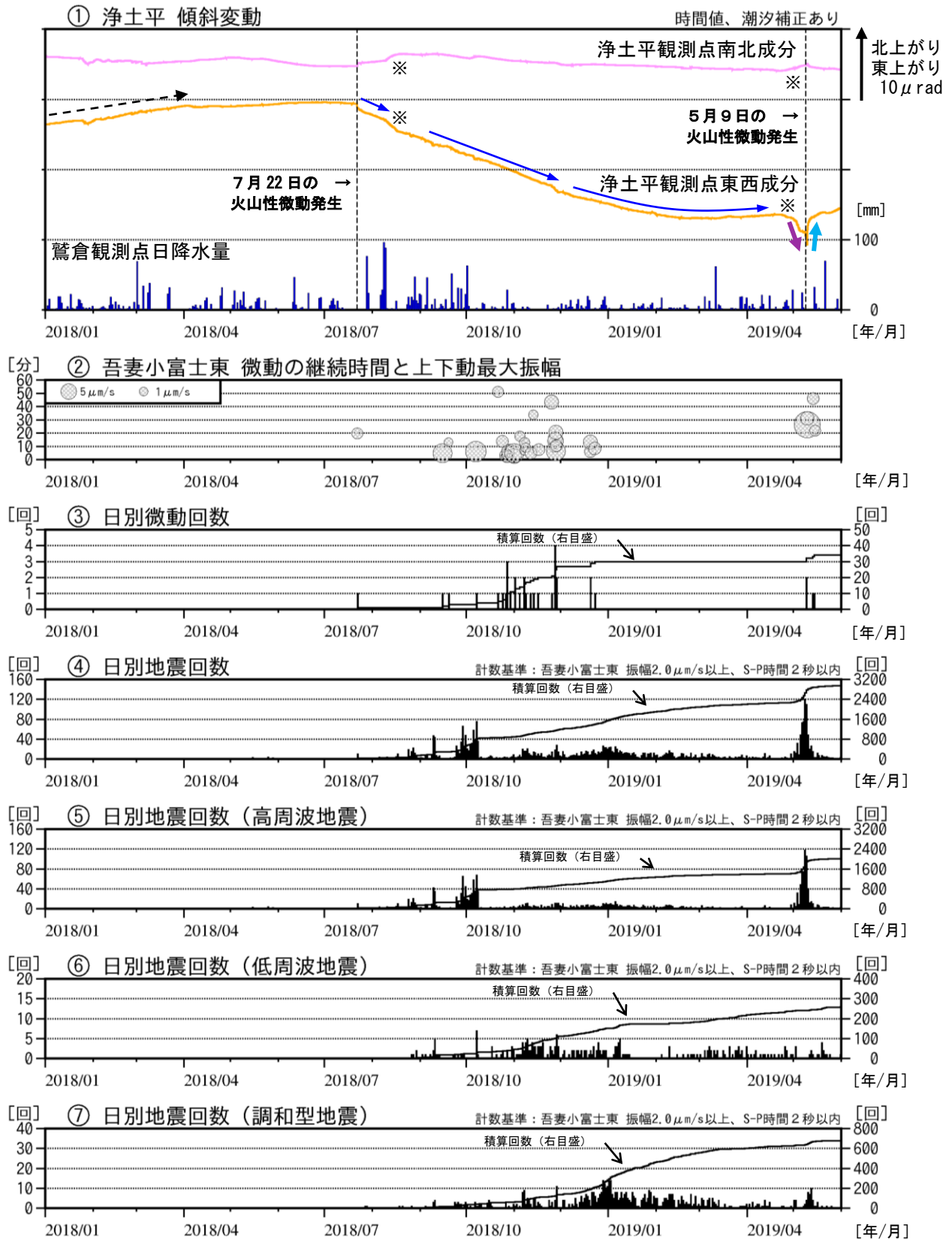
図2 吾妻山 浄土平観測点における傾斜変動、火山性微動の発生状況及び日別地震回数 (2018年1月～2019年5月)
