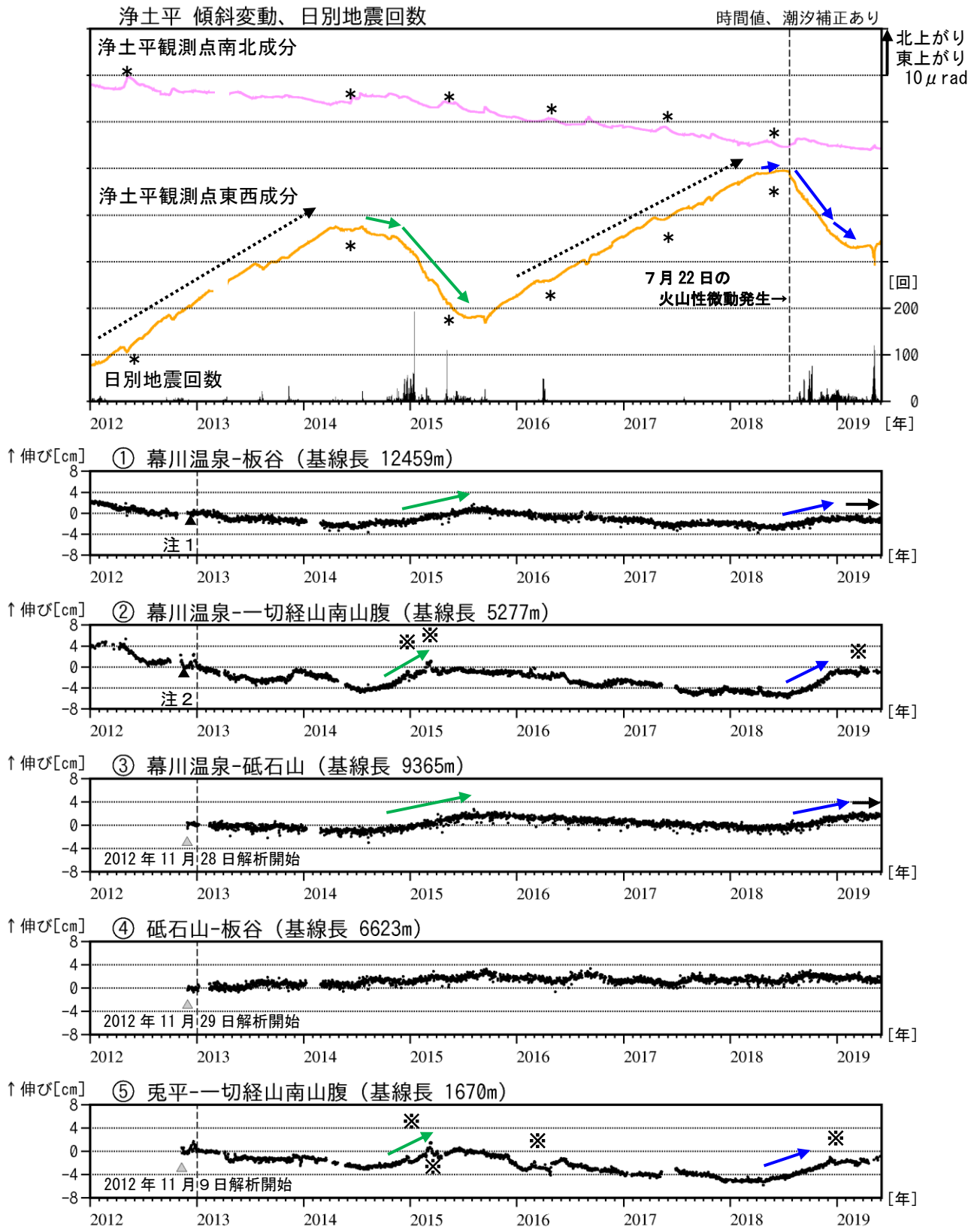
図9 吾妻山 傾斜変動及びGNSS基線長変化図（2012年1月～2019年5月）
