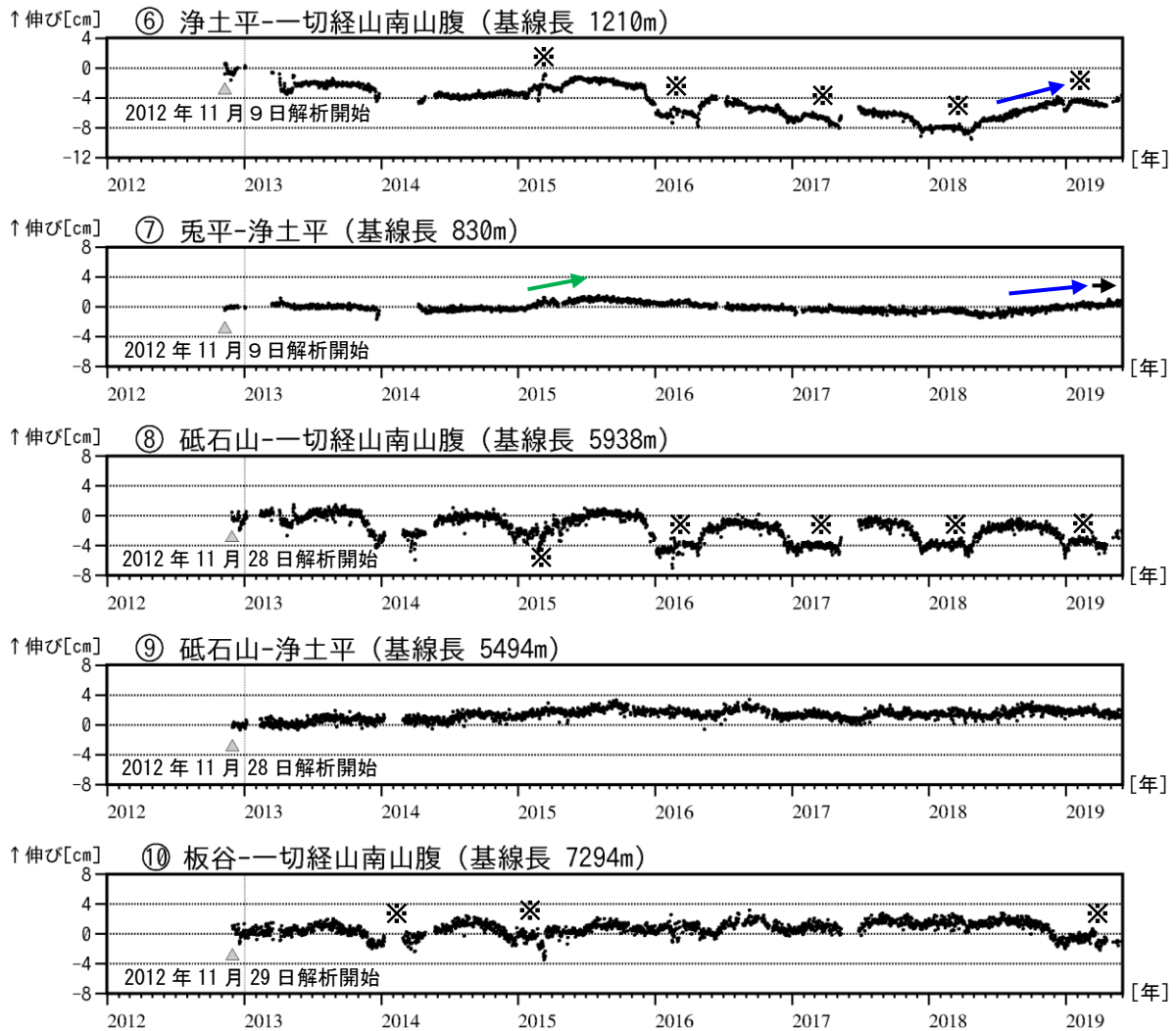
図10 吾妻山 GNSS 基線長変化図（2012年11月～2019年5月）
