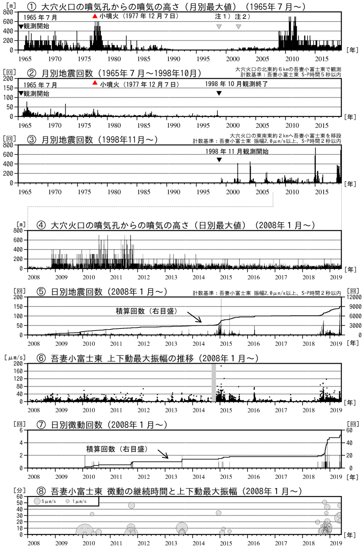
図7 吾妻山 火山活動経過図（1965年7月～2019年5月）
