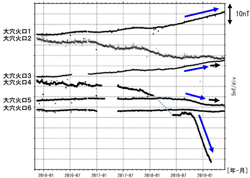
図20 吾妻山 全磁力連続観測点の全磁力値変化（2015年11月～2019年5月）
