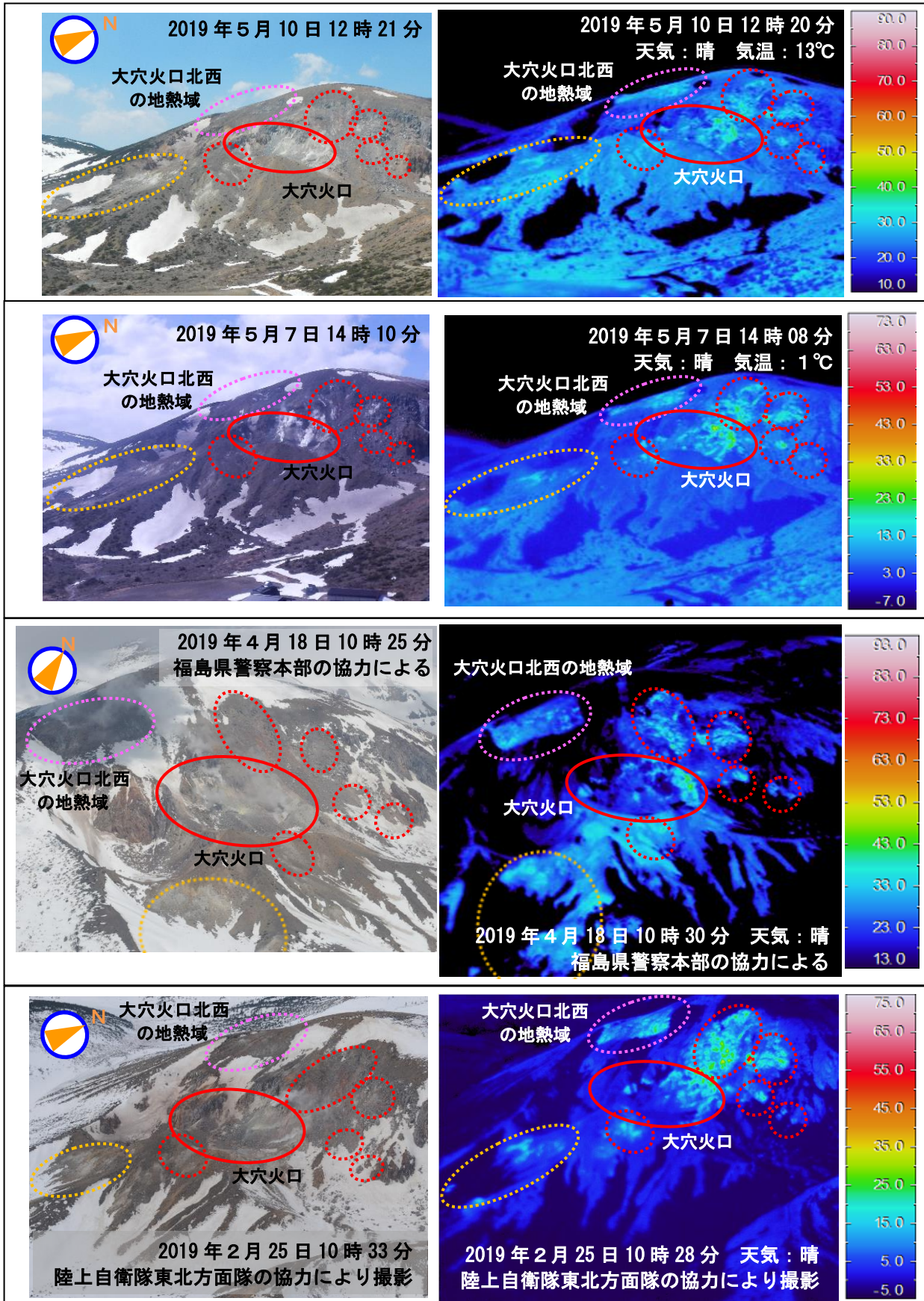
図 16 吾妻山 大穴火口付近及びその周辺の状況と地表面温度分布
