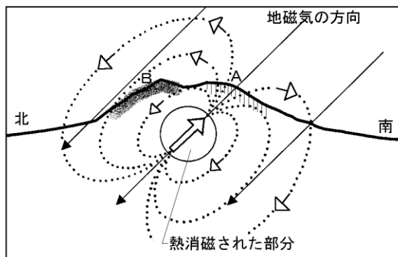
図21 熱消磁に伴う全磁力変化のモデル
