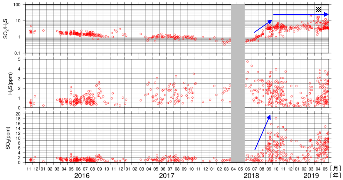
図 18 吾妻山 火山ガス観測装置による観測（2015年11月～2019年5月）
