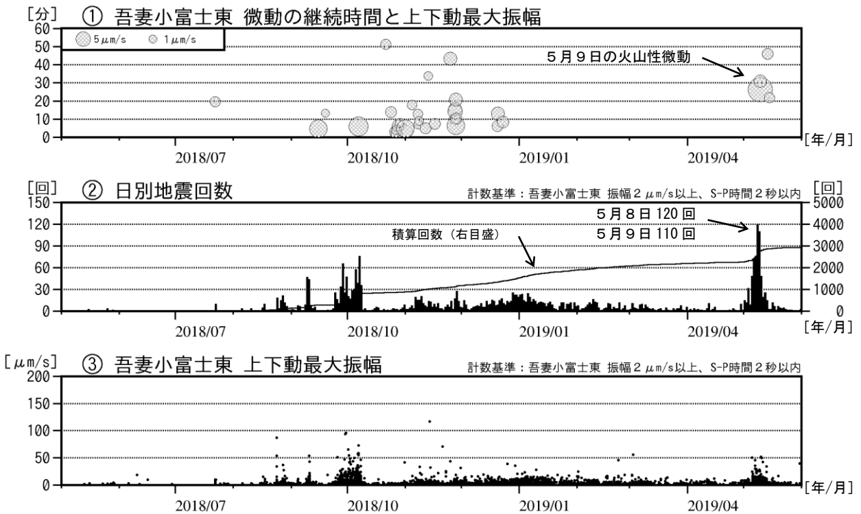
図3 吾妻山 火山性微動の発生状況及び地震回数（2018年5月～2019年5月）
