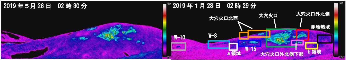
図12 吾妻山 浄土平3監視カメラ（熱映像）による大穴火口周辺の地熱域の状況
