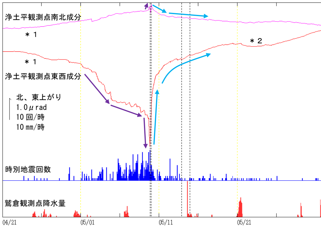
図6 吾妻山 浄土平観測点における傾斜変動 （2019年4月21日～5月31日、分値、潮汐補正済み）
