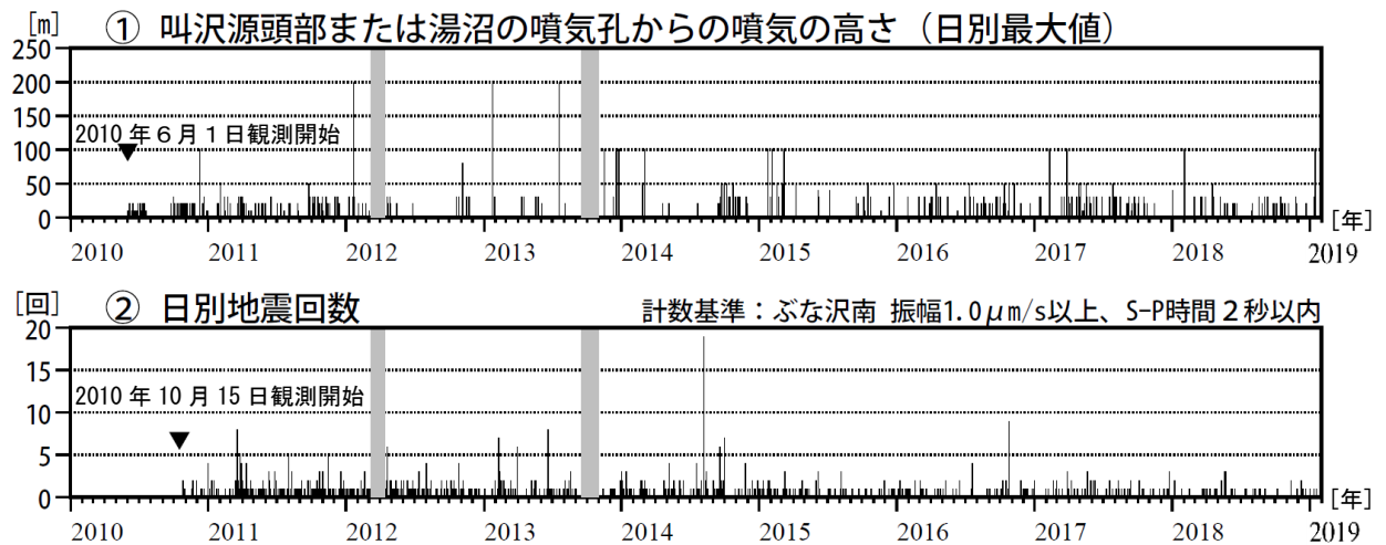
図2 秋田焼山 火山活動経過図（2010年6月～2019年1月）
