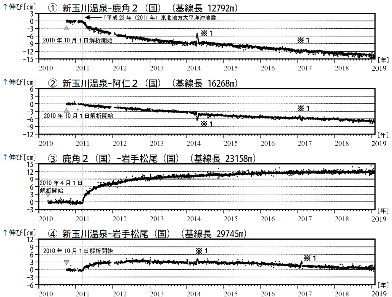
図3 秋田焼山 GNSS 1) 基線長変化図（2010年4月～2019年1月）
