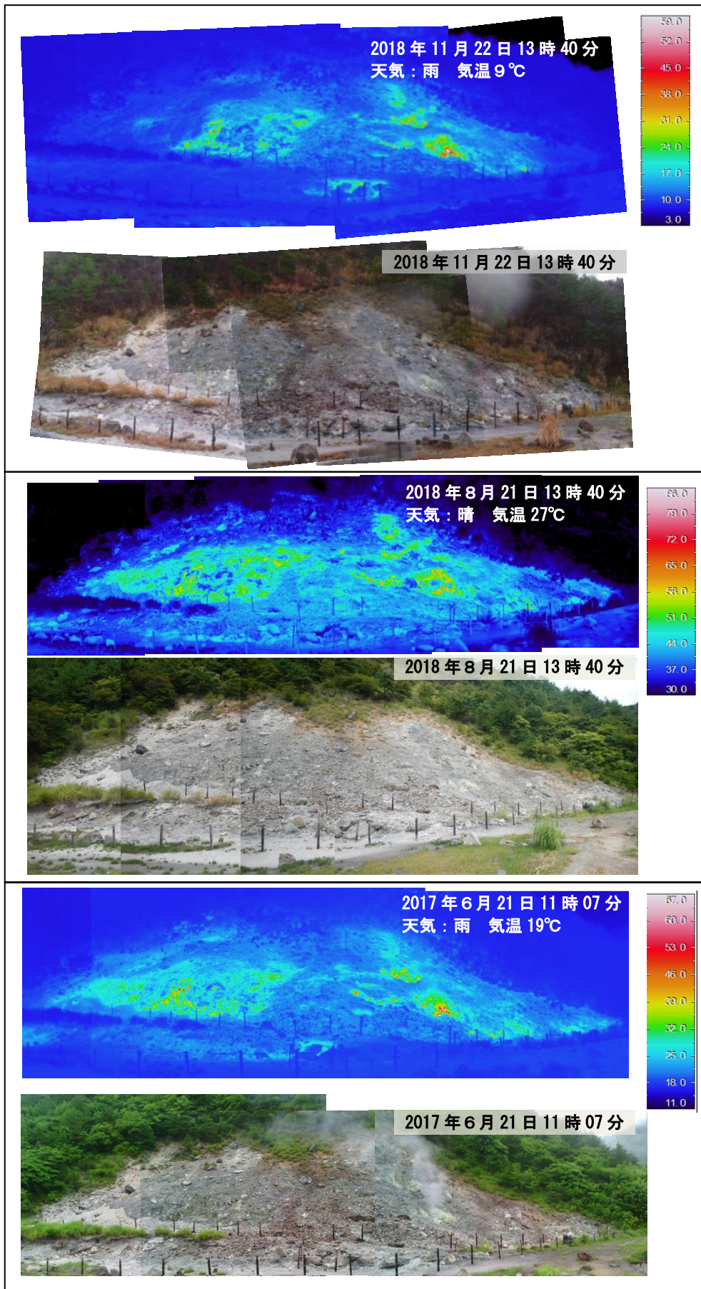
図2 鳴子 南西から撮影した胡桃ヶ岳南西麓の地熱域の状況と地表面温度分布
