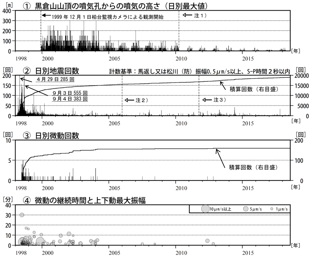
図 7 岩手山 火山活動経過図（1998 年 1 月～2018 年 7 月）
