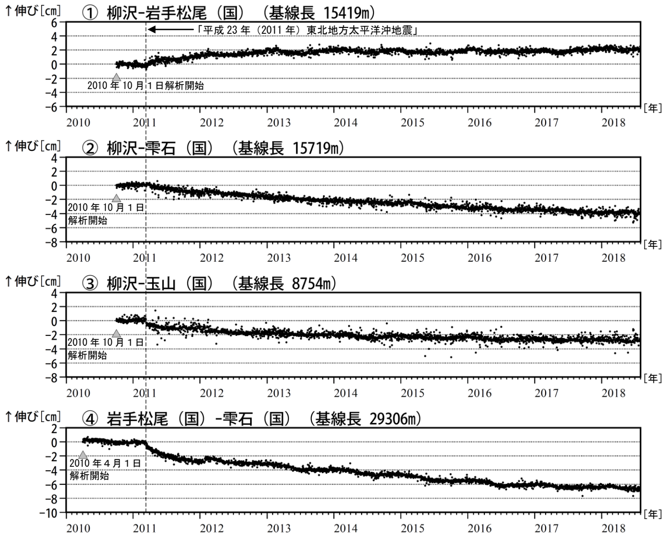
図 9 岩手山 GNSS 1) 基線長変化図（2010 年 4 月～2018 年 7 月）
