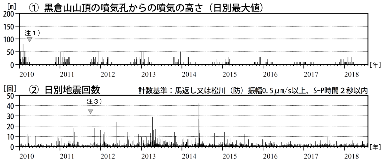
図 8 岩手山 噴気の高さ及び日別地震回数（2010 年 1 月～2018 年 7 月）
