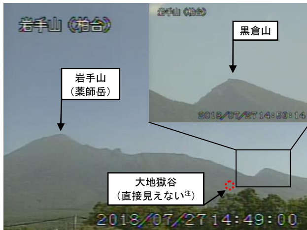
図 1 岩手山 黒倉山の噴気の状況 （7 月 27 日）
