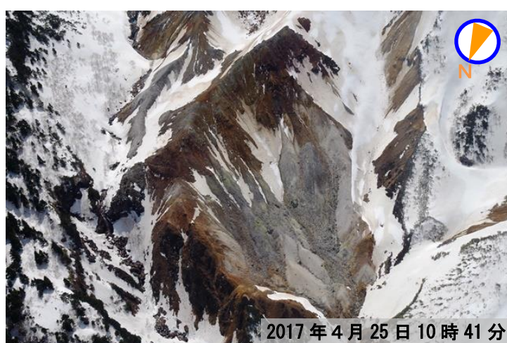
図 6 岩手山 上空からの大地獄谷の状況
