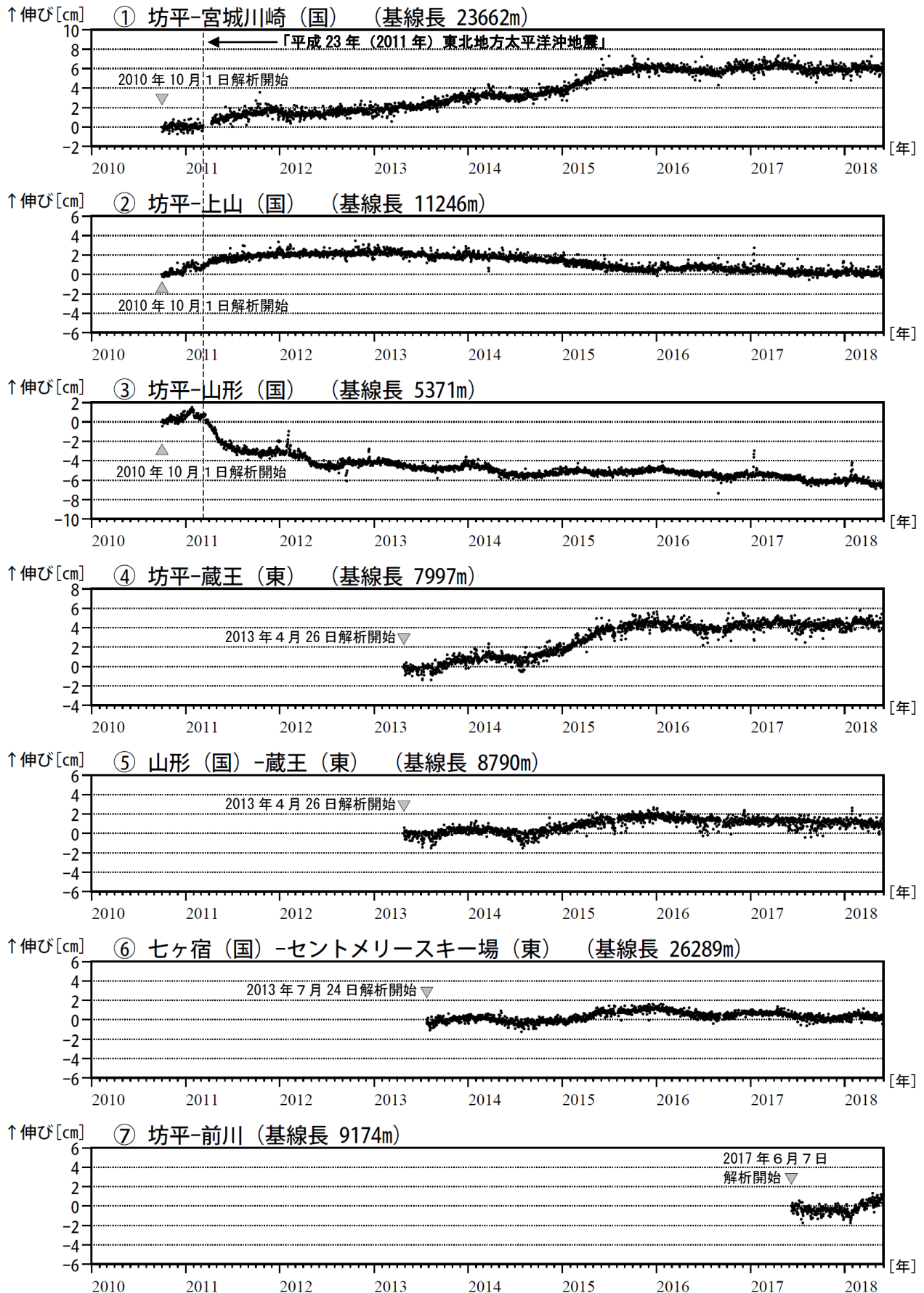
図 4 蔵王山 GNSS 基線長変化図 (2010 年 10 月～2018 年 5 月)
