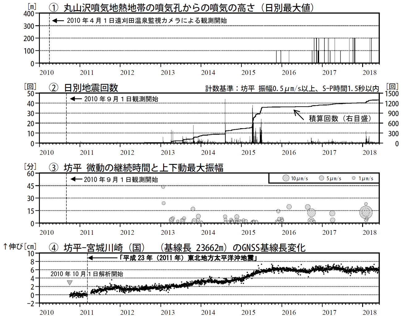
図 2 蔵王山 火山活動経過図（2010年 4 月～2018年 5 月）
