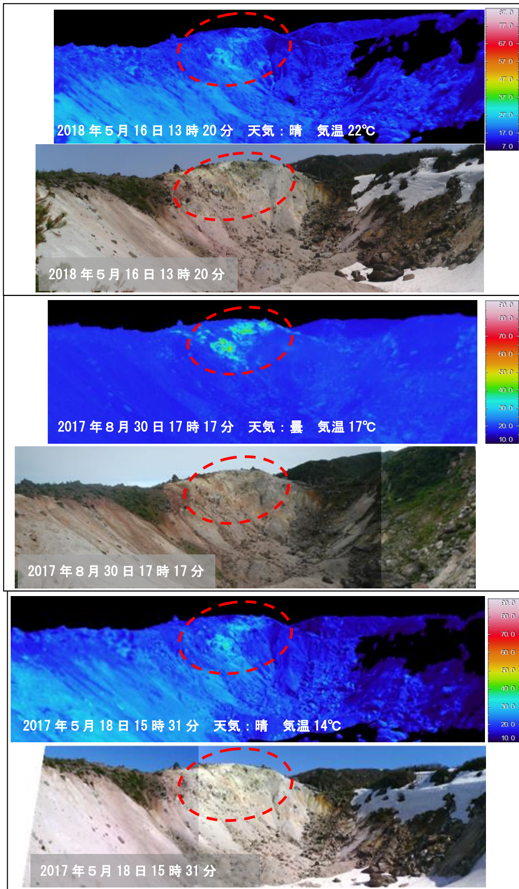
図7 栗駒山 北西から撮影した地獄釜の状況と地表面温度分布
