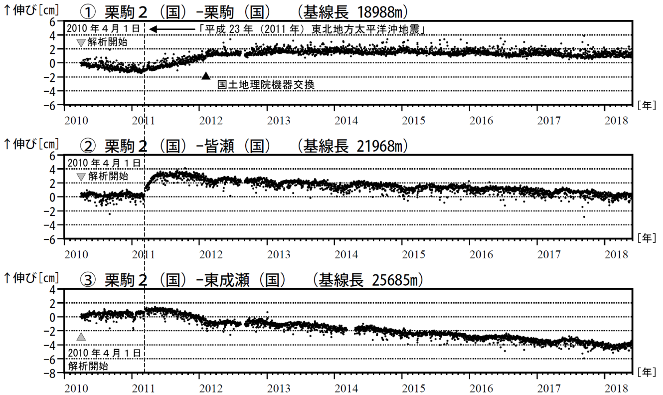
図 9 栗駒山 GNSS 2) 基線長変化図（2010 年 4 月～2018 年 5 月）
