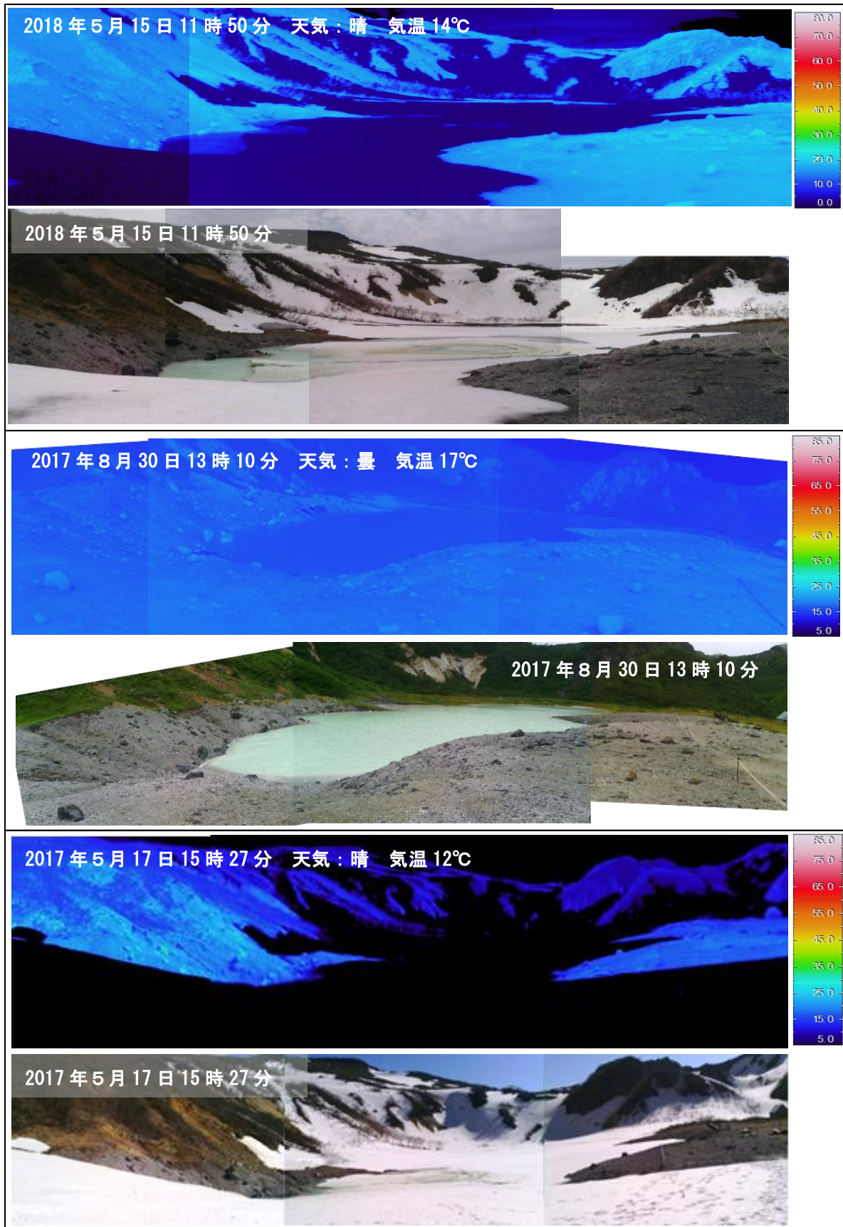
図 4 栗駒山 北東から撮影した昭和湖の状況と地表面温度分布
