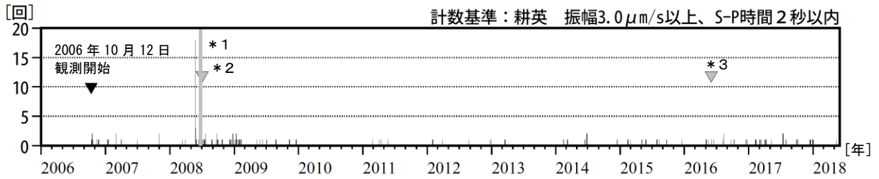
図 8 栗駒山 日別地震回数（2006 年 10 月～2018 年 5 月）
