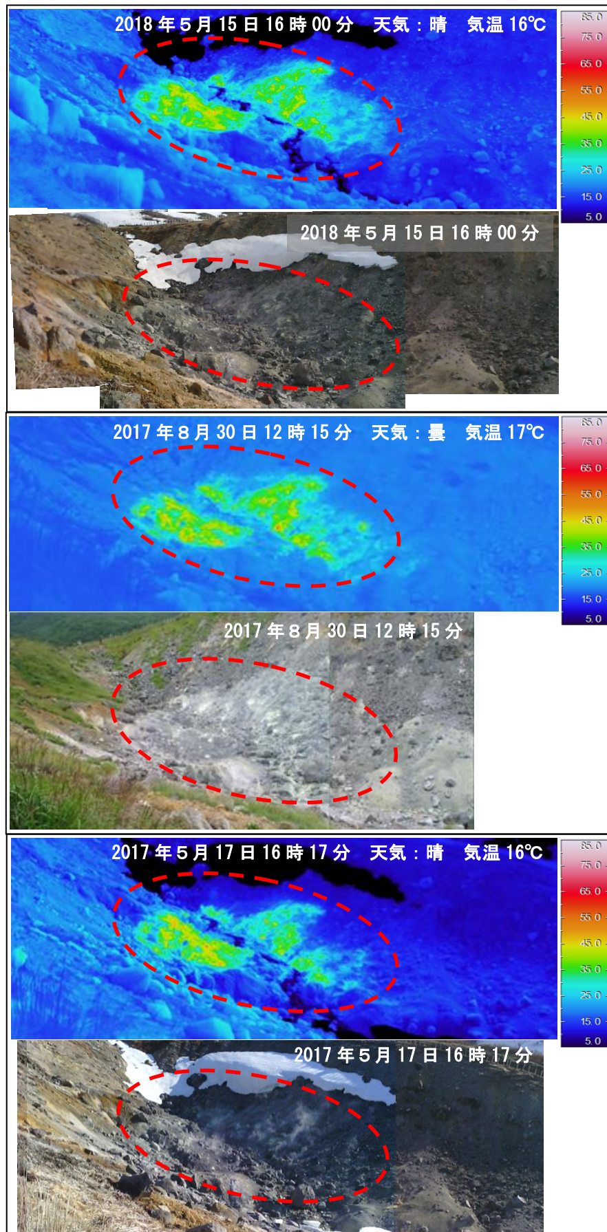
図5 栗駒山 北東から撮影したゼッタ沢上流の状況と地表面温度分布
