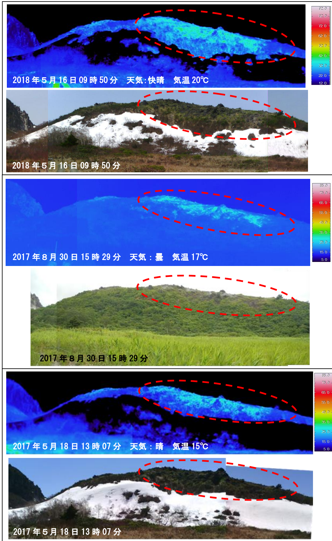
図6 栗駒山 東から撮影したゆげ山の状況と地表面温度分布
